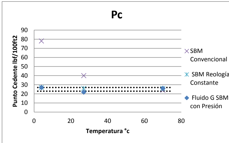
Imagen 3-28: Punto Cedente para los fluidos evaluados con presión
