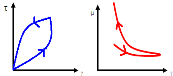
Fig: Curvas de comportamiento reopético (hay histéresis)
