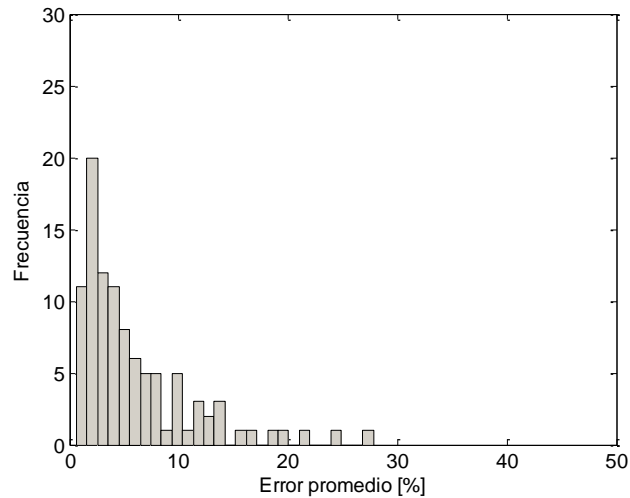
Figura 5.4 Distribución de error relativo promedio después de haber realizado 100 experimentos con radios de cobertura promedio de 100 m y variación de \pm 1\%
