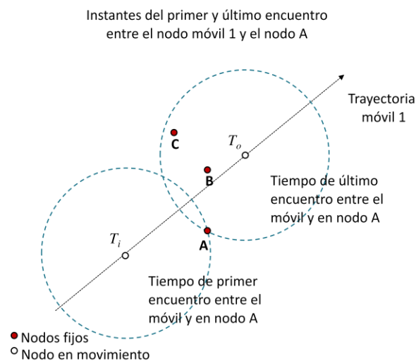
Figura 3.3 Registro de los tiempos en que un nodo en movimiento detecta por primera y por última vez a un nodo estático (en este caso nodo estático A)
