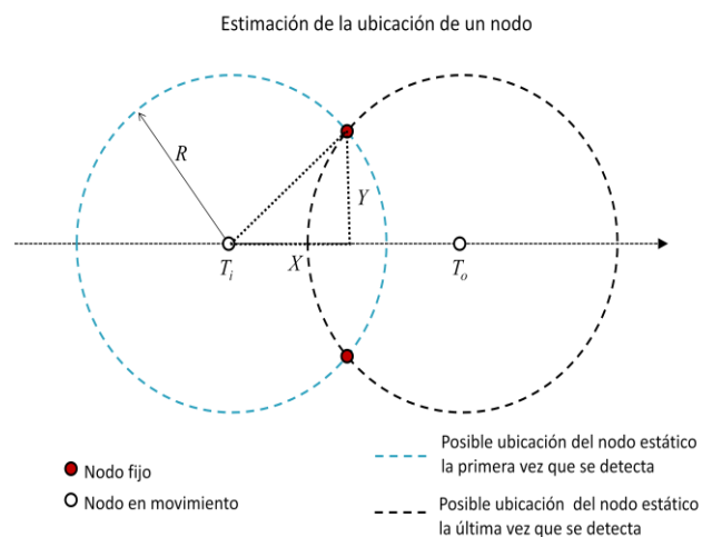
Figura 3.4 Solución geométrica de la ubicación de un nodo fijo calculada por un nodo móvil
