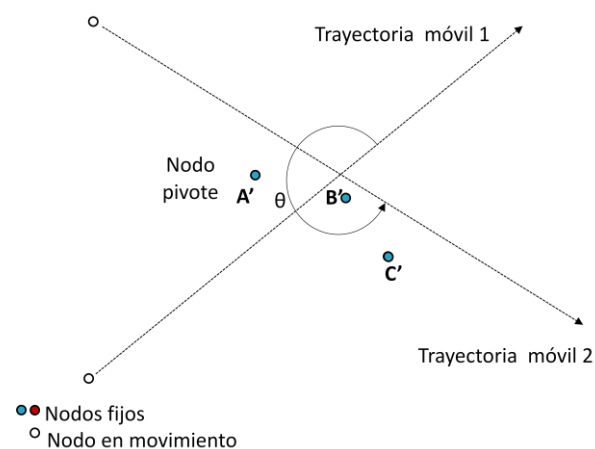
Figura 3.10 Constelación mejorada obtenida al descartar los nodos que no se superponen.
