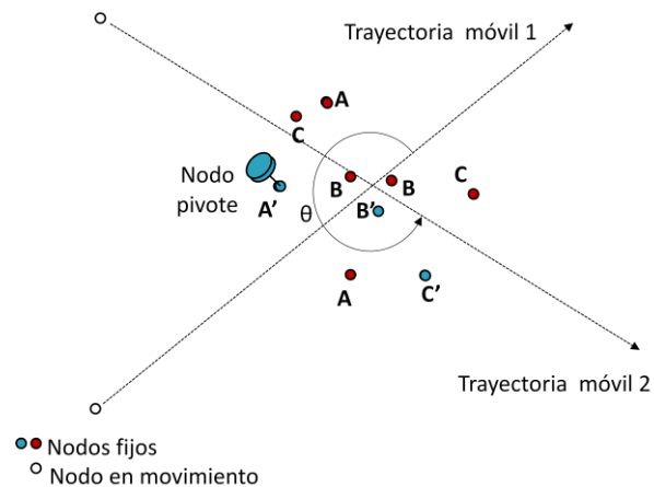
Figura 3.9 Rotación de dos constelaciones superpuestas, tomando como pivote el nodo A' en ambas constelaciones.
