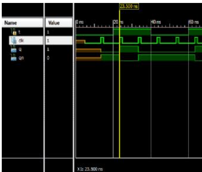
Figura 3.9.12-B Q = complemento de la última Q y Qn = complemento de la última Qn
