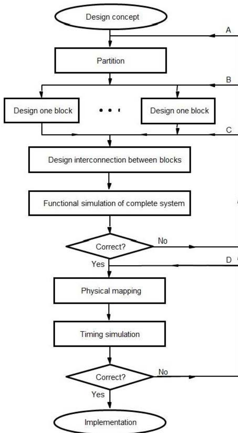
Figura 2.3.1 Flujo de diseño
