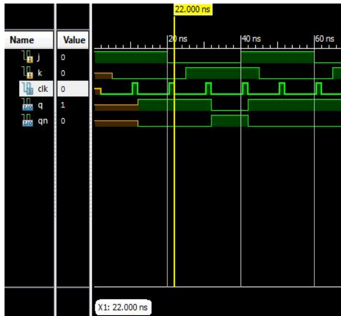
Figura 3.9.10-A Q = \text{ultima } Q y Qn = \text{ultima } Qn
