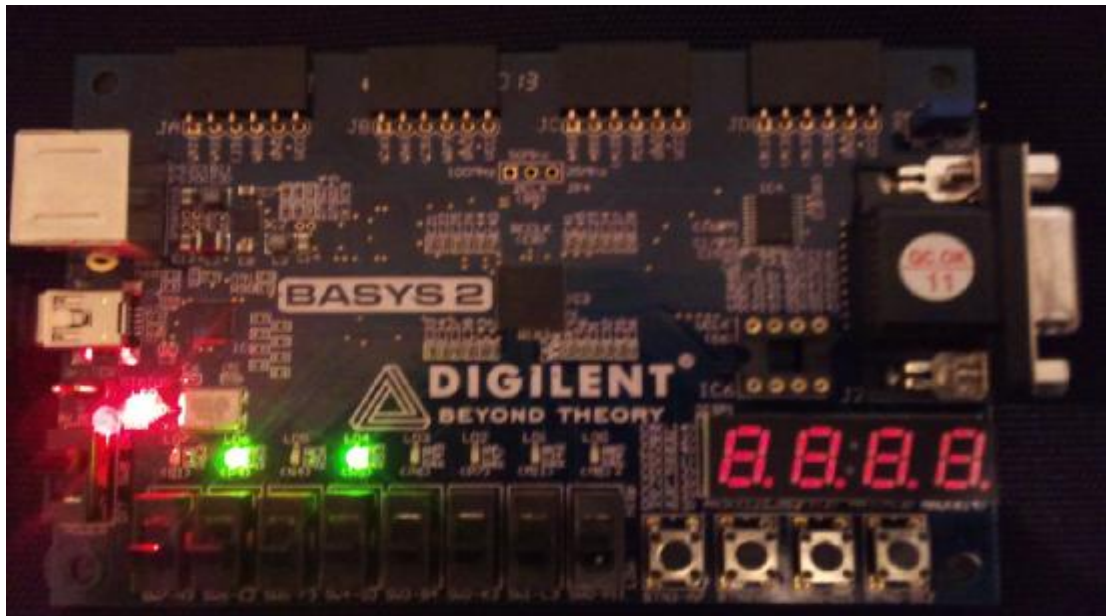
Figura 3.12.14 Tarjeta de prueba, Estado=B, Reset=0.
