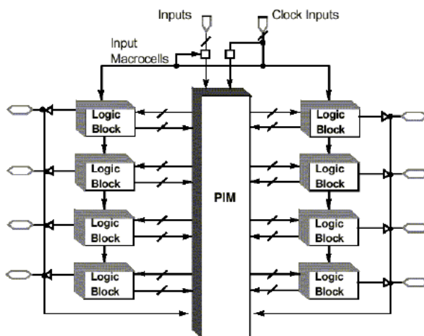
Figura 2.1.5 Arquitectura CPLD
