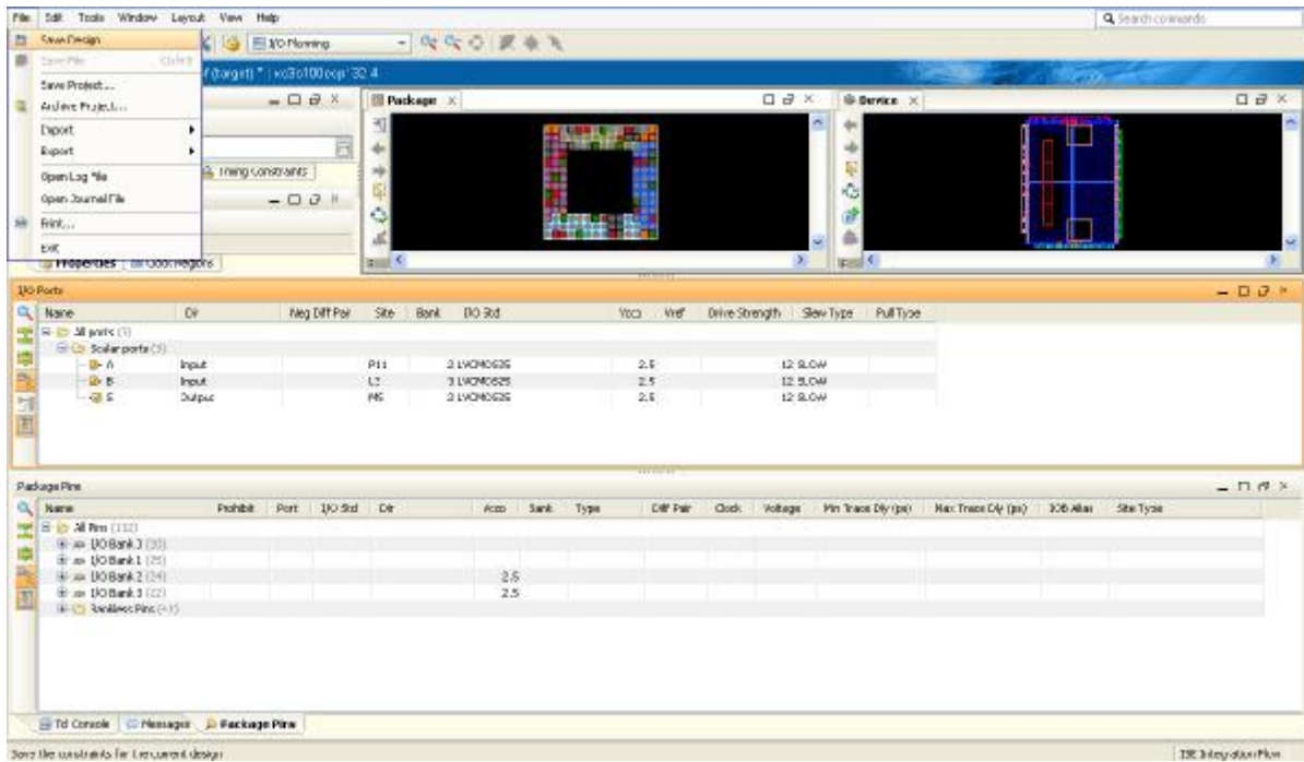
Figura 3.3.7 Guardar diseño.
