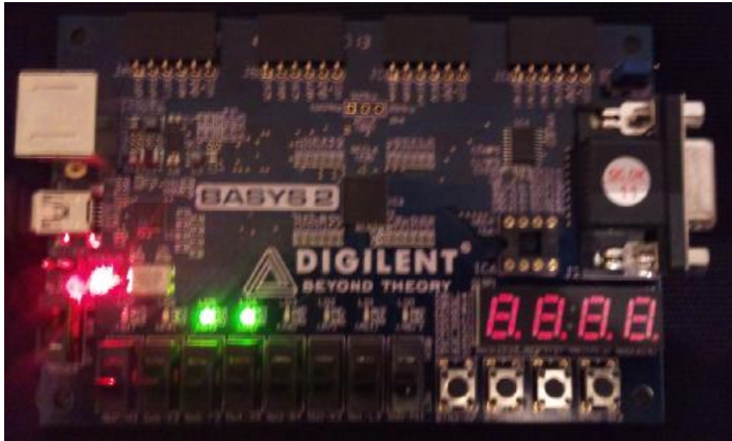
Figura 3.12.13 Tarjeta de prueba, Estado=A, Reset=0.
