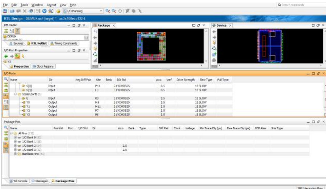
Figura 3.6.35 Asignación de pines I/O DEMUX
