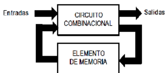
Figura 3.9.1 Sistema Secuencial
