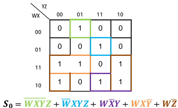
Figura 3.4.9 Simplificación de S_0
