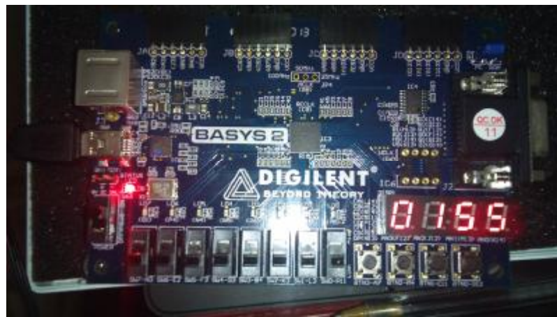
Figura 3.11.15 Contador en 0155
