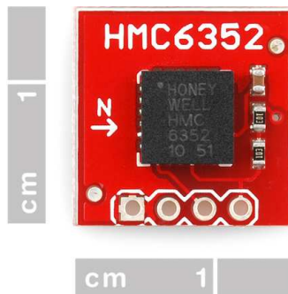
Figura 19. Brújula digital modelo HMC6352 y dimensiones.
