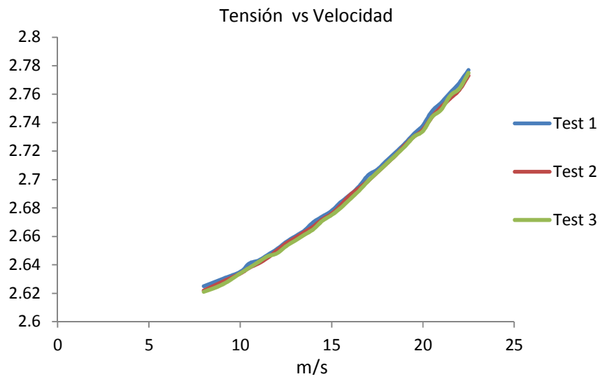
Figura 15. Resultados de caracterización -Tubo de Pitot 3.
