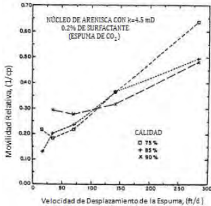
Fig. 3.23 Movilidad relativa para espuma de CO_2 Heller y colaboradores, 1985)
