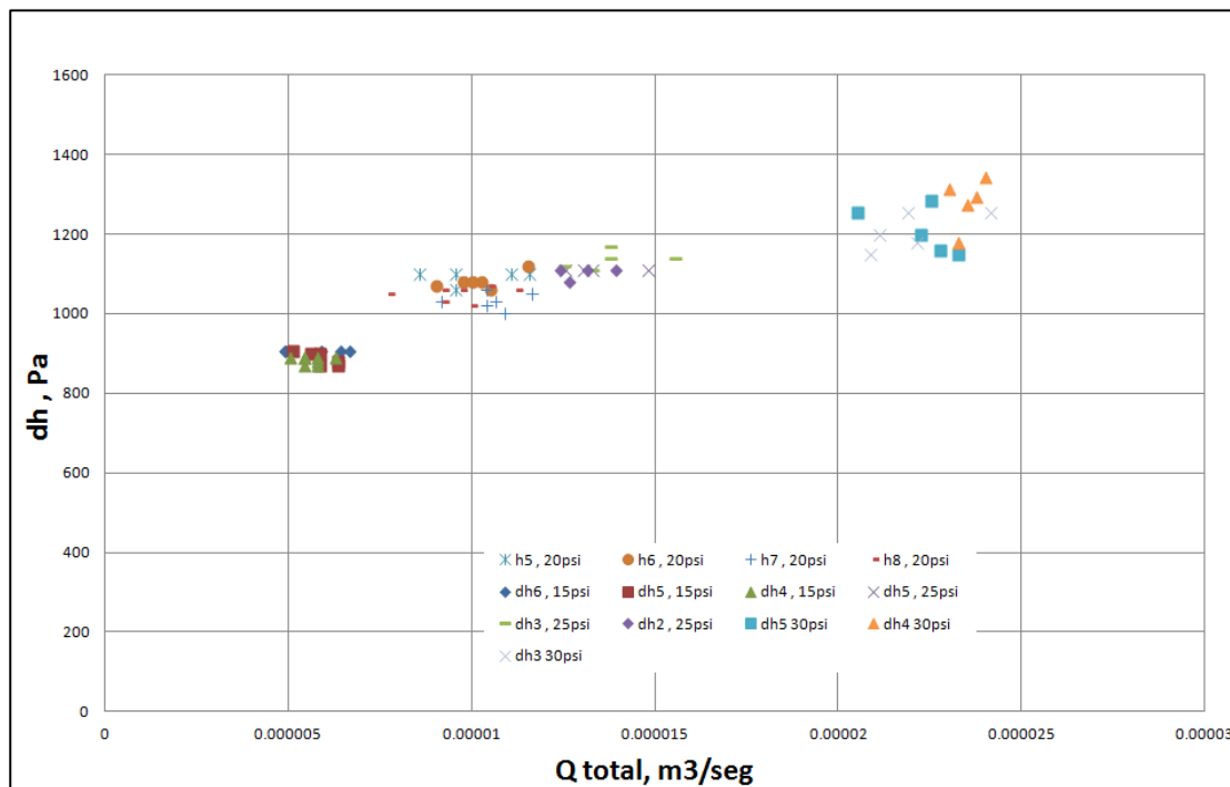
Fig.6.15 Caída de presión para distintos gastos bajo régimen permanente
