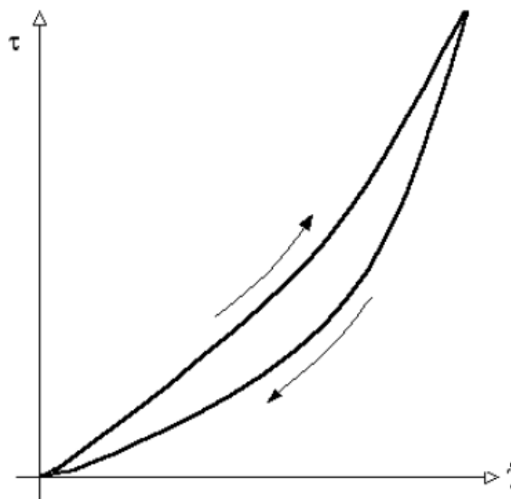
Fig. 5.4 Comportamiento de un fluido reopéctico
