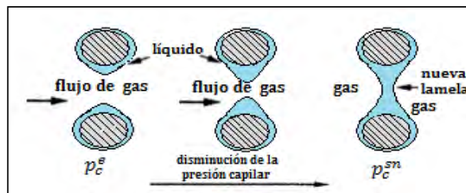
Fig.3.8 Disminución de la presión capilar para la formación de una lamela mediante el mecanismo Snap-off
