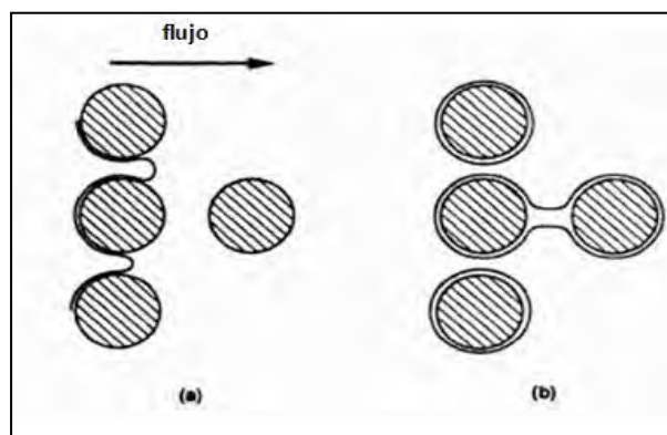
Fig. 3.10 Esquema del mecanismo Leave-behind. (a) Invasión de gas y (b) lamelas estables. (Kovscek & Radke, 1994)
