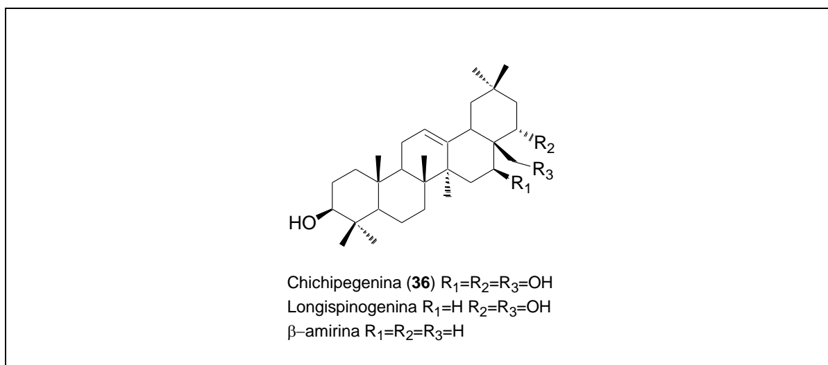
Figura 16. Estructura de chichipegénina, longispinogénina y β-amirina, aislados de diferentes especies de cactáceas.
