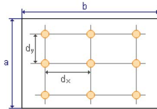
Figura 3. Cálculo de las distancias entre luminarios.
