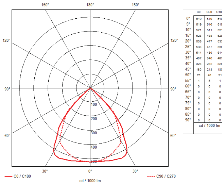
Figura 12 Curva fotométrica.
