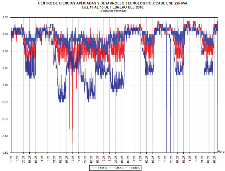
Gráfica 4 Factor de potencia.
