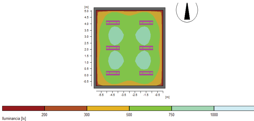
Figura 22 Nivel útil.
