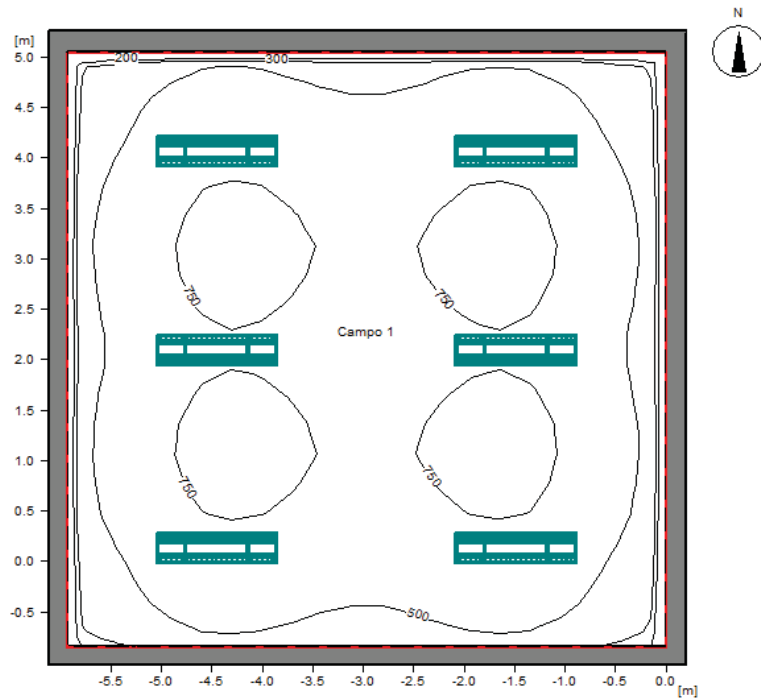
Figura 23 Líneas isométricas.
