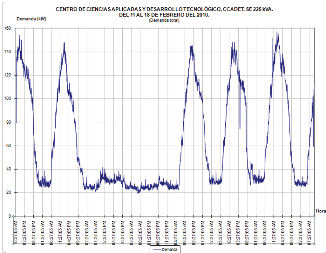
Gráfica 1. Demanda total.
