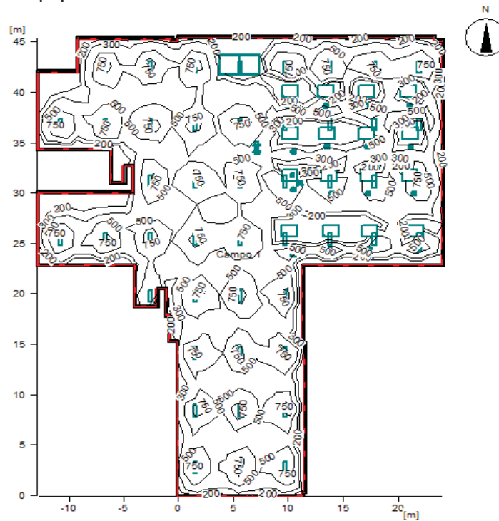
Figura 27 Líneas isométricas.
