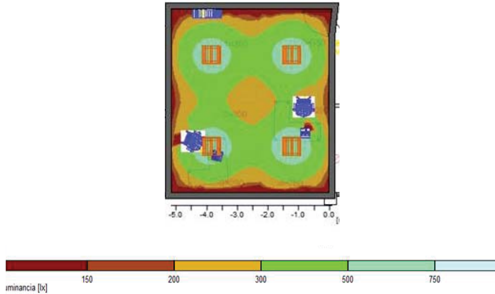
Figura 18 Nivel útil.
