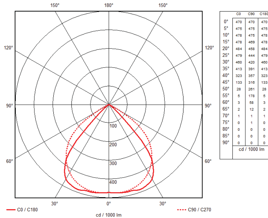
Figura 17 Curva fotométrica.
