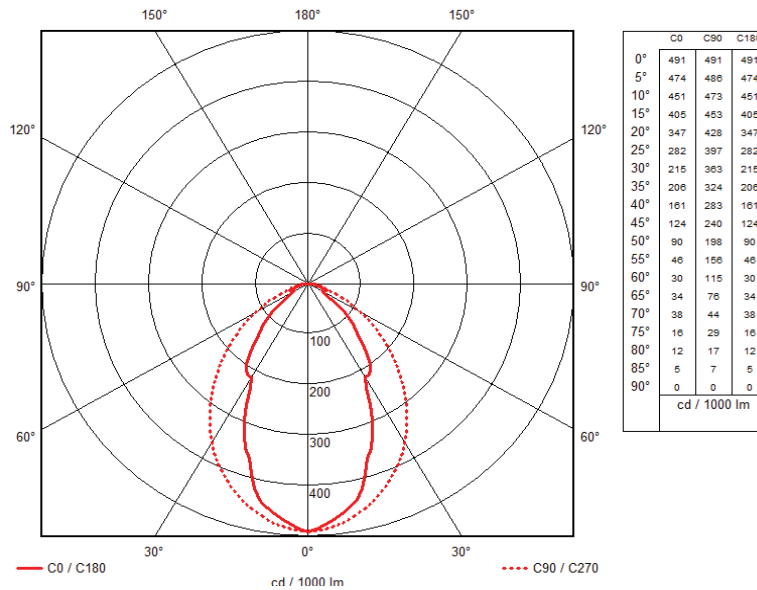
Figura 25 Curva fotométrica.
