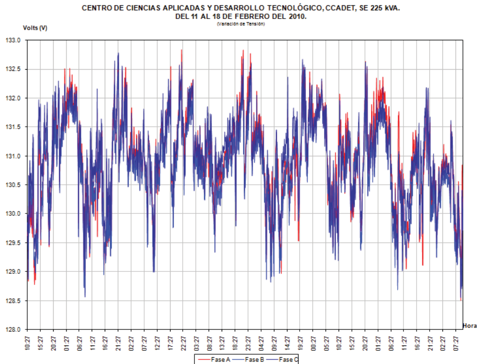
Gráfica 3. Variación de tensión.
