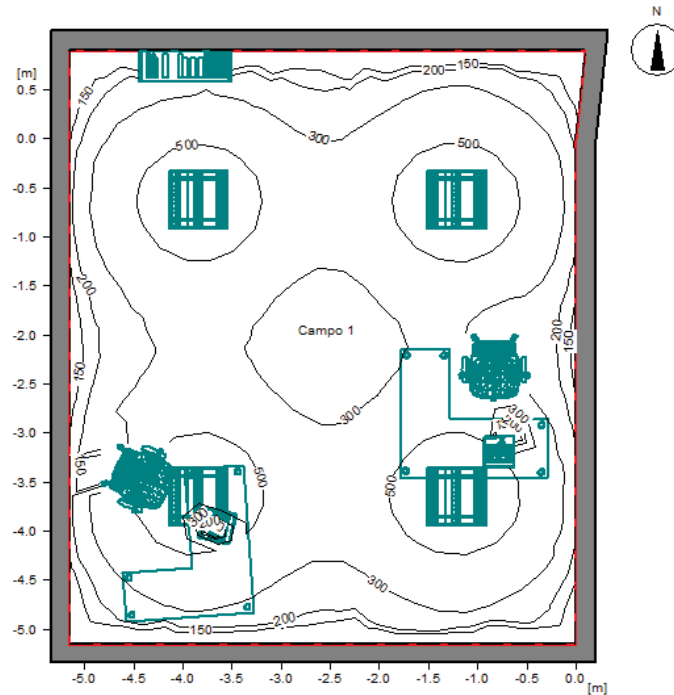
Figura 19 Líneas isométricas.
