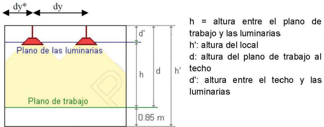
Figura 5 Distancia entre luminarios.
