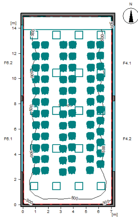
Figura 14 Líneas isométricas
