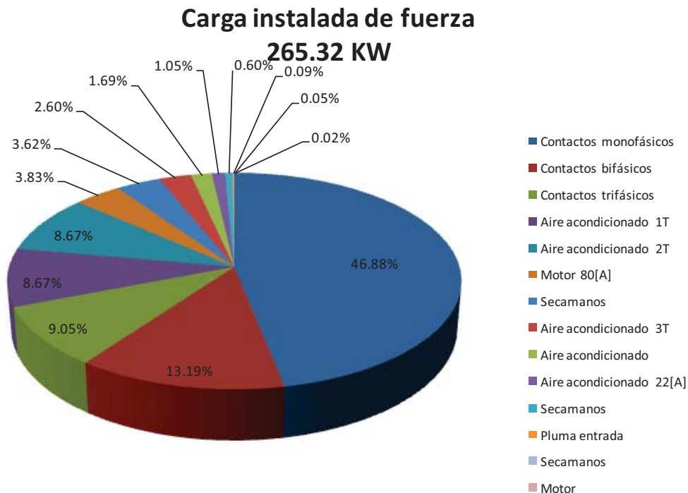
Gráfica 5. Carga instalada en el edificio principal.
