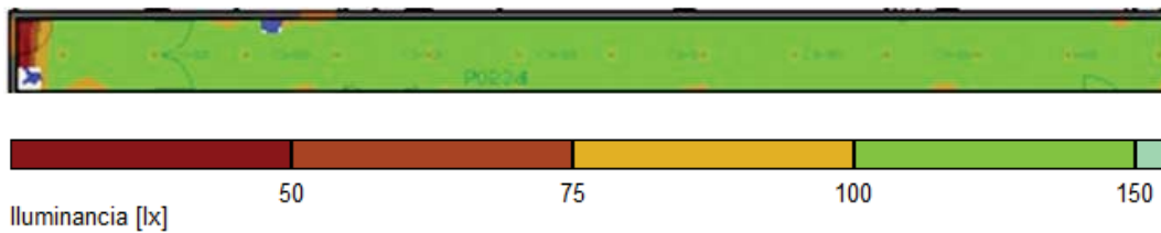
Figura 30 Nivel útil.
