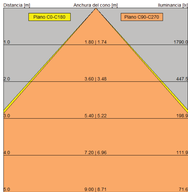
Figura 13 Diagrama cónico
