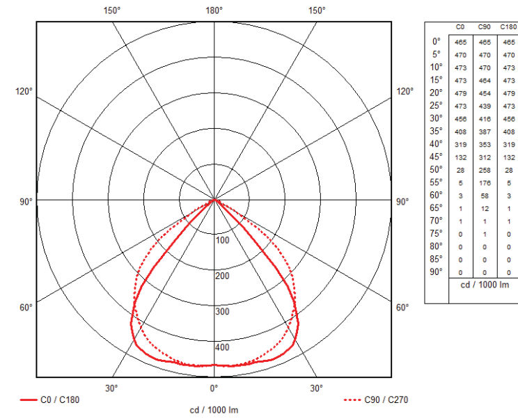
Figura 21 Curva fotométrica
