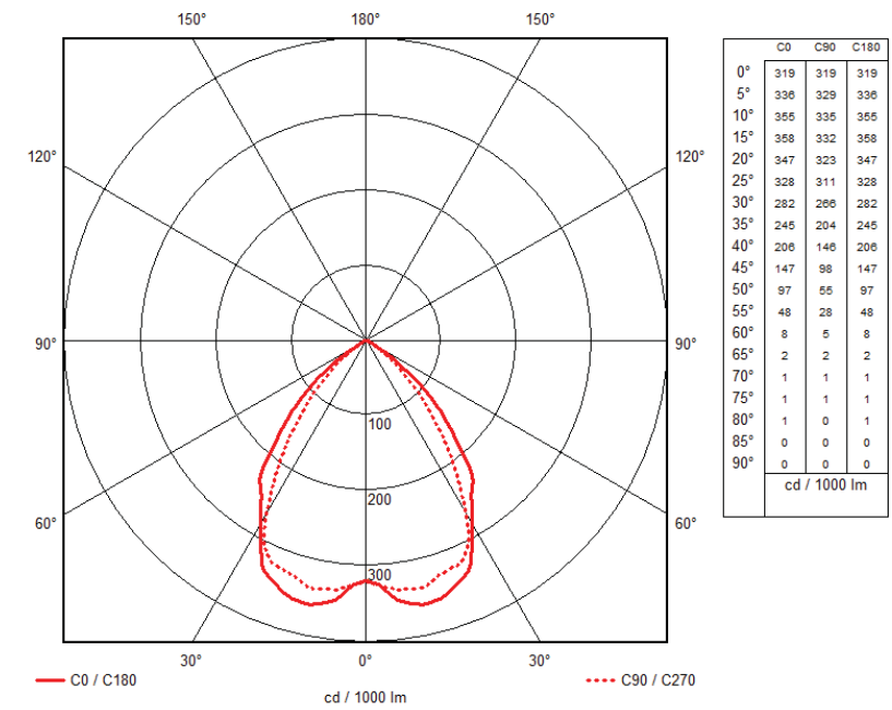
Figura 29 Curva fotométrica.
