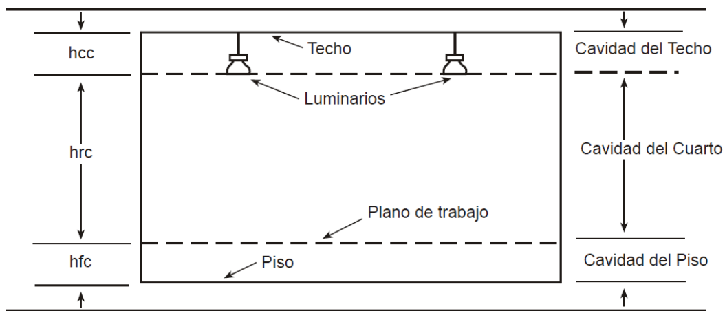
Figura 33 Método de cavidad zonal.
