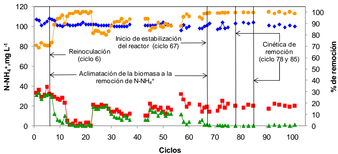
Figura 4. 1 Desempeño del reactor SBR en la etapa 1 – 100 \text{ mg L}^{-1} \text{ N-NH}_4^+ . ( \blacklozenge ) \text{N-NH}_4^+ inicio ciclo, \text{mg L}^{-1} , ( \blacksquare ) \text{N-NH}_4^+ final fase aerobia, \text{mg L}^{-1} , ( \blacktriangle ) \text{N-NH}_4^+ final fase anóxica, \text{mg L}^{-1} , ( \bullet ) \text{N-NH}_4^+ % de remoción.
