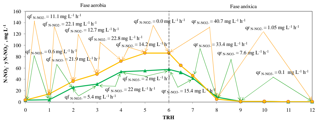
Figura 4. 28 Estudio cinético de remoción, ciclo 207 - etapa 3. (■) N-NH 4 + , mg L -1 , (▲) N-NO 3 - , mg L -1 , (●) N-NO 2 - , mg L -1 .
