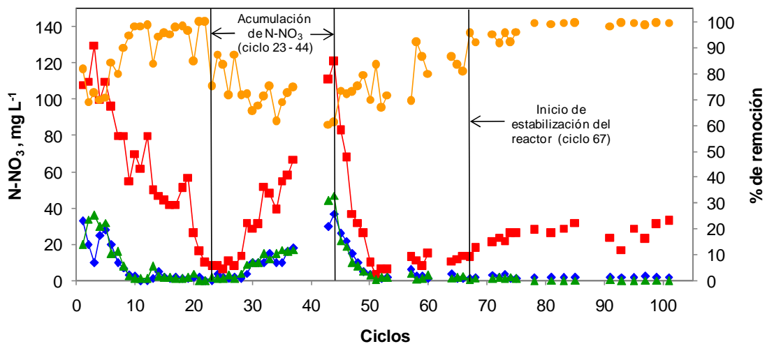
Figura 4. 2 Desempeño del reactor SBR en la etapa 1 – \text{N-NO}_3^- . ( \blacklozenge ) \text{N-NO}_3^- inicio ciclo, \text{mg L}^{-1} , ( \blacksquare ) \text{N-NO}_3^- final fase aerobia, \text{mg L}^{-1} , ( \blacktriangle ) \text{N-NO}_3^- final fase anóxica, \text{mg L}^{-1} , ( \bullet ) \text{N-NO}_3^- % de remoción.
