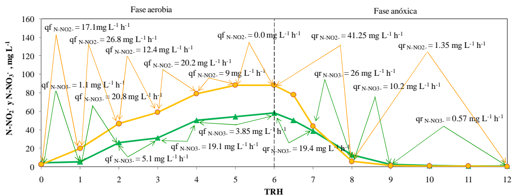
Figura 4. 29. Estudio cinético de remoción, ciclo 219 - etapa 3. (■) \text{N-NH}_4^+ , \text{mg L}^{-1} , (▲) \text{N-NO}_3^- , \text{mg L}^{-1} , (●) \text{N-NO}_2^- , \text{mg L}^{-1} .
