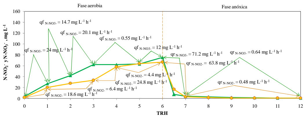
Figura 4. 30. Estudio cinético de remoción, ciclo 273 - etapa 4. (■) \text{N-NH}_4^+ , \text{mg L}^{-1} , (▲) \text{N-NO}_3^- , \text{mg L}^{-1} , (●) \text{N-NO}_2^- , \text{mg L}^{-1} .
