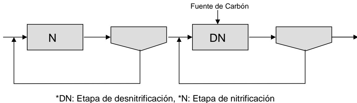
Figura 2. 9 Sistema separado de lodos (Bernet N. y Spérandio M., 2006).
