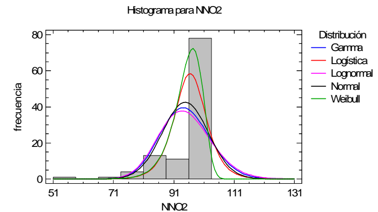
Figura A.1. Ajuste de distribuciones de los datos de operación del SBR
