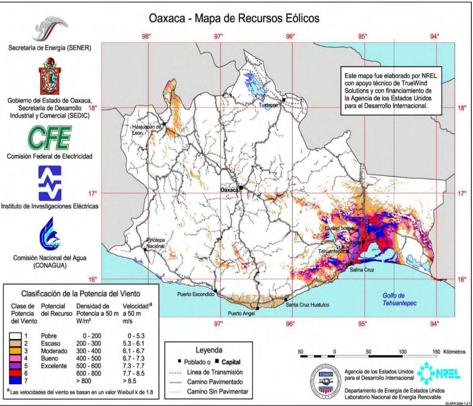
Figura 3.16 Mapa de recursos eólicos del estado de Oaxaca FUENTE: (NREL, 2004)
