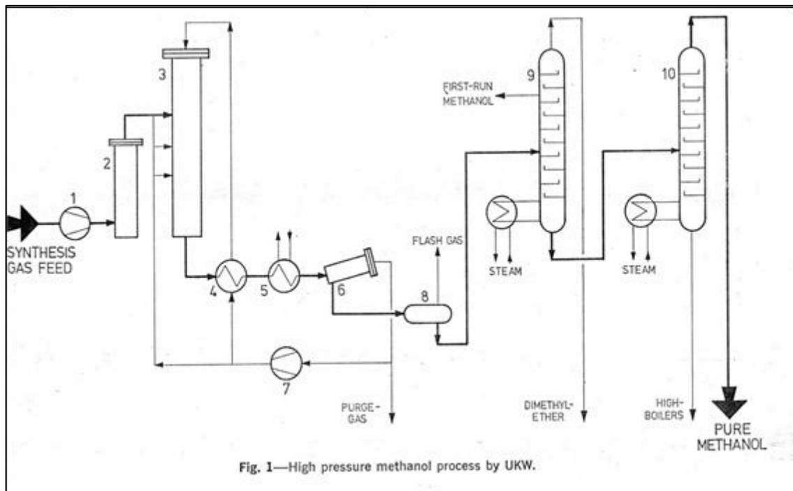
Figura. 5.5 muestra el diagrama de flujo del proceso de síntesis de metanol Unión Rheinische Braunkohlen-AG Kraftstoff (UKW). (fuente Hydrocarbon processing, September 1970, pag 279)
