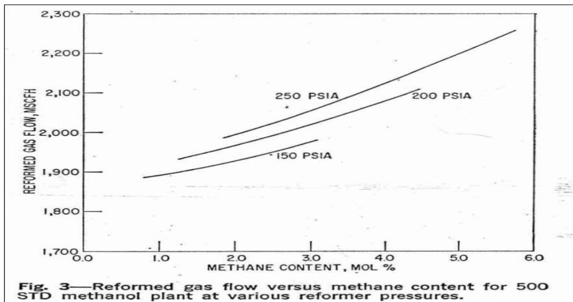
Figura 5.14 Gráfica de flujo de gas vs contenido de metano a varias presiones de reformado (fuente Hydrocarbon processing, March 1969, pag 149)
