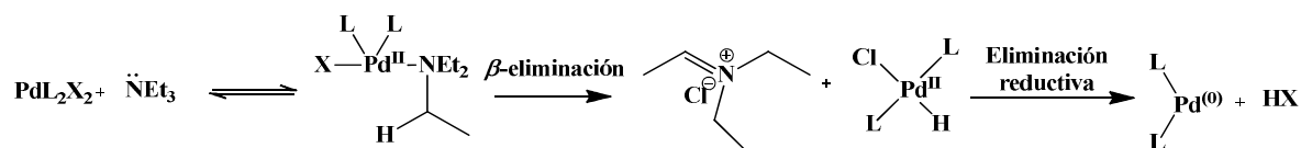
Esquema 16. Regeneración de la especie catalítica. 43
