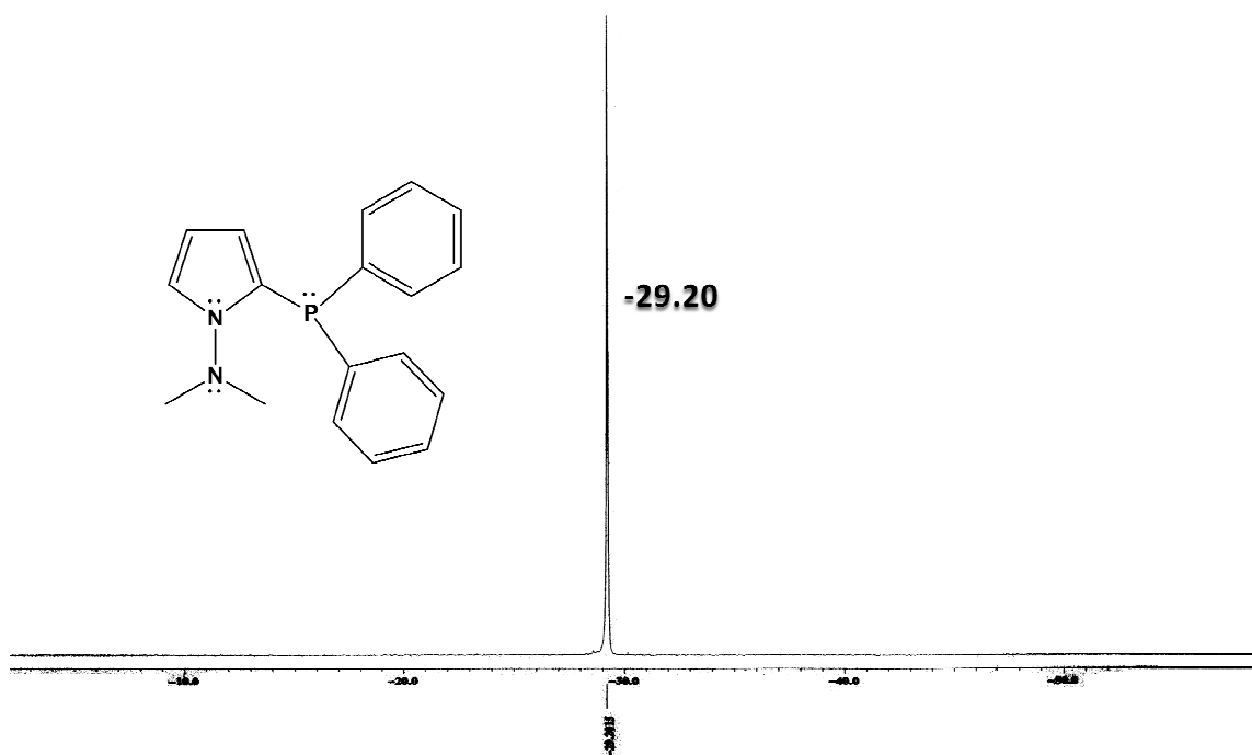
Figura 15. Espectro de RMN ^{31}\text{P} ( \text{CDCl}_3 ) del ligante 1a .
