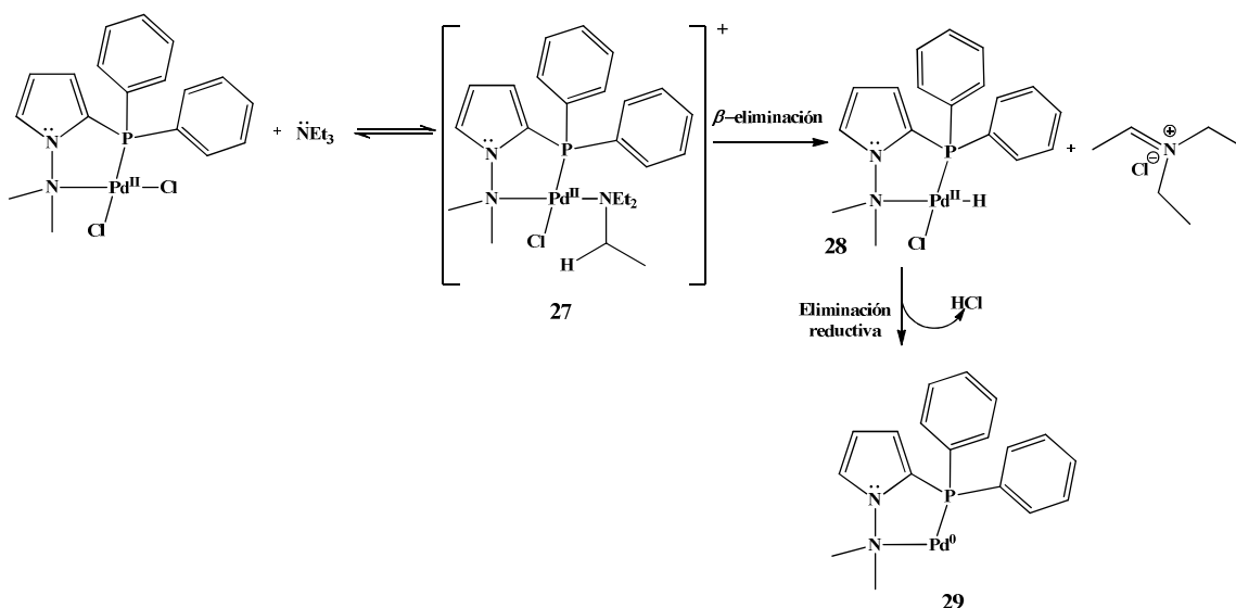
Esquema 29. Generación de la especie activa.
