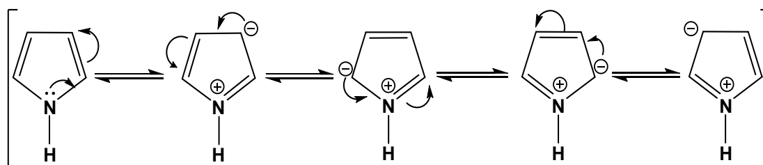
Esquema 5. Estructuras de resonancia del pirrol.
