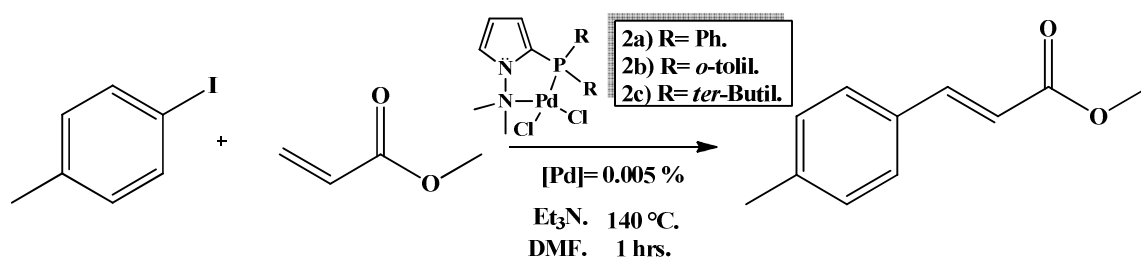
Esquema 28. Condiciones de la reacción modelo tipo Heck.
