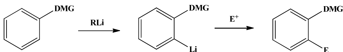
Esquema 8. Reacción de orto metalacion.
