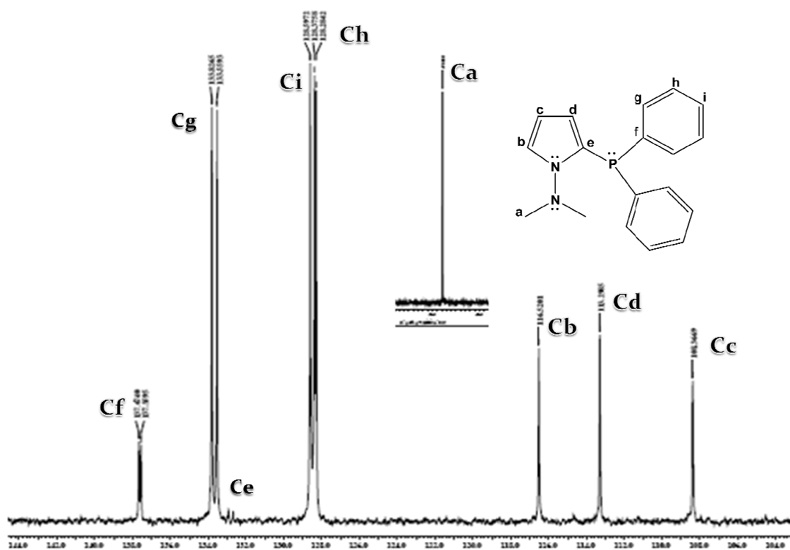
Figura 14. Espectro de RMN ^{13}\text{C} ( \text{CDCl}_3 ) del ligante 1a .
