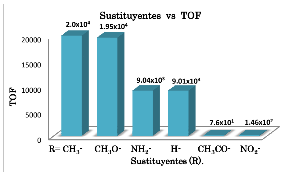
Grafico 6. Variación del sustituyente vs TOF.
