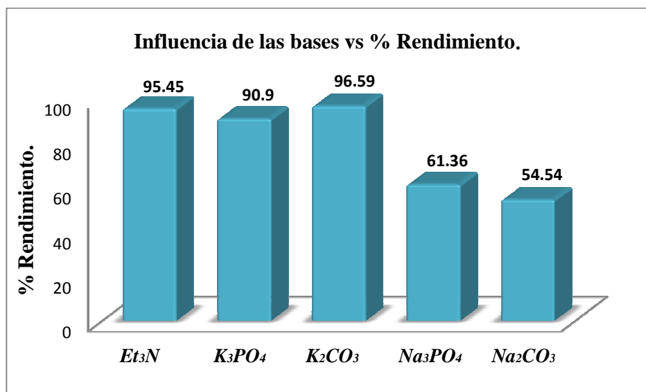
Grafico 3. Dependencia del rendimiento con respecto a la base empleada.
