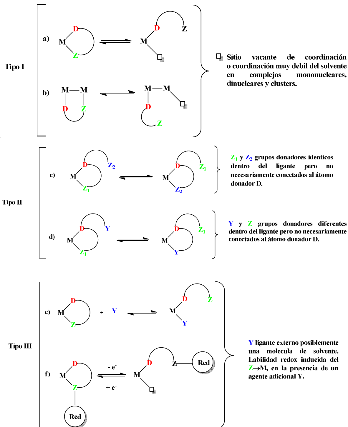
Esquema 3. Tipos de hemilabilidad. El tipo III se extiende a complejos dinucleares o clusters.
