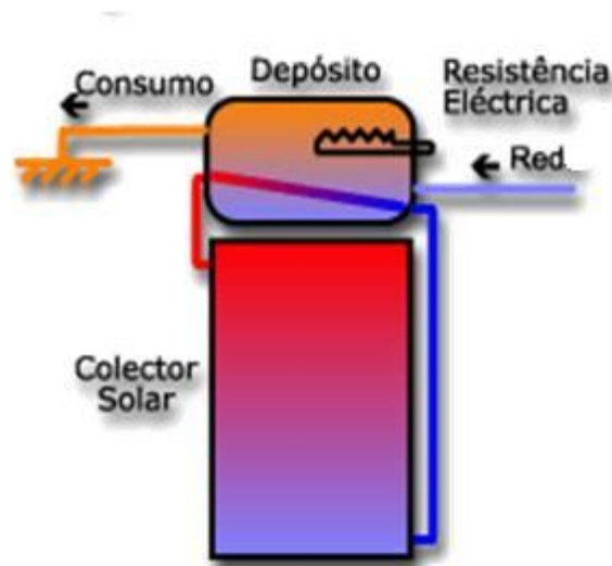
Figura 2.5 Esquema de circulación natural. Fuente: adaptado de [20]
