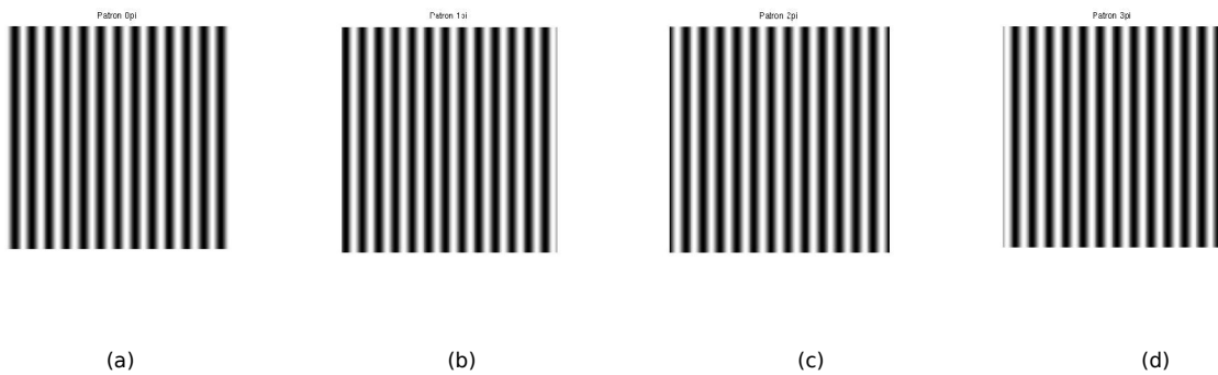
Fig. 3.8. Patrones generados numéricamente con \alpha_1 = 0 , \alpha_2 = 1/2\pi , \alpha_3 = \pi y \alpha_4 = 3/2\pi de escalonamiento de fase (a), (b), (c), (d) respectivamente.
