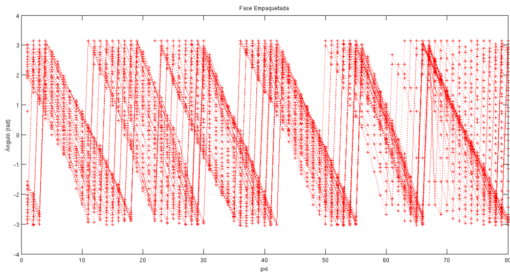
Fig. 4.13. Gráfica de fase empaquetada.
