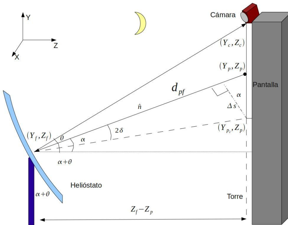
Fig. 3.9. Arreglo geométrico característico del campo de pruebas de helióstatos.
