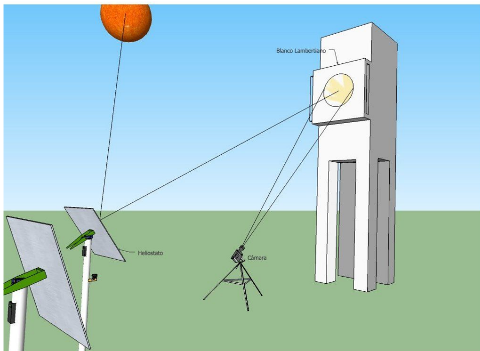
Fig. 3.2 Arreglo para prueba de proyección solar.
