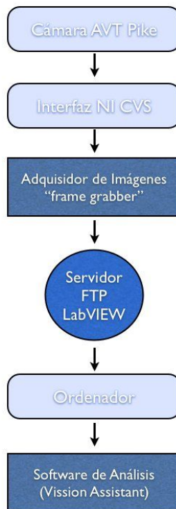
Fig. 3.6. Diagrama de flujo para adquisición de imágenes con cámara AVT Pike.
