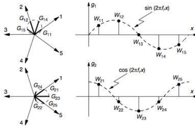
Fig. 2.10. Algoritmo de cinco muestreos para medir la fase.
