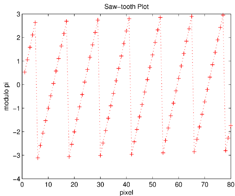
Fig. 2.11. Valores de fase empacada para un patrón teórico de franjas.
