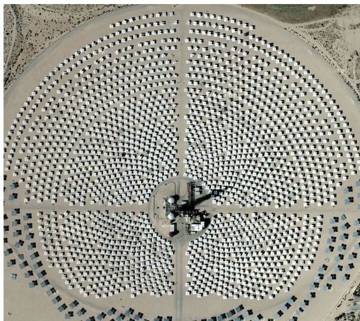
Fig. 1.6. Vista aérea de la planta termo solar Solar Two en Barstow, California.
