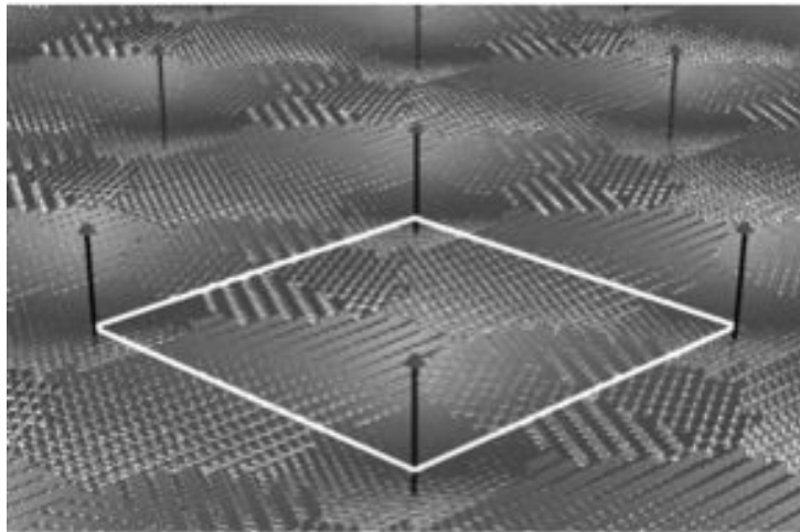
Fig. 1.12. Arreglo teórico de un campo de heliostatos Multi-Torre.
