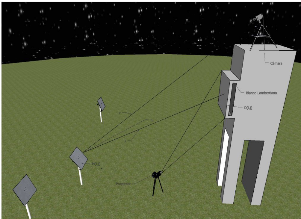
Fig. 3.4. Arreglo para prueba de deflectometría.
