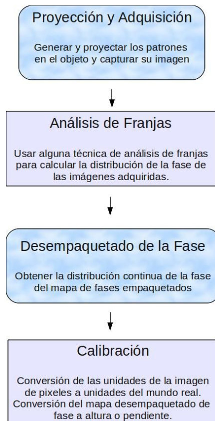
Fig. 2.2 Diagrama de flujo para el proceso de análisis de franjas.
