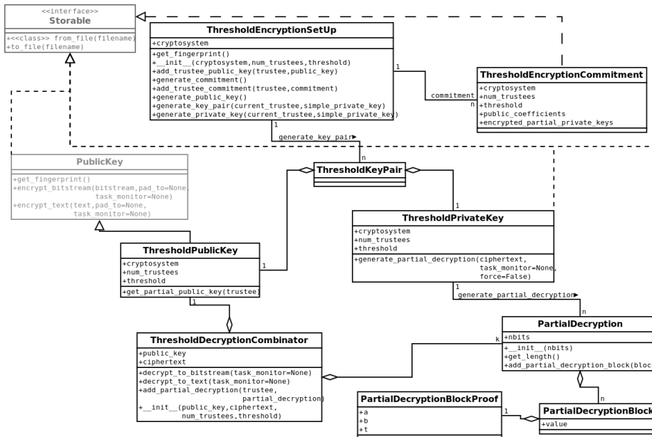
Figura 3.3.1: Diagrama de clases simplificado para ElGamal de umbral en PloneVoteCryptoLib
