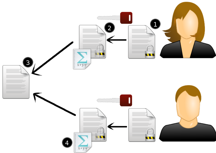
Figura 3.1.3: Descifrado distribuido en un esquema de umbral 2 de 3.
