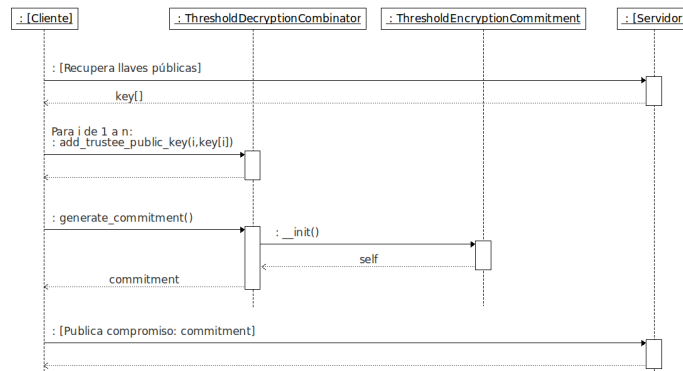
Figura 3.3.2: Diagrama de interacción de clases para generación de compromisos
