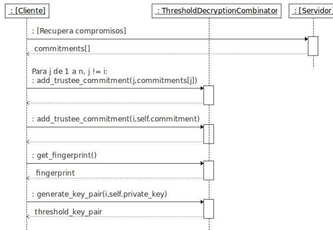
Figura 3.3.3: Diagrama de interacción de clases para generación de par de claves de umbral
