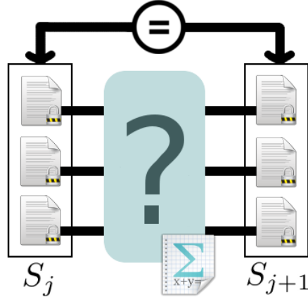
Figura 4.1.2: Objetivos de un proceso de mezcla verificable.
