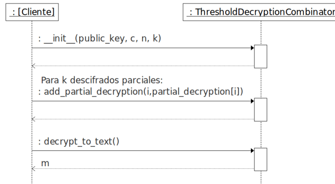
Figura 3.3.4: Diagrama de interacción de clases para la combinación de descifrados parciales
