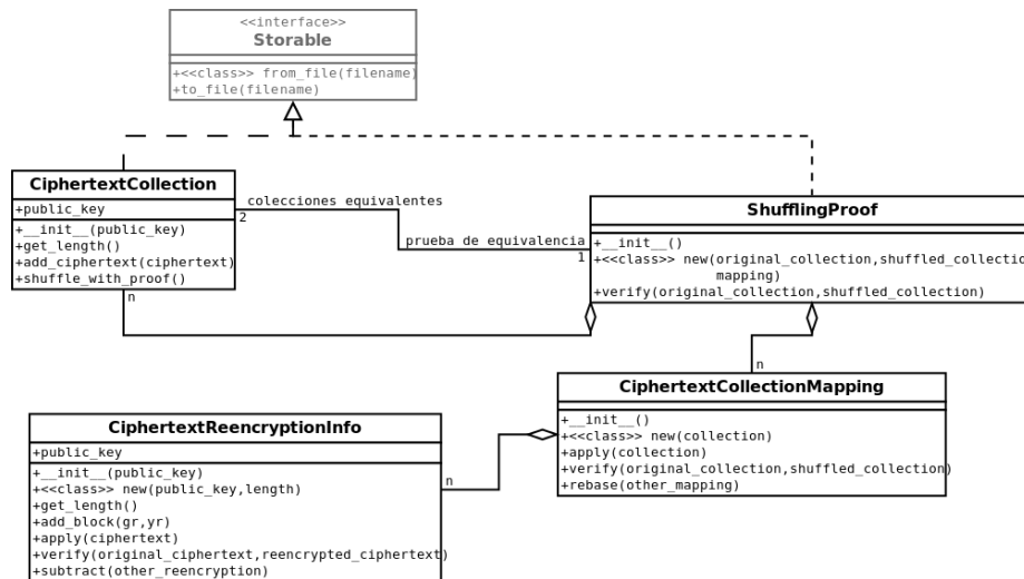
Figura 4.3.1: Diagrama de clases simplificado para soporte de mezclas verificables por recifrado en ElGamal en PloneVoteCryptoLib
