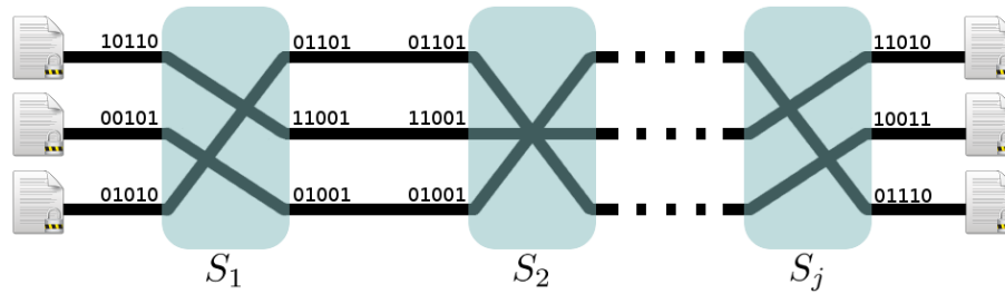
Figura 4.1.1: Esquema general de una red de mezcla.
