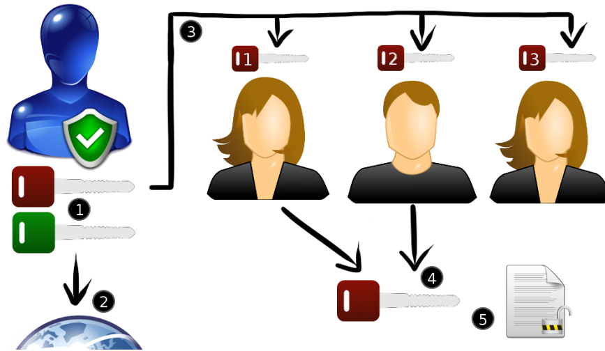
Figura 3.1.1: Compartición de llaves con umbral 2 de 3, usando un agente confiable.
