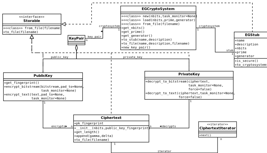
Figura 2.3.1: Diagrama de clases simplificado para ElGamal en PloneVoteCryptoLib
