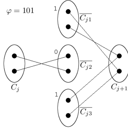
Figura 4.2.1: Ejemplo de asociaciones reveladas en nuestra prueba en conocimiento cero de C_j \approx_S C_{j+1} .
