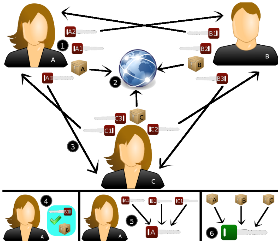
Figura 3.1.2: Compartición de llaves con umbral 2 de 3, mediante un protocolo distribuido seguro.
