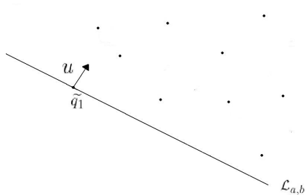
Figura 3.2: Un vector u tal que \langle \tilde{q}_1 - \tilde{q}_l, u \rangle > 0 .
