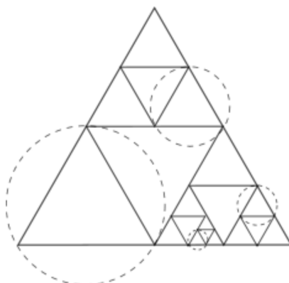
Figura 4.1: Vecindades de puntos que no son vértices.
