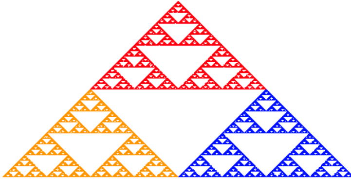
Figura 5.2: Imagen del triángulo de Sierpinski bajo alguna de las tres contracciones.
