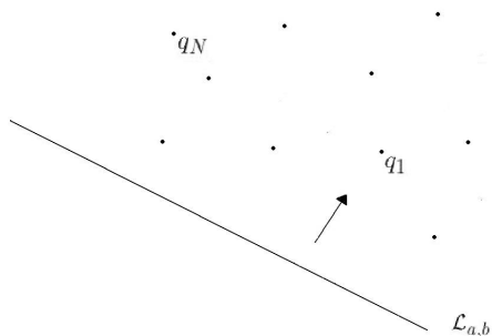
Figura 3.1: La recta \mathcal{L}_{a,b} toca a lo más un punto del conjunto Q .
