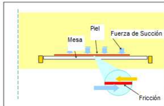
(figura 4.3.-. Descripción de las fuerzas actuantes sobre el plano de trabajo)
