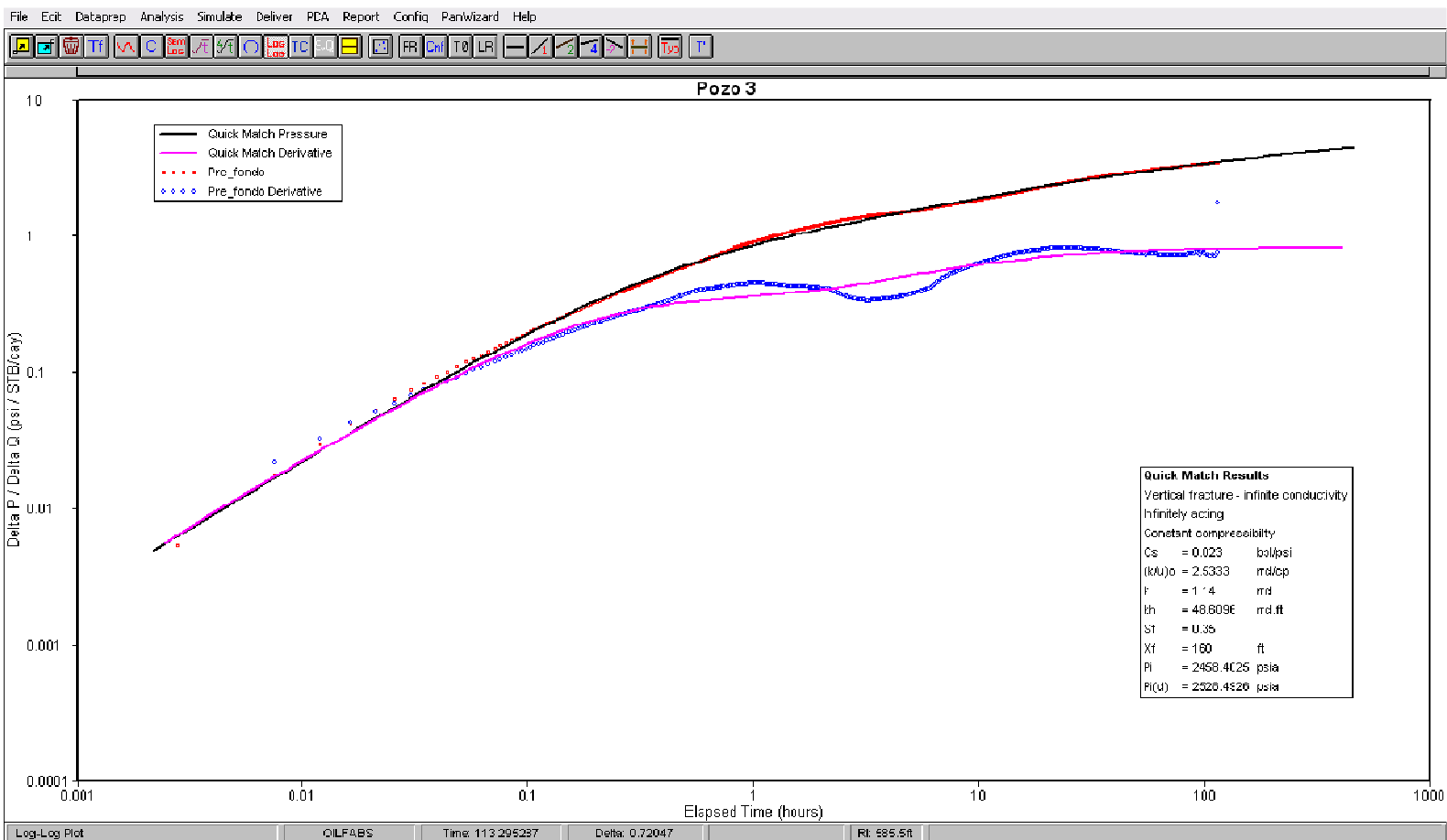
Figura 3.8 (Continuación) – Ajuste de la prueba de presión para el Pozo 3
