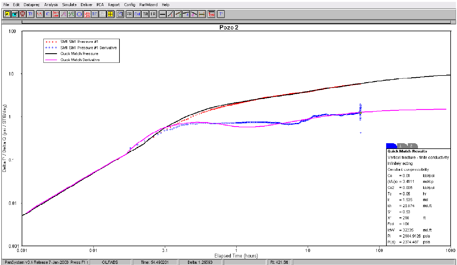
Figura 3.5 (Continuación) – Ajuste de la prueba de presión para el Pozo 2
