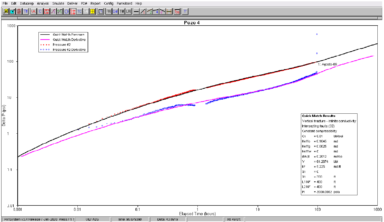
Figura 3.12 (Continuación) – Ajuste de la prueba de presión para el Pozo 4
