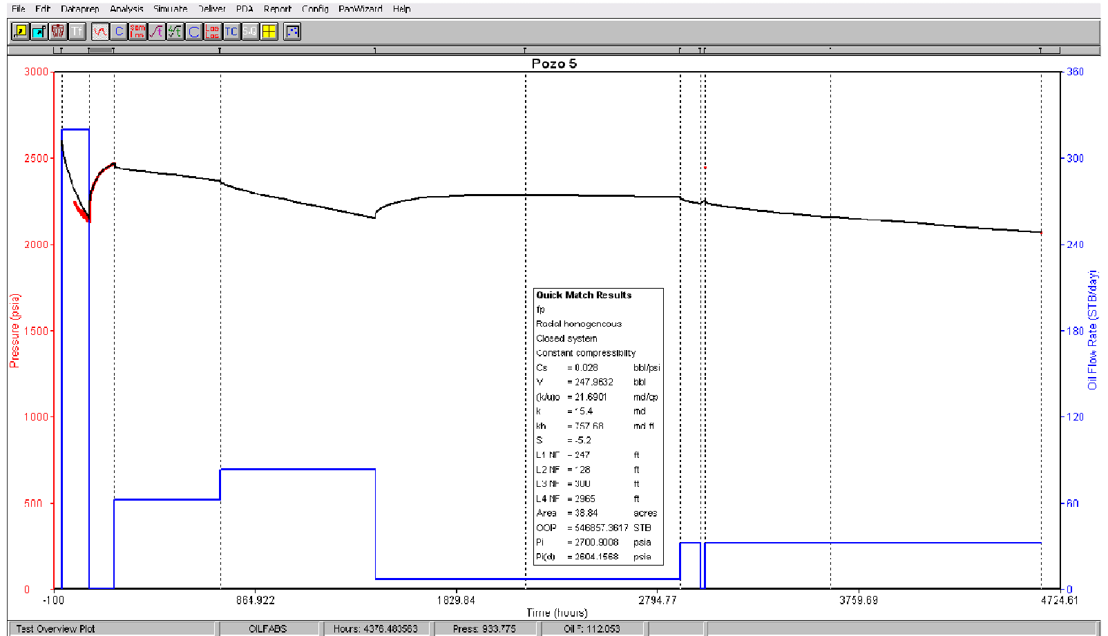
Figura 3.14 – Ajuste de la prueba de presión para el Pozo 5
