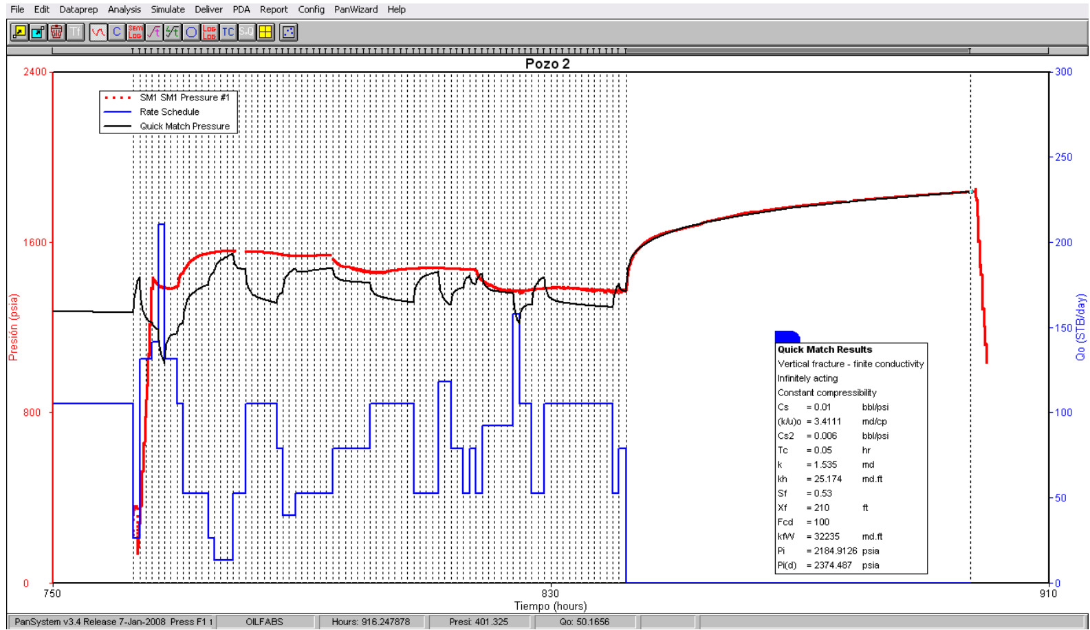
Figura 3.4 – Ajuste de la prueba de presión para el Pozo 2
