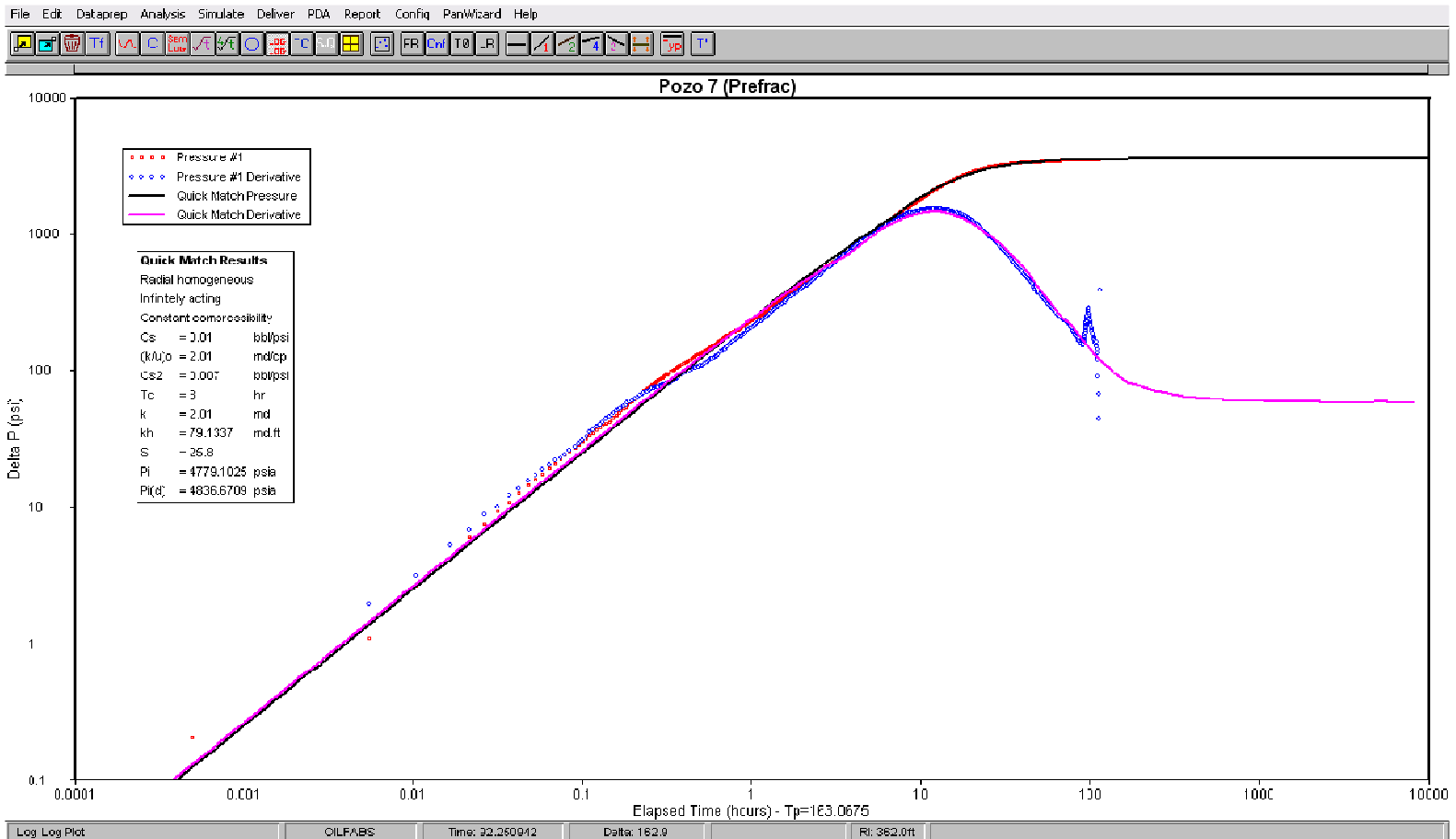
Figura 3.20 (Continuación) – Ajuste de la prueba de presión para el Pozo 7
