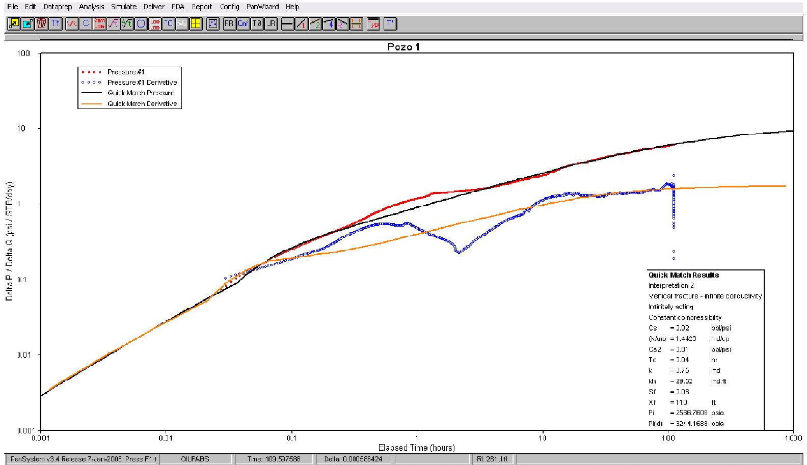
Figura 3.2 (Continuación) – Ajuste de la prueba de presión para el Pozo 1
