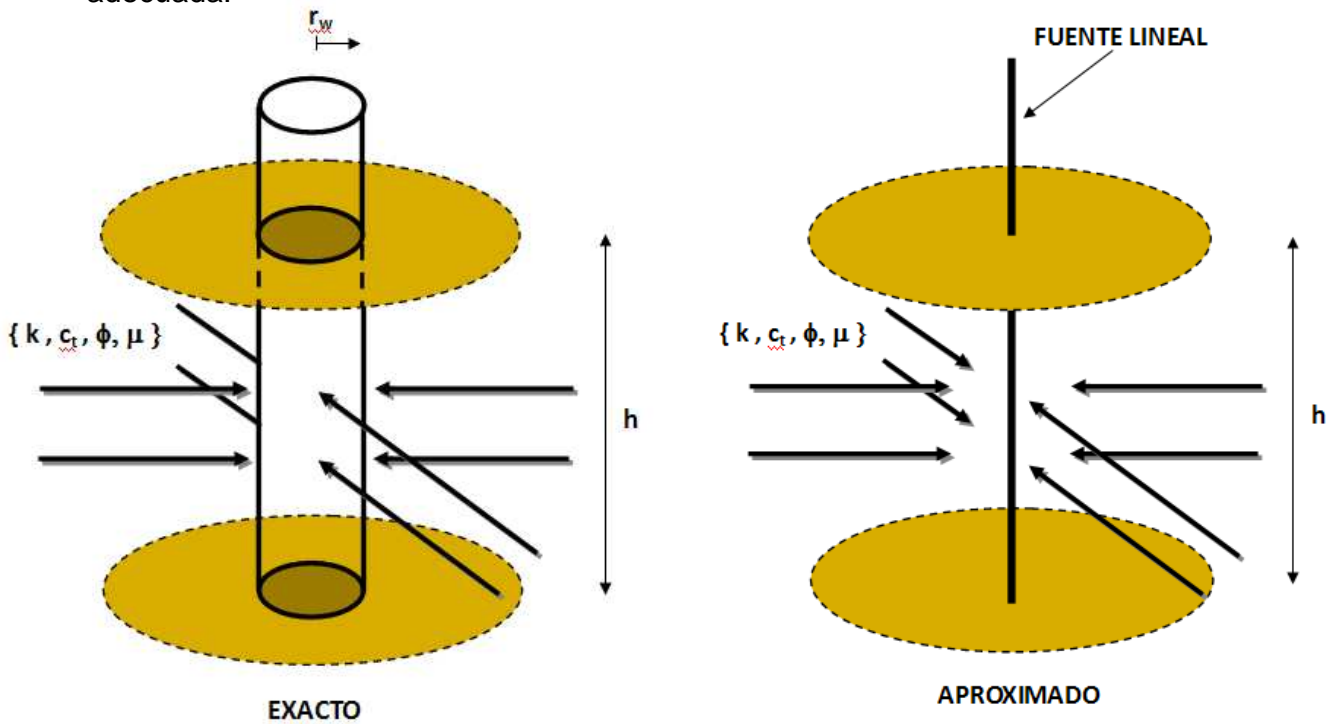
Figura 1.19 – Simplificación del modelo de flujo radial
