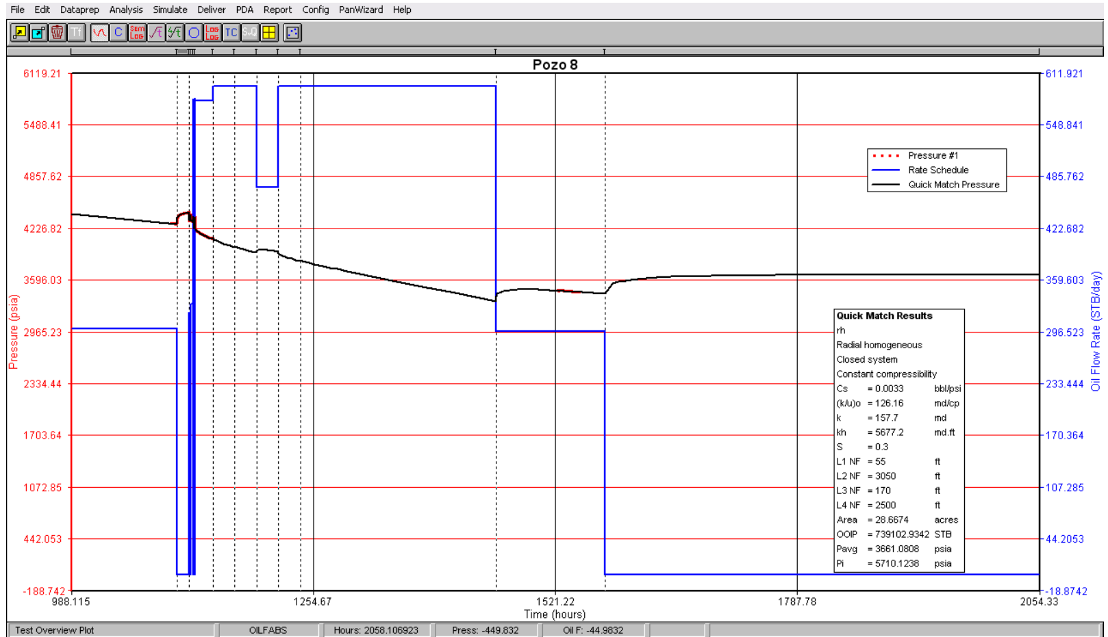
Figura 3.22 – Ajuste de la prueba de presión para el Pozo 8
