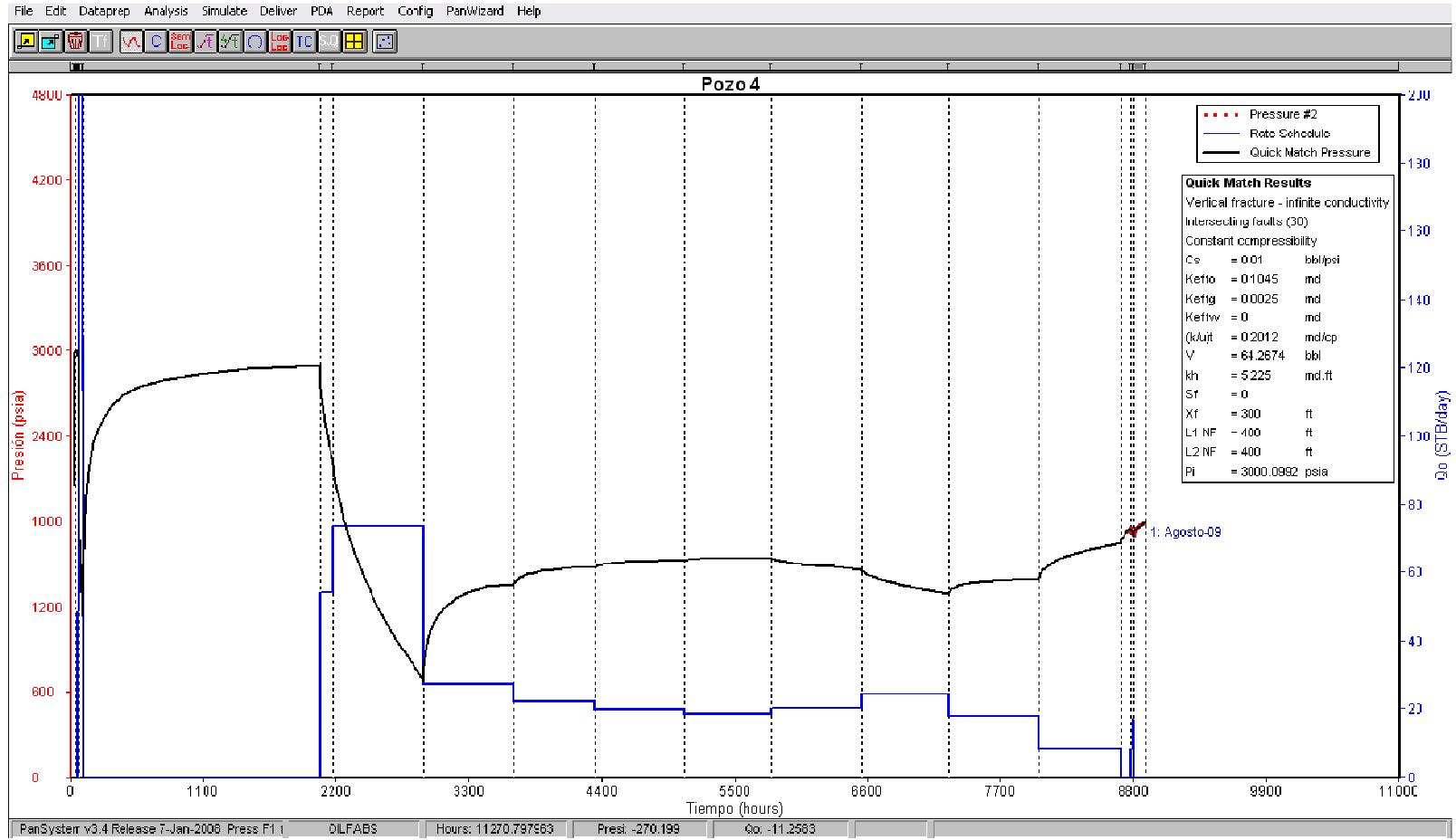
Figura 3.10 – Ajuste de la prueba de presión para el Pozo 4
