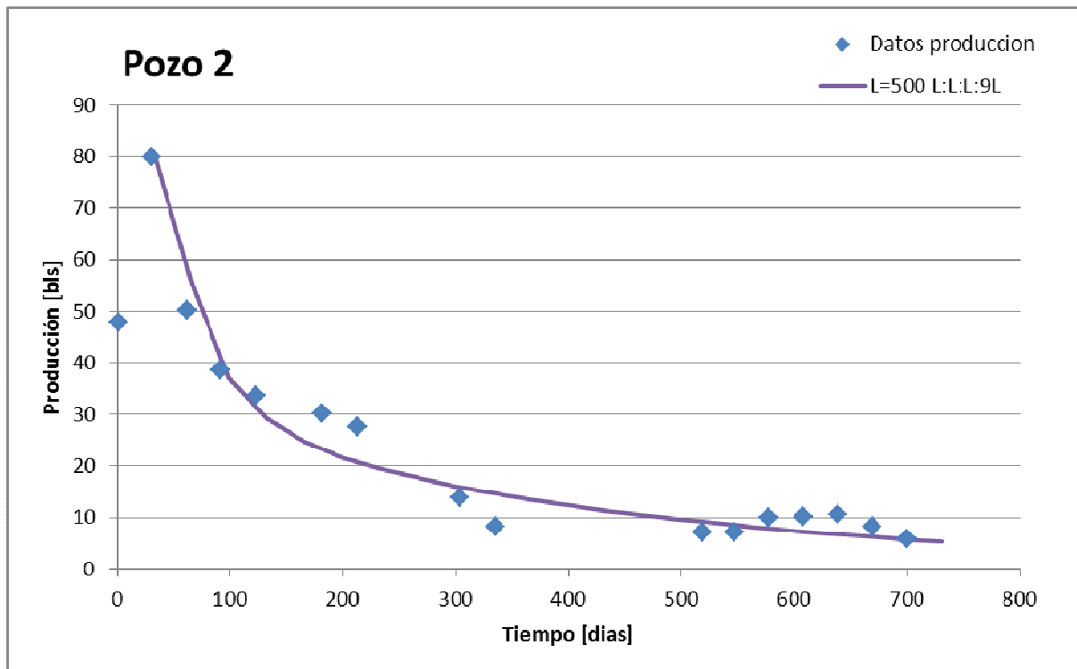
Figura 4.6 – Ajuste del pronóstico con el historial de producción
