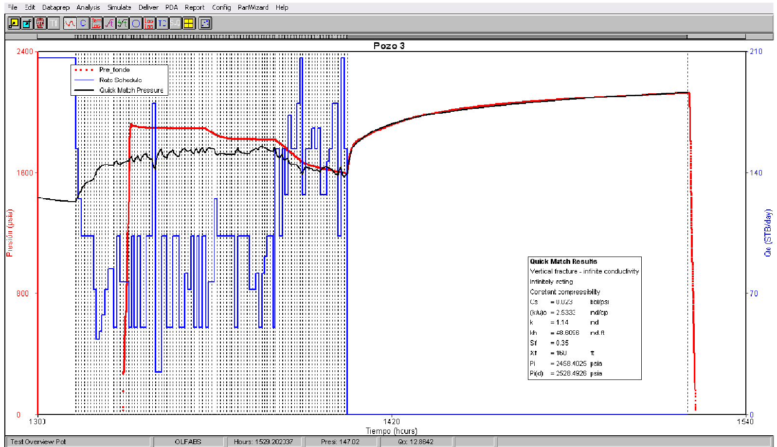
Figura 3.7 – Ajuste de la prueba de presión para el Pozo 3
