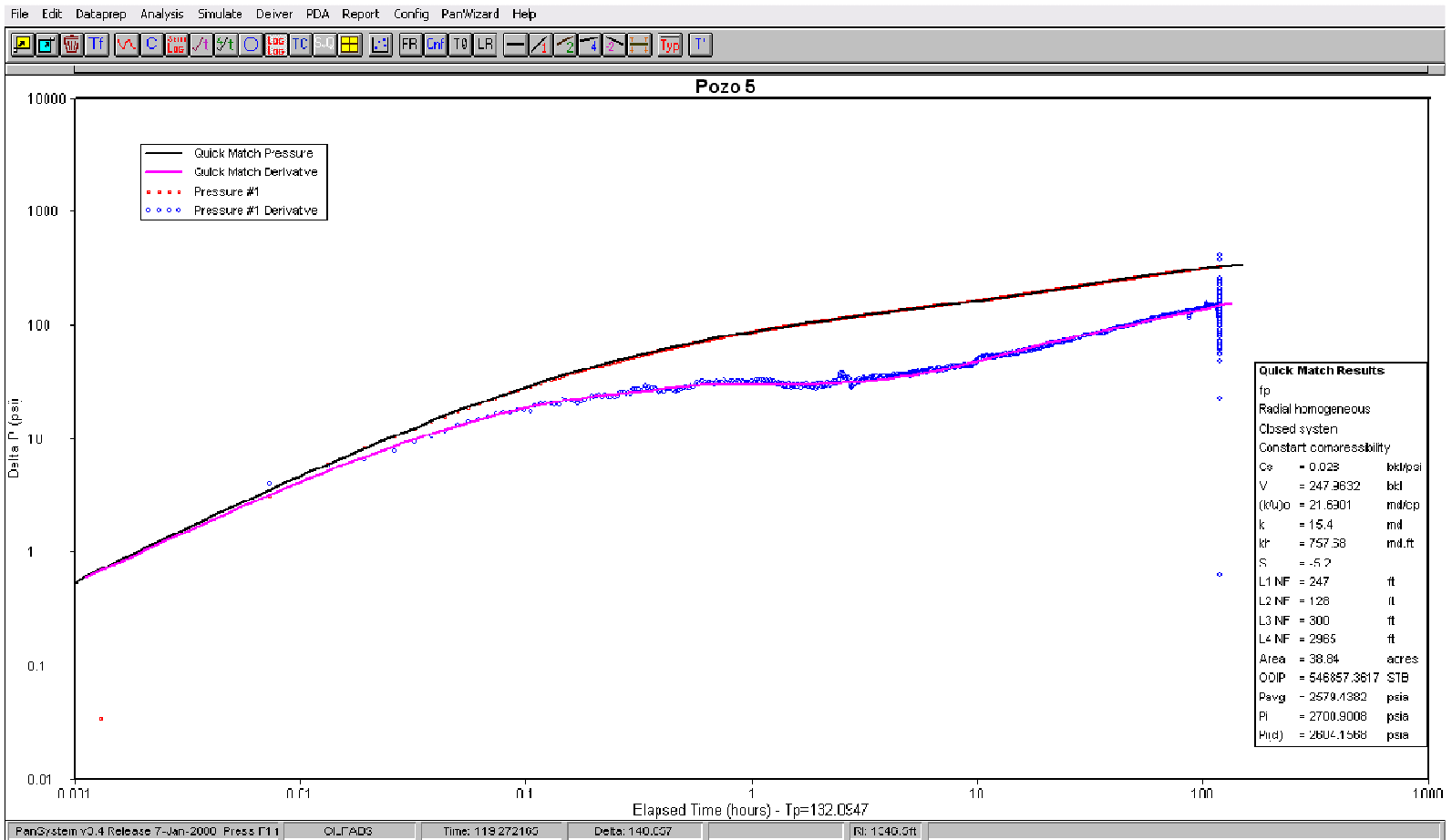
Figura 3.15 (Continuación) – Ajuste de la prueba de presión para el Pozo 5
