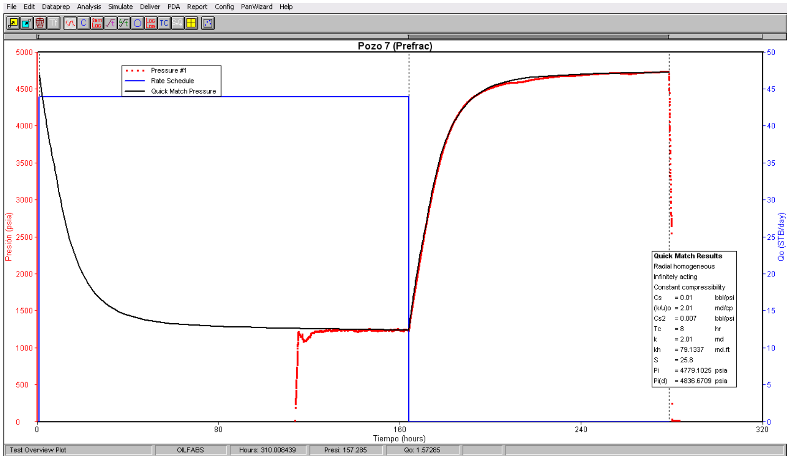
Figura 3.19 – Ajuste de la prueba de presión para el Pozo 7
