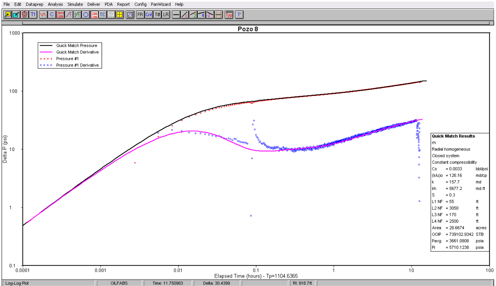
Figura 3.23 (Continuación) – Ajuste de la prueba de presión para el Pozo 8
