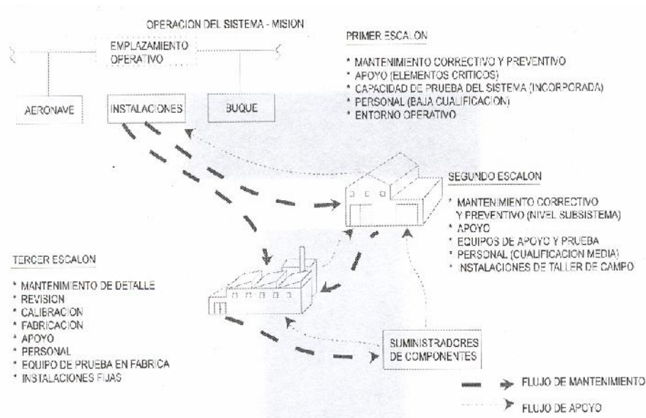
FIGURA 4. OPERACIÓN DEL SISTEMA Y FLUJO DE MANTENIMIENTO
