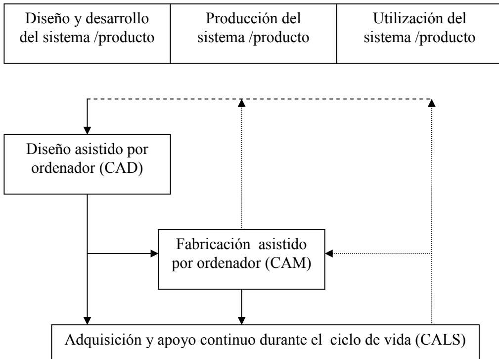
FIGURA 43. APLICACIÓN DE CALS EN EL CICLO DE VIDA DEL SISTEMA
