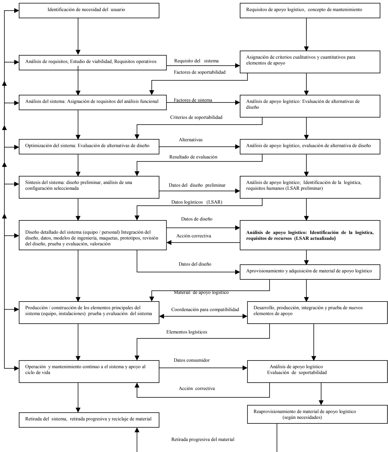
Figura 11. LOGÍSTICA DEL PROCESO DE DESARROLLO DEL SISTEMA
