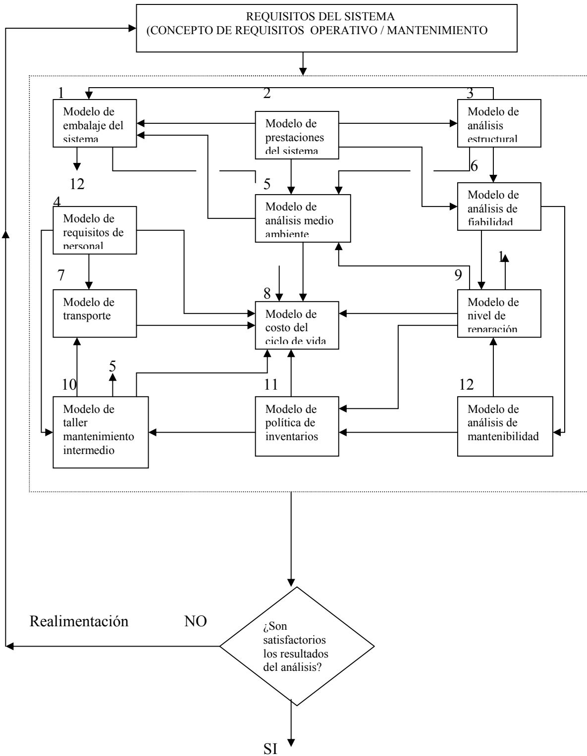
FIGURA 18. LA INTEGRACIÓN DE MODELOS ANALÍTICOS
