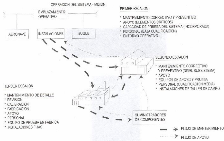
FIGURA 4. OPERACIÓN DEL SISTEMA Y FLUJO DE MANTENIMIENTO
