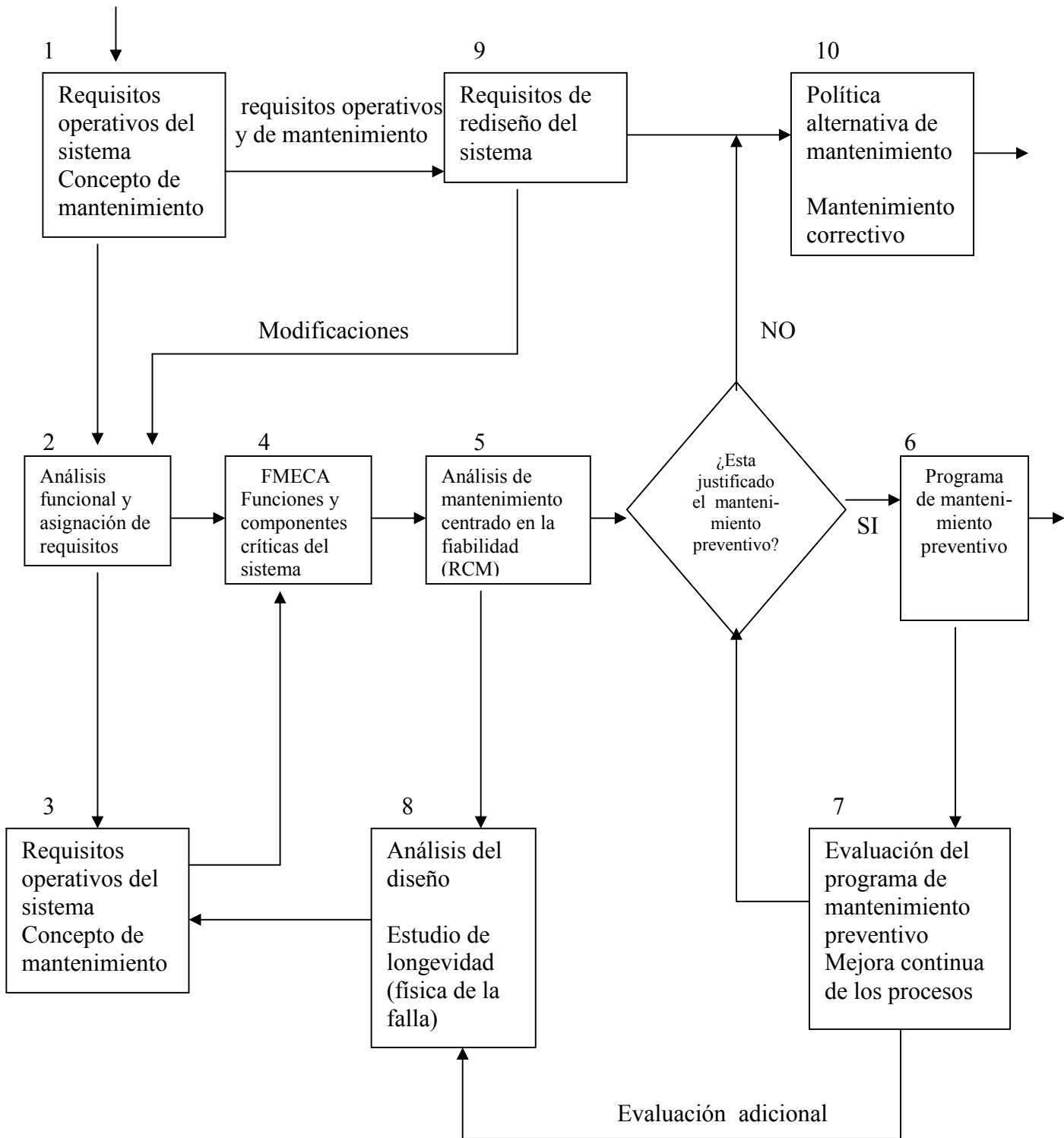
FIGURA 37. INTEGRACIÓN DE HERRAMIENTAS PARA EL MANTENIMIENTO PREVENTIVO
