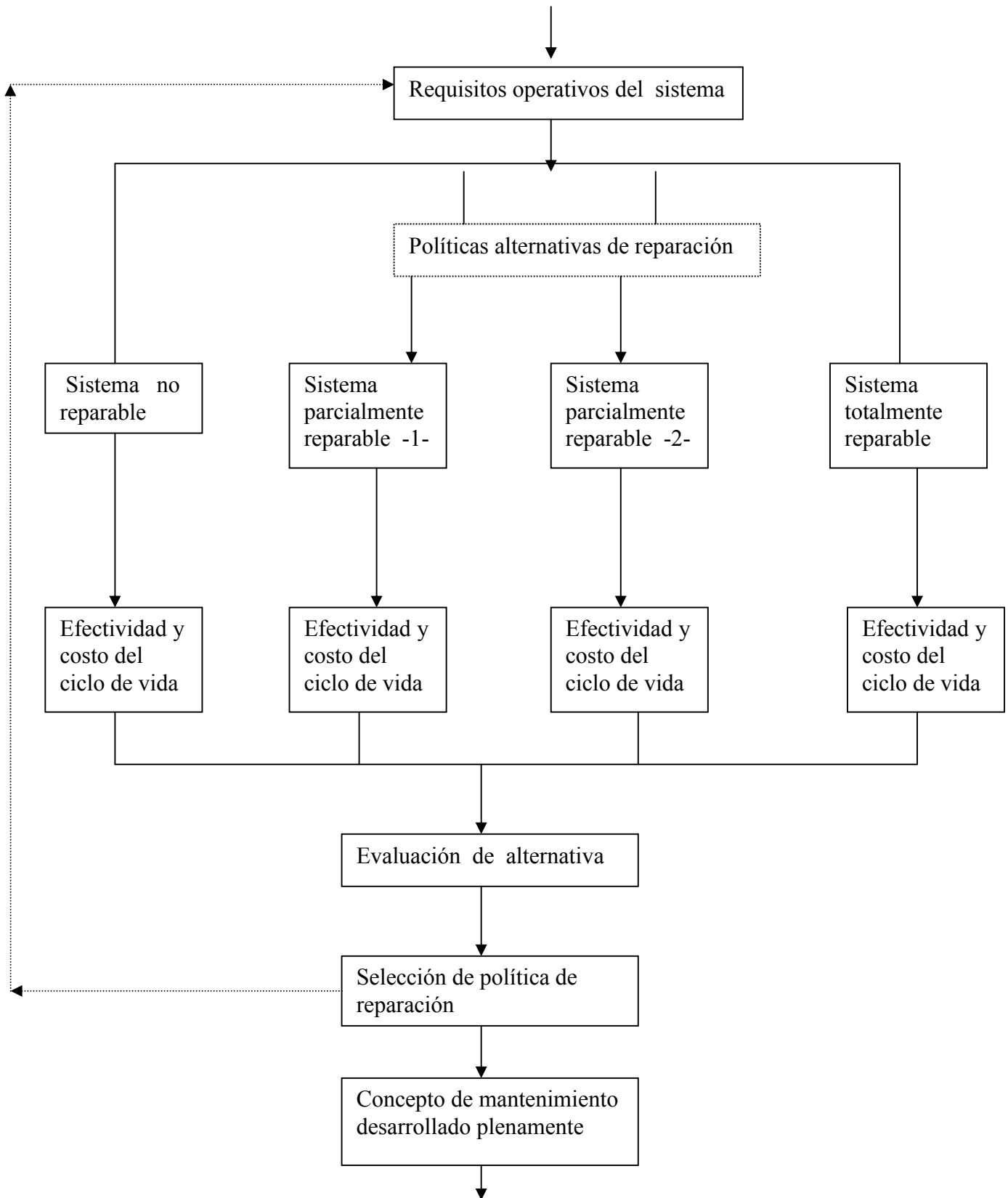
FIGURA 14. EVALUACIÓN Y OPTIMIZACIÓN DE LA POLÍTICA DE REPARACIÓN
