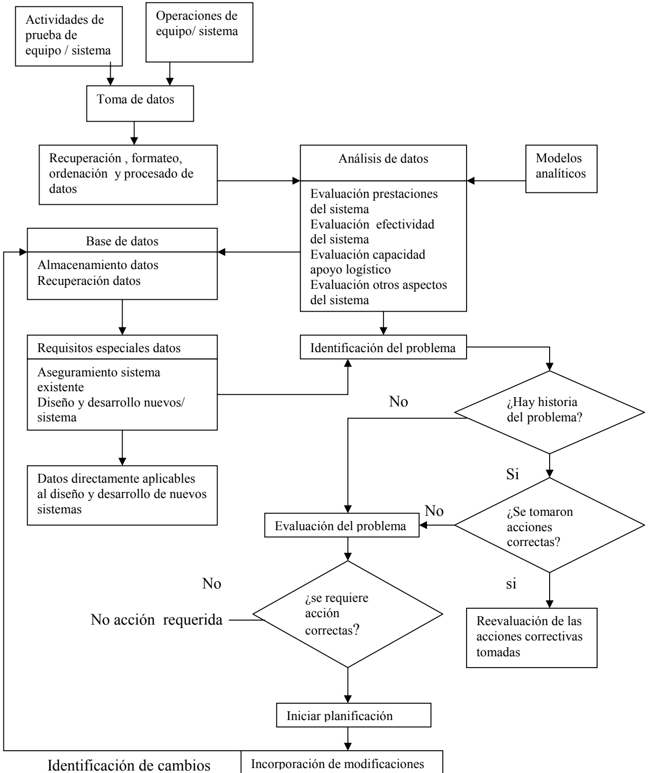
FIGURA 48. CICLO DE EVALUACIÓN DEL SISTEMA Y ACCIONES CORRECTIVAS
