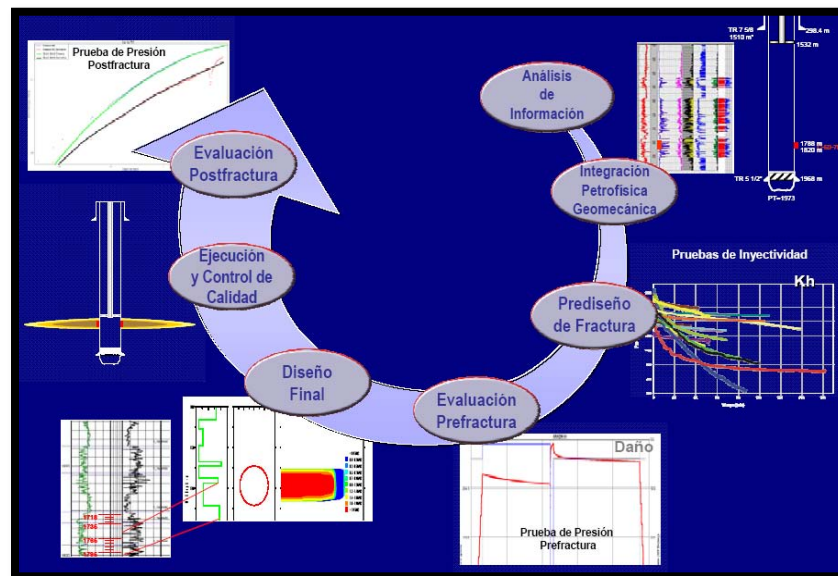
Figura 4.30 Proceso de fracturamiento hidráulico (Tomado de Pemex Región Norte, 2005).
