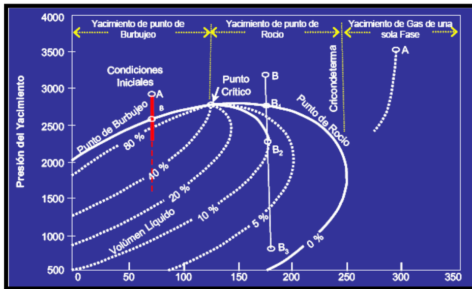
Figura 4.23 Diagrama de fases (Tomado de Pemex Región Norte, 2005).
