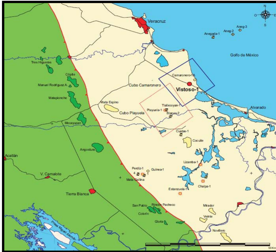
Figura 3.48 Localización del campo Vistoso. (Tomado de Pemex, 2004).
