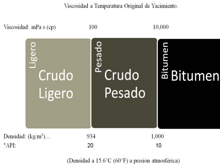
Figura 3.67 Definición de bitumen y de petróleo pesado tomando como base la viscosidad, densidad y °API (Tomado de Briones, 2011).
