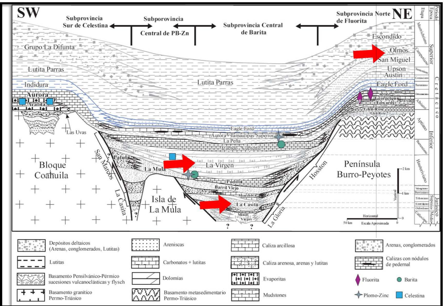
Figura 3.17 Sección transversal A-A', mostrando la configuración interna restituida (anterior a la Orogenia Larámide), de la cuenca mesozoica del Noroeste de México. (Tomada de González Sánchez, 2007).
