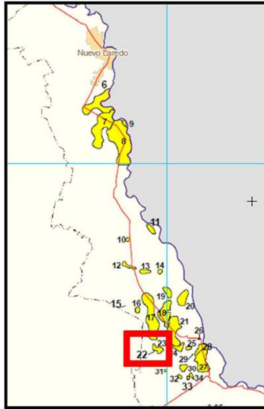
Figura 3.6 Localización del Campo Levita (Marcado con el número 22) (Tomado de PEP, 2009.)
