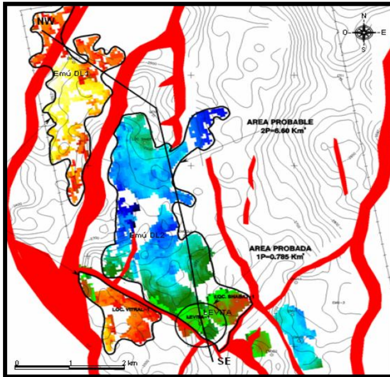
Figura 3.7 Mapa estructural de las areniscas del campo Levita. El campo se encuentra entre dos fallas de crecimientos importantes y las fallas sintéticas compartimentan los yacimientos. (Tomado de Pemex, 2003).
