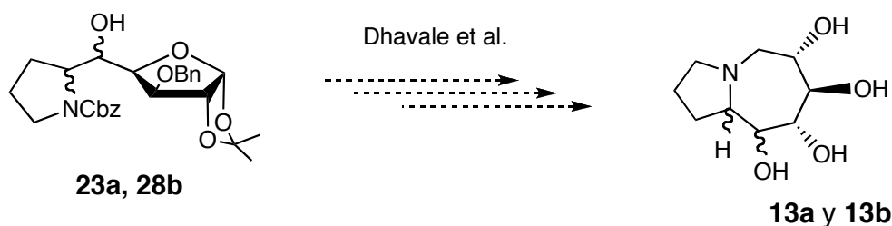
Esquema 27. Obtención de 13a y b a partir de 23a y 28b .
