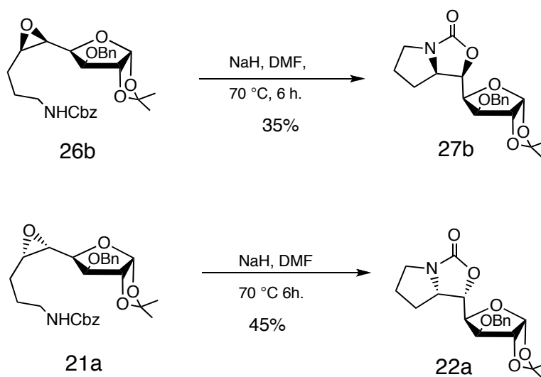
Esquema 25. Obtención de 22a y 27b
