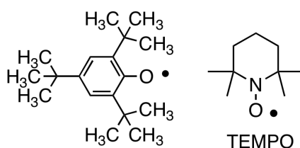
Figura 6. Radicales estables cinéticamente por efecto estérico.
