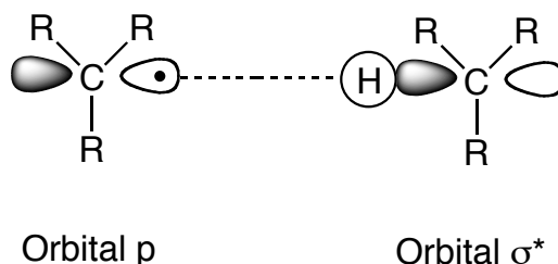
Esquema 5. Interacción "lineal" intramolecular
