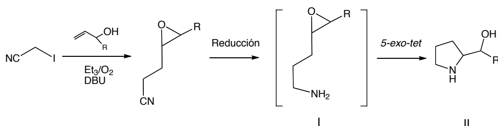
Esquema 15. Ruta planeada para la síntesis de 2-hidroxipirrolidinas.
