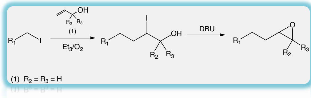
Esquema 28. Método general de obtención de los epóxidos.
