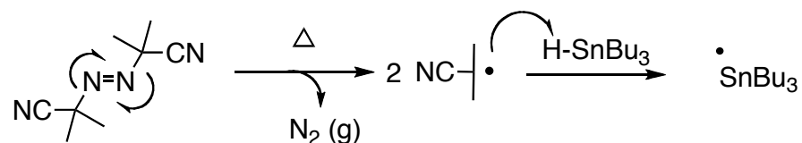
Esquema 9. Etapa de iniciación del radical tributilestanil por AIBN
