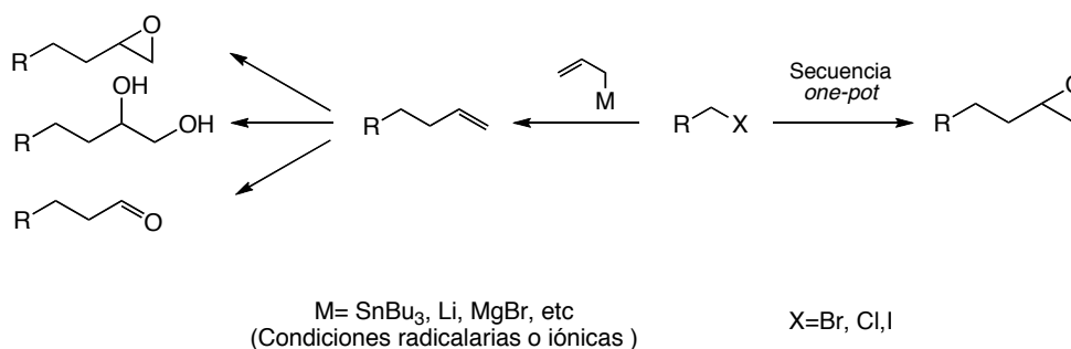
Esquema 13. Productos típicos obtenidos de una reacción de alilación
