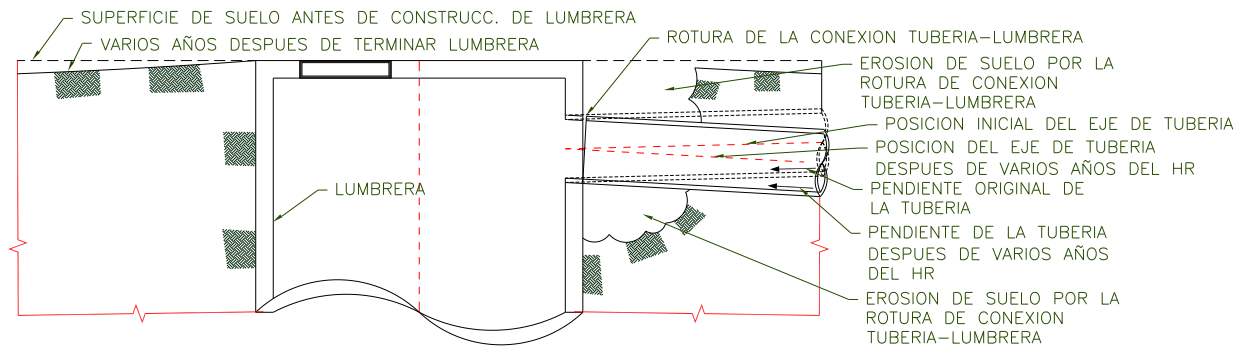
Figura 91. Daños en la conexión lumbrera-tubería por el HR cerca de la superficie de suelo.
