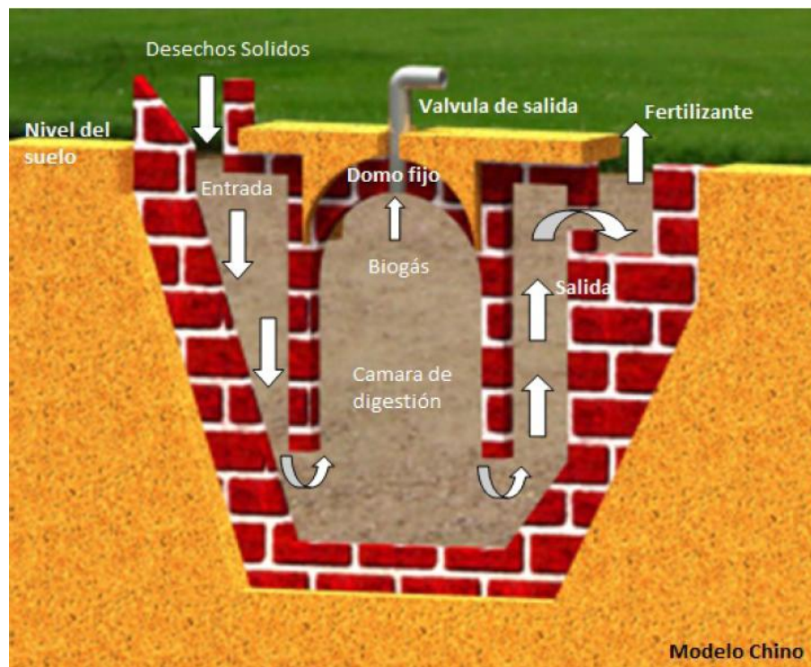
Figure 1.2: Modelo de biodigestor chino
