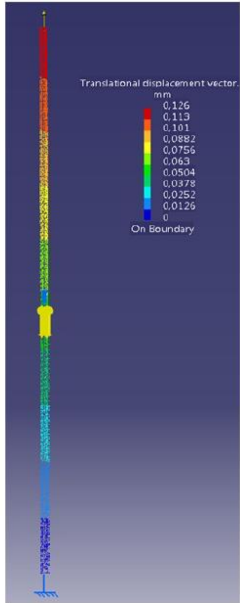
Figure 3.26: Análisis del tubo a tensión Figure 3.27: Desplazamientos del tubo
