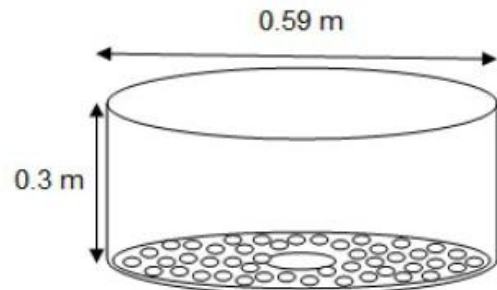
Figure 3.14: Volumen de control reducido
