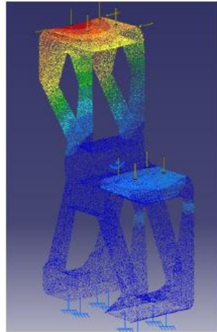
Figure 3.30: Esfuerzos en el soporte Figure 3.31: Desplazamientos del soporte
