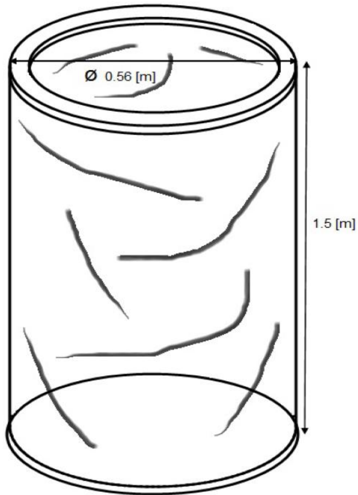
Figure 3.7: Gasómetro flexible
