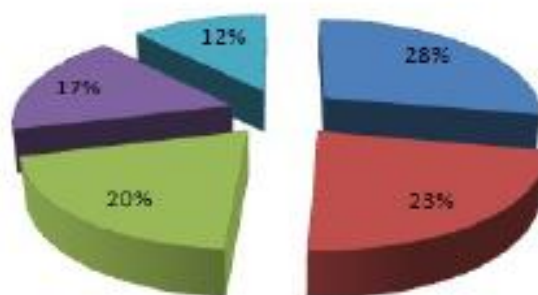
Figure 1.5: Principales orígenes de metano
