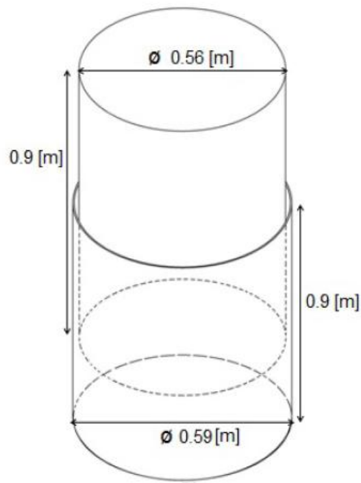
Figure 3.6: Gasómetro con domo flotante
