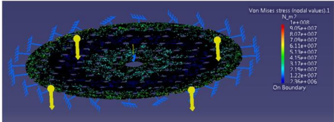
Figure 3.20: Concentración de esfuerzos
