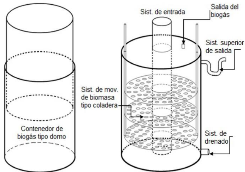
Figure 2.19: Diseño preliminar del prototipo
