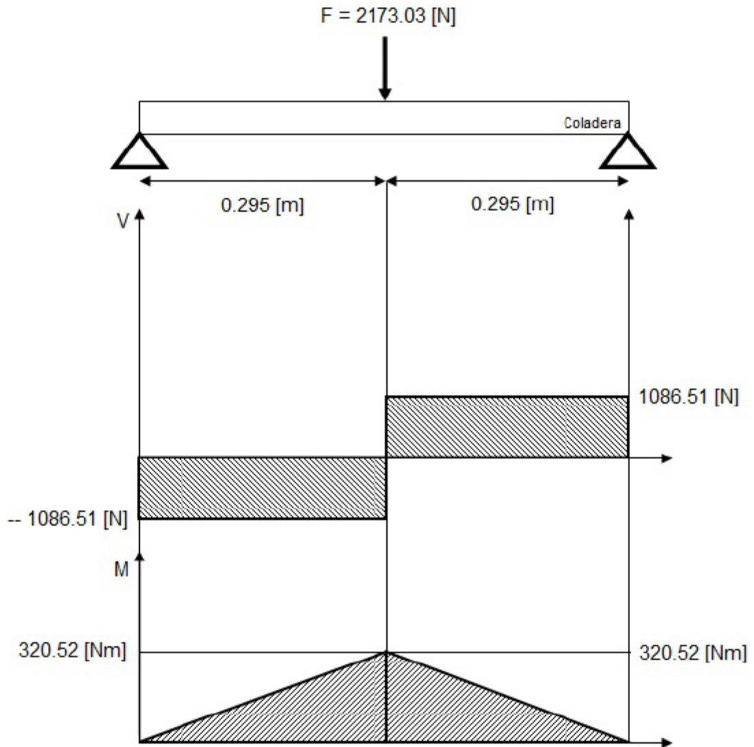
Figure 3.19: Grafica de fuerzas cortantes y momentos flectores
