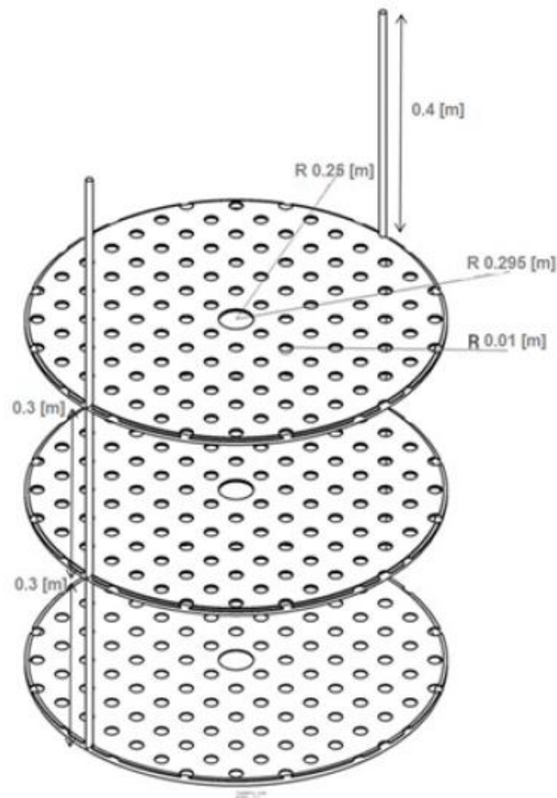
Figure 3.8: Dimensiones del sistema de movimiento de biomasa
