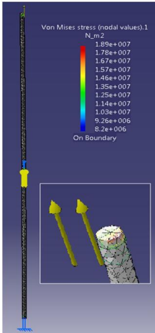
Figure 3.24: Esfuerzos en la barra mediante Von Mises
