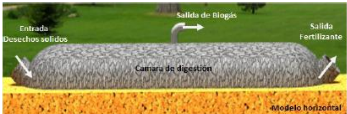
Figure 1.4: Modelo de biodigestor tipo horizontal
