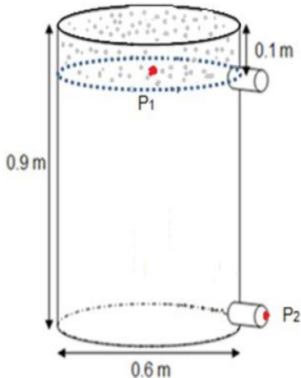
Figure 3.11: Tiempo de drenado del contenedor
