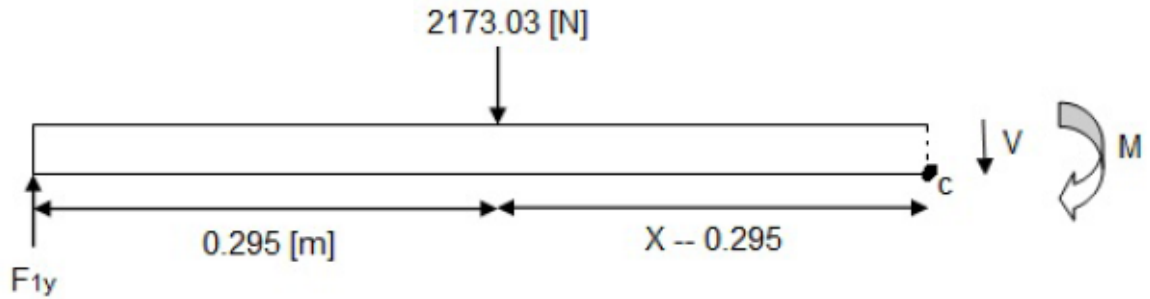
Figure 3.18: Segunda sección de la barra
