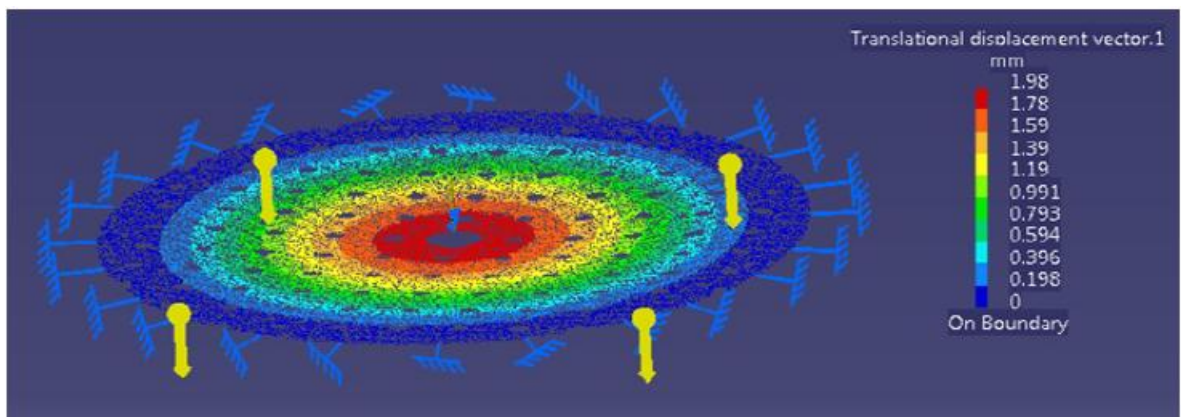
Figure 3.22: Desplazamiento sobre la pieza
