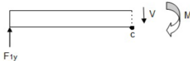
Figure 3.17: Primera sección de la barra
