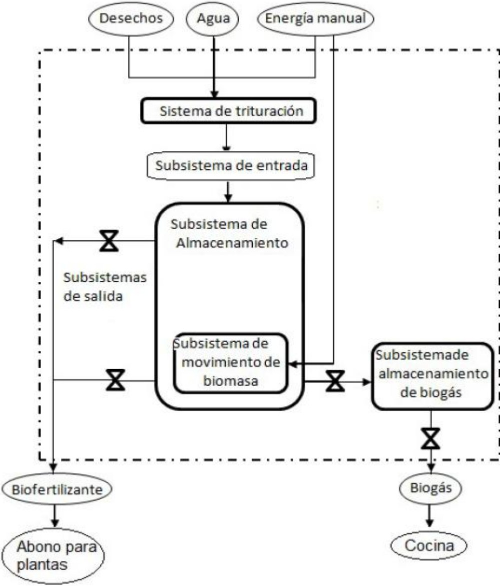
Figure 2.1: Diagrama de flujo del proceso
