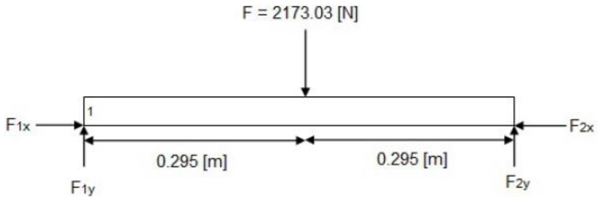
Figure 3.16: Diagrama de cuerpo libre
