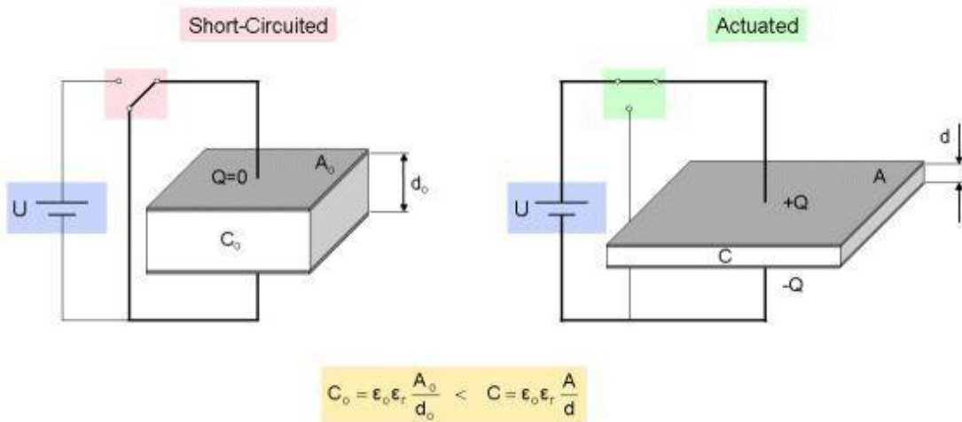
Figura 85. Diferencia entre un EAP en estado de trabajo y uno en reposo
