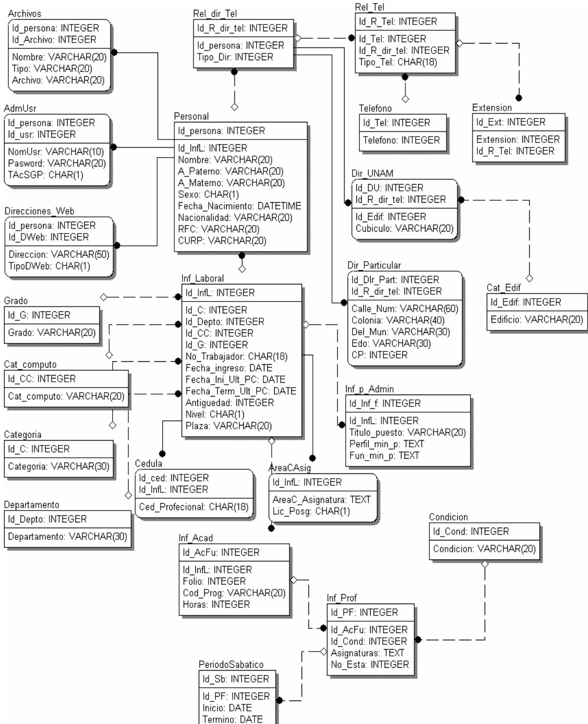
Figura 2.5 Diseño Físico
