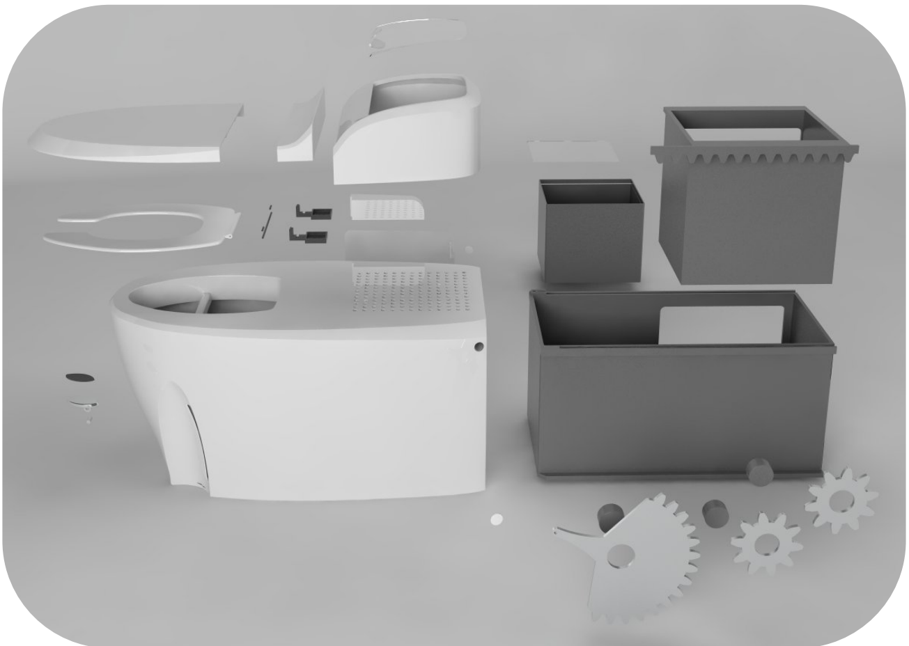
Figura 47. Despiece, explosivo.
