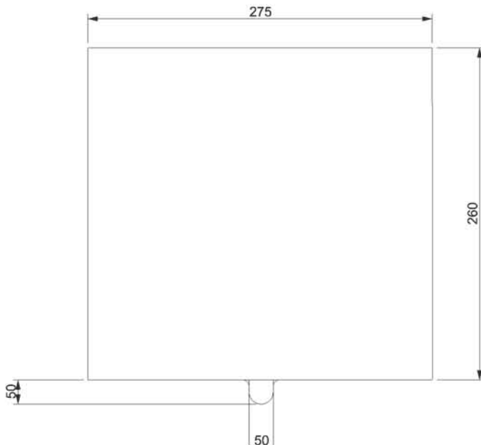
VISTAS SUPERIOR
