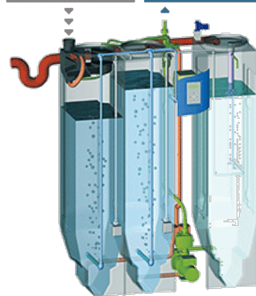
Figura 32. Tratamiento de aguas grises.
