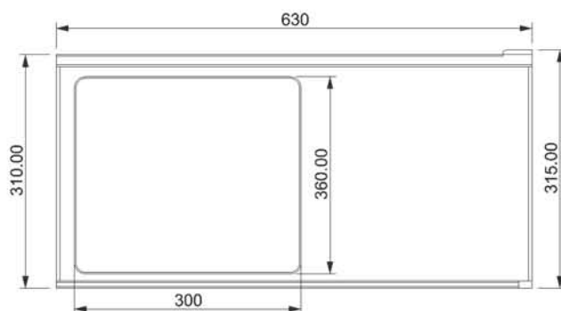
VISTAS SUPERIOR
