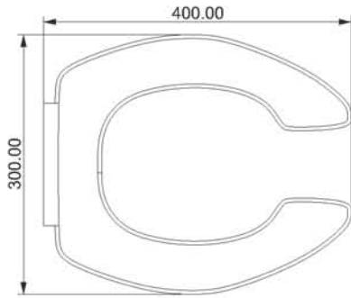
VISTAS SUPERIOR
