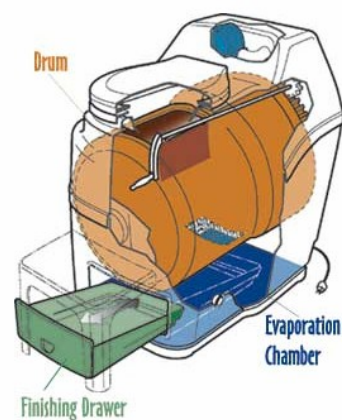
Figura 23. Baño Sun-mar, funcionamiento.
