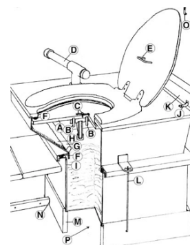
Figura 21. Baño Cotuit, funcionamiento.
