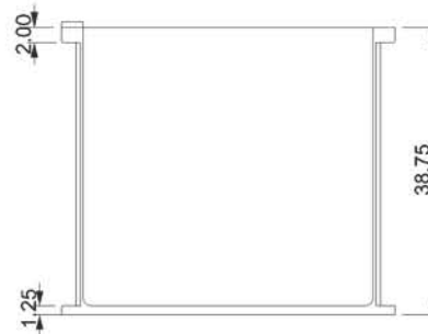
VISTA LATERAL
