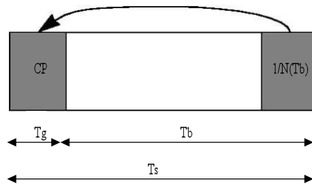
Figura 4. 4. Estructura del símbolo OFDMA en el dominio del tiempo.
