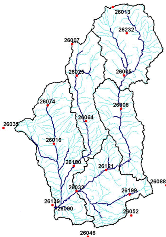
Figura 4.3 Distribución de estaciones climatológicas
