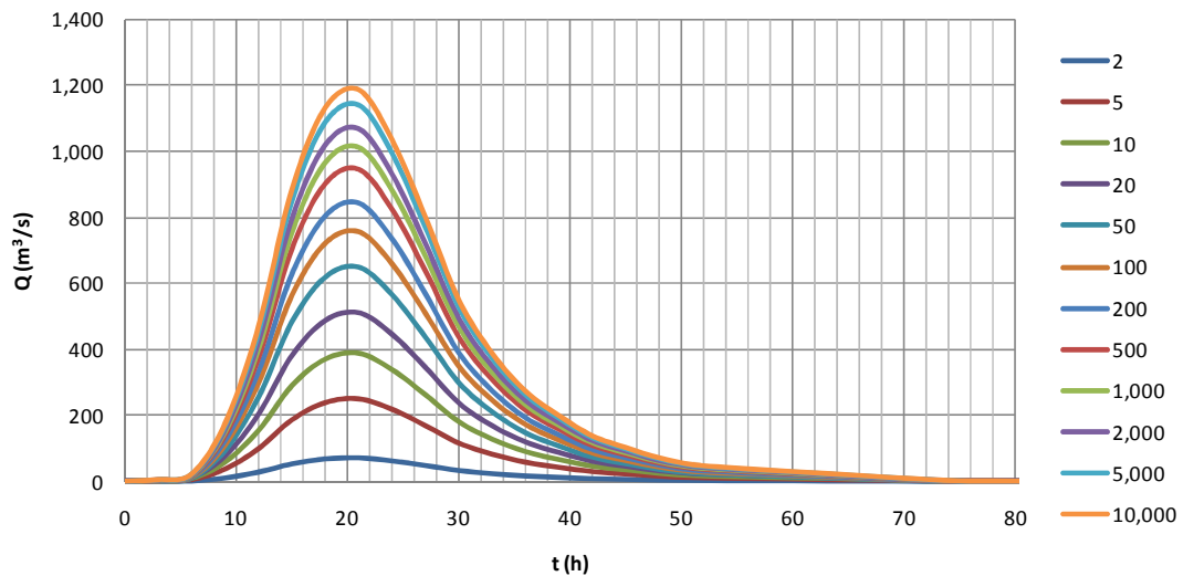
Figura 4.28 Hidrogramas de escurrimiento directo para diferentes periodos de retorno, El Molinito
