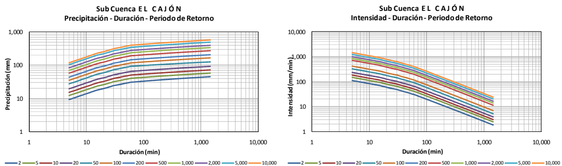
Figura 4.13 Curvas a) hp - d - Tr y b) i - d - Tr de la subcuenca El Cajón
