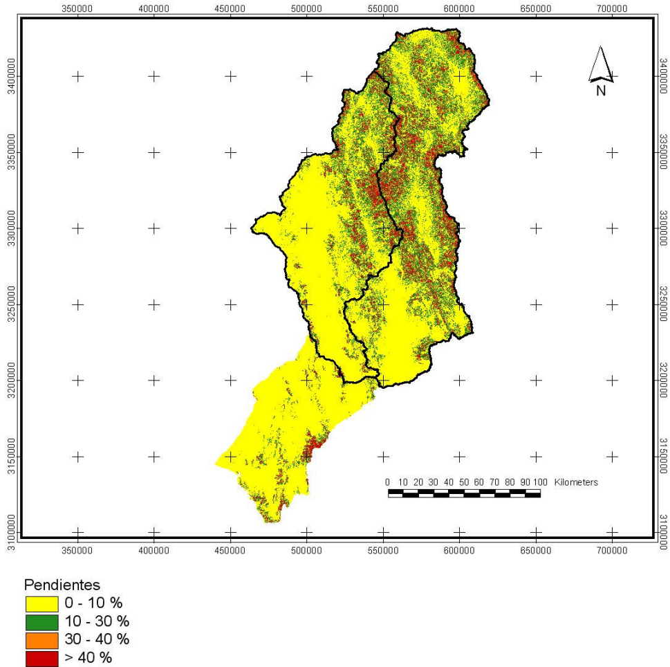
Figura 4.1 Distribución de pendientes en la Cuenca del Río Sonora
