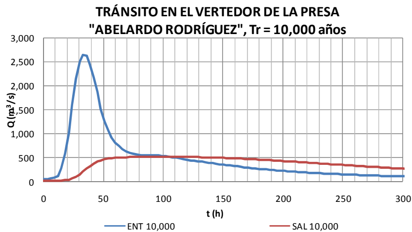
Figura 4.38 Configuración 2. Tránsito de avenidas sobre el vertedor de la presa Abelardo L. Rodríguez.
