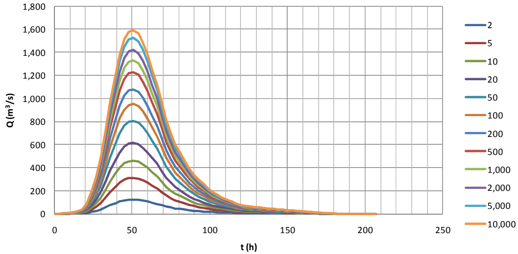
Figura 4.27 Hidrogramas de escurrimiento directo para diferentes periodos de retorno, El Orégano
