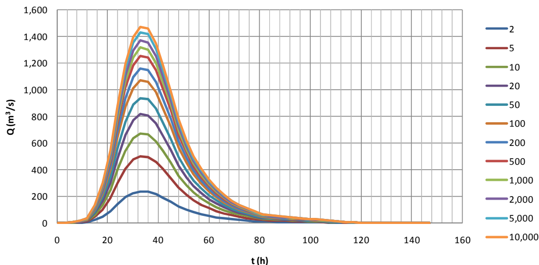
Figura 4.31 Hidrogramas de escurrimiento directo para diferentes periodos de retorno, El Zanjón
