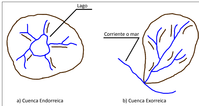
Figura 2.2 Clasificación de una cuenca en función de las salidas
