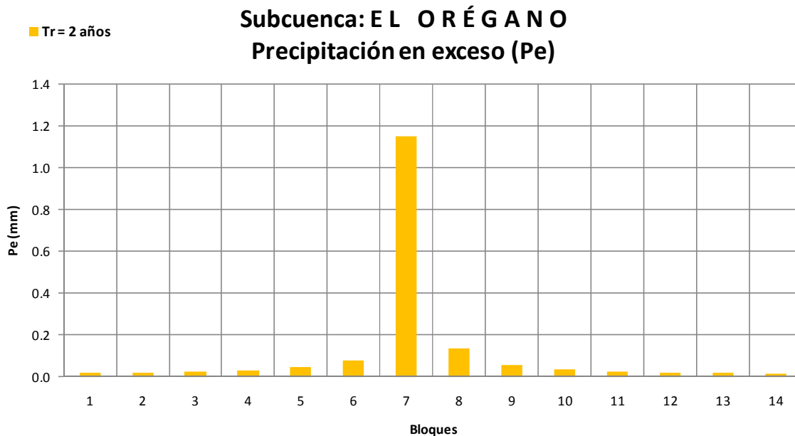
Figura 4.16 Precipitación efectiva en bloques alternos en la subcuenca El Orégano, Tr = 2 Años
