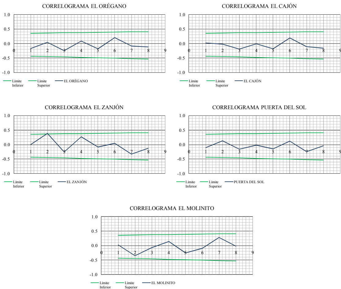
Figura 4.5 Correlogramas para las diferentes subcuencas en el sitio en estudio
