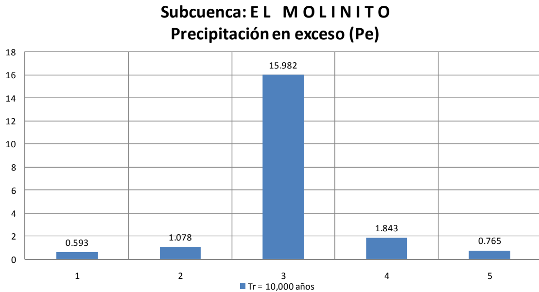
Figura 4.18 Precipitación efectiva en bloques alternos en la subcuenca El Molinito, Tr = 10,000 Años
