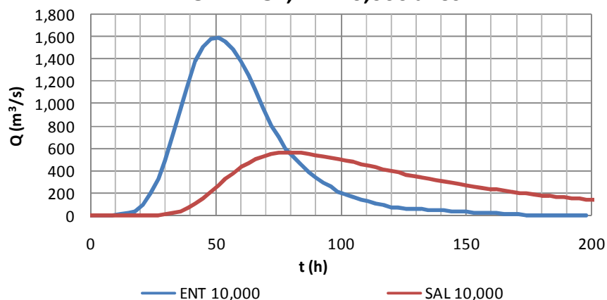
Figura 4.33 Configuración 1. Tránsito de avenidas sobre el vertedor de la presa El Molinito
