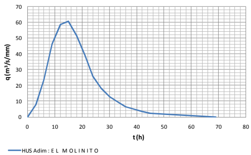
Figura 4.23 Hidrograma Unitario, subcuena El Molinito
