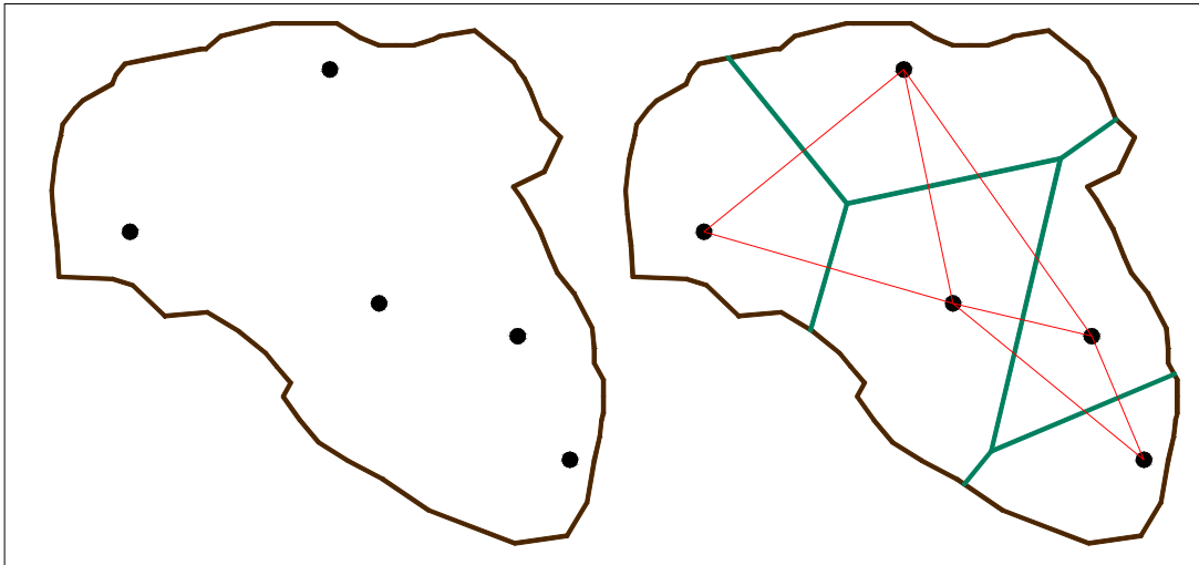
Figura 3.7 Precipitación media. Polígonos de Thiessen
