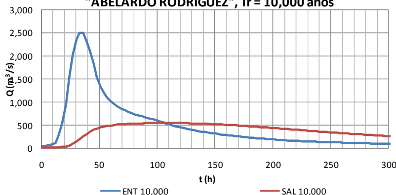
Figura 4.34 Configuración 1. Tránsito de avenidas sobre el vertedor de la presa Abelardo Rodríguez L.
