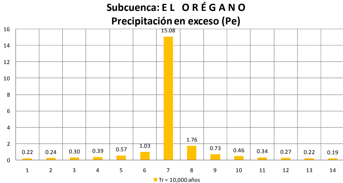
Figura 4.17 Precipitación efectiva en bloques alternos en la subcuenca El Orégano, Tr = 10,000 Años
