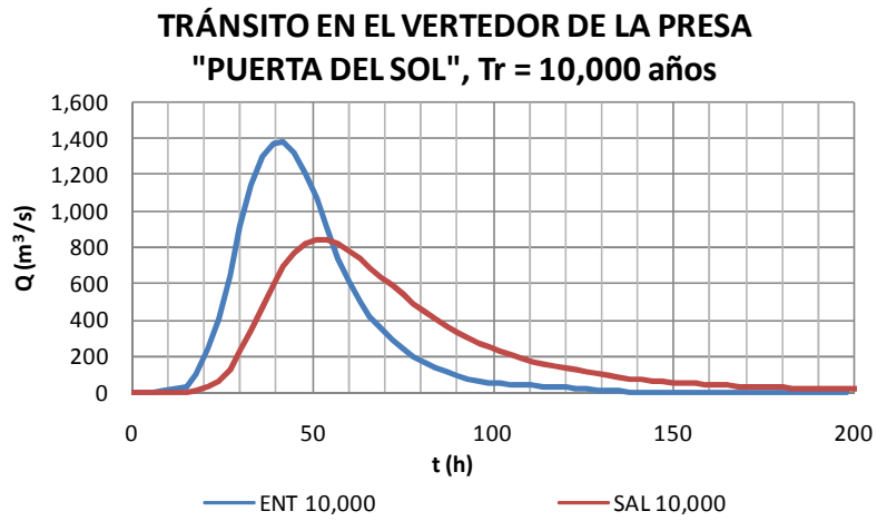
Figura 4.44 Configuración 4. Tránsito de avenidas sobre el vertedor de la presa Puerta del Sol
