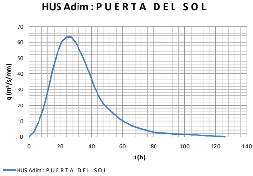
Figura 4.24 Hidrograma Unitario, subcuena Puerta del Sol
