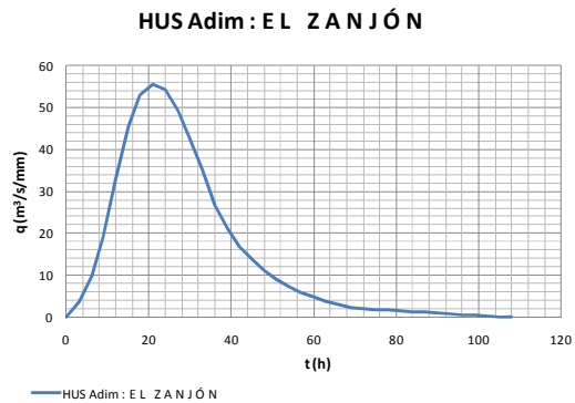
Figura 4.26 Hidrograma Unitario, subcuena El Zanjón
