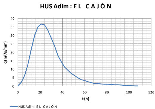
Figura 4.25 Hidrograma Unitario, subcuena El Cajón
