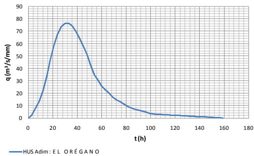
Figura 4.22 Hidrograma Unitario, subcuena El Orégano
