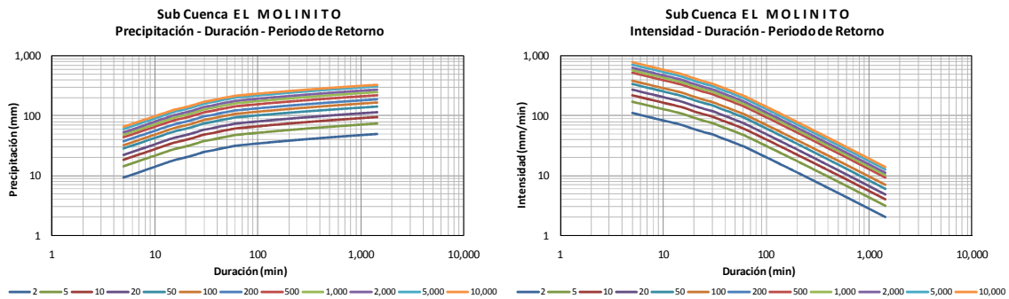
Figura 4.12 Curvas a) hp - d - Tr y b) i - d - Tr de la subcuenca El Molinito
