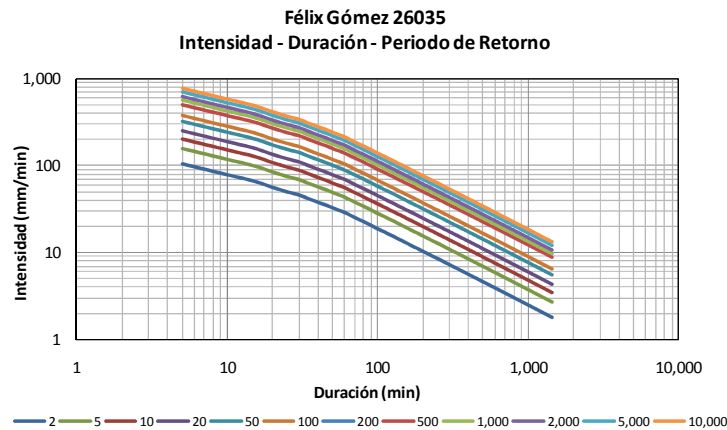
Figura 4.9 Curva i - d - Tr de la estación Félix Gómez
