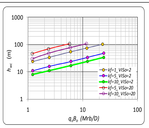
Figura 3.15. Curvas de h_{wc} en función k_f para una partición de porosidad matriz-fractura de 85%-15%.
