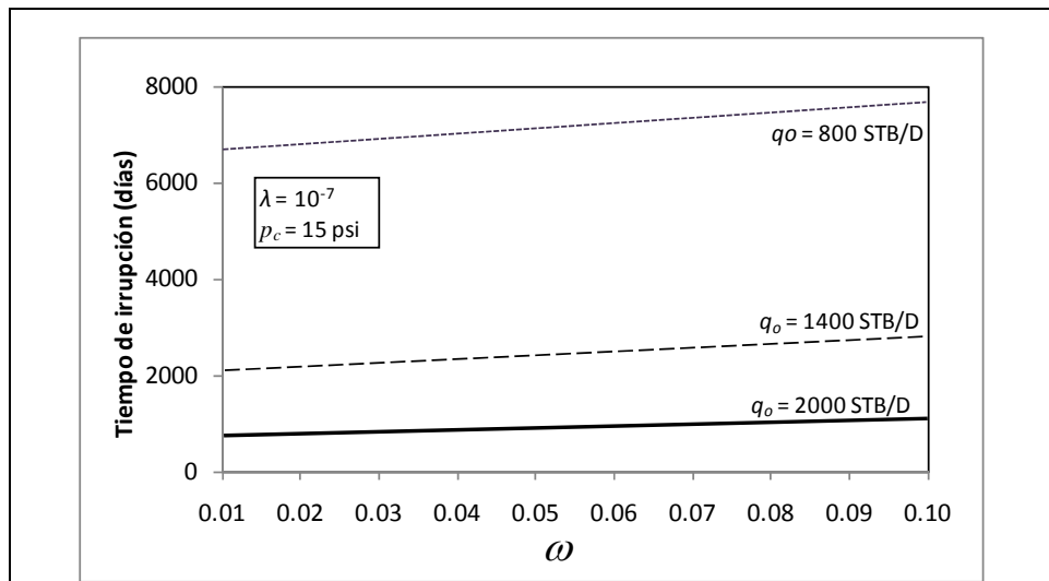
Figura 1.10. Efecto de \omega en el tiempo de irrupción del agua.
