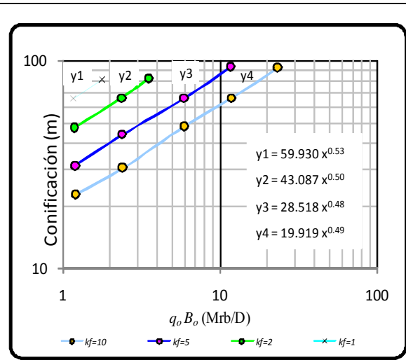
Figura 3.11. Curvas de h_{wc} en función k_f para \mu_o = 10 cp.
