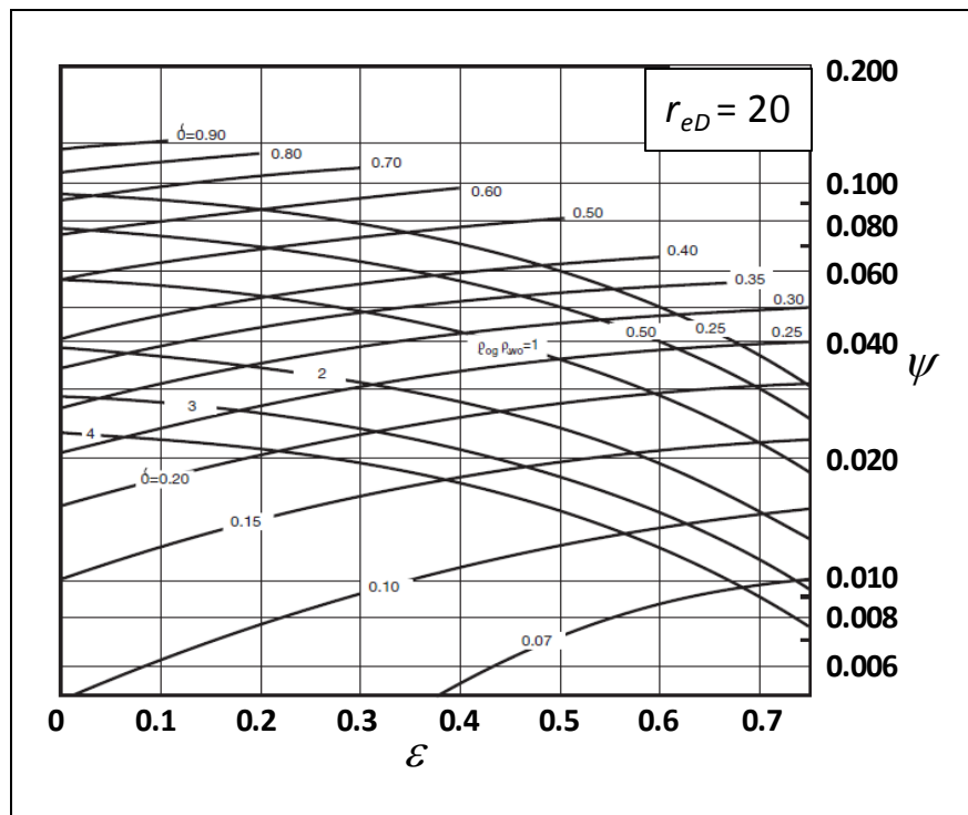
Figura 1.15. Funciones adimensionales para r_{eD} = 20 .
