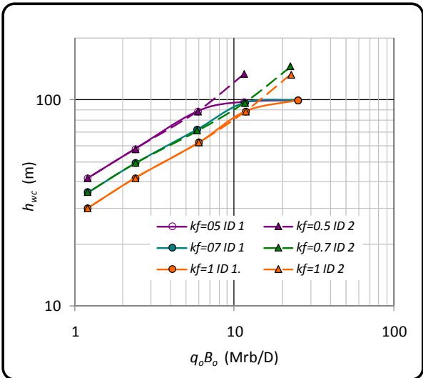
Figura 3.8. Comparación de h_{wc} alcanzada en cada intervalo disparado.
