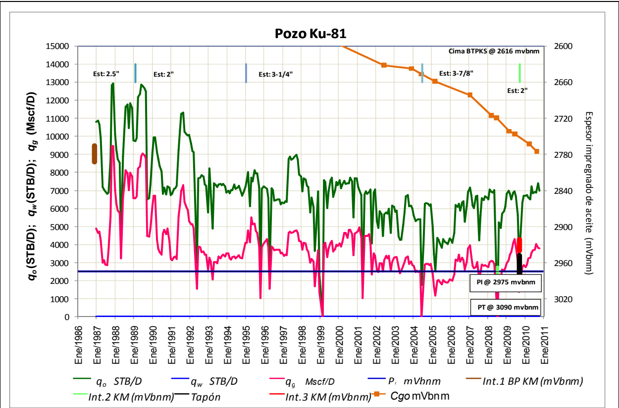
Figura 6.4. Historia de Explotación del pozo Ku-81.
