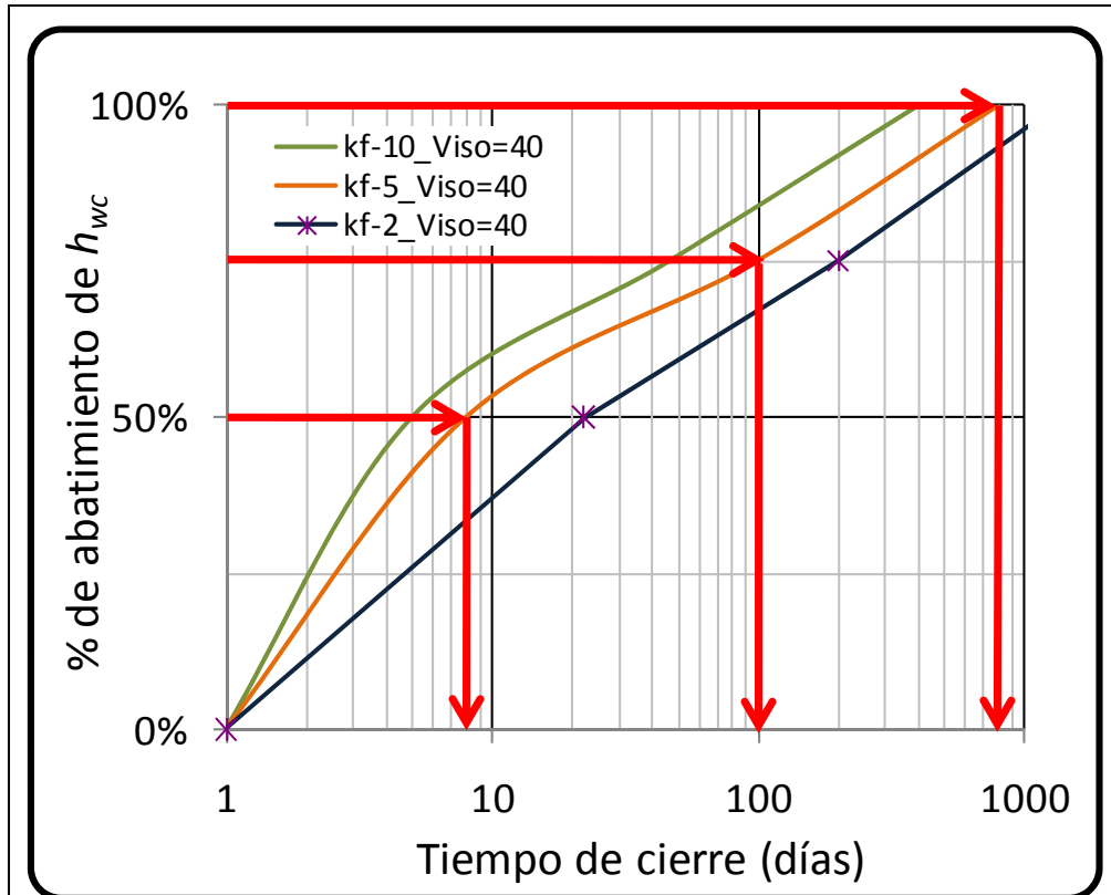
Figura 6.8. Determinación del tiempo de cierre del pozo para la reconfiguración de cono de agua.
