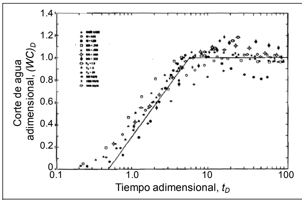
Figura 1.6. Resultados normalizados de corte de agua.
