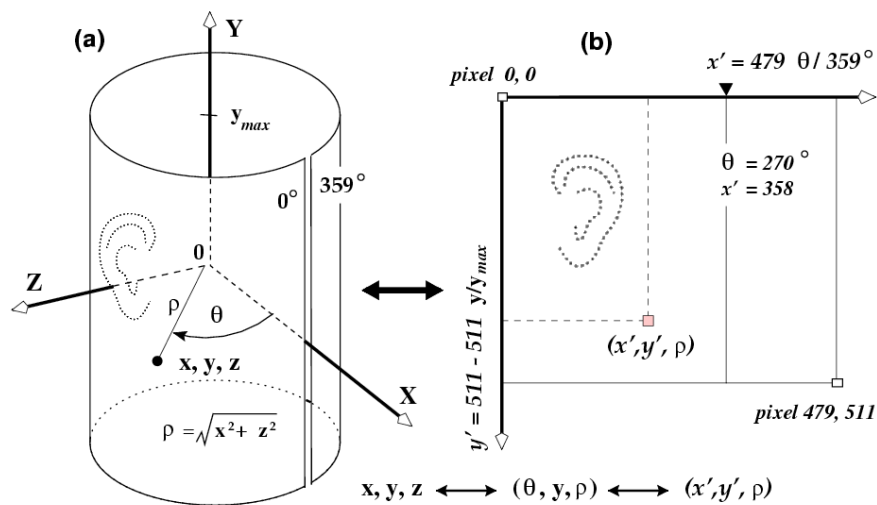
Figura 10: Representación e interpretación del escáner láser
