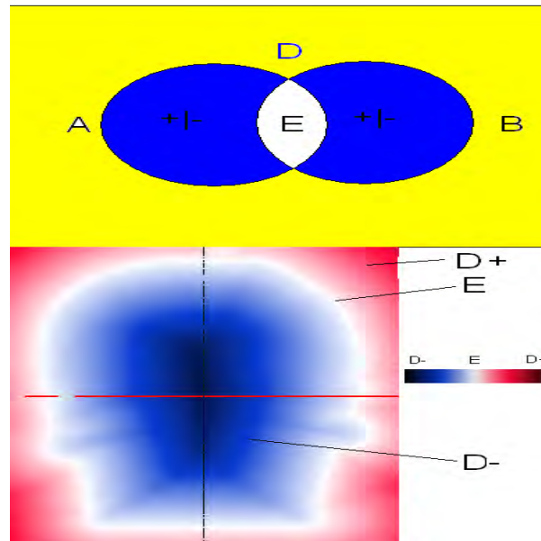
Figura 19: diagrama de Venn para diferencias simétricas de dos conjuntos en azul y la diferencia simétrica de un campo de distancia con un campo de distancia
