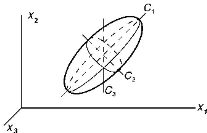
Figura 32: interpretación geométrica de las componentes principales
