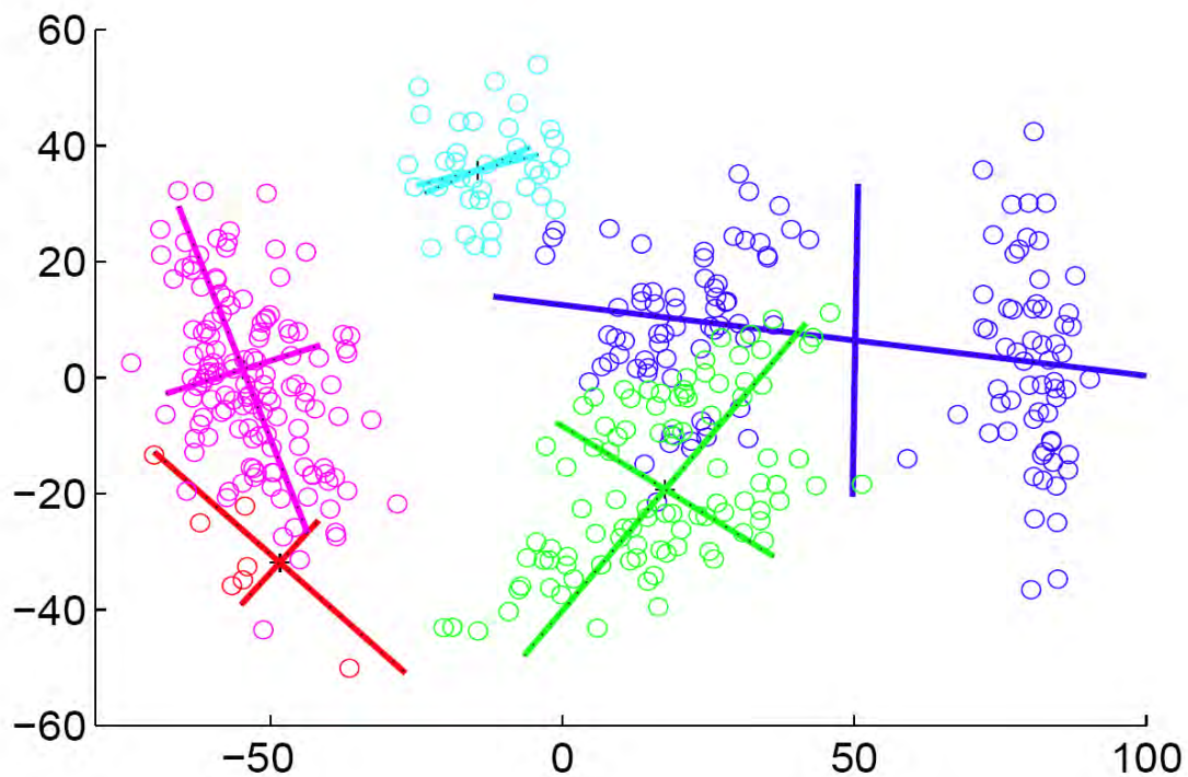
Figura 30: nubes de puntos y sus componentes principales
