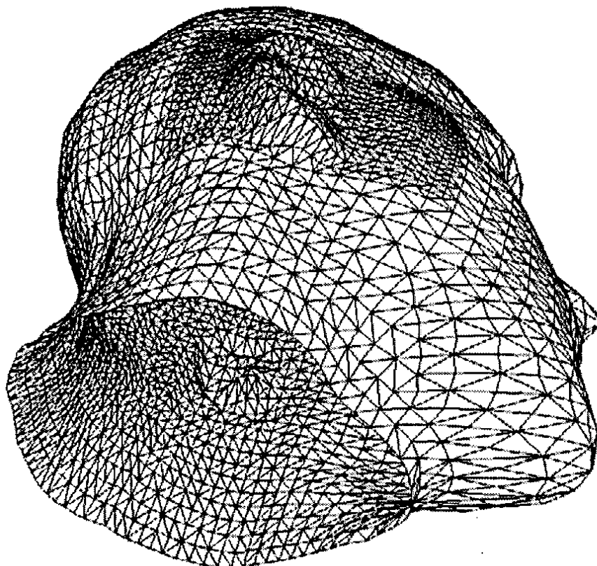
Figura 12: modelo obtenido del escáner láser. La zona alrededor de la oreja se malló a mayor resolución por ser de interés particular en el proyecto original.
