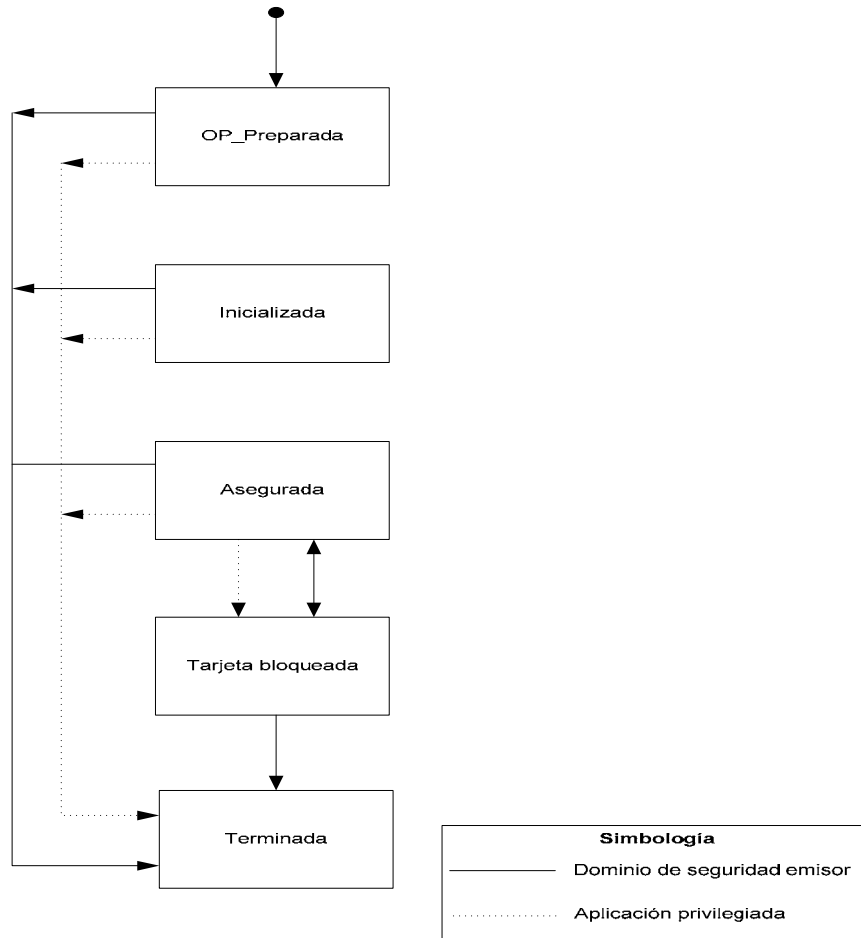
Figura 10. Diagrama de transición de los estados del ciclo de vida de la tarjeta
