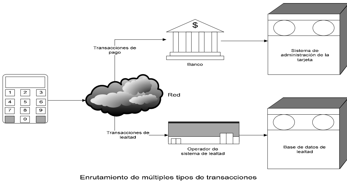
Figura 38. Operación de una tarjeta inteligente gestionada por el SGTI, con interfaces de los sistemas del emisor y del operador del programa de lealtad
