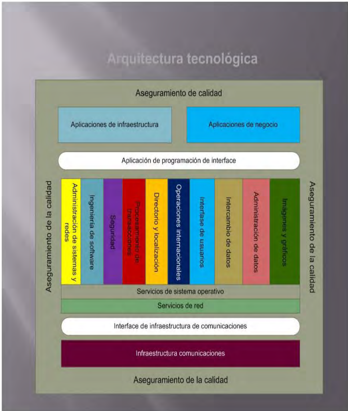
Figura 59. TRM de TOGAF, componentes y estructura de la arquitectura tecnológica
