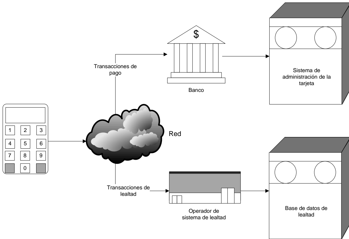
Figura 28. Enrutamiento de múltiples tipos de transacciones
