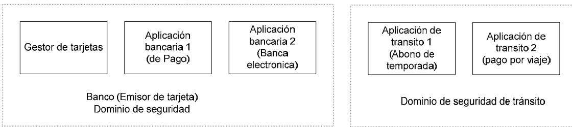
Figura 21. Dominios de seguridad de la arquitectura multiaplicaciones
