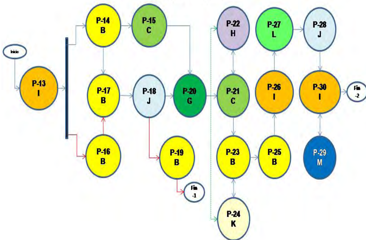
Diagrama de contexto de los procesos de postemisión de tarjeta inteligente
