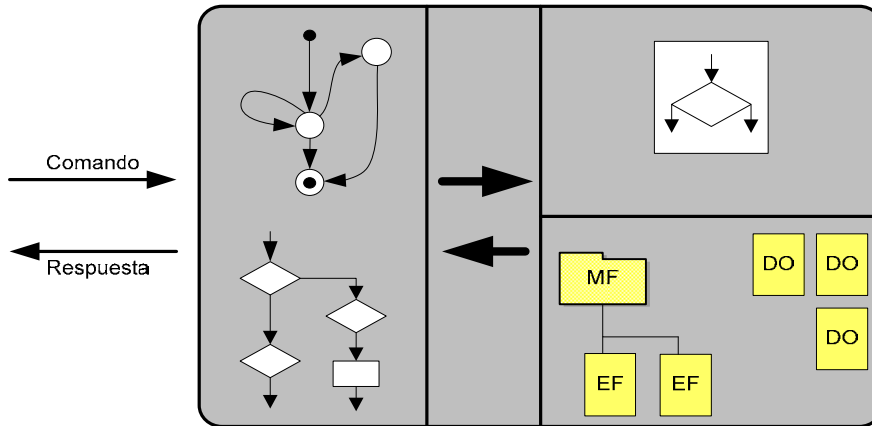
Figura 15. Arquitectura de aplicación basada en código
