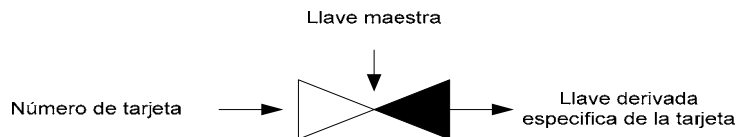
Figura 32. Método para derivar llaves simétricas
