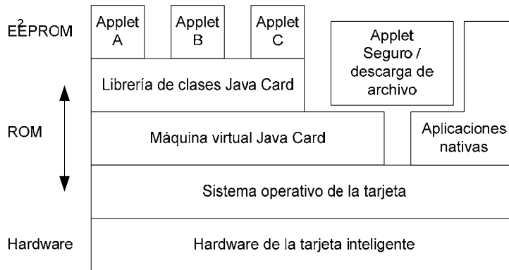
Figura 16. Entorno de ejecución de Java Card
