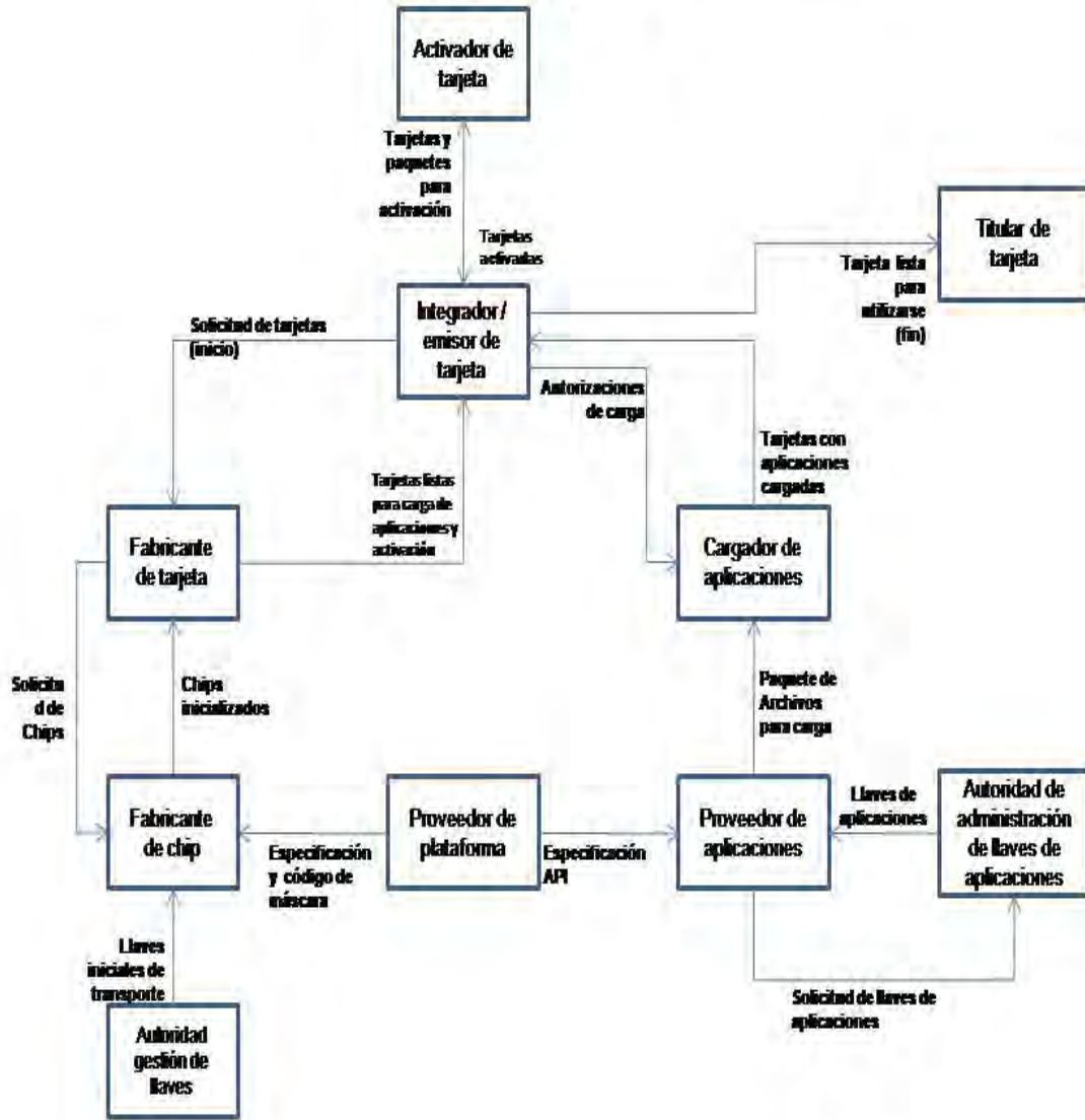
Figura 55. Diagrama de contexto del flujo de datos de los procesos de preemisión y emisión en el SGTI
