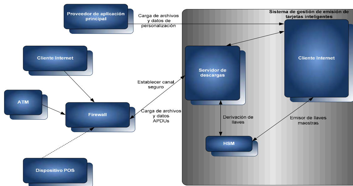
Infraestructura de descarga Postemisión
