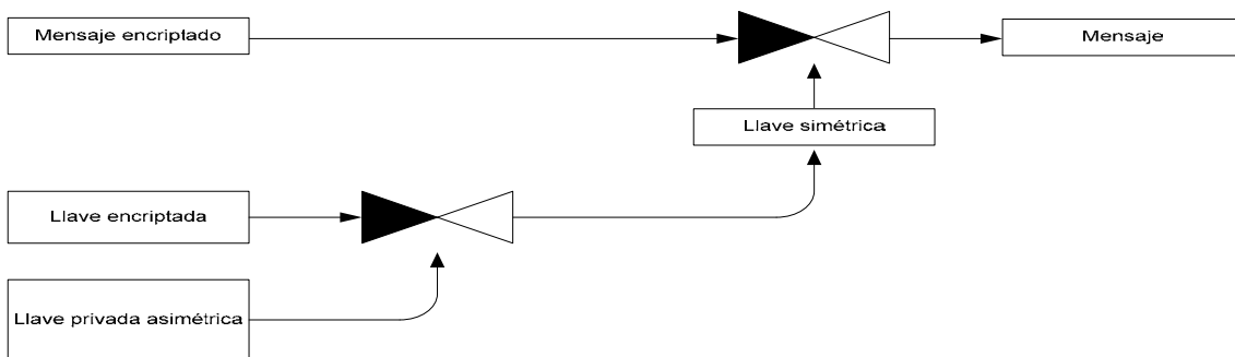
Figura 35. Procedimiento para el intercambio de llaves usando una combinación de algoritmos simétricos y asimétricos
