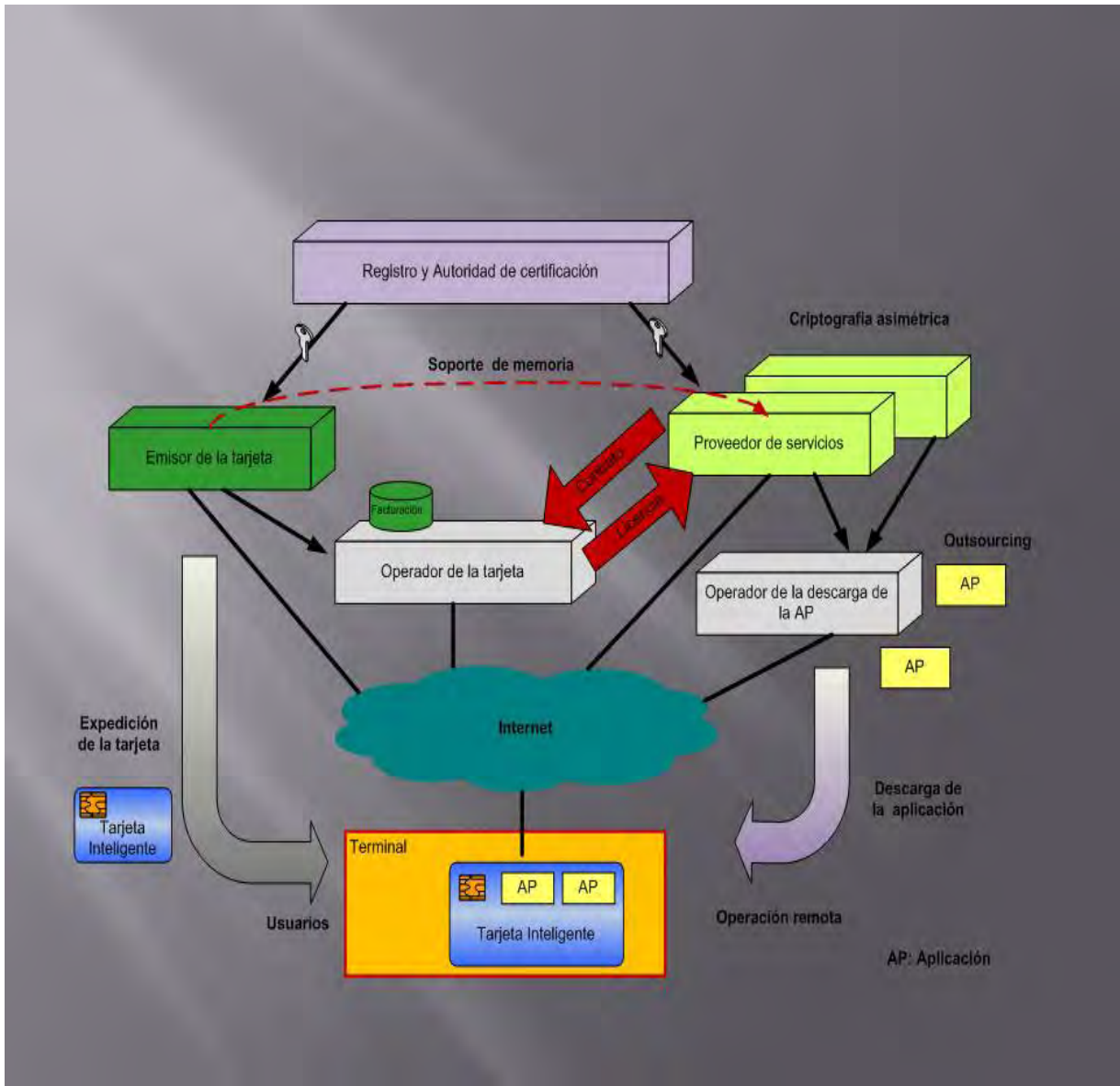
Figura 37. Servicios soportados en la gestión de una tarjeta inteligente por diferentes sistemas de información
