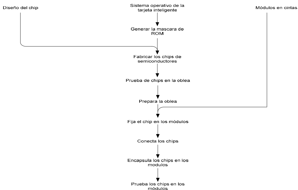
Figura 8. La producción de chips y módulos
