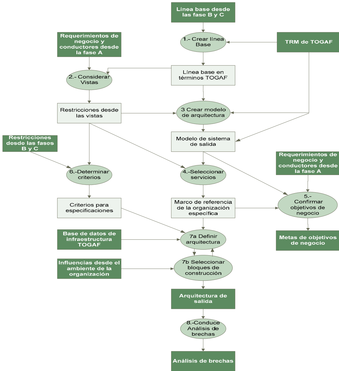
Figura 58. Flujo para la integración de la Línea base de la arquitectura tecnológica
