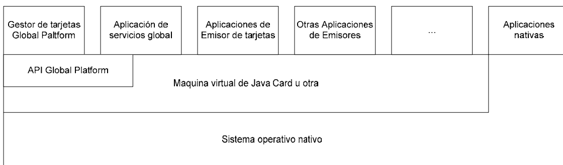
Figura 20. Ambiente Global Platform de multiaplicaciones/multiproveedores
