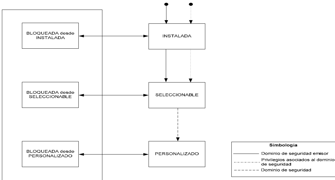
Figura 11. Diagrama de transición de los estados del ciclo de vida de las aplicaciones
