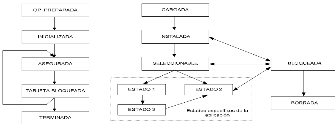
Figura 22. Ciclo de vida de la tarjeta y aplicaciones
