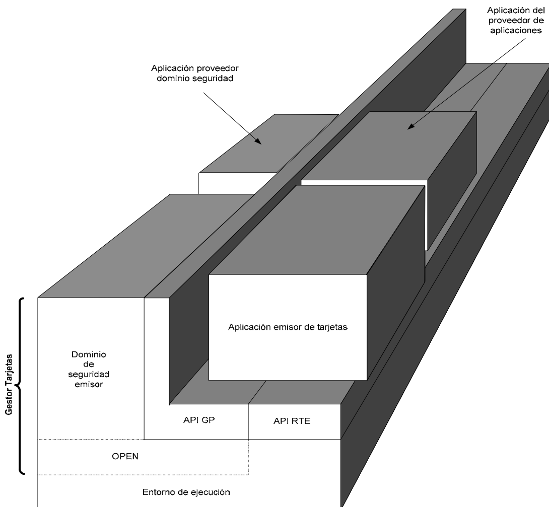
Figura 23. Arquitectura de la tarjeta Global Platform
