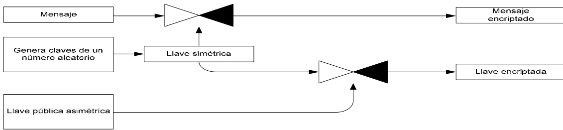
Figura 34. Procedimiento para el intercambio de llaves usando una combinación de algoritmos criptográficos simétricos y asimétricos
