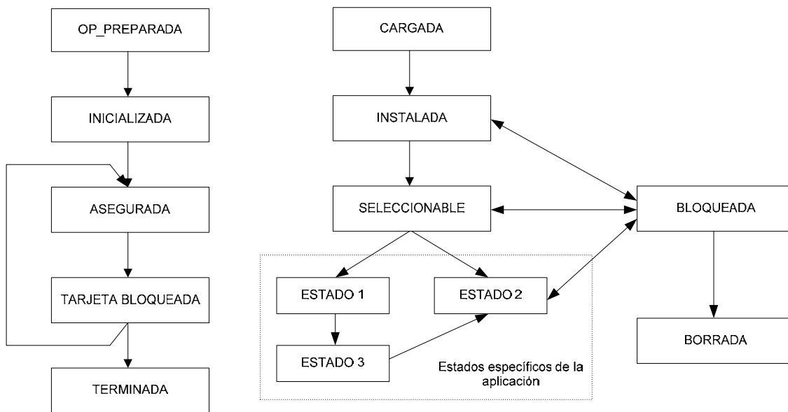
Figura 51. Ciclo de vida de las tarjetas y las aplicaciones
