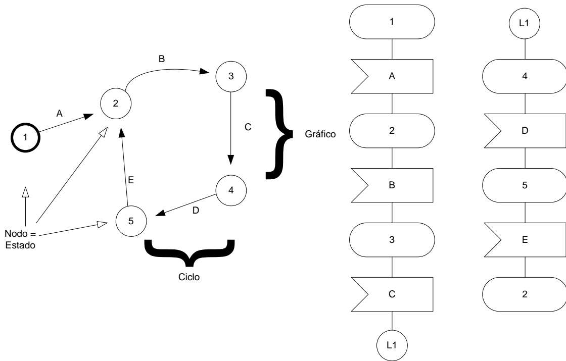
Figura 6. Dos diferentes representaciones de diagramas de estado
