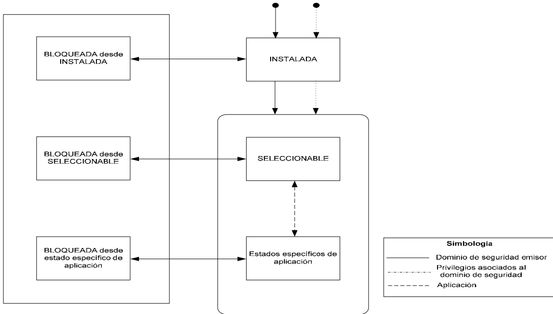
Figura 11. Diagrama de transición de los estados del ciclo de vida de las aplicaciones
