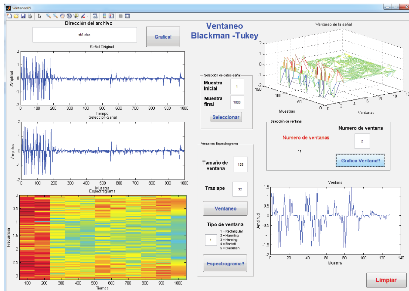
Figura 8.8: Ambiente de trabajo Blackman-Tukey para señal EMG asociada a extensión de bíceps (Ventana Hamming, tamaño de ventana de 128 y traslape 32)
