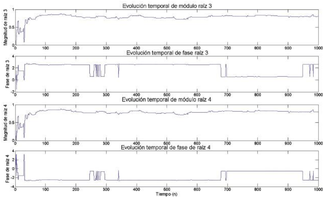
Figura 8.38: Evolución temporal del módulo y fase para la raíz 3 y 4 de la señal mioeléctrica asociada a máxima fuerza de flexión de bíceps.
