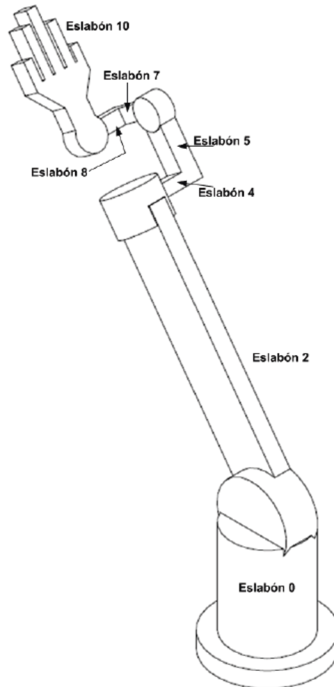
Figura 2.4: Asignación de números a cada eslabón que compone el mecanismo propuesto
