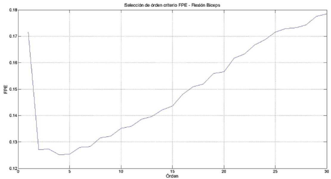
Figura 8.12: Criterio FPE selección de orden de señal EMG asociada a flexión de bíceps (RLS-factor de memoria de 0.99)
