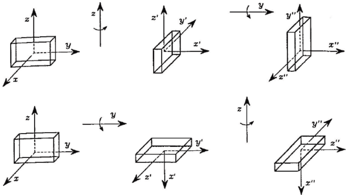
Figura 2.2: Rotaciones alrededor del marco fijo [21]
