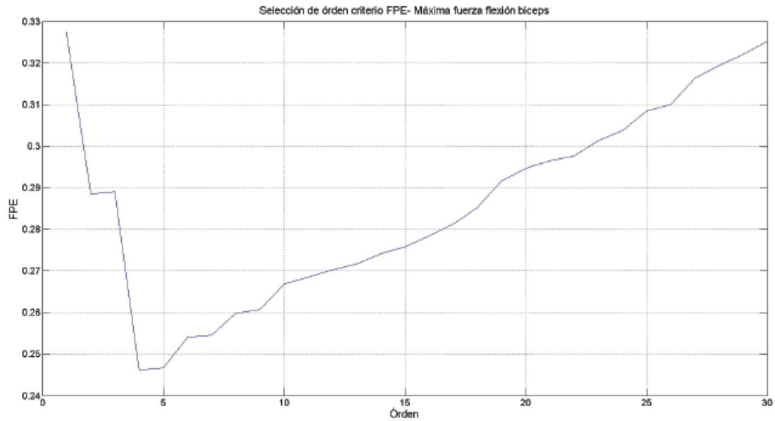
Figura 8.16: Criterio FPE selección de orden de señal EMG asociada a máxima fuerza en flexión de bíceps (RLS-factor de memoria de 0.99)
