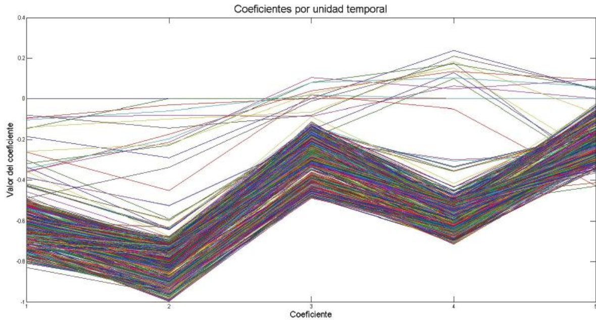
Figura 7.2: Coeficientes por unidad temporal de proceso AR(5) .
