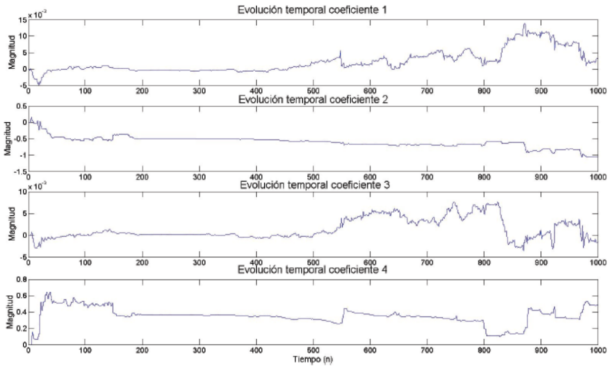
Figura 8.31: Evolución temporal de cada coeficiente de la señal mioeléctrica asociada a extensión de bíceps.
