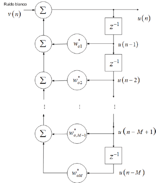
Figura 5.2: Filtro generador de proceso AR
