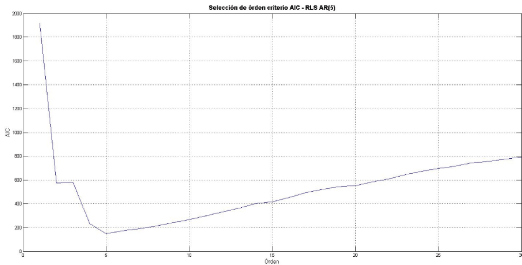
Figura 5.5: Criterio AIC para selección de orden del proceso AR(5) no estacionario
