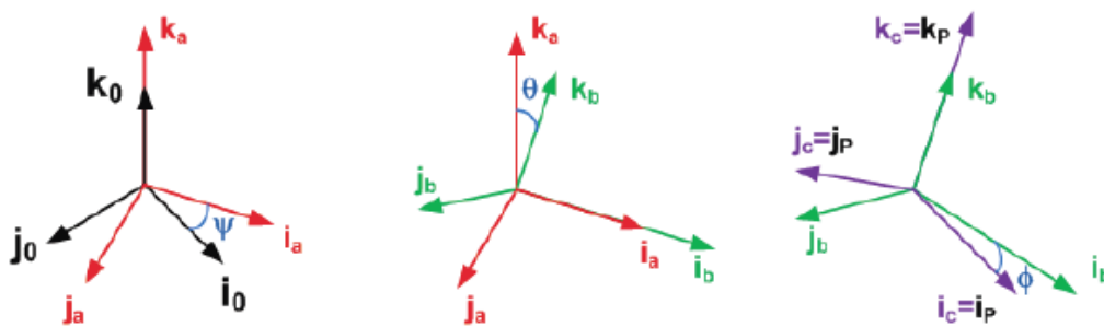
Figura 2.16: Definición de ángulos de Euler de r_P^0
