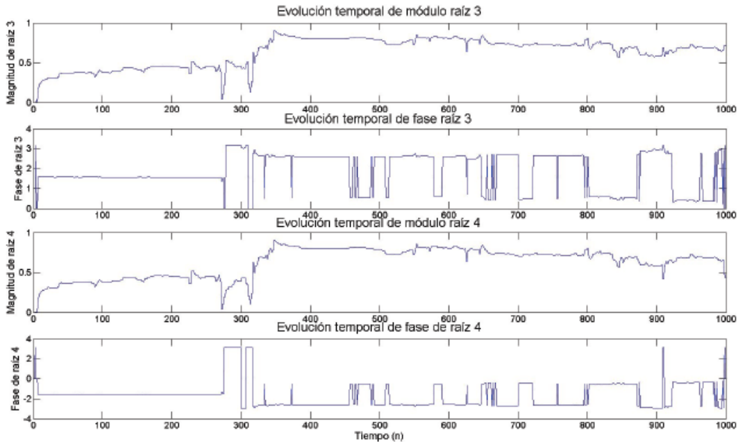
Figura 8.34: Evolución temporal del módulo y fase para la raíz 3 y 4 de la señal mioeléctrica asociada a flexión de bíceps.
