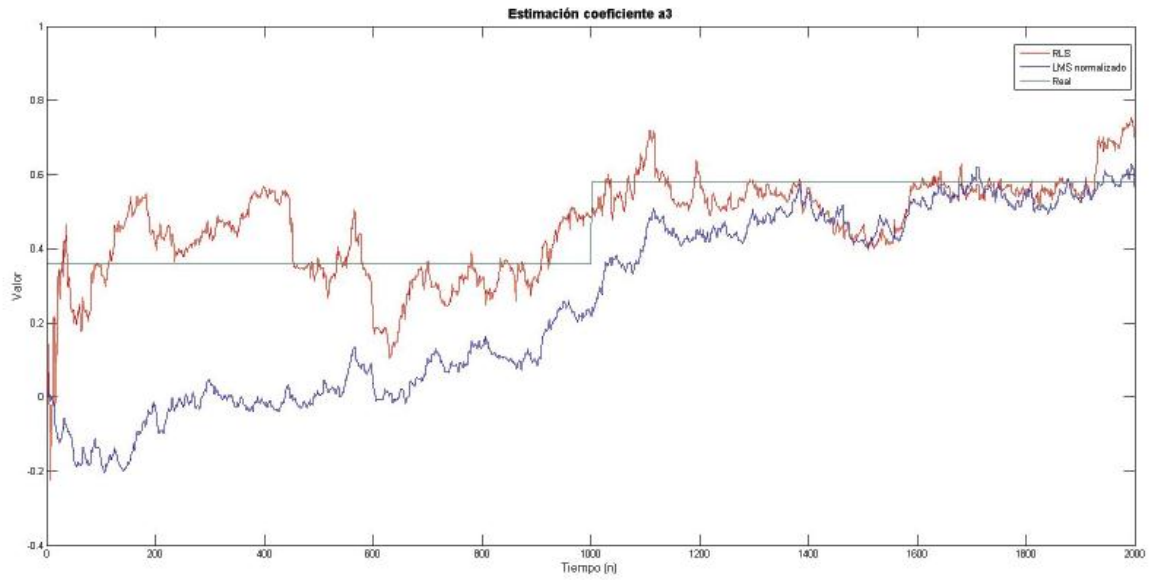
Figura 6.8: Evolución temporal del coeficiente 3 estimado del proceso AR(5) no estacionario
