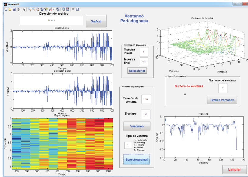
Figura 8.5: Ambiente de trabajo periodograma para señal EMG asociada a flexión de bíceps (Ventana rectangular, tamaño de ventana de 128 y traslape 32)
