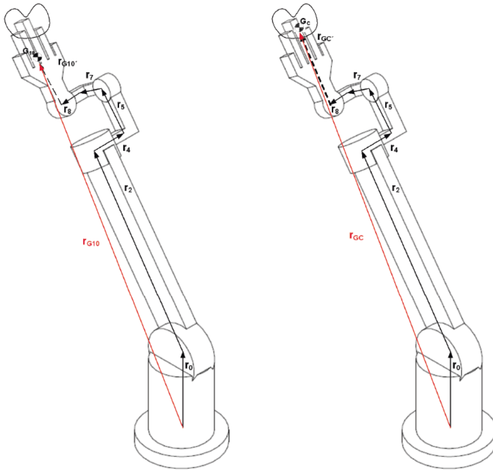
Figura 3.3: Definición de las posiciones de los centros de gravedad (continuación)
