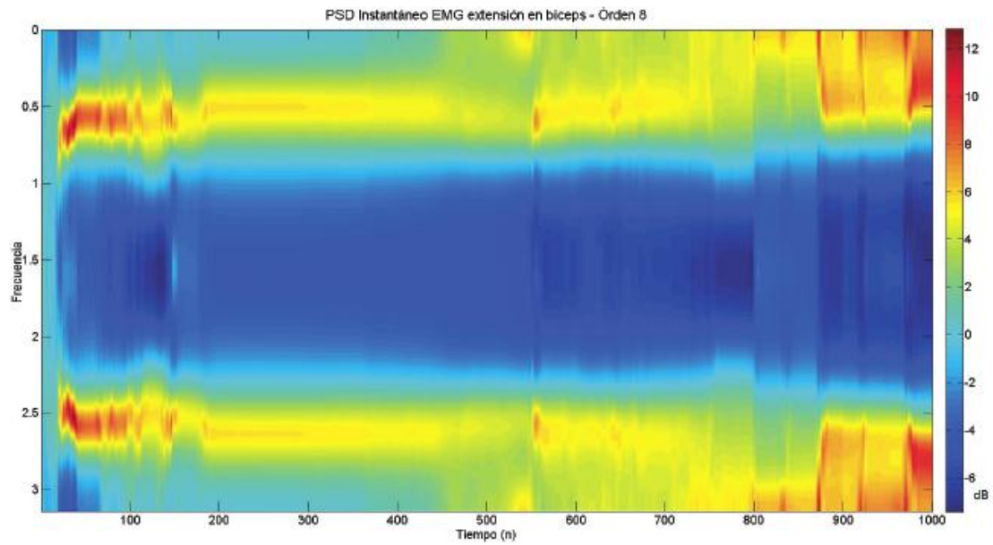
Figura D.4: Evolución temporal de densidades espectrales de potencias estimadas de señal EMG asociada a extensión de bíceps (RLS-factor de memoria de 0.99, orden 8)
