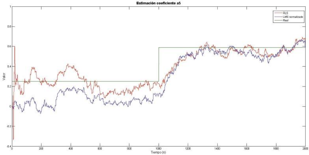
Figura 6.10: Evolución temporal del coeficiente 5 estimado del proceso AR(5) no estacionario
