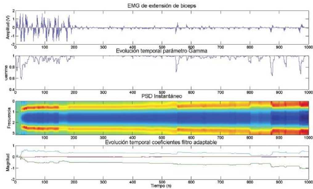
Figura 8.24: Evolución temporal del PSD, del parámetro \gamma y de los coeficientes del filtro para la señal EMG asociada a extensión de bíceps.
