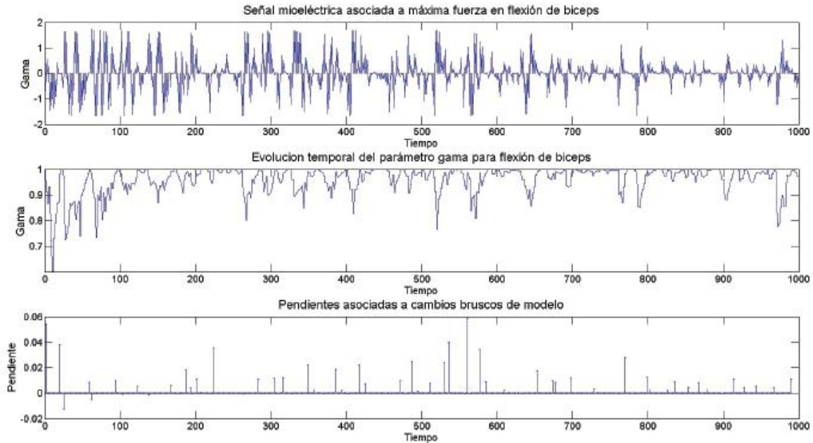
Figura 8.29: Señal mioeléctrica asociada a máxima fuerza de flexión de bíceps, evolución temporal del parámetro \gamma y de las pendientes asociadas a cambios bruscos en \gamma .
