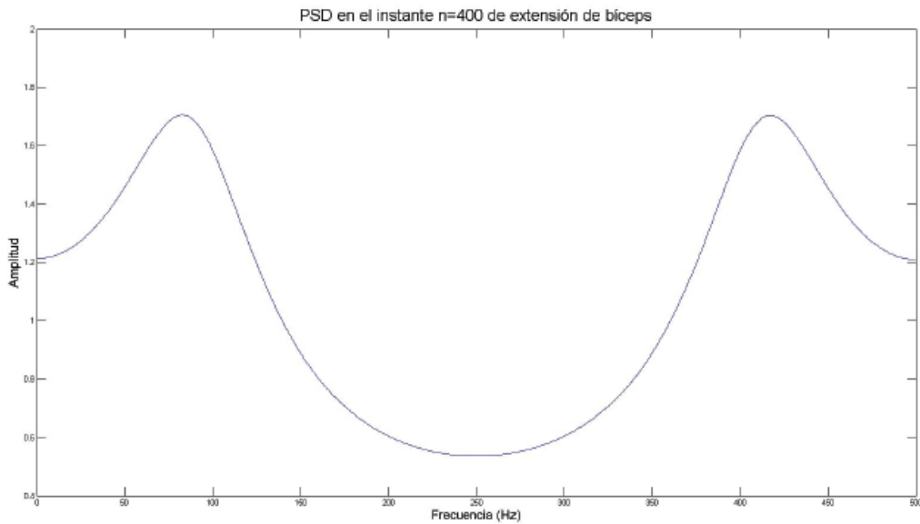
Figura 8.43: PSD en el instante n=400 de extensión de bíceps
