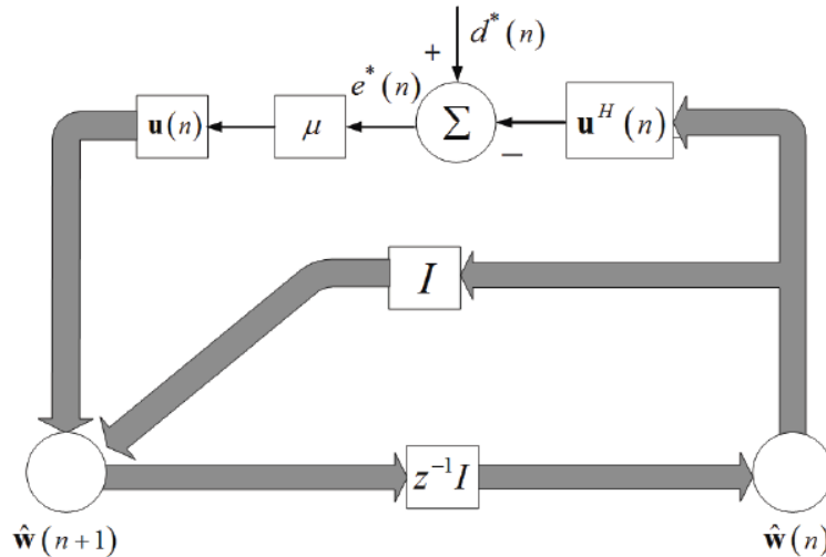
Figura 6.4: Diagrama de flujo del algoritmo LMS
