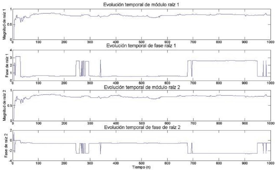
Figura 8.37: Evolución temporal del módulo y fase para la raíz 1 y 2 de la señal mioeléctrica asociada a máxima fuerza de flexión de bíceps.
