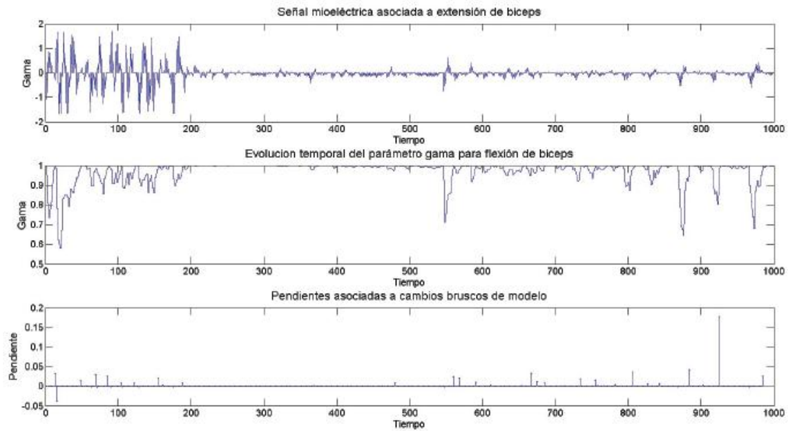
Figura 8.28: Señal mioeléctrica asociada a extensión de bíceps, evolución temporal del parámetro \gamma y de las pendientes asociadas a cambios bruscos en \gamma .
