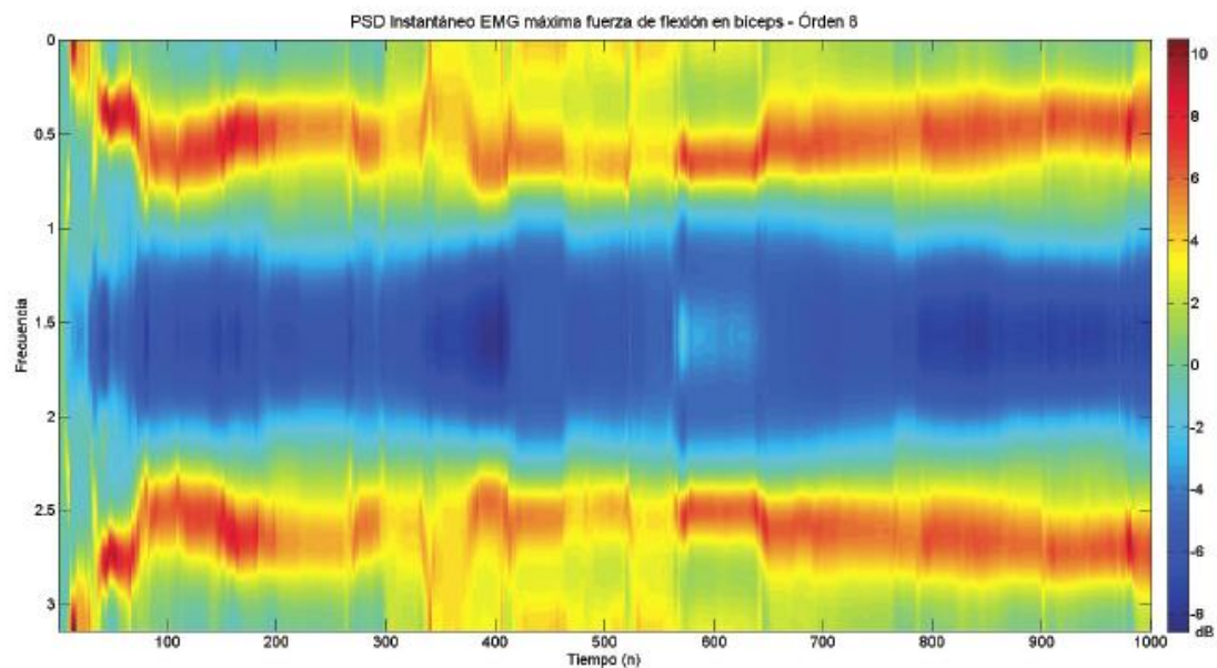
Figura D.6: Evolución temporal de densidades espectrales de potencias estimadas de señal EMG asociada a máxima fuerza de flexión de bíceps (RLS-factor de memoria de 0.99, orden 8)
