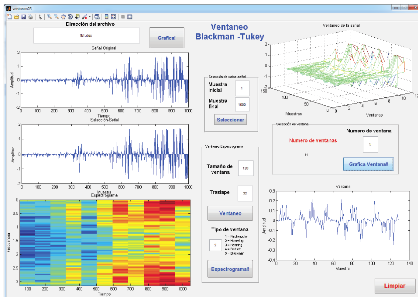
Figura 8.6: Ambiente de trabajo Blackman-Tukey para señal EMG asociada a flexión de bíceps (Ventana Hamming, tamaño de ventana de 128 y traslape 32)
