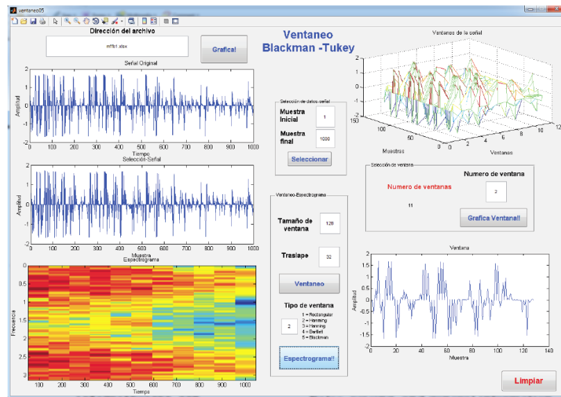
Figura 8.10: Ambiente de trabajo Blackman-Tukey para señal EMG asociada a máxima fuerza de flexión de bíceps (Ventana Hamming, tamaño de ventana de 128 y traslape 32)
