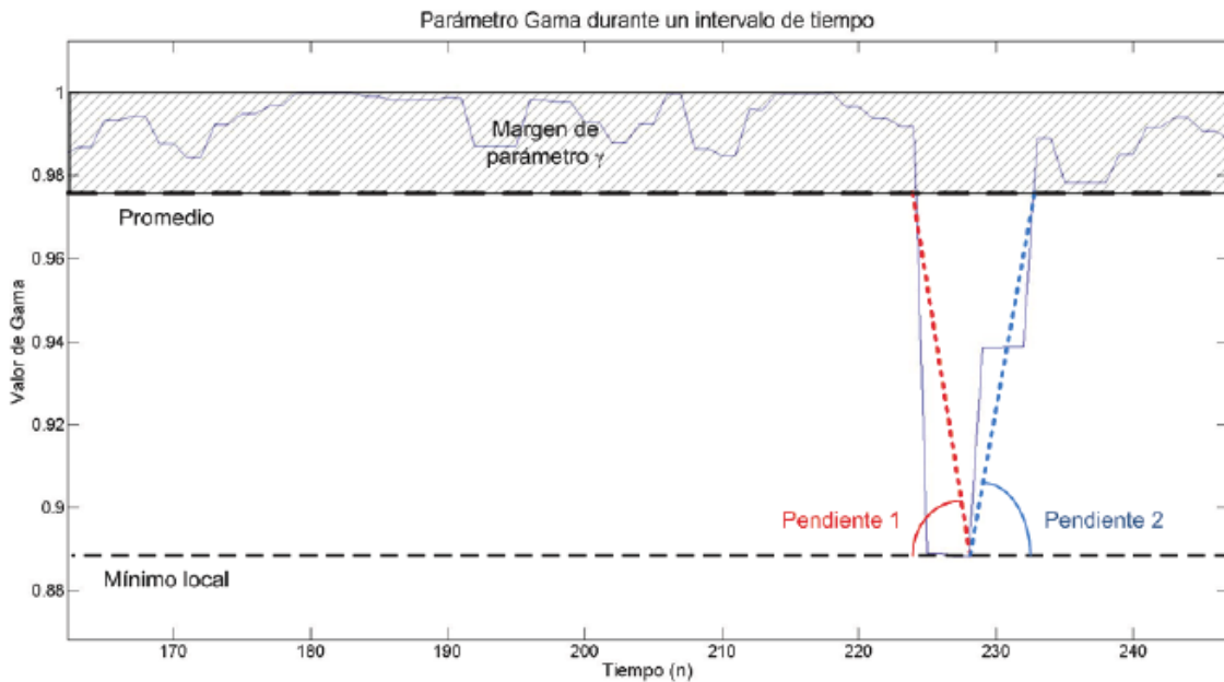
Figura 8.26: Parámetro \gamma dentro de un intervalo de tiempo y características dentro de la zona fuera del margen establecido.
