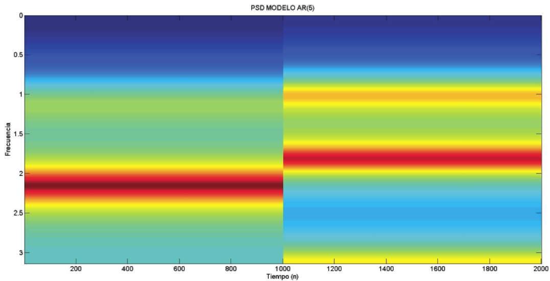
Figura 6.11: Evolución temporal de densidades espectrales de potencias teóricas del proceso AR(5) no estacionario
