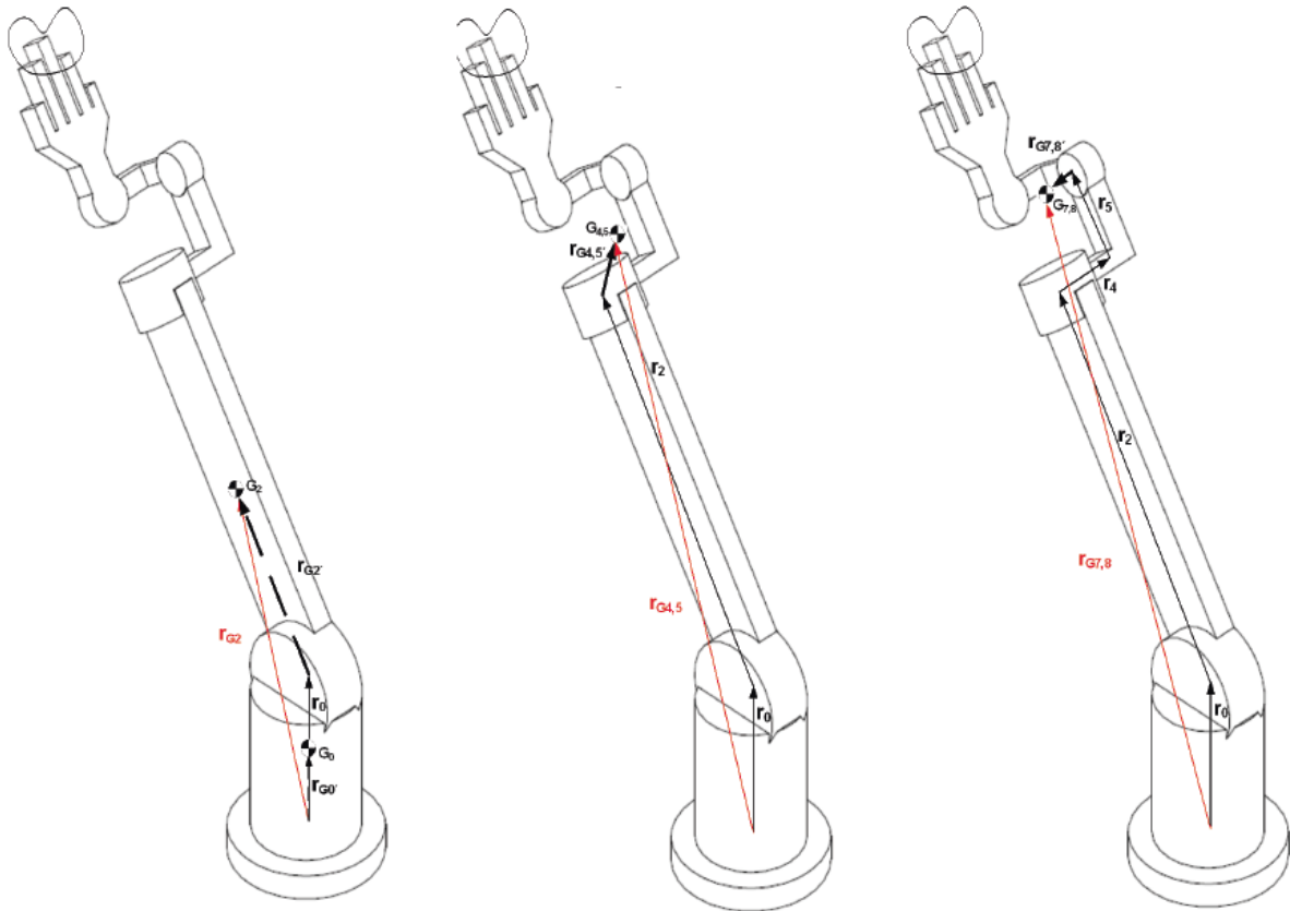
Figura 3.2: Definición de las posiciones de los centros de gravedad
