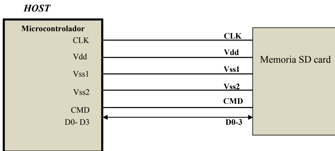
Figura 2.4. Topología del bus SD.
