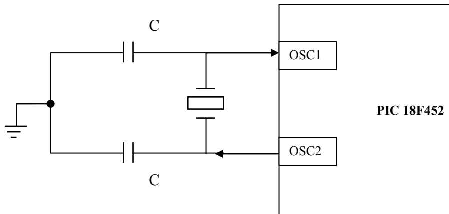
Figura 3.4. Circuito oscilador externo basado en cristal de cuarzo.
