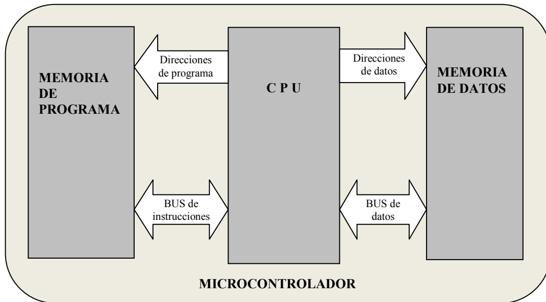
Figura 2.32. Arquitectura Harvard.
