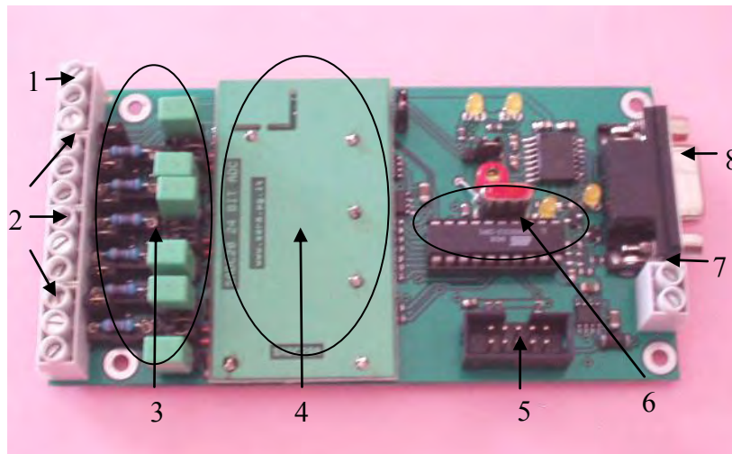
Figura 2.27. Tarjeta SADC20.
