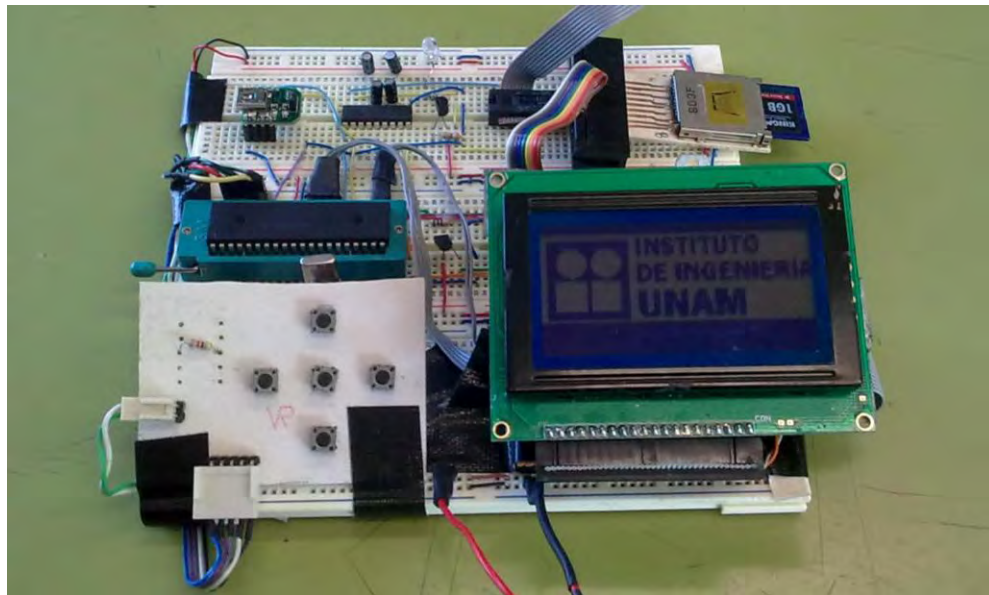
Figura 4.1. Hardware de la interfaz montado en tarjetas protoboard.
