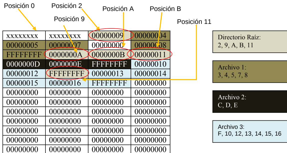
Figura 2.23. Seguimiento de los archivos en una tabla FAT.
