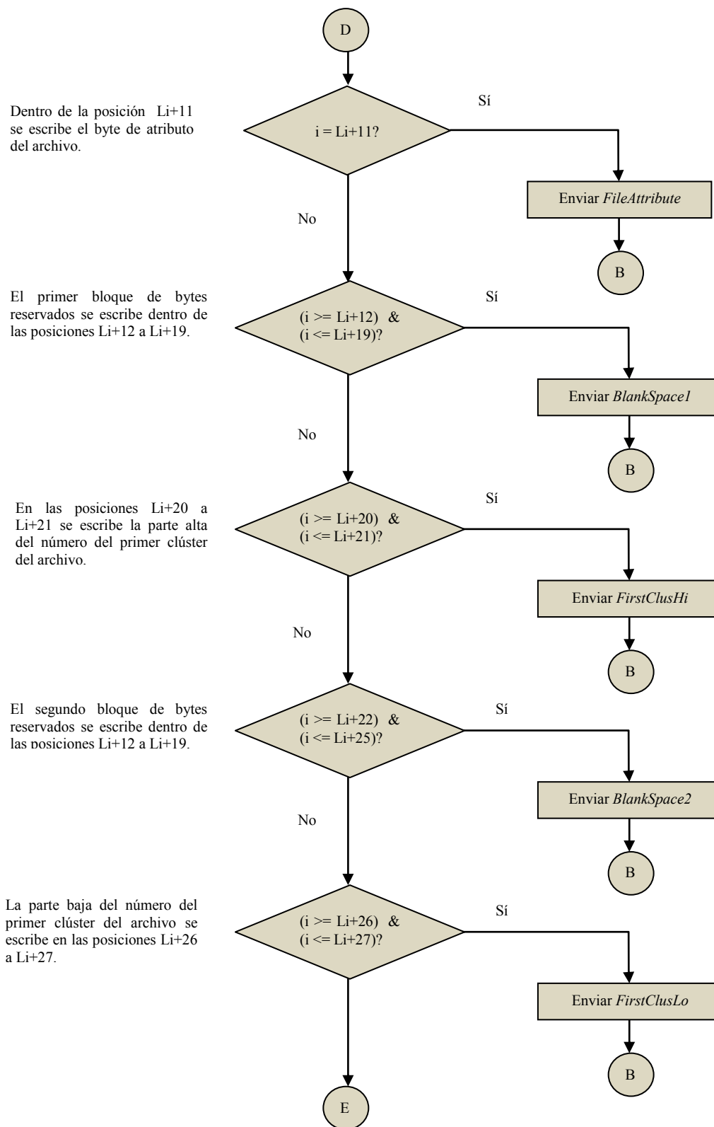
Figura 3.58. Diagrama de la función WriteRootDir (2 de 3).
