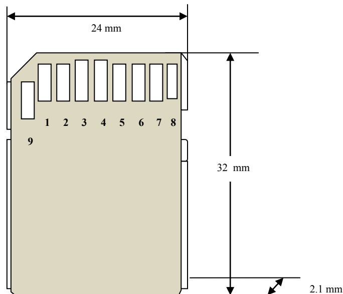
Figura 3.5. Disposición de terminales en una tarjeta de memoria SD.
