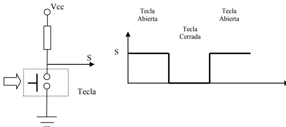
Figura 2.33. Comportamiento ideal de una tecla o botón.
