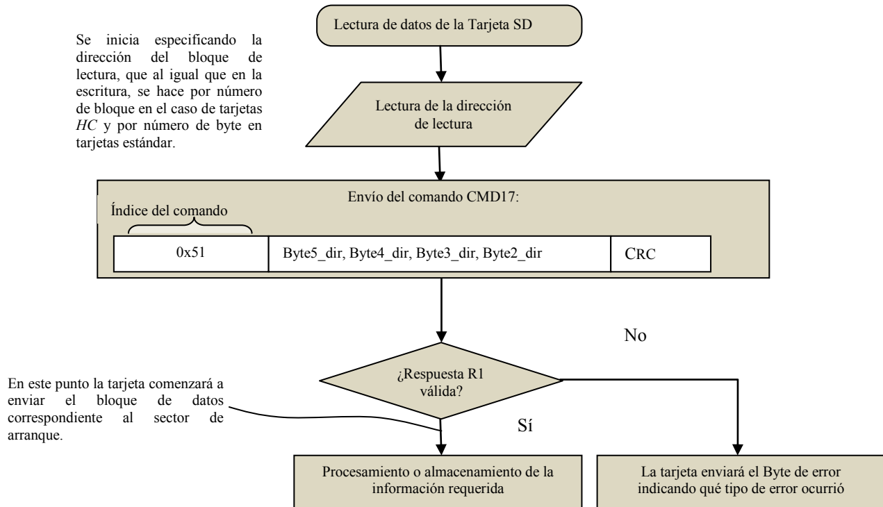
Figura 3.20. Diagrama de flujo para la lectura de datos de la memoria SD.
