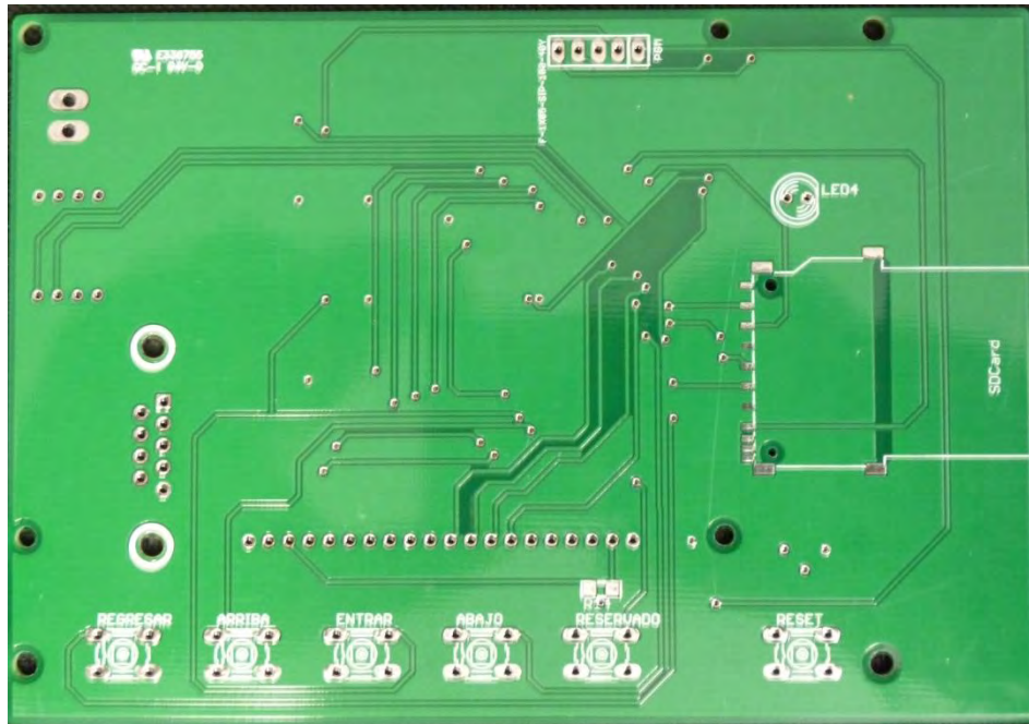
Figura 4.46. Fotografía de la parte superior de la placa fabricada.
