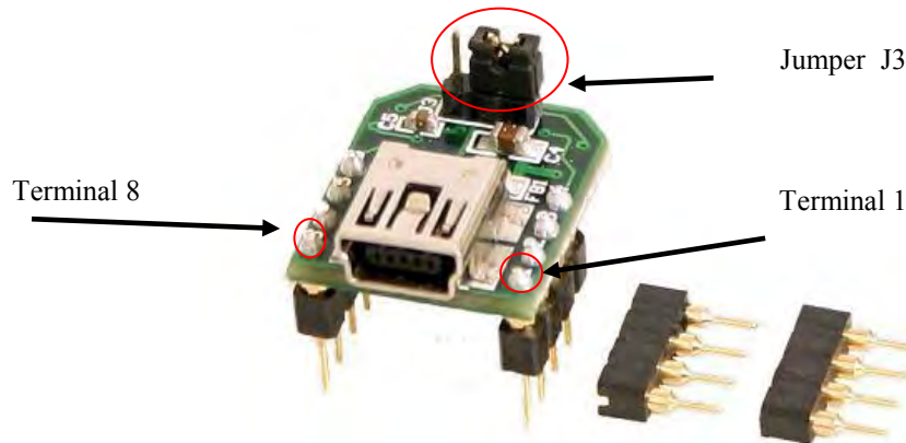
Figura 3.8. Módulo UB232R.
