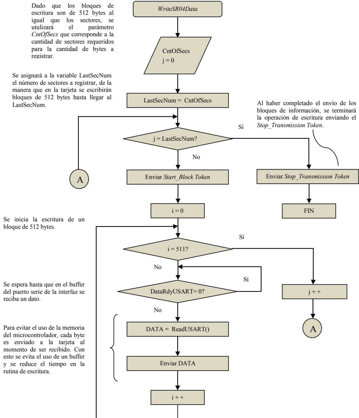
Figura 3.62. Diagrama de la función de registro de los datos de la unidad sísmica SR04 en las tarjetas de memorias SD.
