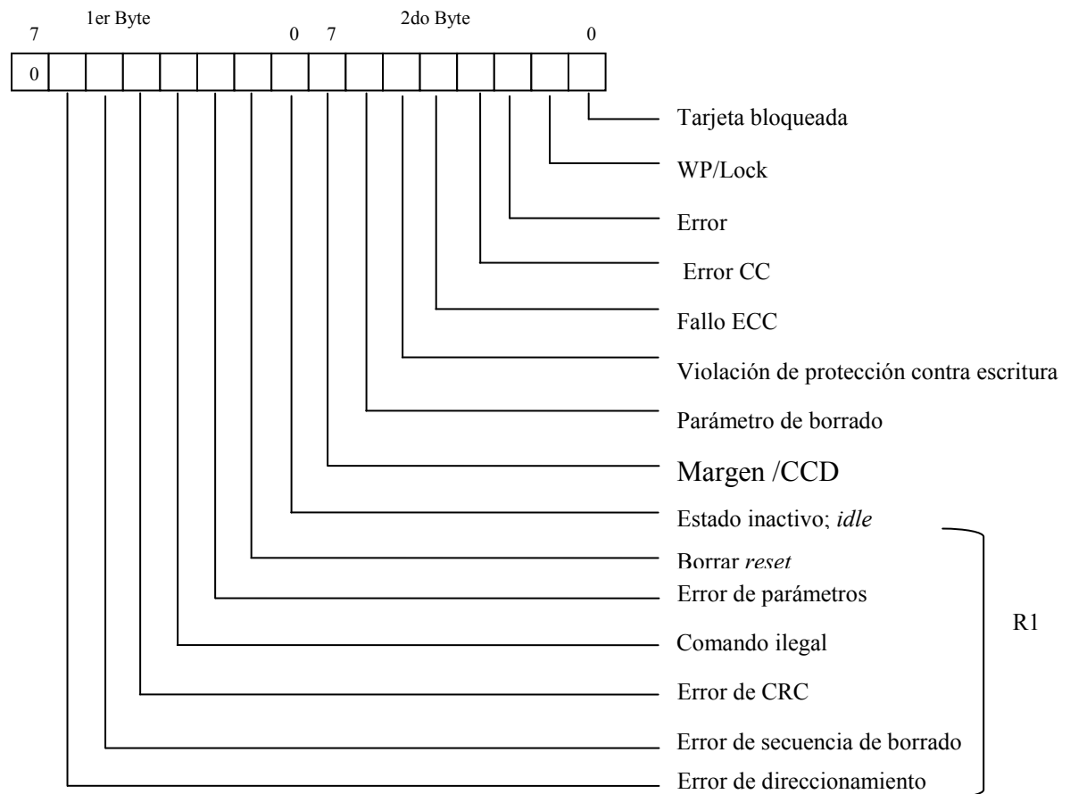
Figura 2.12. Formato de la respuesta R2.
