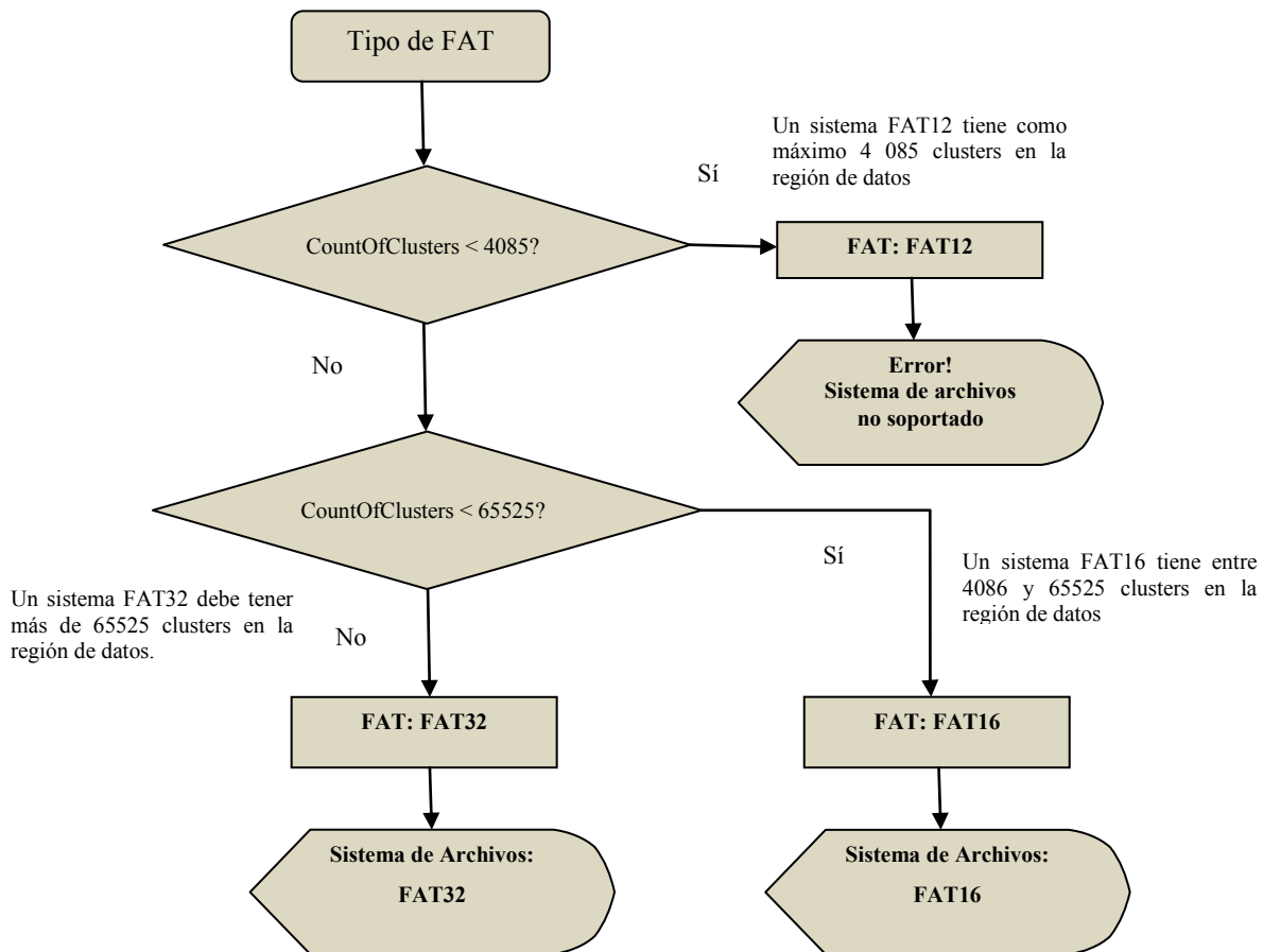
Figura 3.25. Determinación del tipo de sistema de archivos.
