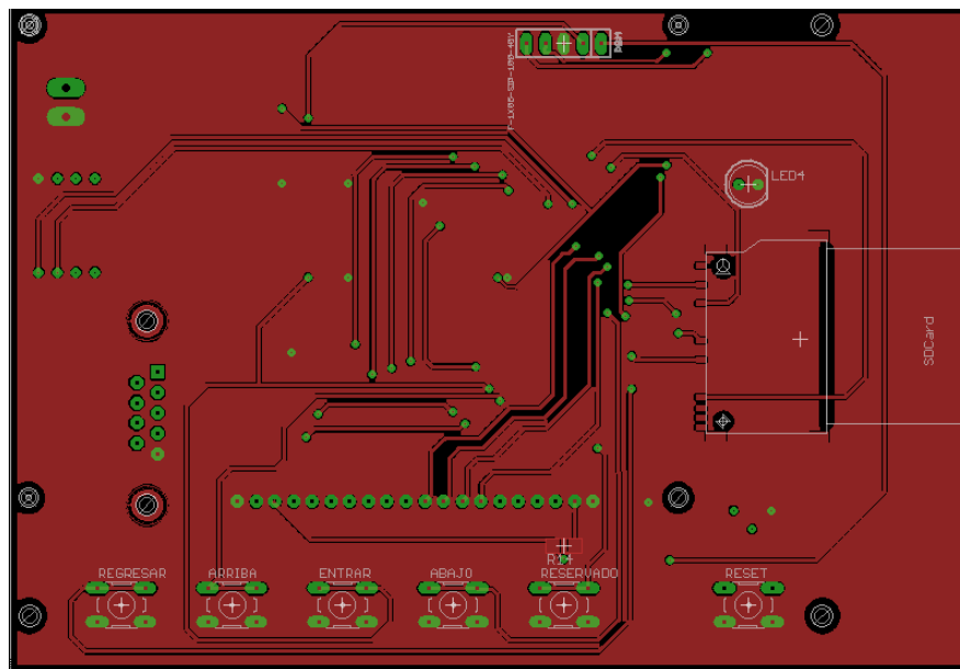
Figura 4.44. Cara superior del PCB de la interfaz de registro.
