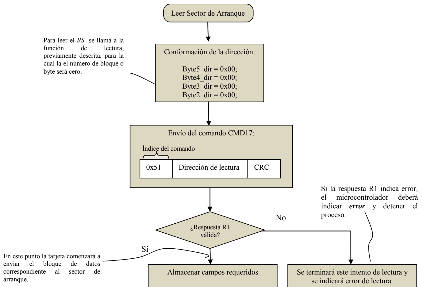
Figura 3.21. Secuencia de lectura del sector de arranque.
