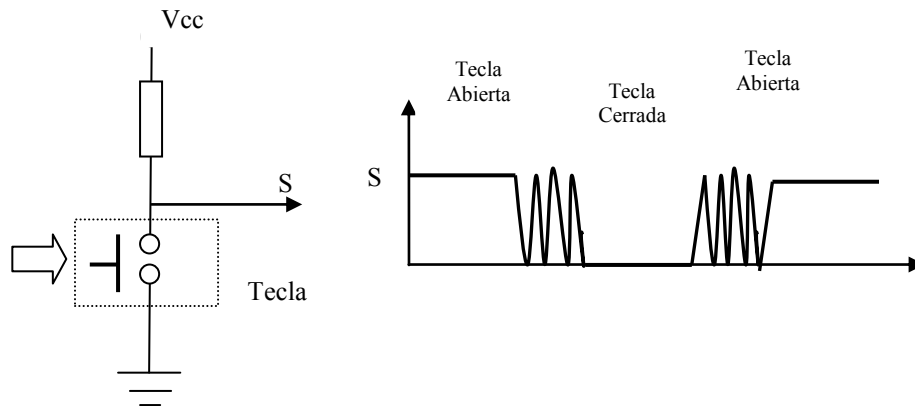
Figura 2.34. Efecto de rebote mecánico al pulsar una tecla.
