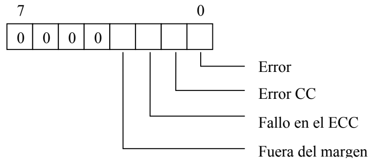
Figura 2.20. Bloque ‘Señal de error de datos’.
