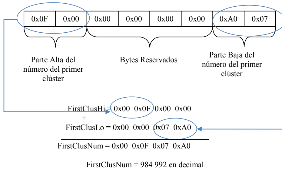
Figura 3.29. Conformación del número del primer clúster.
