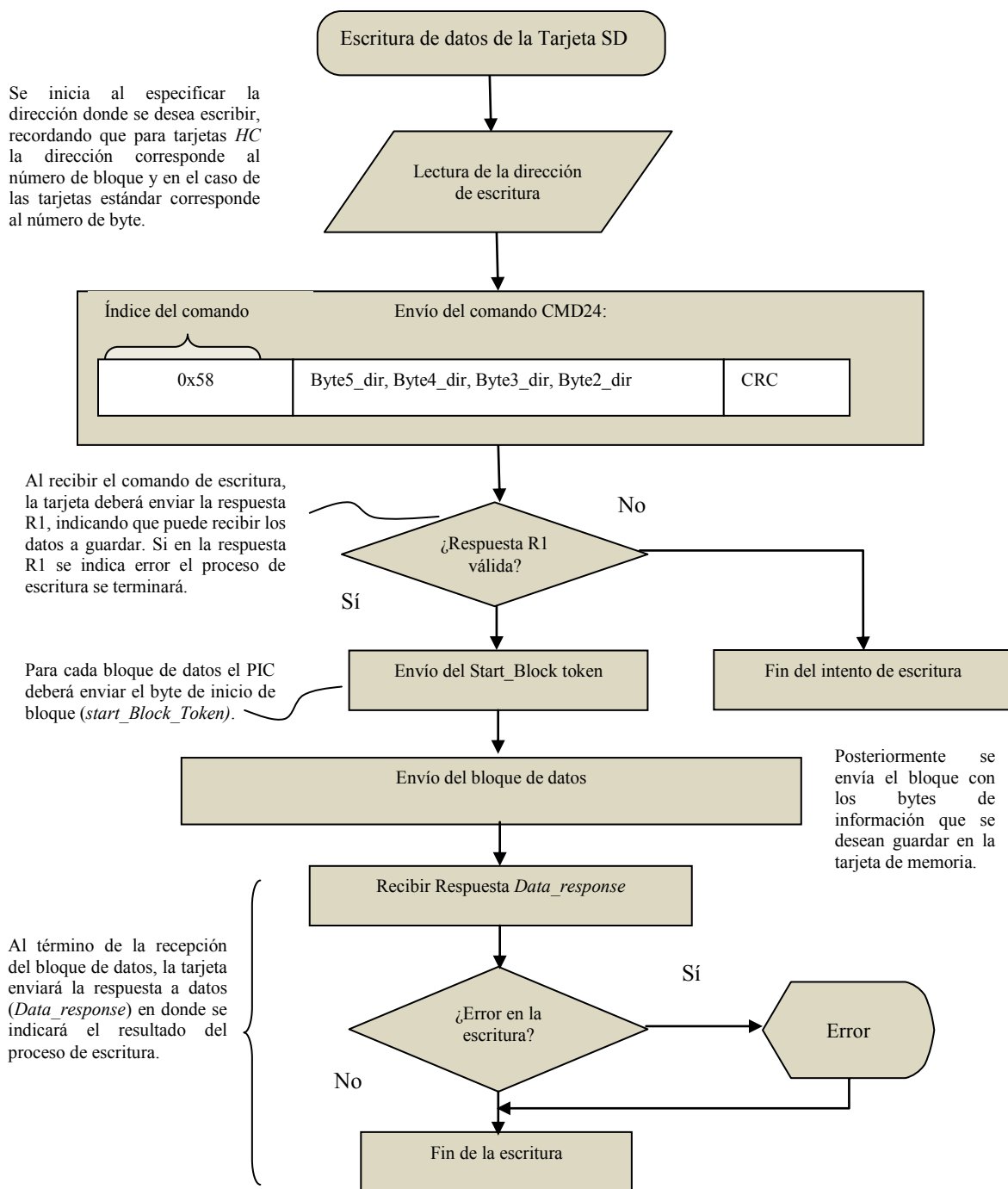
Figura 3.19. Diagrama de flujo para la escritura de datos en la memoria SD.
