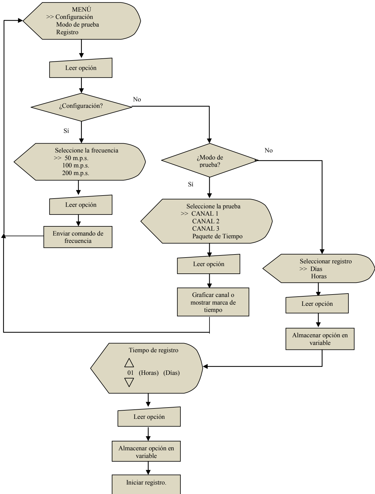
Figura 3.48. Diagrama de flujo de los menús mostrados en el display gráfico.
