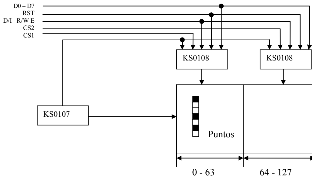
Figura 3.10. Bloques internos del display gráfico JHD12864E.
