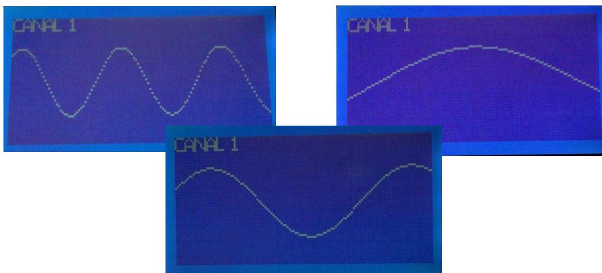
Figura 4.12. Gráficas obtenidas del canal 1 a 50, 100 y 200 mps.
