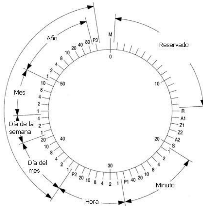
Figura 2.28. Codificación de los datos de tiempo enviados por un transmisor DCF77.
