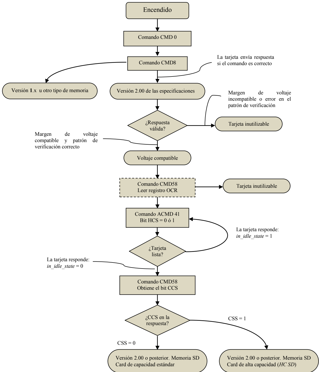
Figura 2.6. Diagrama de flujo de la inicialización de la tarjeta de memoria SD en el modo SPI.
