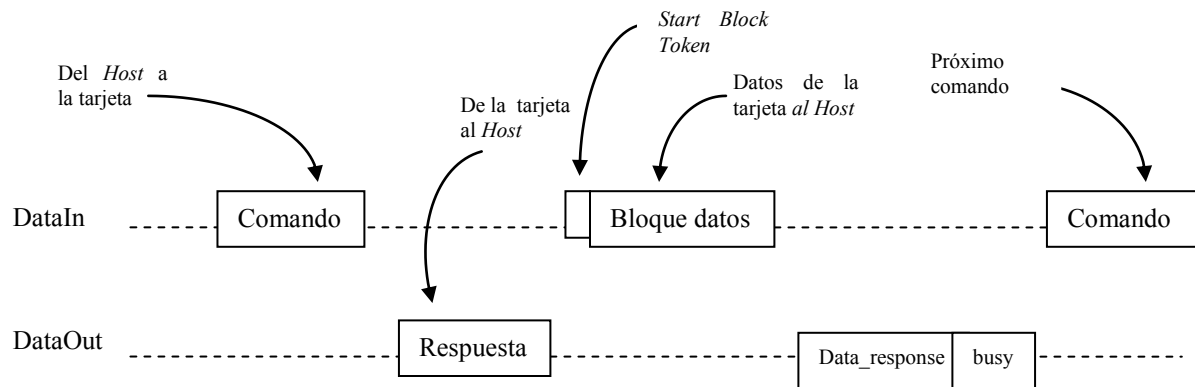
Figura 2.9. Diagrama de la operación de escritura de un bloque de datos.
