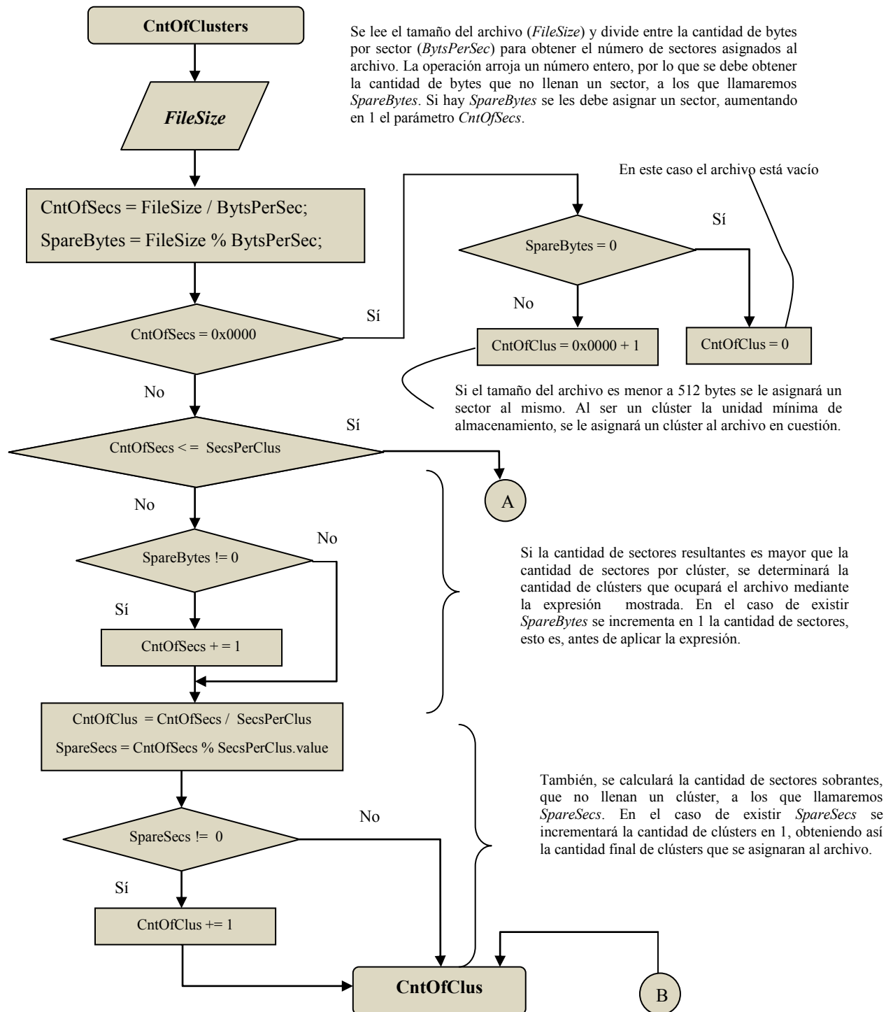
Figura 3.31. Determinación de la cantidad de clústers para un archivo (1 de 2).
