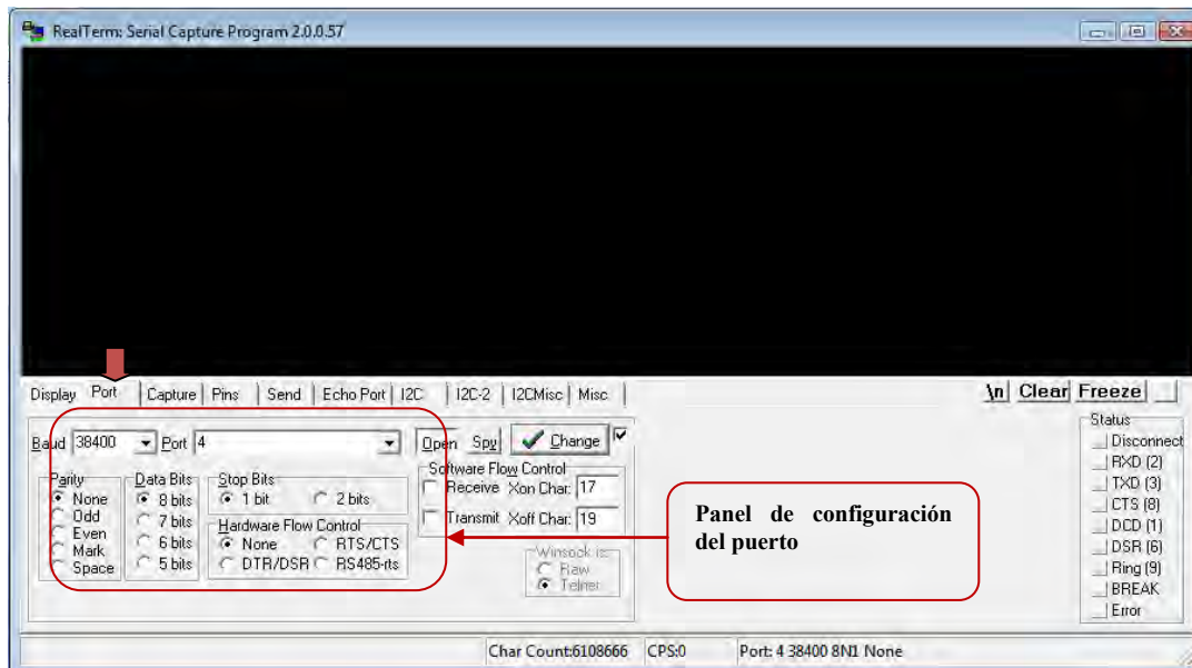
Figura 4.15. Configuración del puerto mediante el programa RealTerm.
