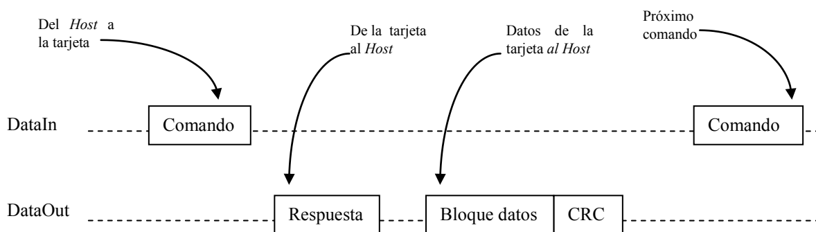
Figura 2.7. Diagrama de la operación de lectura de un bloque de datos.
