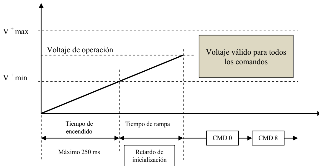
Figura 3.13. Secuencia de encendido de la tarjeta de memoria SD.
