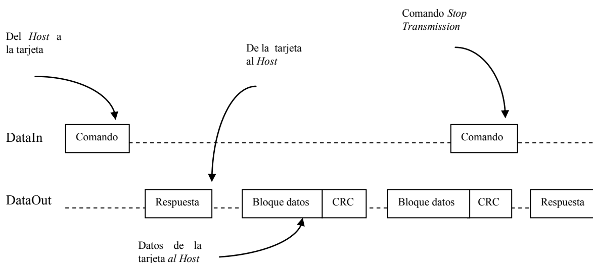
Figura 2.8. Diagrama de la operación de lectura múltiple de bloques de datos.
