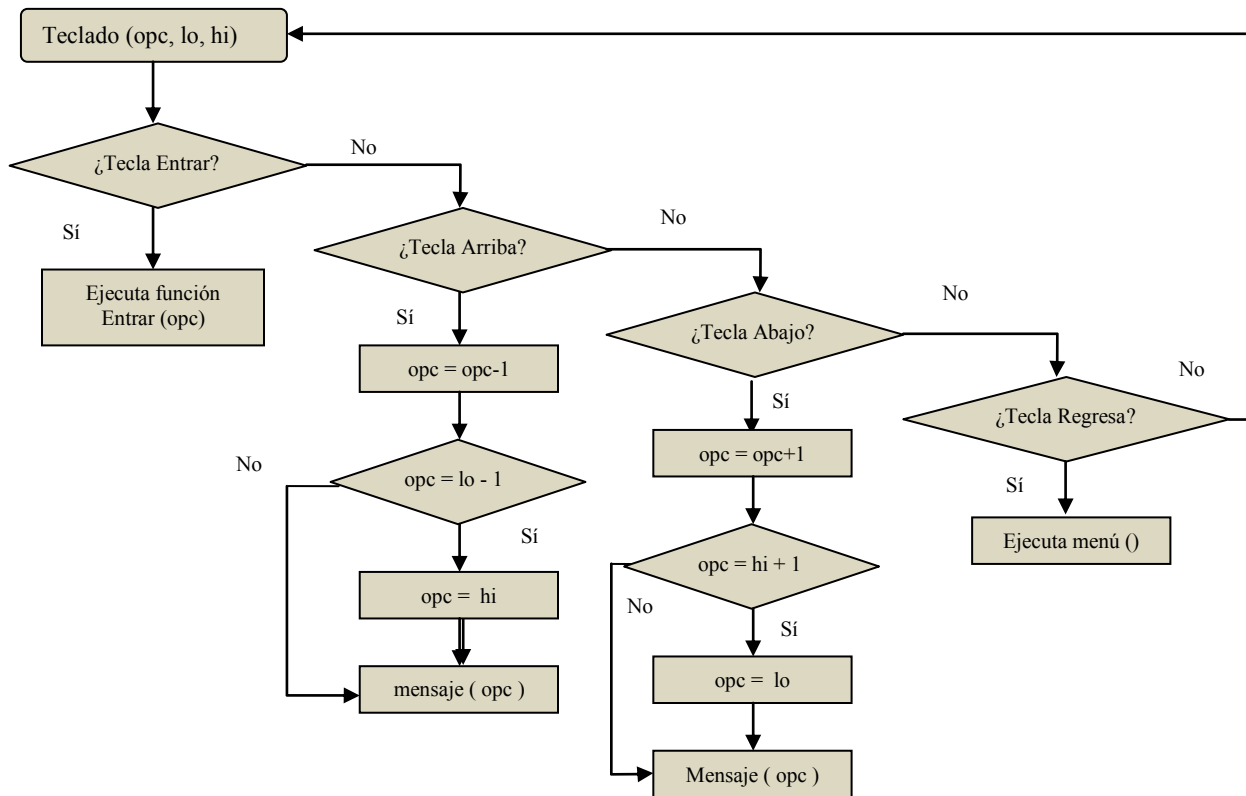
Figura 3.44. Diagrama de flujo del manejo del teclado.
