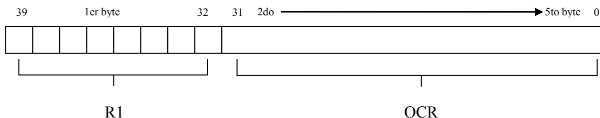
Figura 2.13. Formato de la respuesta R3.
