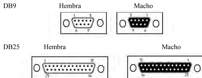
Figura 2.39. Conectores DB9 y DB25 para la comunicación serial RS 232.
