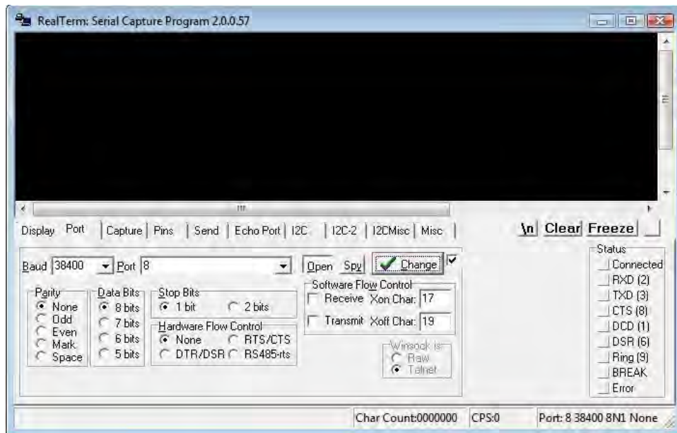
Figura 3.39. Panel de opciones del software RealTerm Serial Capture.
