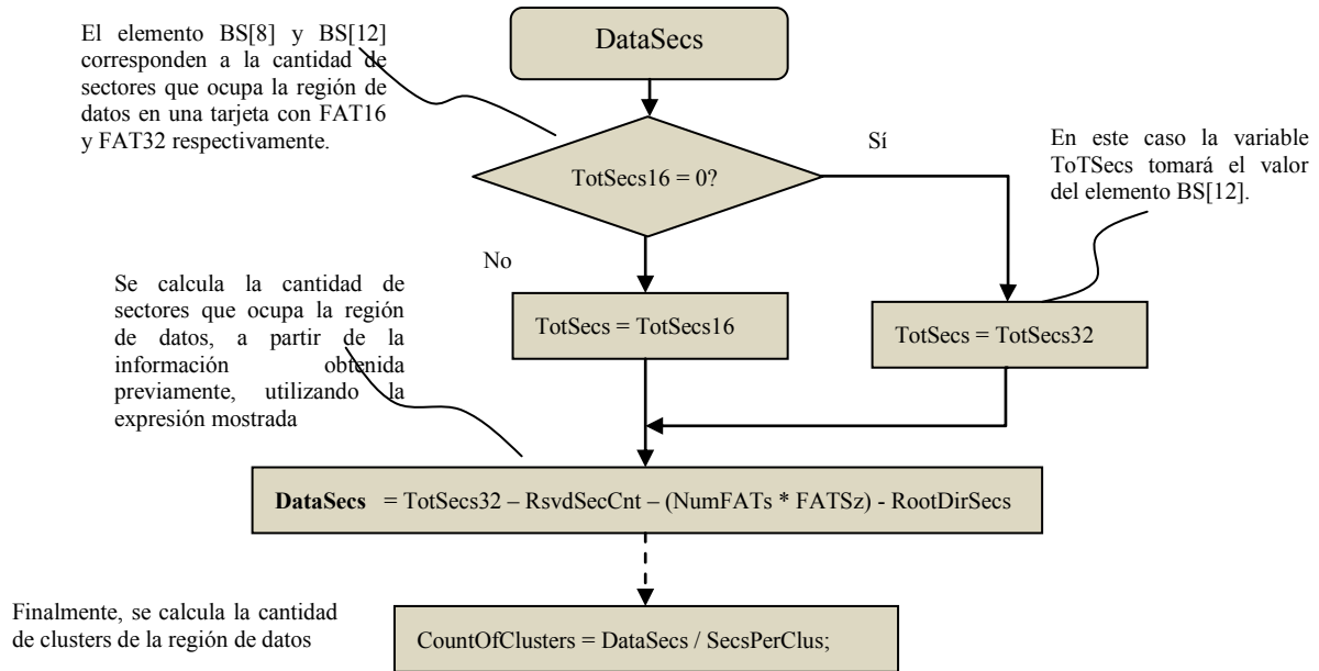
Figura 3.24. Cálculo de la cantidad de sectores en la región de datos.
