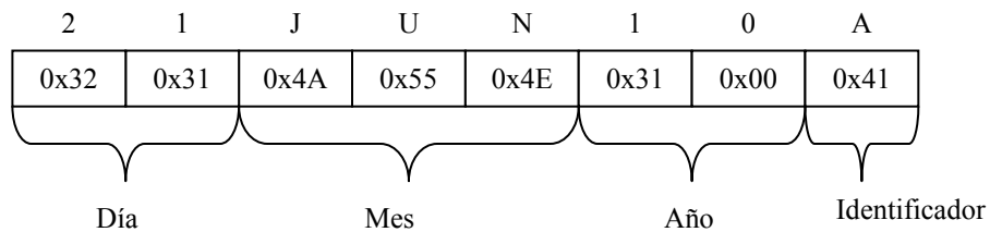
Figura 3.30. Disposición del nombre del archivo en la entrada del directorio raíz.
