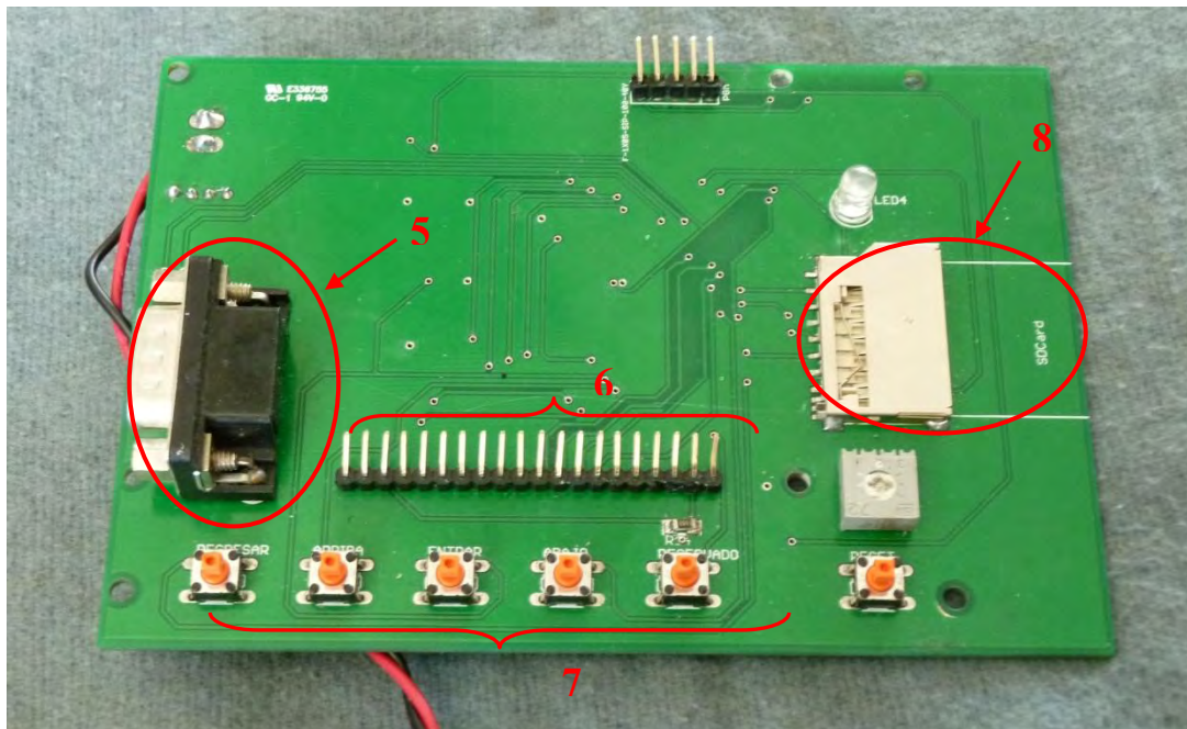
Figura 4.48. Lado superior de la tarjeta final de la Interfaz de registro.
