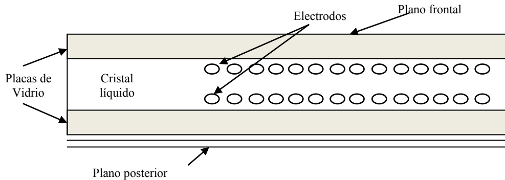
Figura 2.36. Estructura básica de un display LCD.
