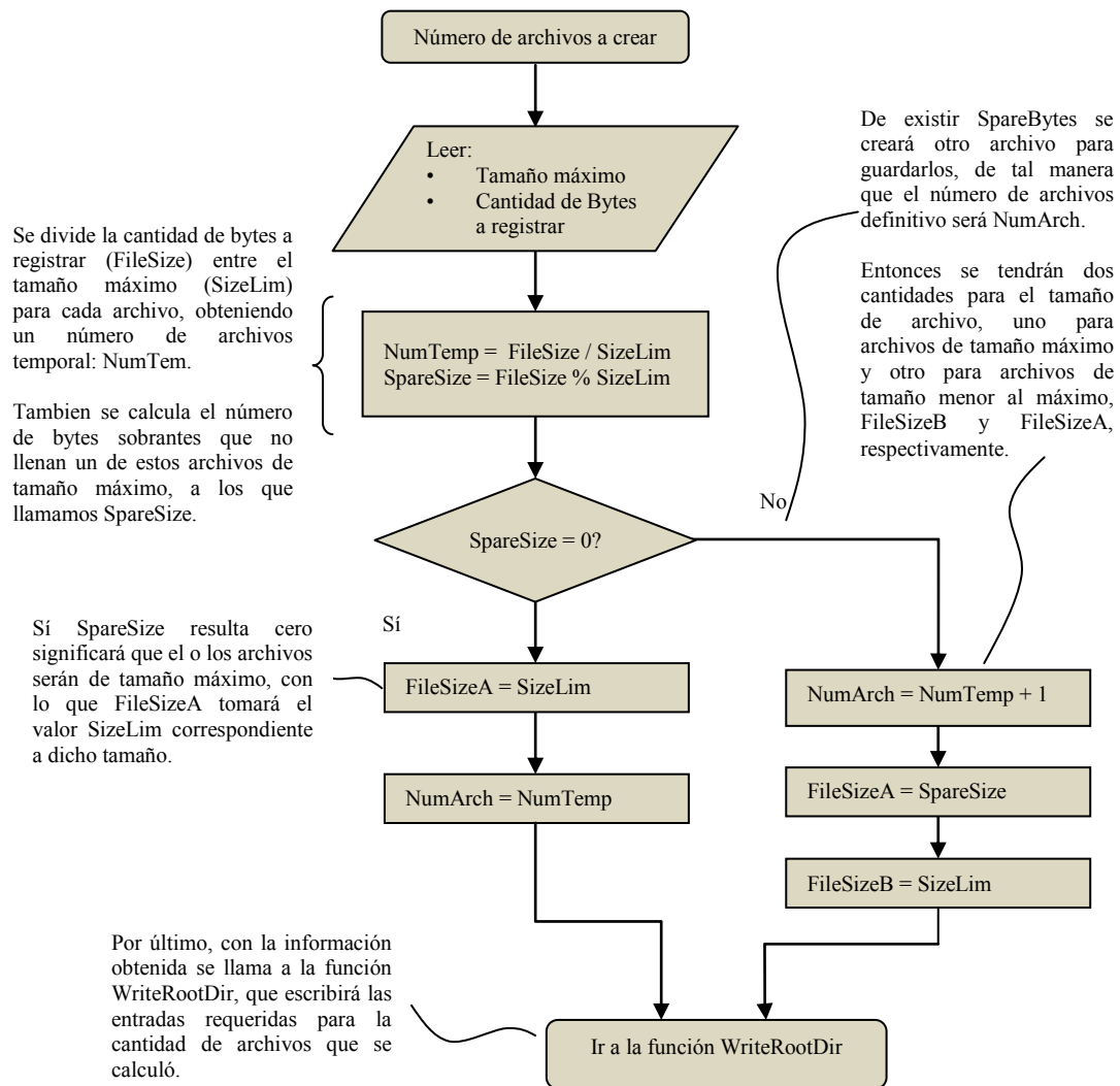
Figura 3.56. Determinación de la cantidad de archivos que se crearán.
