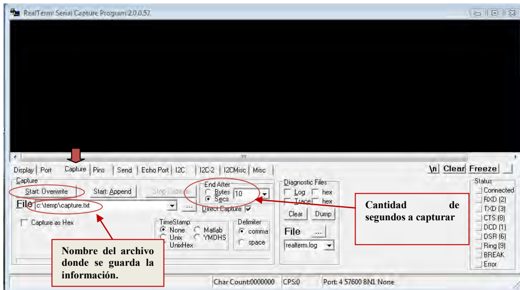
Figura 4.16. Opciones de captura en RealTerm.
