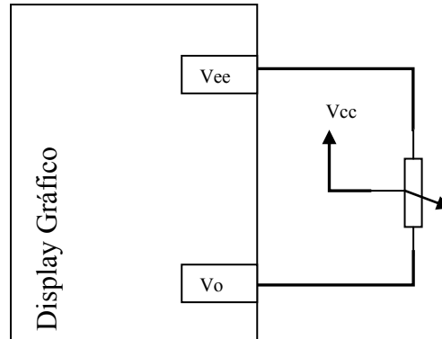
Figura 3.12. Circuito de ajuste del contraste del display gráfico.
