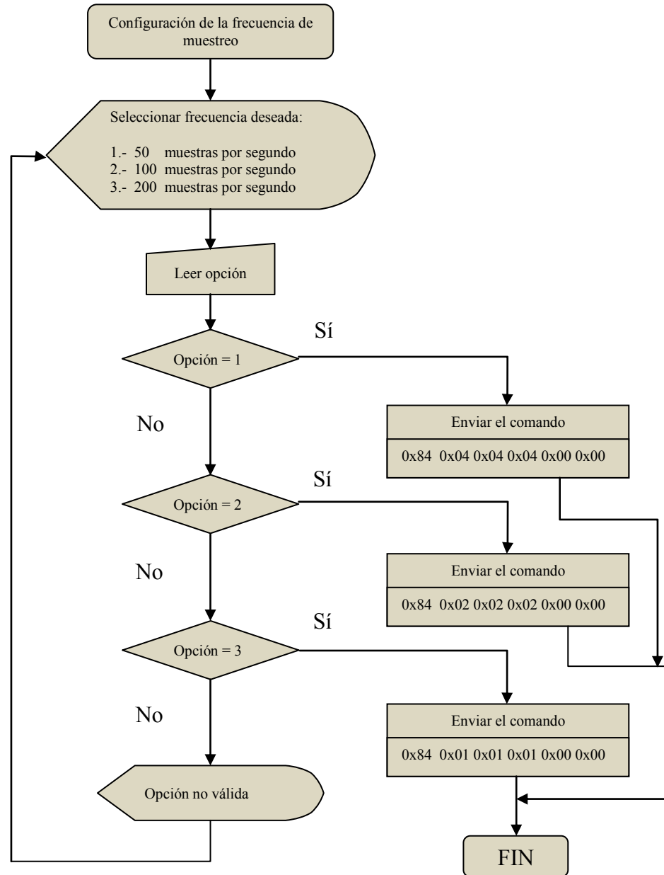
Figura 3.43. Diagrama de flujo para la función de configuración de la frecuencia de muestreo de la unidad sísmica SR04.
