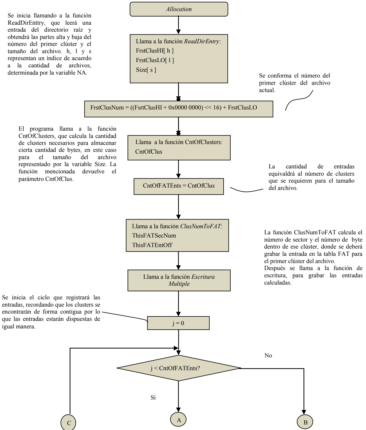
Figura 3.60. Diagrama de la función Allocation (1 de 2).
