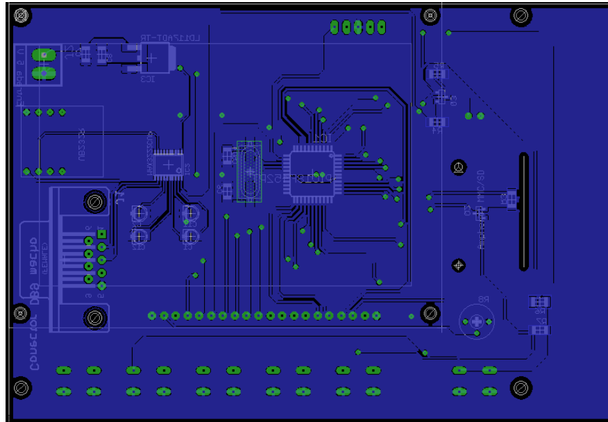
Figura 4.43. Cara inferior del PCB de la interfaz de registro.
