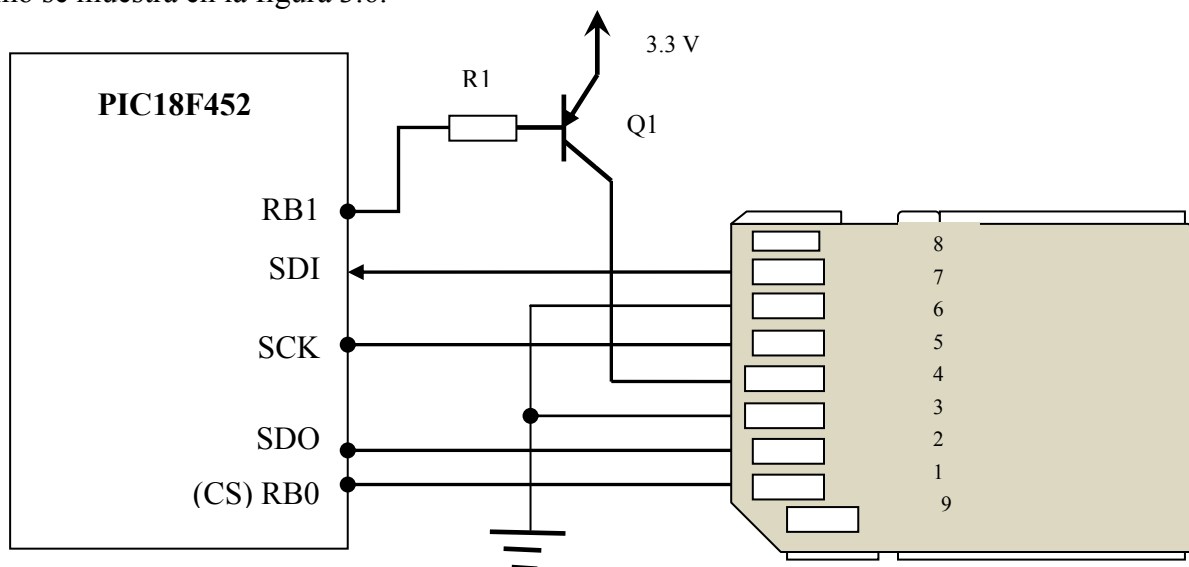
Figura 3.6. Conexión de la tarjeta SD con el microcontrolador.
