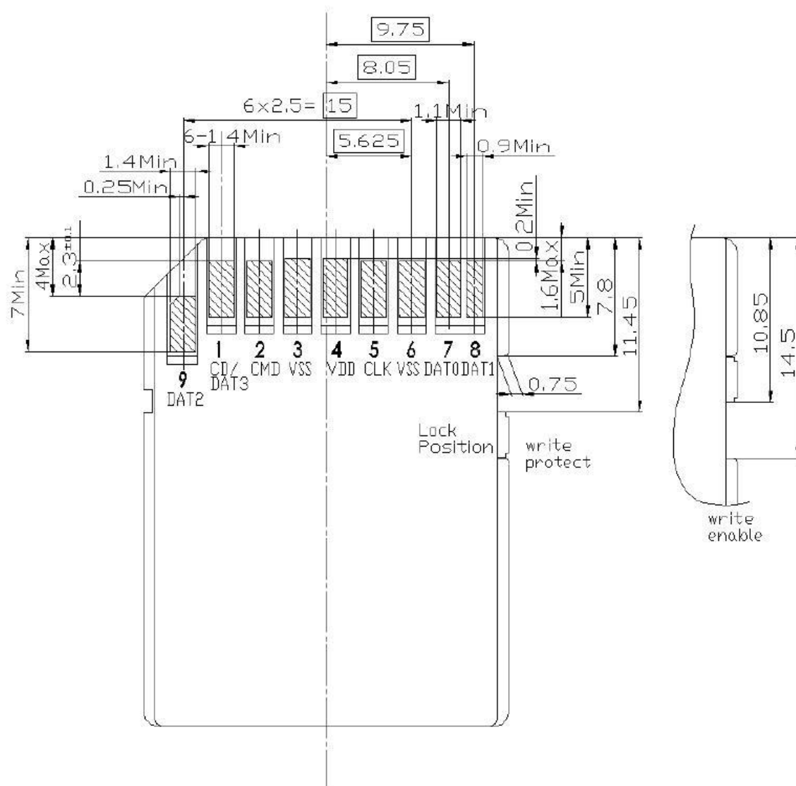
Figura 2.2. Forma y dimensiones de las tarjetas de memoria flash SD.
