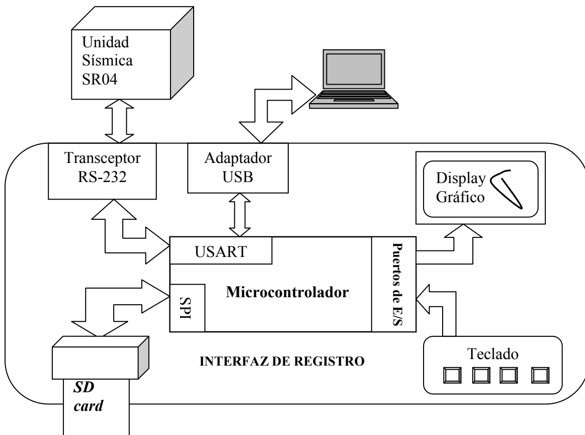
Figura 3.1. Elementos que conformarán el Hardware del sistema.
