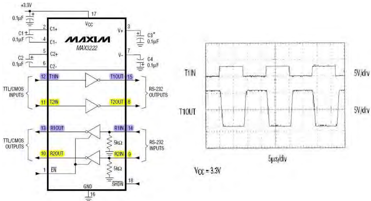
Figura 2.40. Transceptor MAX 3222 para comunicación serial RS 232.
