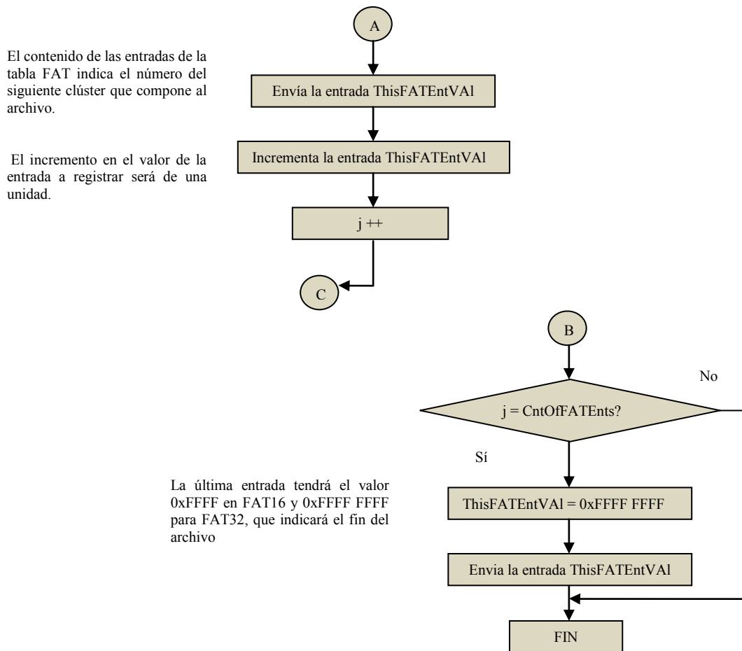
Figura 3.61. Diagrama de la función Allocation (2 de 2).
