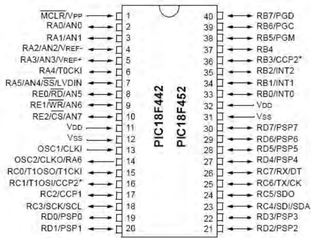
Figura 3.3. Aspecto del microcontrolador PIC18LF452 en empaque DIP.
