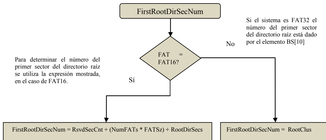
Figura 3.26. Determinación del primer sector del directorio raíz.
