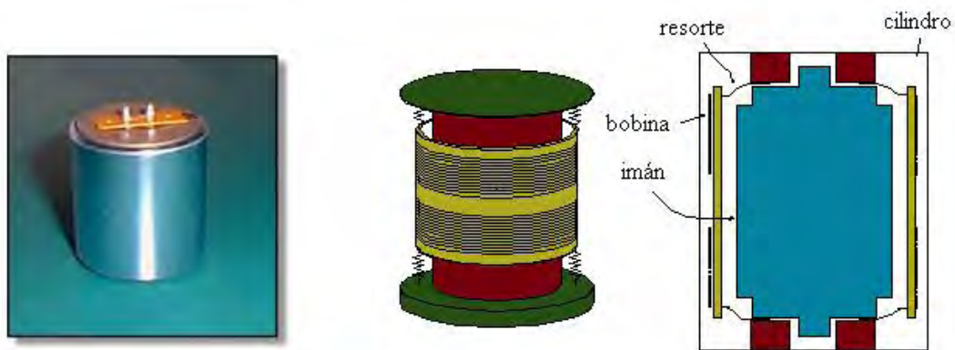
Figura 2.26. Geófono GS – 11D.
