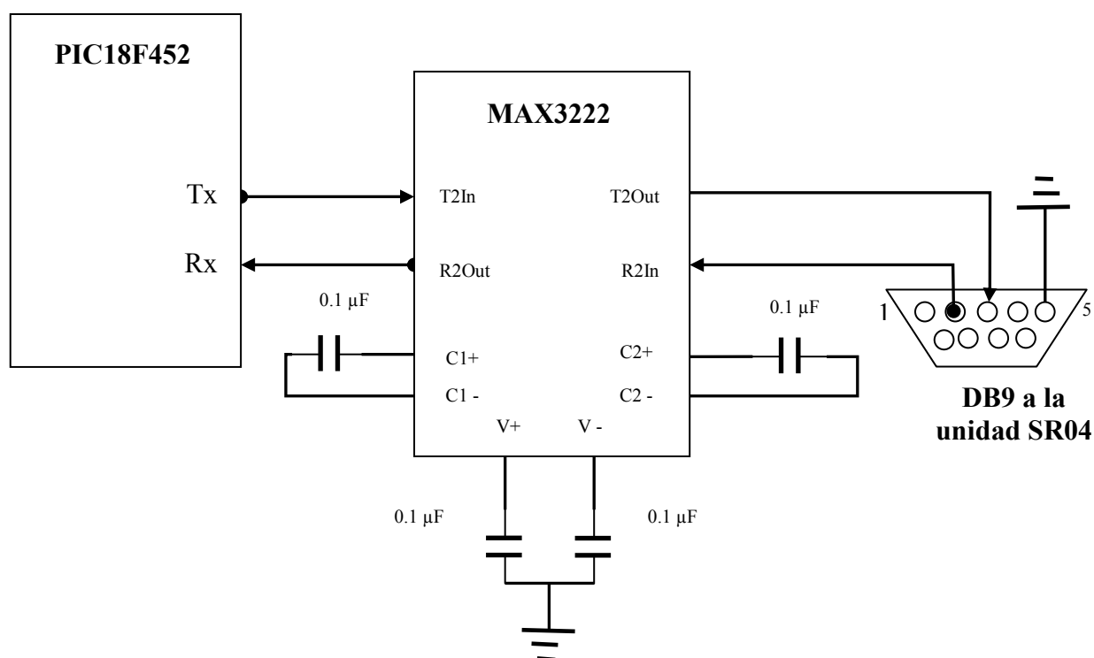
Figura 3.7. Conexión del transceptor con el microcontrolador.
