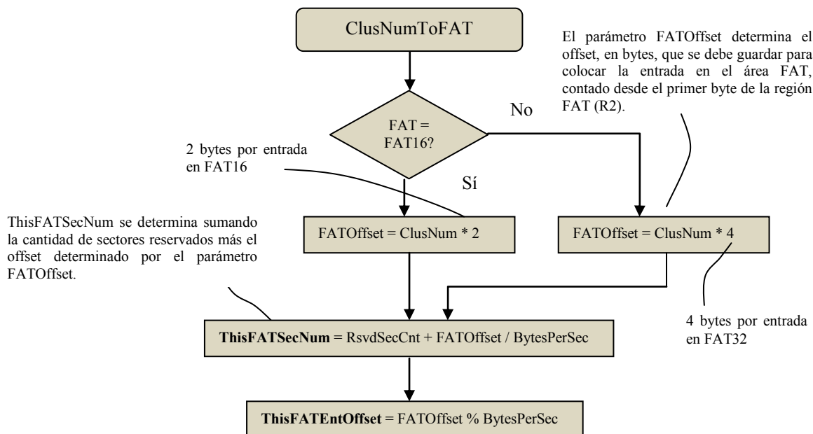
Figura 3.33. Determinación de la posición de la entrada de un clúster en la tabla FAT.
