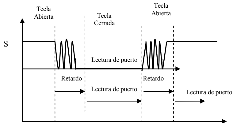
Figura 2.35. Uso de retardos para evitar el efecto de rebote mecánico.
