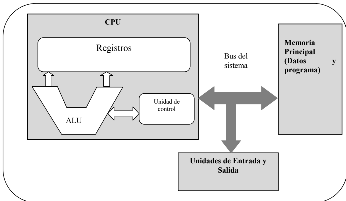
Figura 2.31. Arquitectura Von Newmann.
