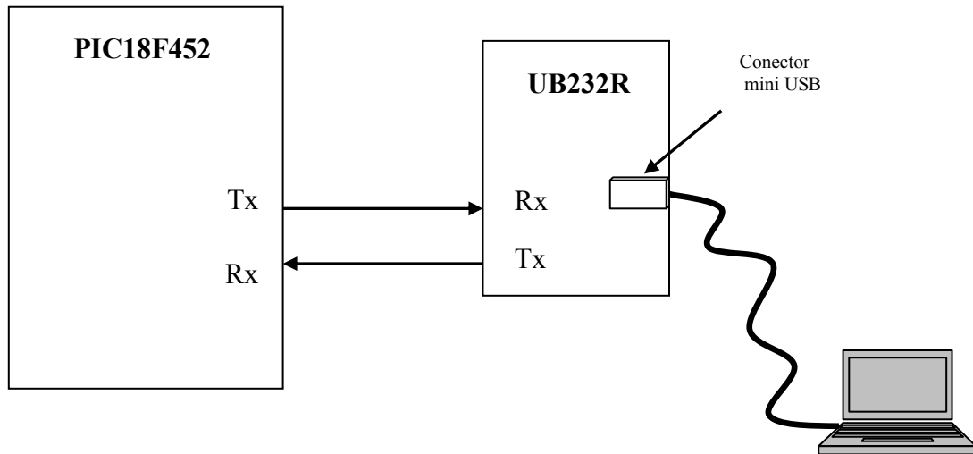
Figura 3.9. Conexión entre el microcontrolador y una PC a través de un adaptador RS -232 a USB.
