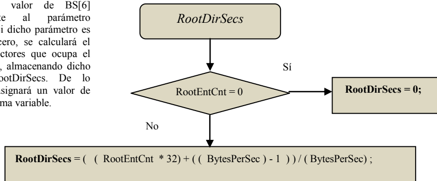
Figura 3.22. Obtención del parámetro RootDirSecs .
