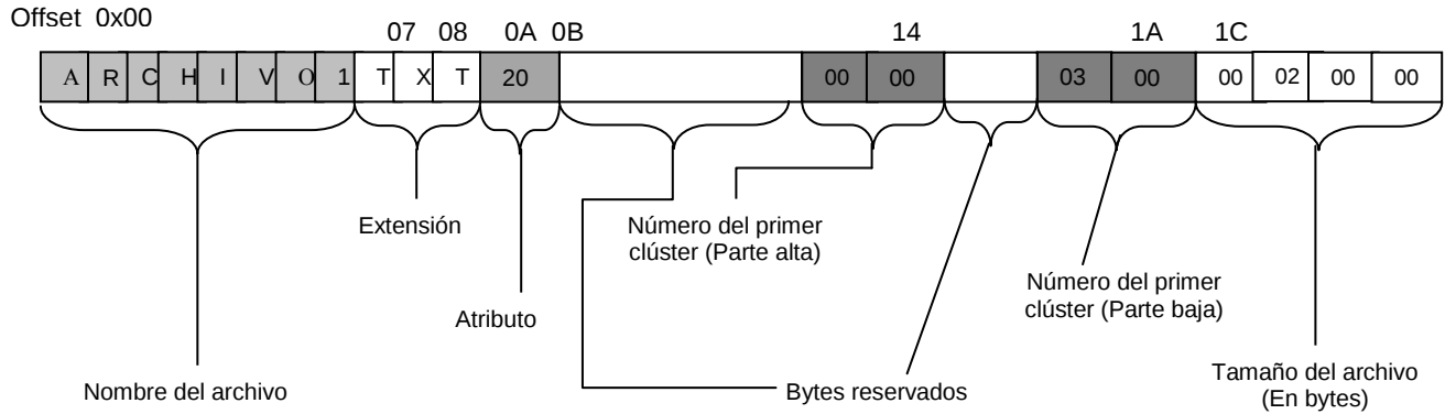
Figura 2.24. Estructura de las entradas en el Directorio Raíz.
