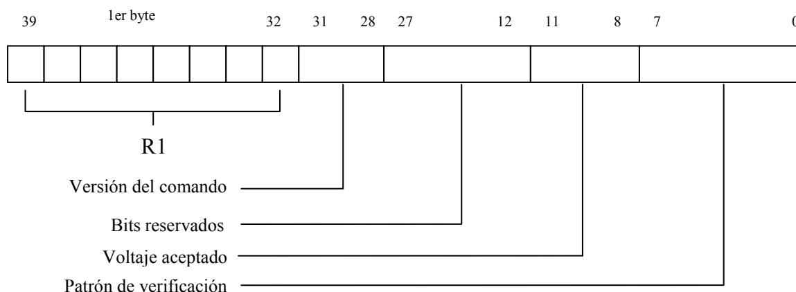
Figura 2.14. Formato de la respuesta R7.
