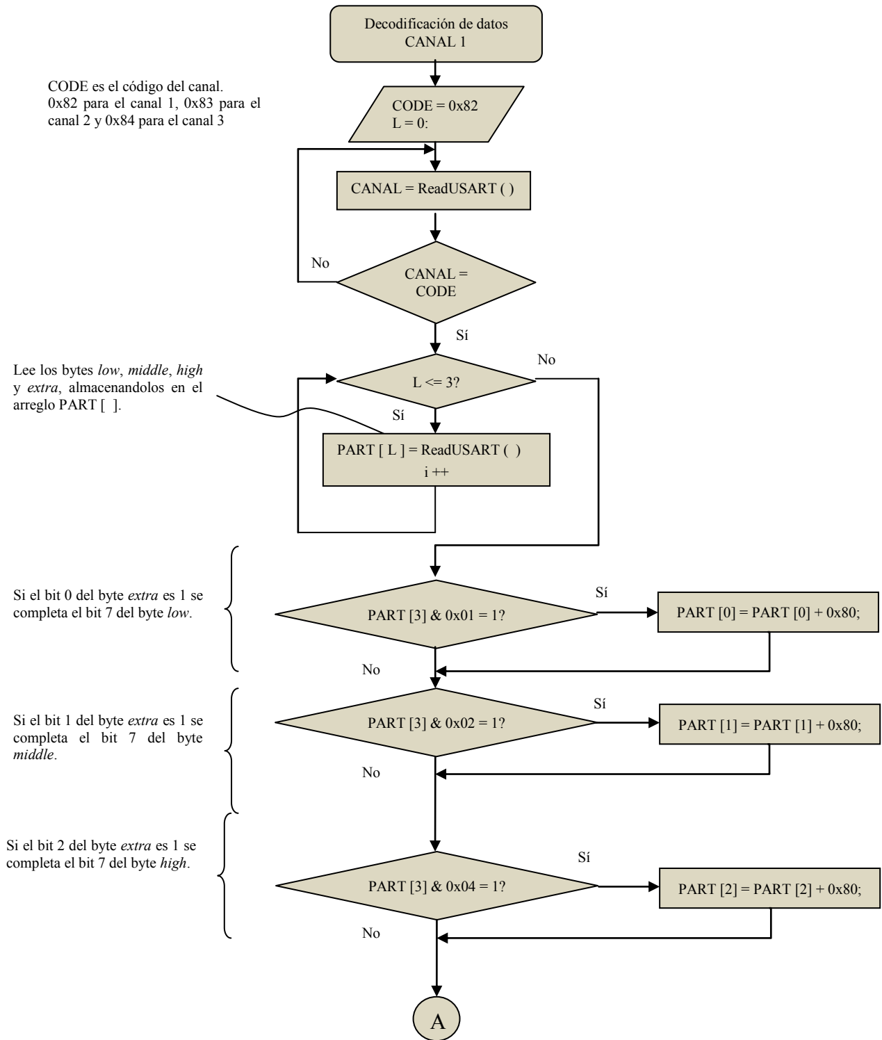
Figura 3.35. Diagrama de flujo para la decodificación de los datos del canal 1 de la unidad SR04 (1 de 2).
