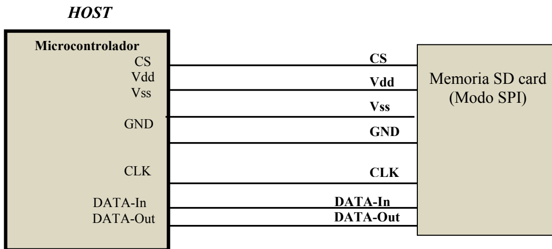
Figura 2.5. Topología del bus SPI.
