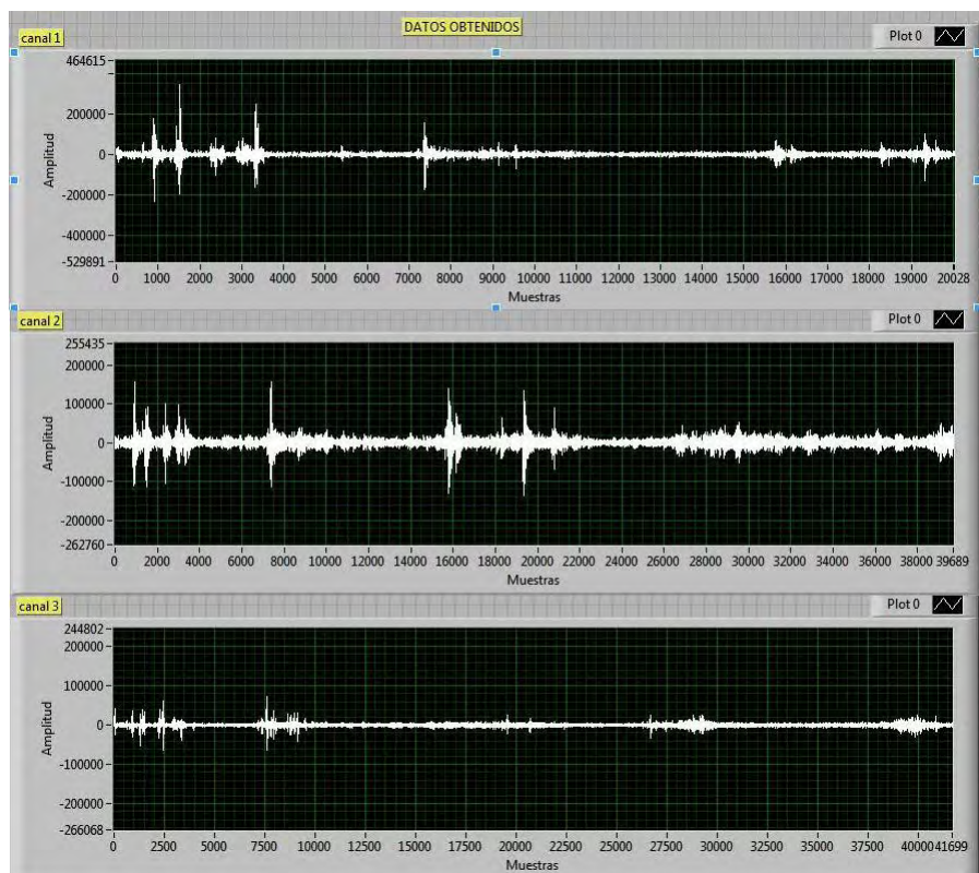
Figura 4.36. Gráficas obtenidas a partir del archivo 13AGO10A.
