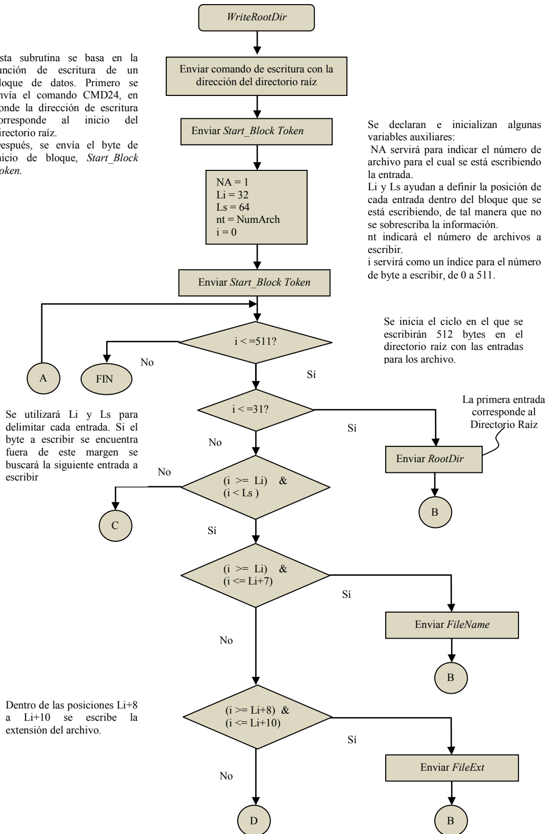
Figura 3.57. Diagrama de la función WriteRootDir (1 de 3).
