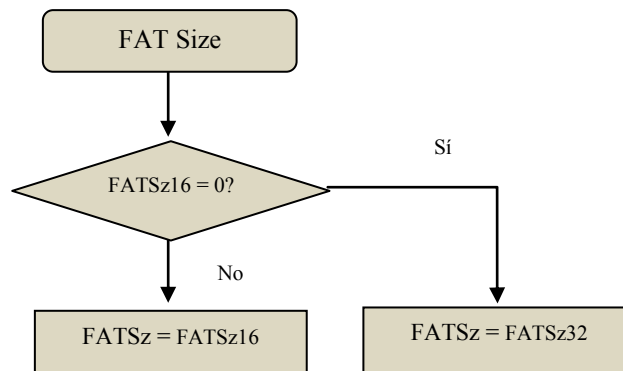
Figura 3.23. Determinación de la cantidad de sectores ocupados por la región FAT.
