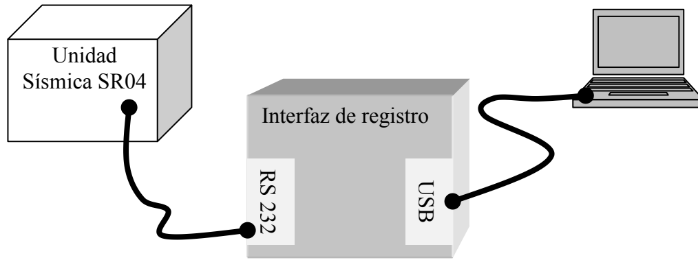
Figura 3.37. Conexión entre la Unidad SR04 la Interfaz de registro y una PC.
