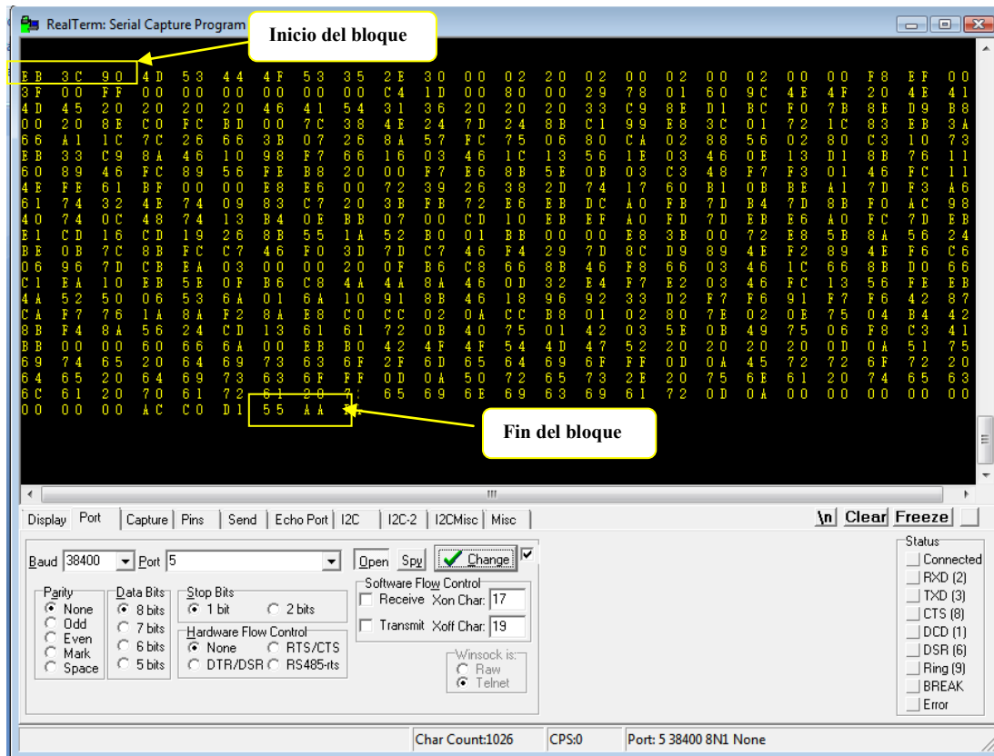
Figura 4.21. Bloque de datos leído de la tarjeta y enviado a la terminal.
