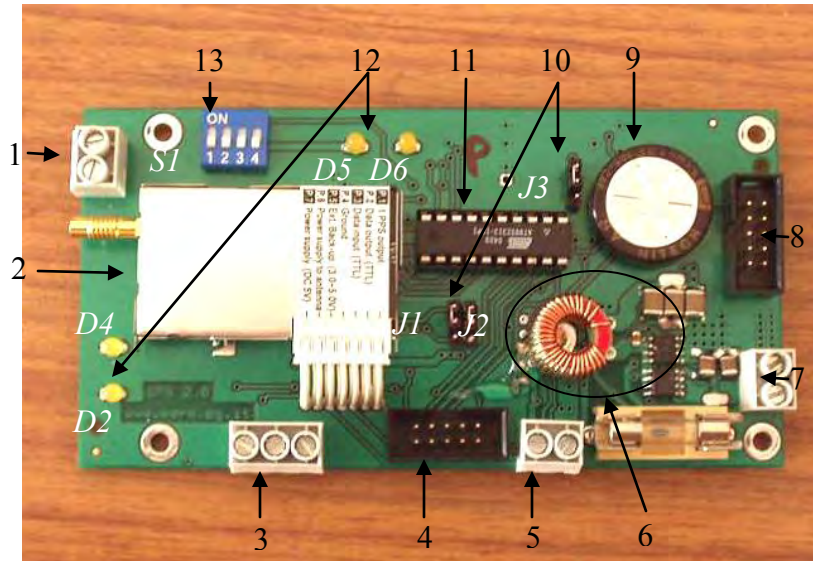
Figura 2.29. Tarjeta GPSDCF.
