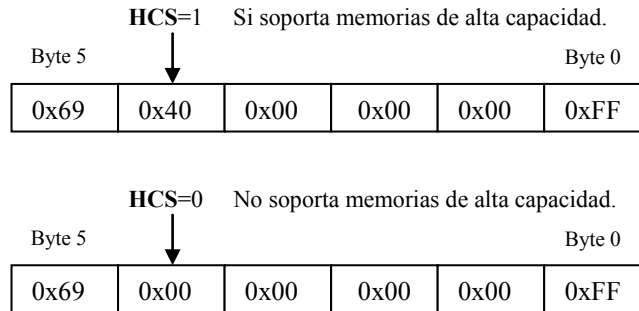
Figura 3.18. Argumentos para el comando ACMD41.
