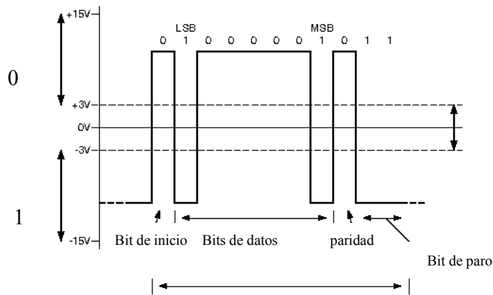
Figura 2.35. Envío del carácter 'A' por RS 232.
