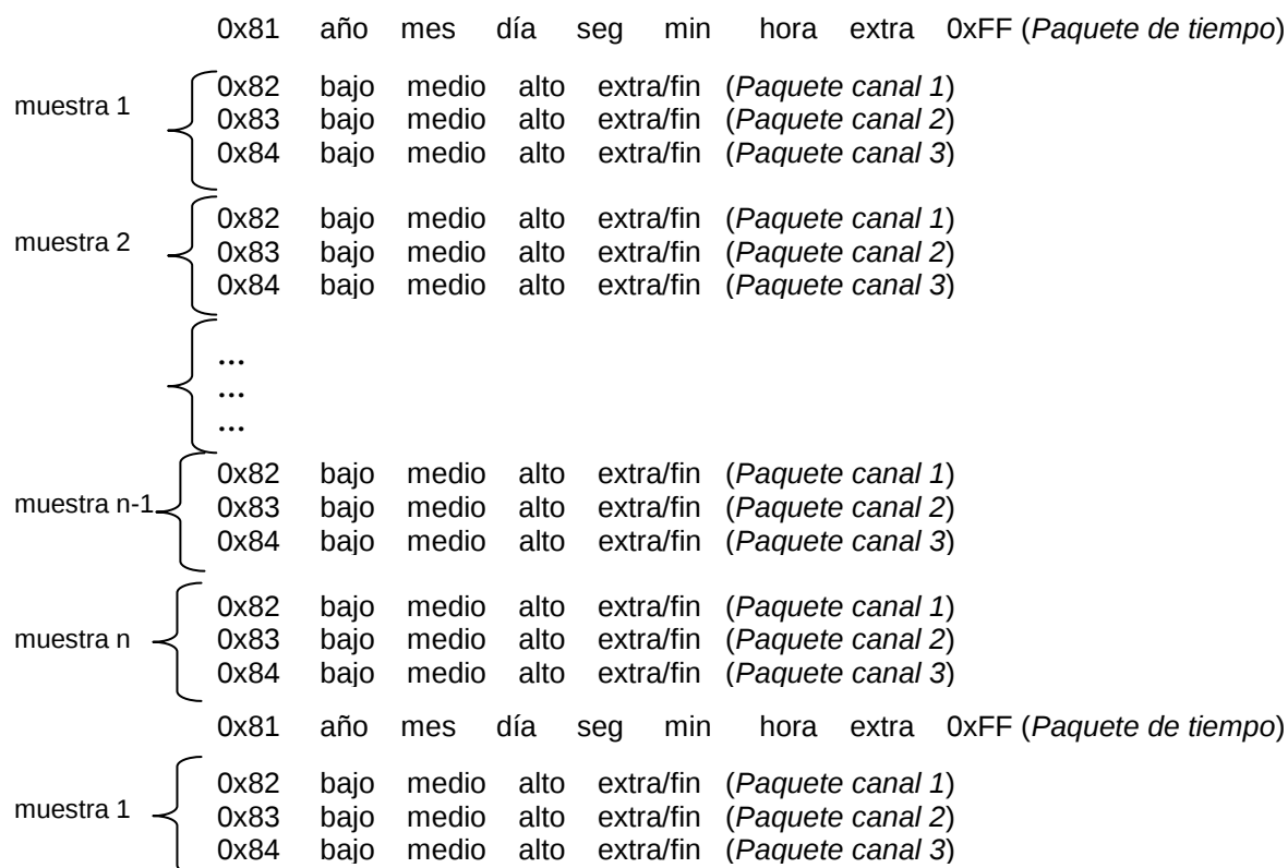
Figura 2.30. Formato de los paquetes de información provenientes de la tarjeta SADC20.
