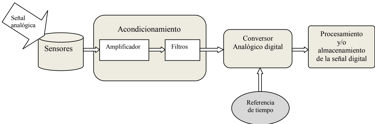
Figura 2.1. Sistema típico de adquisición y registro de datos.
