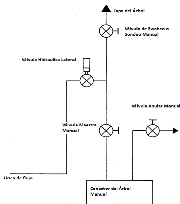
Figura 2.3. Árbol Submarino Sencillo
