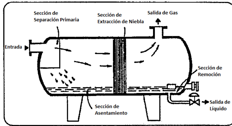
Figura 4.1. Diseño Básico de un Separador
