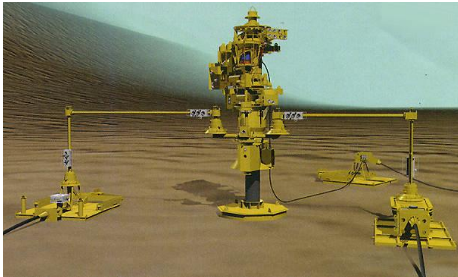
Figura 2.2. Árbol Submarino.
