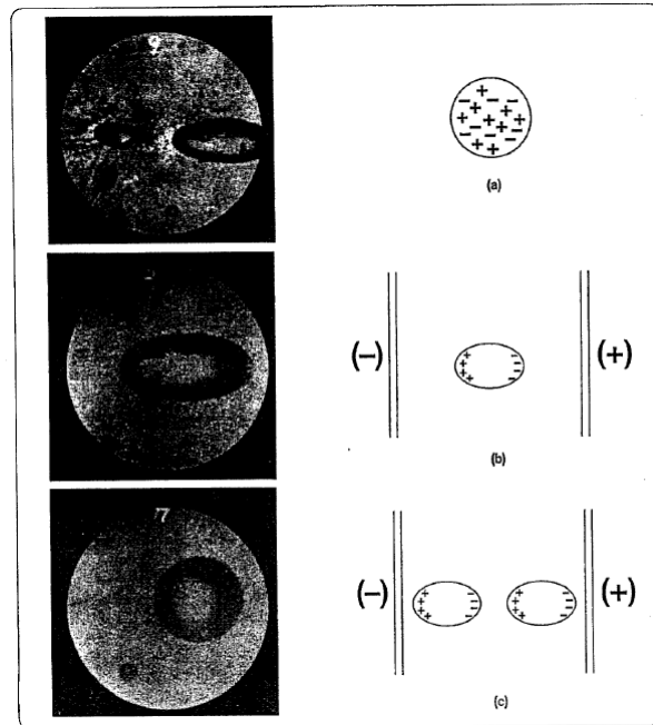
Figura 5.7. Gota de Agua en un Campo Eléctrico
