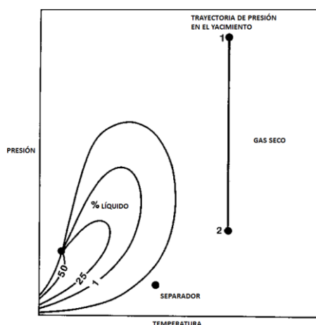
Figura 3.7. Envolverte de Fases del Gas Seco
