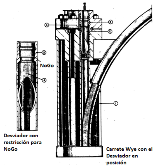
Figura 2.10. Carrete Wye y Desviadores
