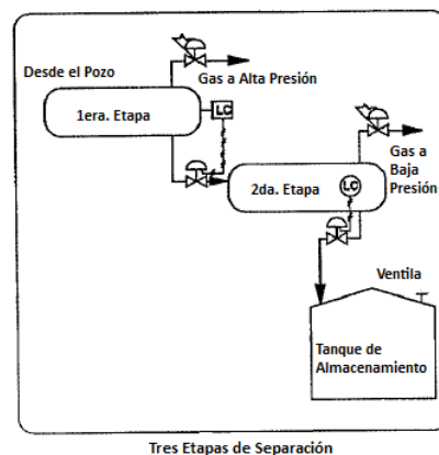
Figura 4.15. Tanque de Almacenamiento, 3era. Etapa de Separación
