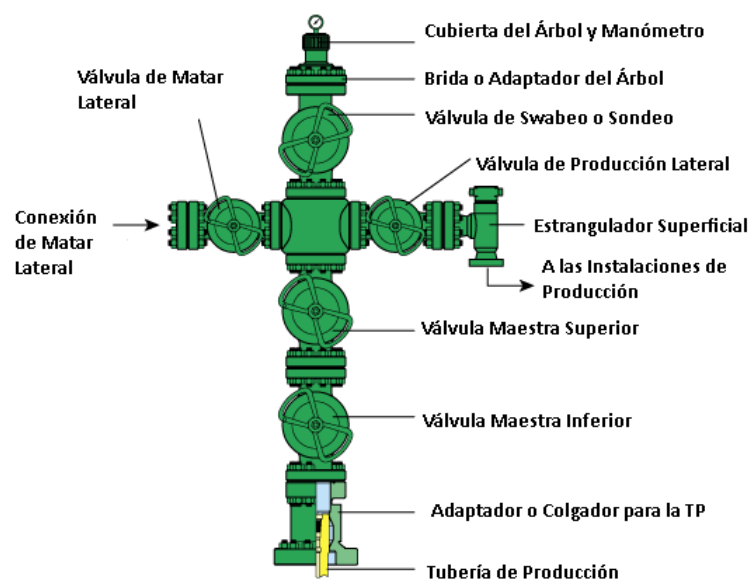
Figura 2.1 Árbol de Válvulas Convencional
