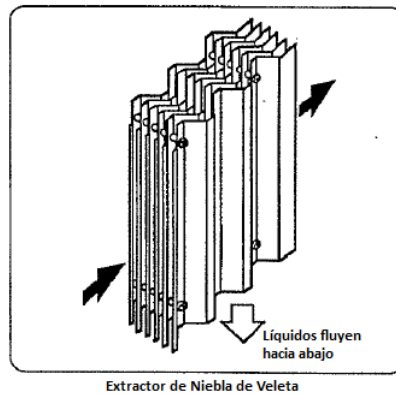
Figura 4.8. Extractor de Niebla de Veleta
