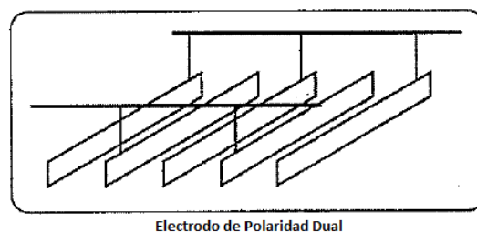
Figura 5.15. Electrodo de Polaridad Dual
