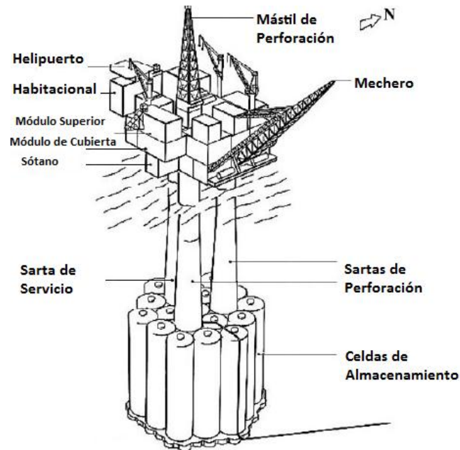
Figura 1.4. Plataforma de Gravedad
