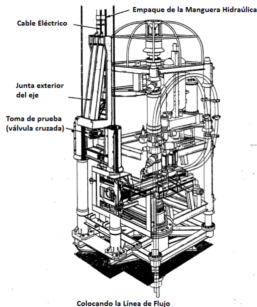
Figura 2.14. Árbol sin asistencia de buzos
