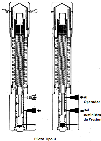
Figura 2.12. Piloto tipo U
