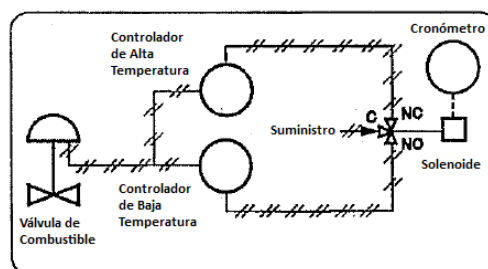
Figura 6.3. Calentamiento Automático
