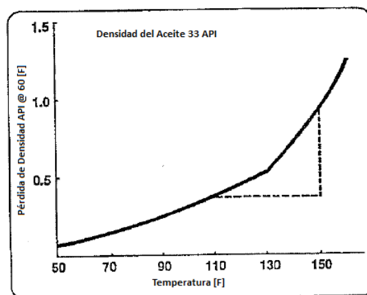
Pérdida de Densidad API vs. Temperatura
