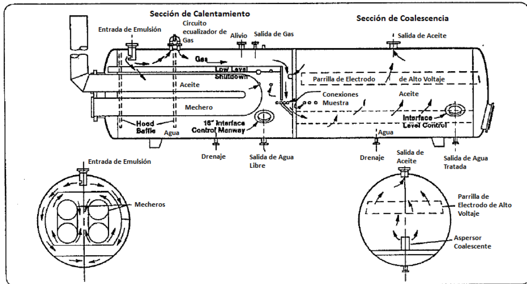
Figura 5.22. Tratador Horizontal Mecánico
