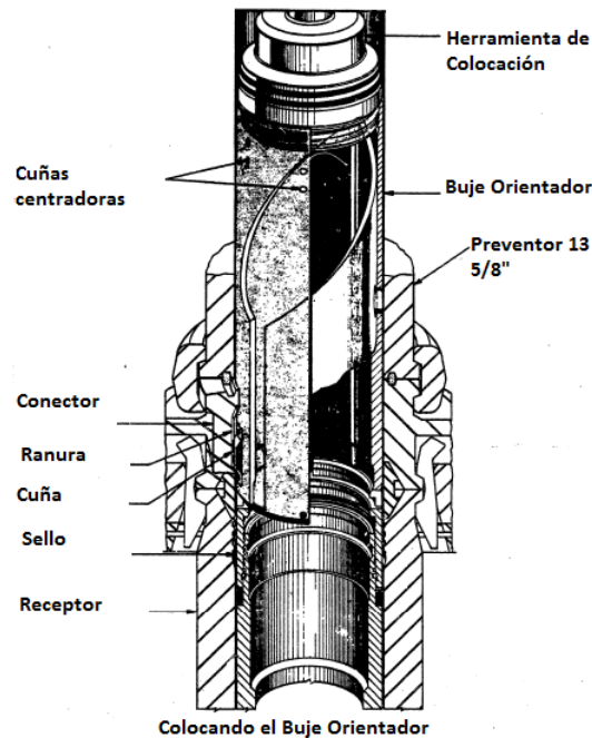
Figura 2.4. Buje Orientador
