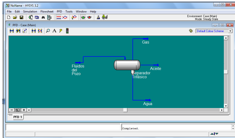
Figura 9.11. Separador Trifásico
