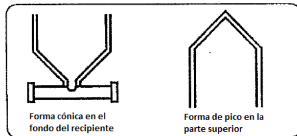
Figura 6.9. Diseños de Recipientes que manejan Arena
