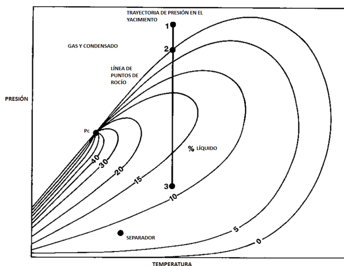
Figura 3.5. Envoltente de Fases de Gas y Condensado
