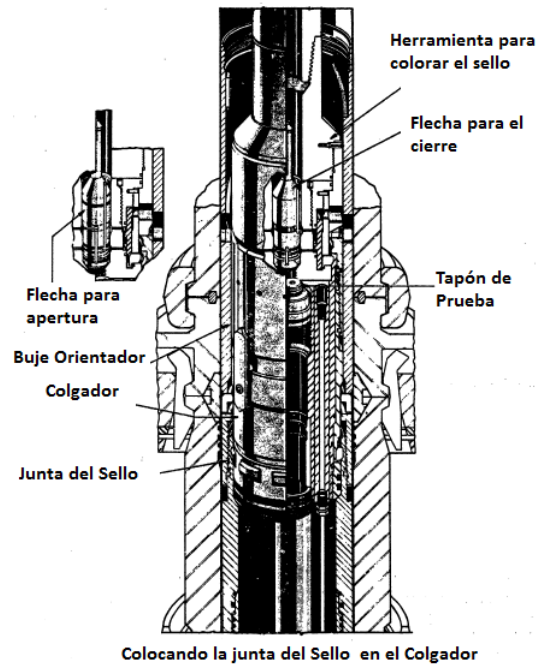
Figura 2.5. Colgador
