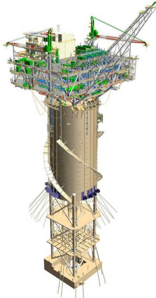
Figura 1.8. Plataforma Spar
