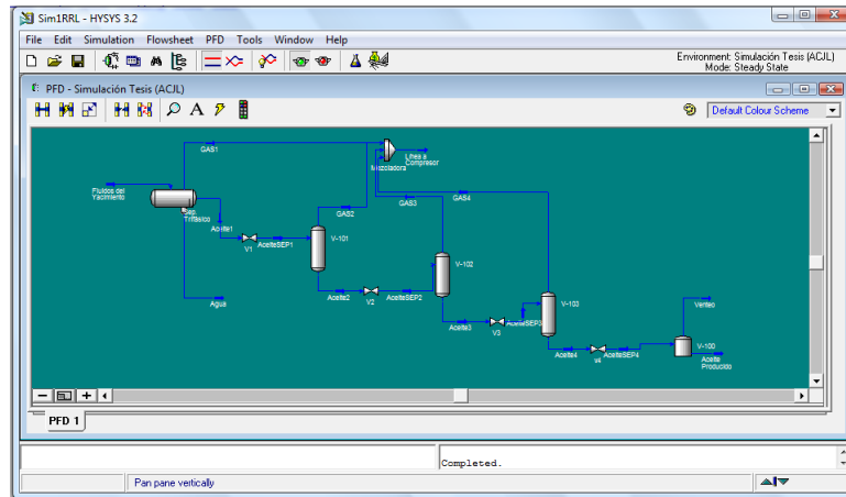
Figura 9.9. Tren de Separación de 5 Etapas
