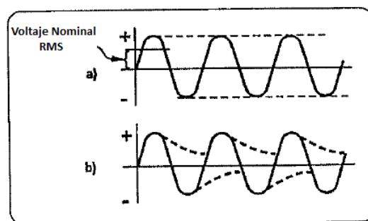
Figura 5.17. Voltaje Nominal RMS
