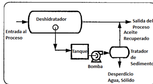
Figura 6.8. Sistema de Tratamiento por Separado
