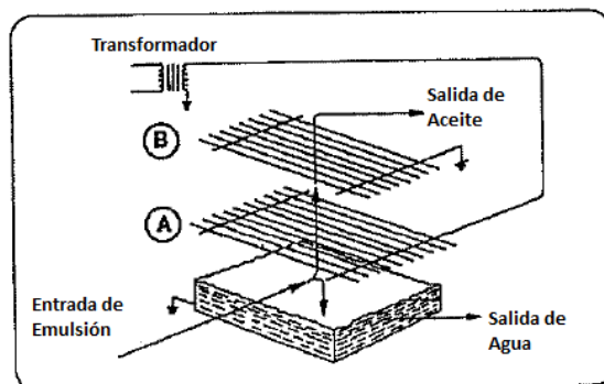
Figura 5.8. Sistema Electrostático Convencional
