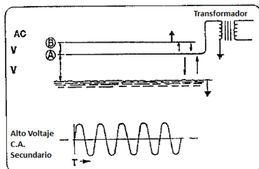
Figura 5.11. Proceso de Campo Alterno
