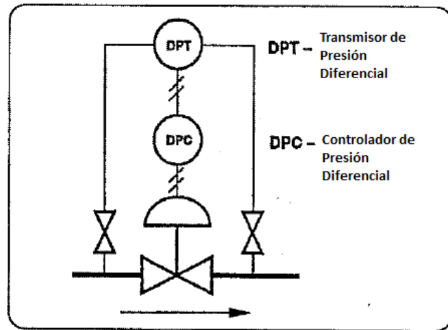
Figura 7.12. Válvula con circuito de Presión Diferencial
