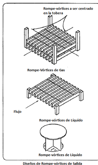
Figura 4.10. Diseños de Rompe-vórtices de Salida
