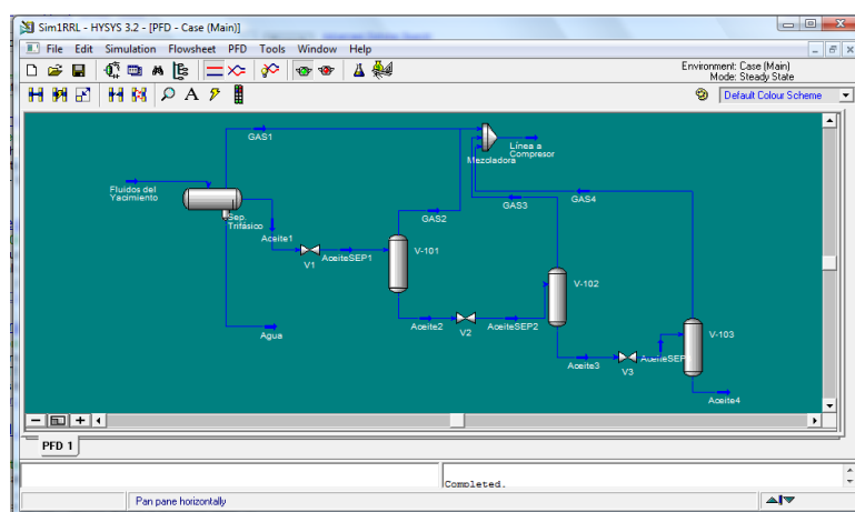
Figura 9.6. Tren de Separación de 4 Etapas.
