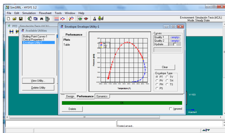
Figura 9.8. Envoltente de Fases del Aceite
