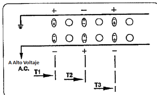
Figura 5.10. Efecto del Campo sobre la Emulsión
