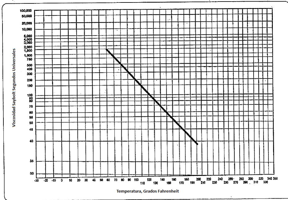
TÍPICO ACEITE DE DENSIDAD INTERMEDIA Gráfica Viscosidad-Temperatura Estándar ASTM para productos de petróleo líquidos
