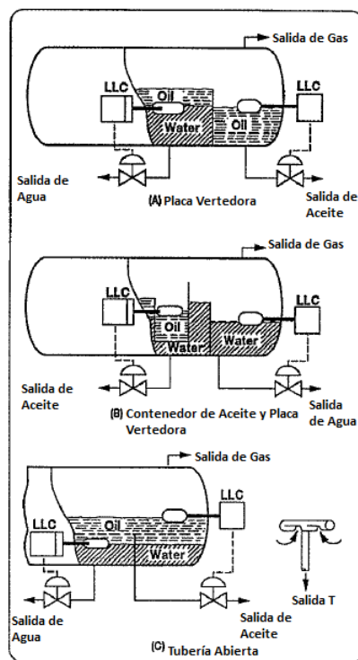
Figura 4.11. Controles de Salida
