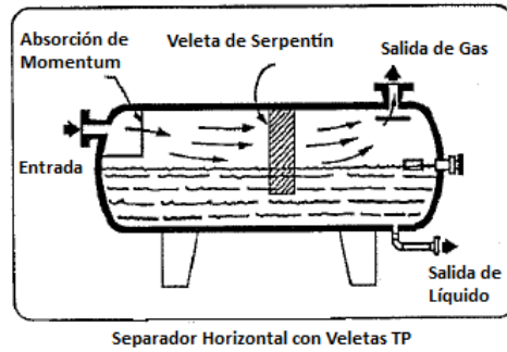
Figura 4.14. Separador Horizontal con Veletas TP
