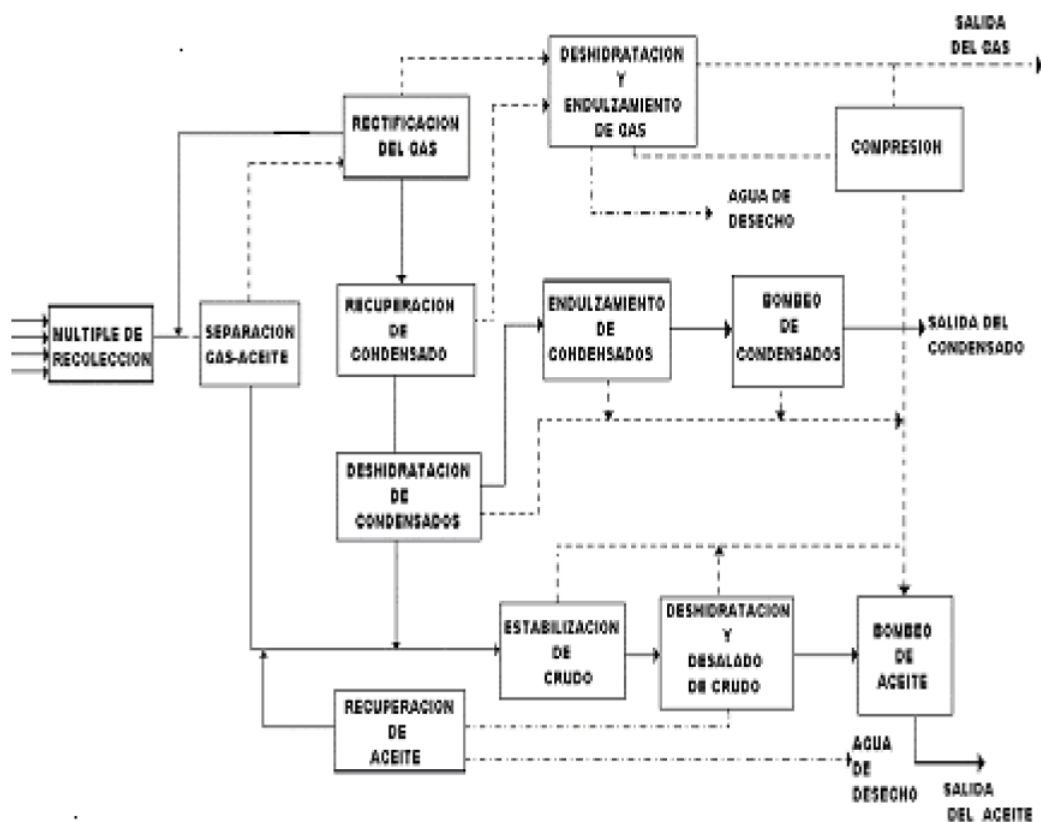
Figura 3.8. Sistema de Producción para Aceite Volátil
