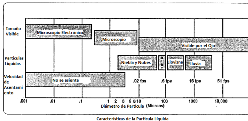
Figura 4.3. Características de la Partícula Líquida
