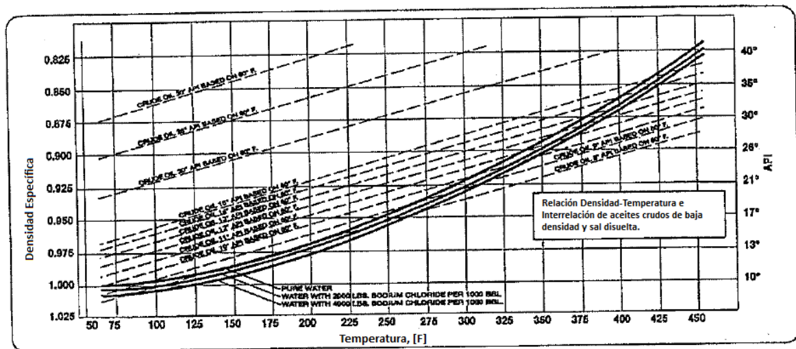
Figura 5.3. Gráfica Densidad-Temperatura
