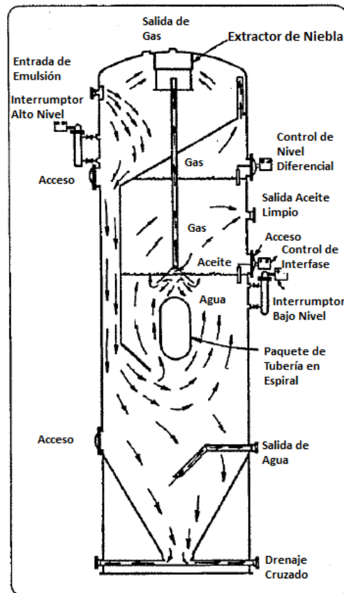
Figura 6.11. Tratador Vertical
