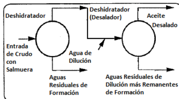
Figura 7.4. Deshidratación de Dos Etapas
