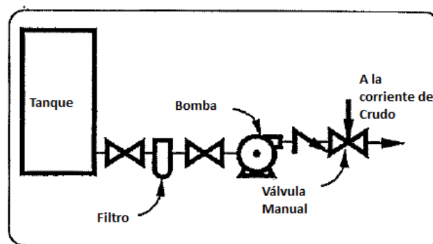
Figura 7.14. Sistema de Inyección de Agua de Dilución
