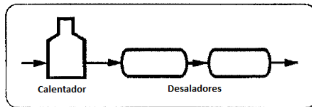
Figura 7.17. Unidad de Calentamiento Independiente
