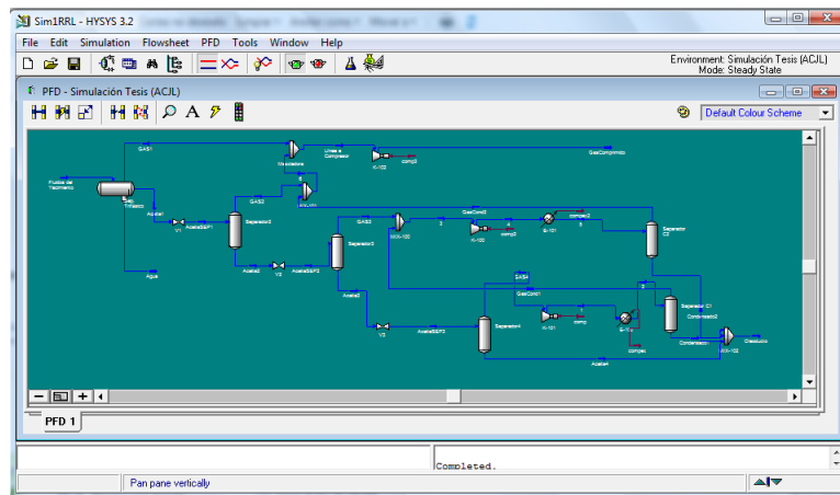
Figura 9.10. Tren de Separación con Scrubbers
