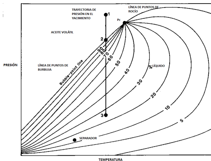
Figura 3.4. Envoltente de Fases del Aceite Volátil
