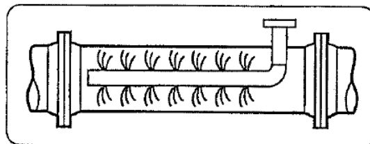
Figura 7.13. Inyector de Mezclado
