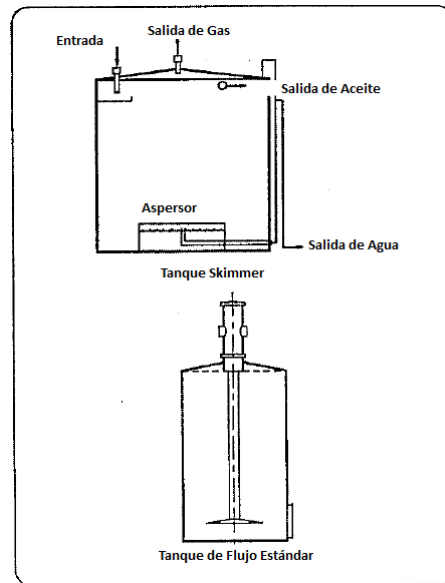
Figura 5.20. Tanques de Almacenamiento
