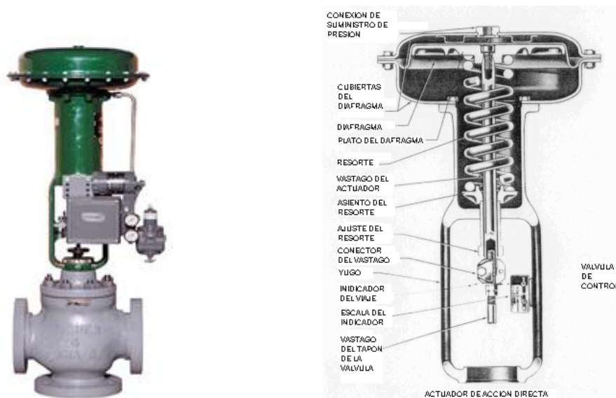
Figura 8.10. Válvula Reguladora de Flujo.
