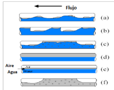
Figura 8.2. Patrones de Flujo
