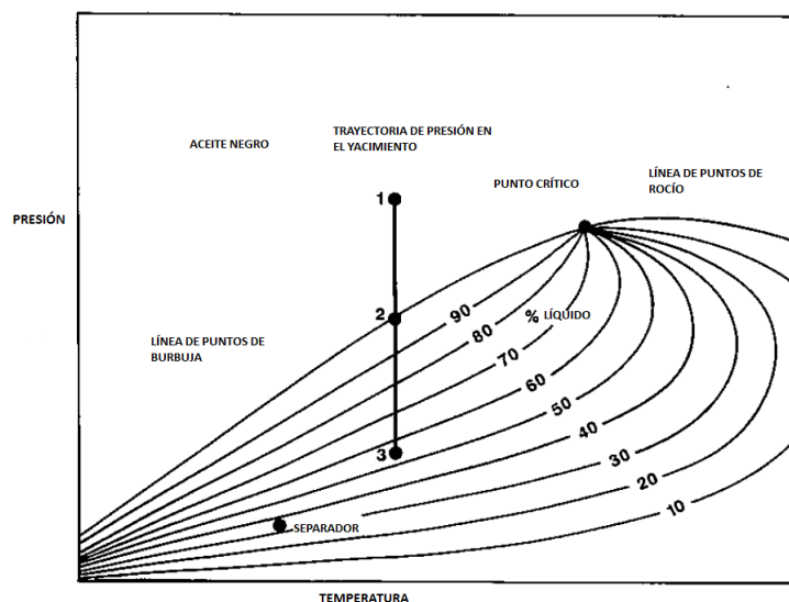
Figura 3.3. Envolvente de Fases del Aceite Negro
