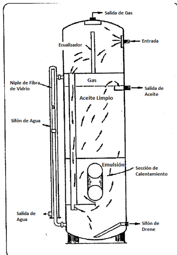
Figura 5.21. Tratador Vertical
