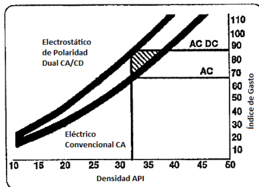
Figura 5.18. Rendimiento de Gastos para Sistemas de AC y AC/DC
