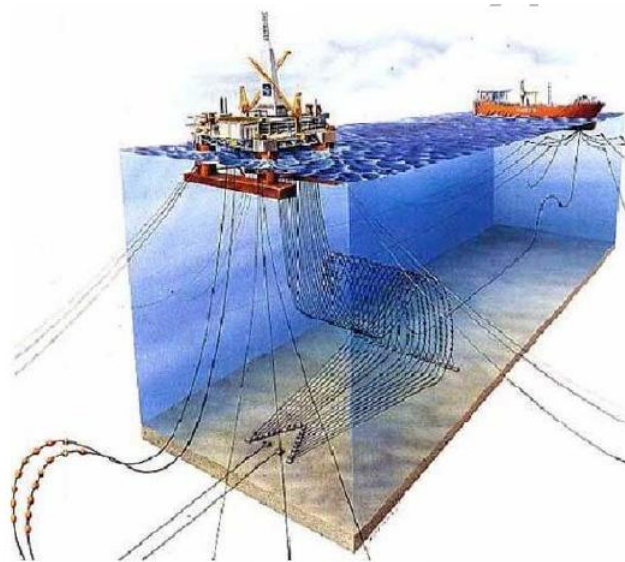
Figura 1.5. Plataforma Semisumergible
