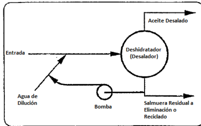
Figura 7.8. Reciclaje Interno
