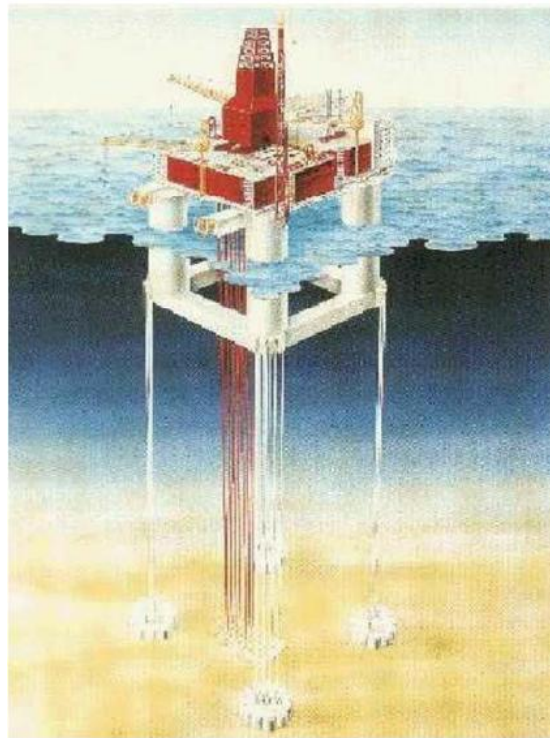
Figura 1.7. Plataforma de Piernas Tensionadas (TLP)
