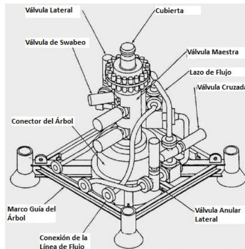
Figura 1.1. Árbol Submarino
