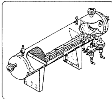
Extractor de Niebla de Placas Paralelas Dixon
