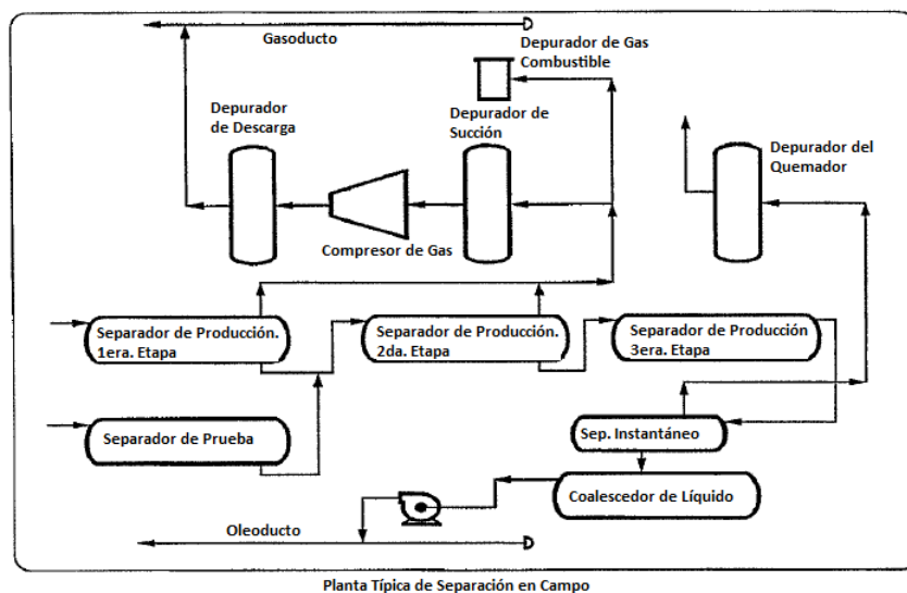
Figura 4.12. Esquema de Separación en Campo
