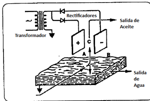
Unidad de Deshidratación Electrostática de Polaridad Dual
