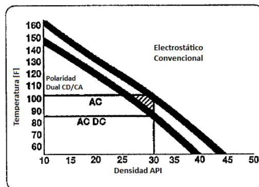
Figura 5.19. Comparación de los Sistemas de AC y AC/DC vs. Temperatura
