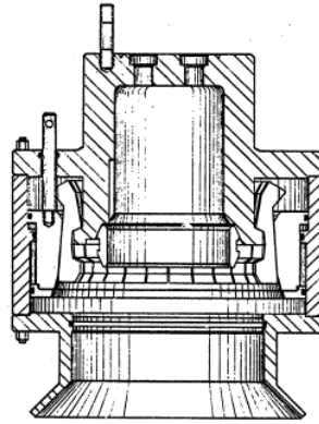
Conector Hidráulico del Árbol
