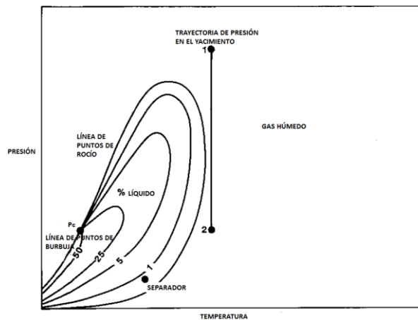
Figura 3.6. Envolverte de Fases del Gas Húmedo
