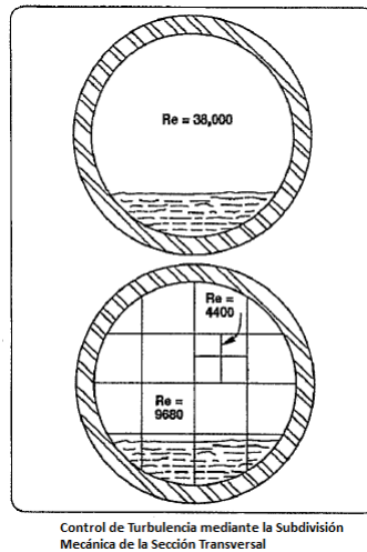
Figura 4.4. Subdivisión Mecánica de la Sección Transversal
