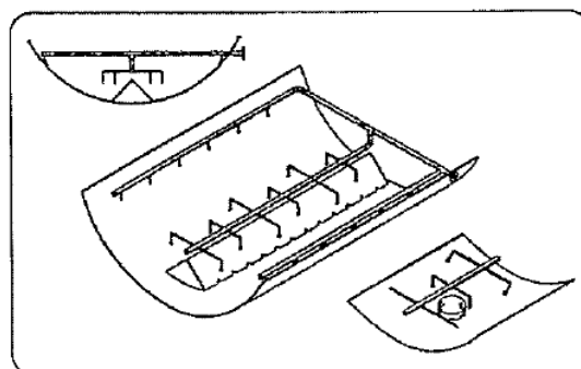
Figura 6.10. Jets y Desagües de para Arena
