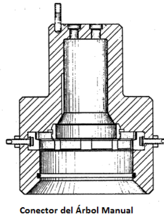
Figura 2.6. Conector Manual del Árbol
