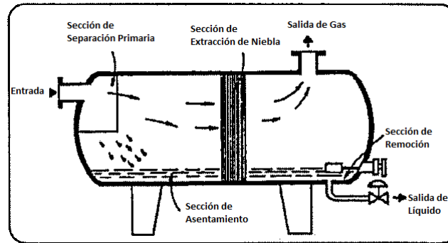
Figura 1.9. Secciones del Separador
