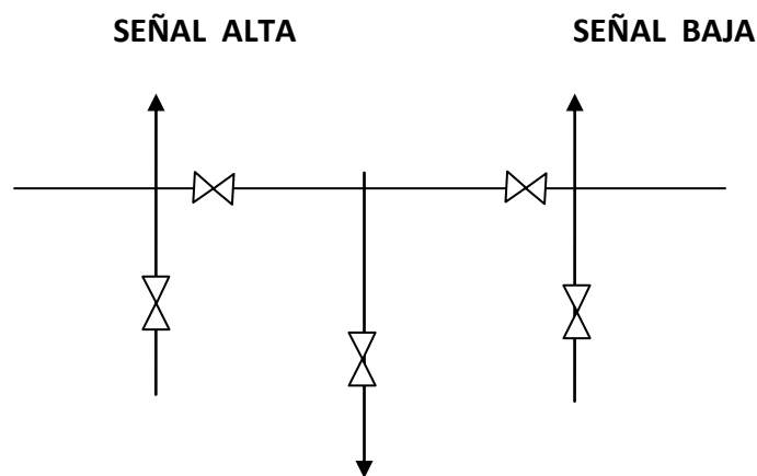
Figura 8.5. Diagrama del Manifold
