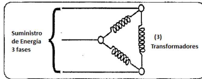
Figura 7.11. Conexión en configuración delta a los Transformadores
