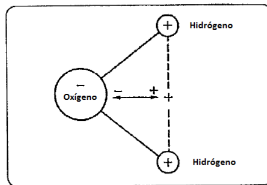
Figura 5.6. Átomo de Agua
