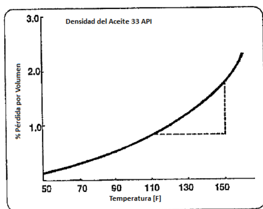
Pérdida por Volumen vs. Temperatura
