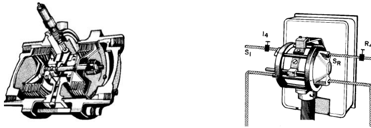
Figura 8.6. Celda diferencial del Registrador de Flujo.
