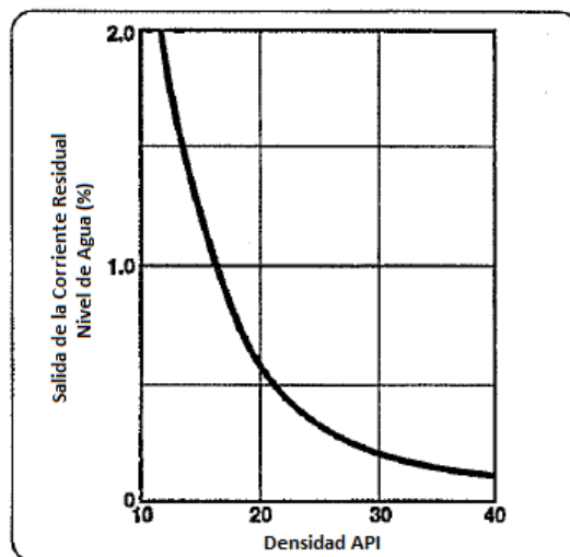
Figura 7.2. Nivel de Remoción % vs. Densidad API
