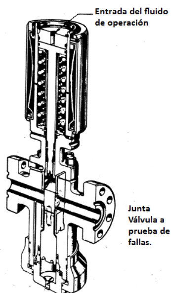
Figura 2.7. Válvula Lateral
