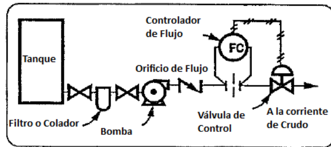
Figura 7.15. Sistema con Sensor y Controlador de Flujo
