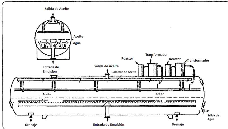
Figura 7.10. Desalador de Alta Capacidad
