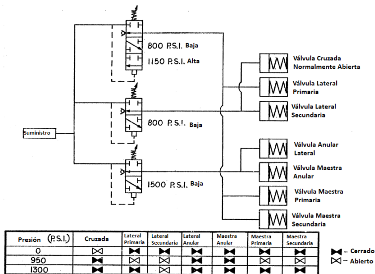
Figura 2.13. Arreglo de válvulas con pilotos
