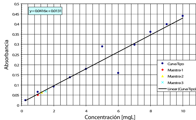
Figura 4.8. Concentración vs absorbancia de la curva tipo, con línea de tendencia y ecuación de la recta. Adicionalmente se muestran los valores de absorbancia de las tres muestras analizadas.
