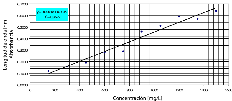
Figura 4.9. Curva tipo para el diesel.
