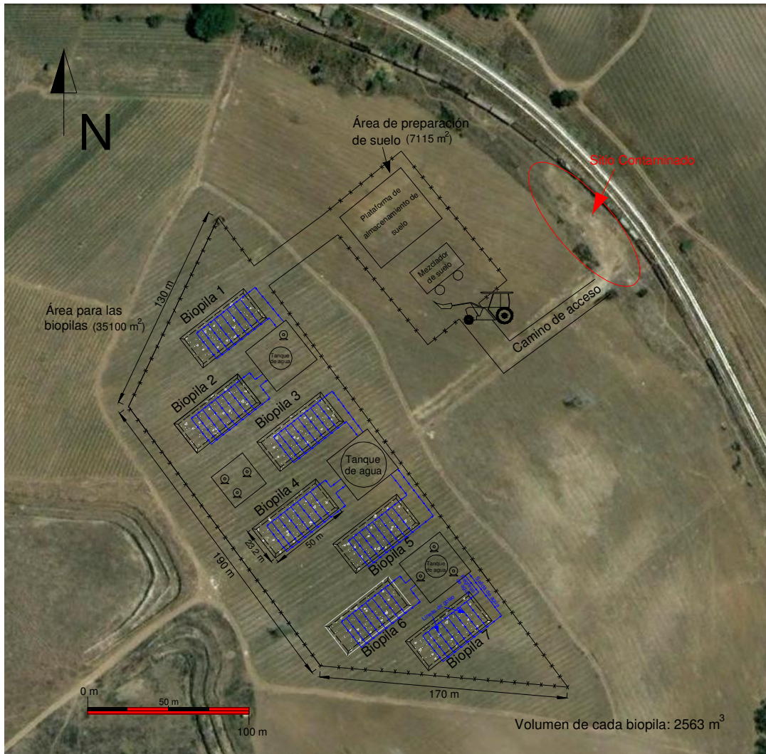
Figura 5.38. Sistema de adición de agua. Las líneas en azul indican las líneas de conducción de agua que ayudarán a la irrigación de las biopilas.
