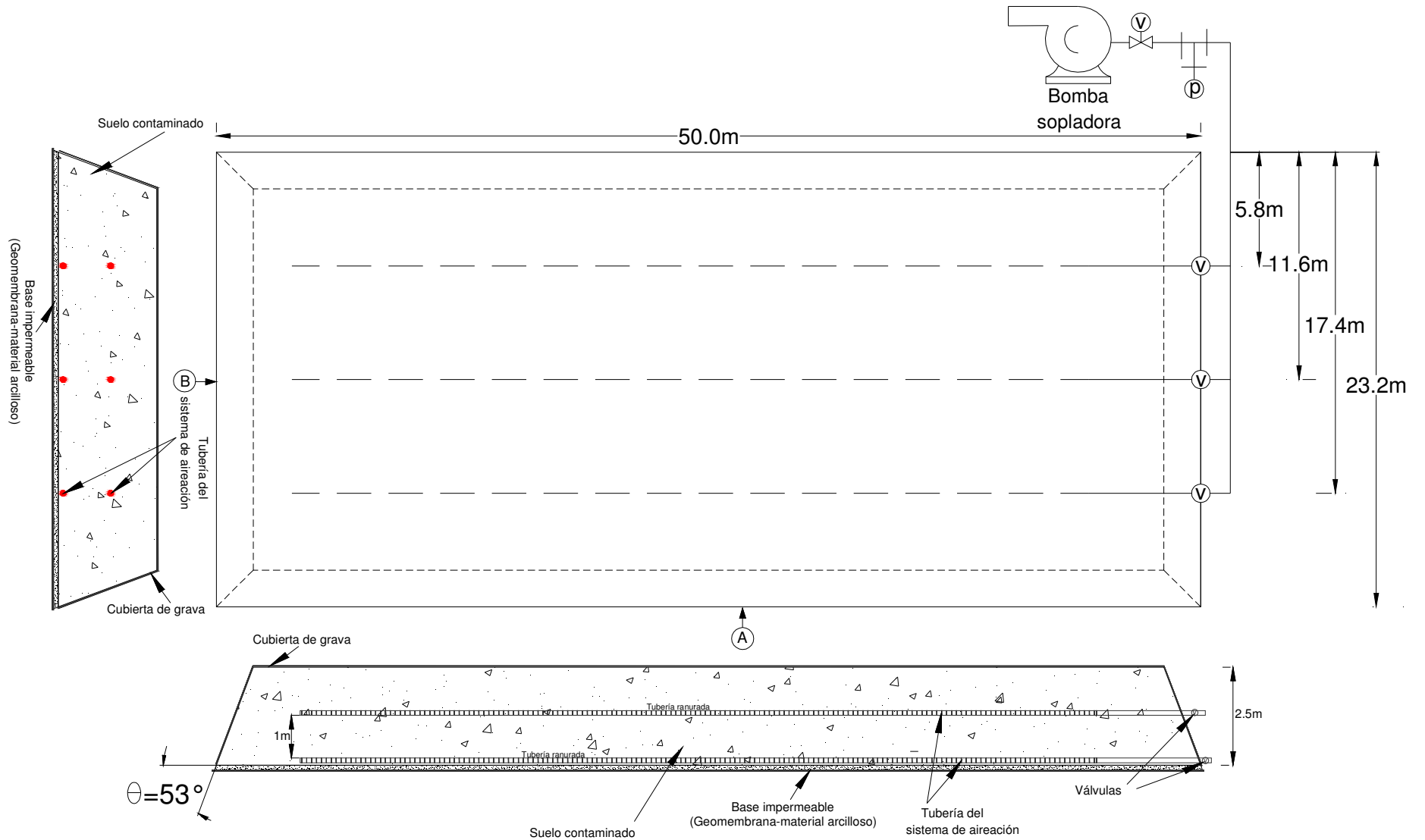
Figura 5.37. Diseño del sistema de aireación. Imagen Central: vista en planta de la biopila; A: vista lateral del sistema; B: vista frontal del sistema de aireación.
