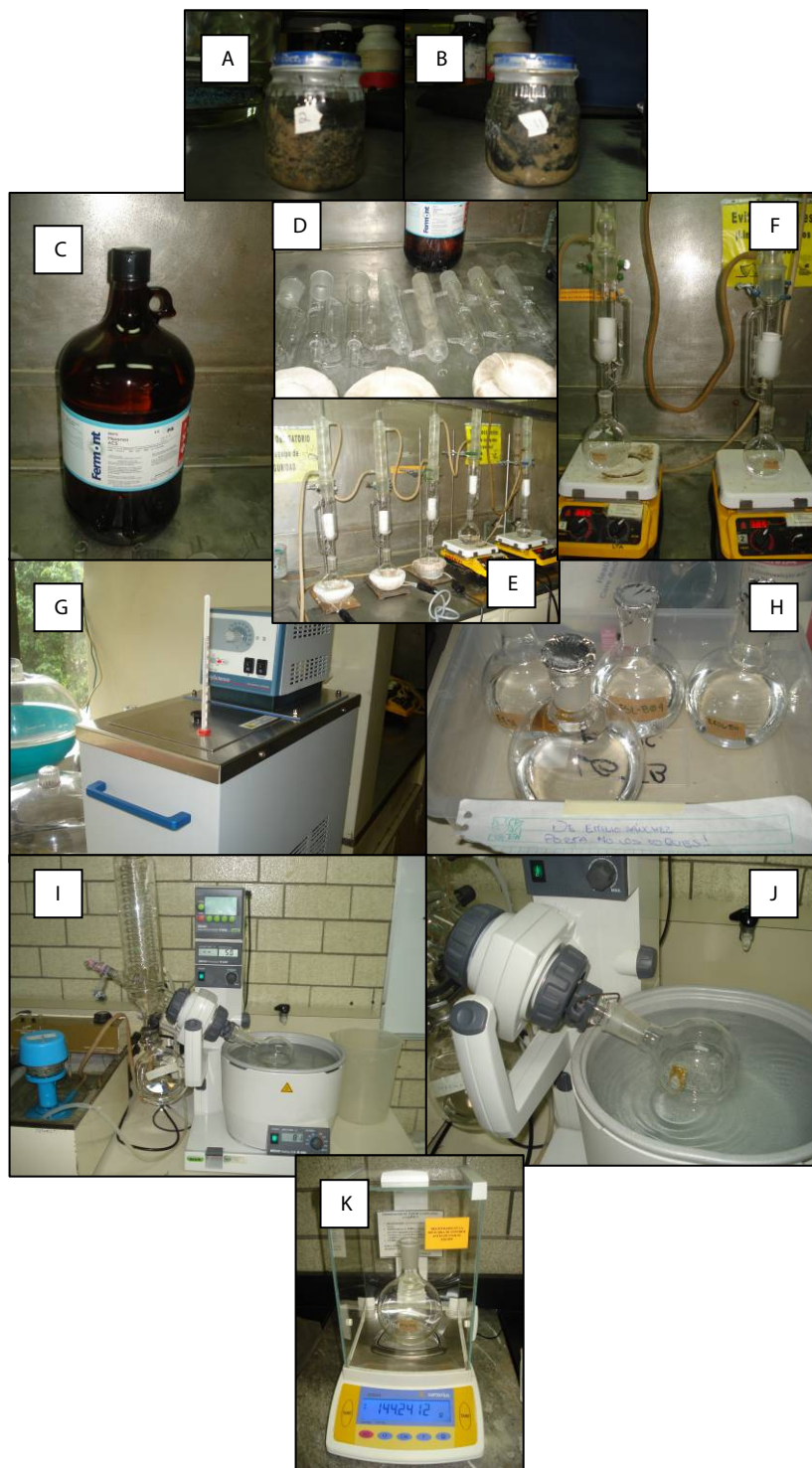
Figura 4.26. Técnica de extracción de TPH aplicado a muestras de biodegradación. A y B muestran el aspecto de dos microcosmos después de la biodegradación; C: solvente usado para realizar la extracción del contaminante (hexano); D-F: equipo soxhlet instalado y funcionando; G: sistema de refrigeración; H: matraces con el extracto producto del suelo, una mezcla de hexano y contaminante; I, J: rotoevaporador que permite la separación del hexano y el contaminante; K: matraz libre de hexano y con el contaminante extraído.
