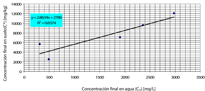
Figura 4.10. Gráfica C_w vs C^* con la que se determinó el valor de k_d .
