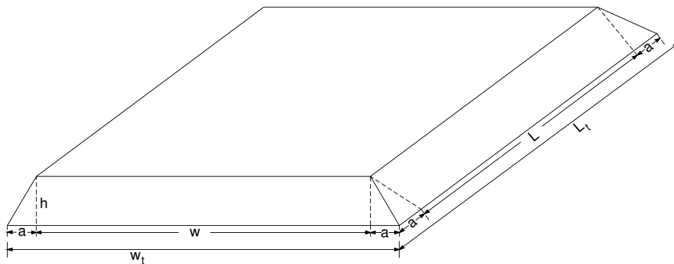
Figura 5.33. Diagrama esquemático de una biopila. W : ancho total (W+2a); W: ancho de la pila; L: largo total (L+2a); L: largo de la biopila; h: altura; a: largo adicional tomando en cuenta la pendiente de las paredes.
