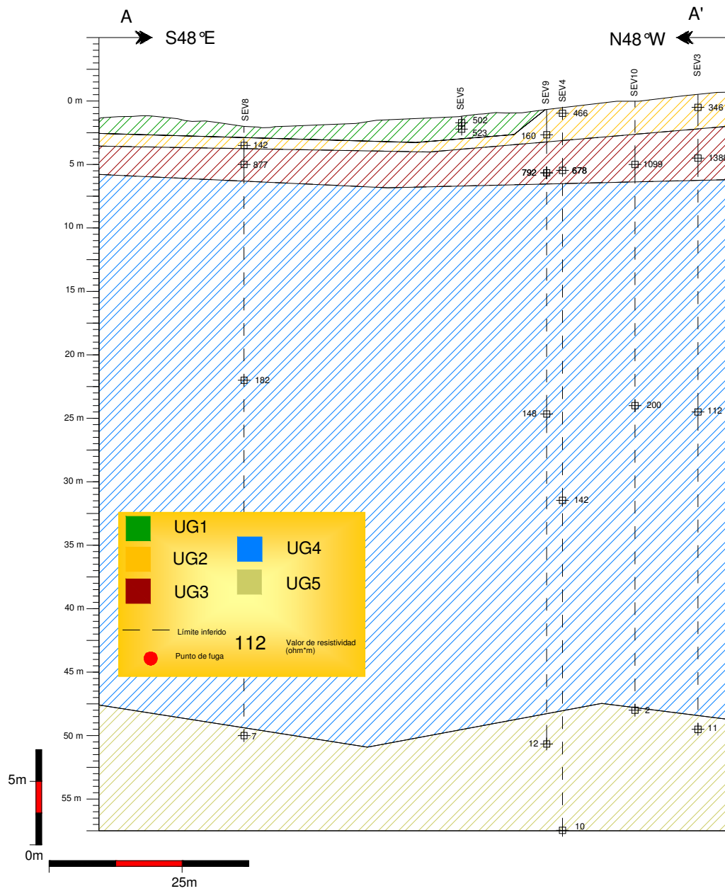
Figura 5.5. Sección geoelectrica AA'.
