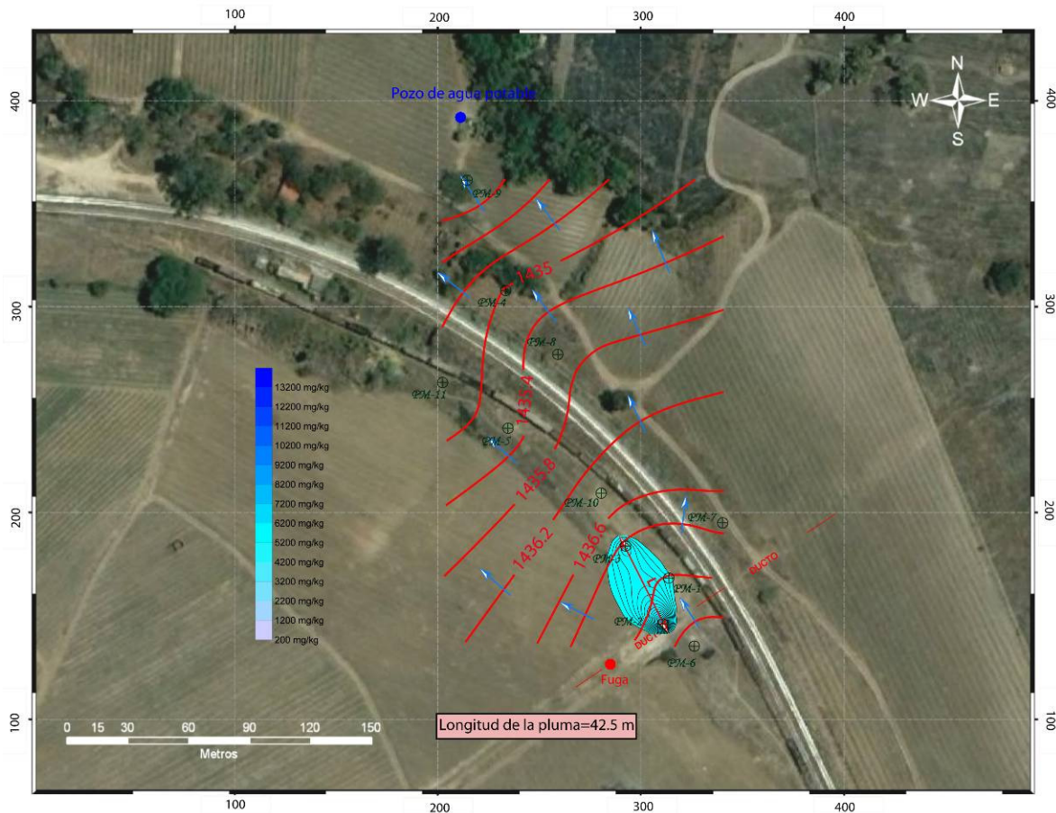
Figura 5.29. Pluma en fase disuelta de naftaleno. Adicionalmente se muestra la dirección de flujo del agua subterránea y las líneas equipotenciales.
