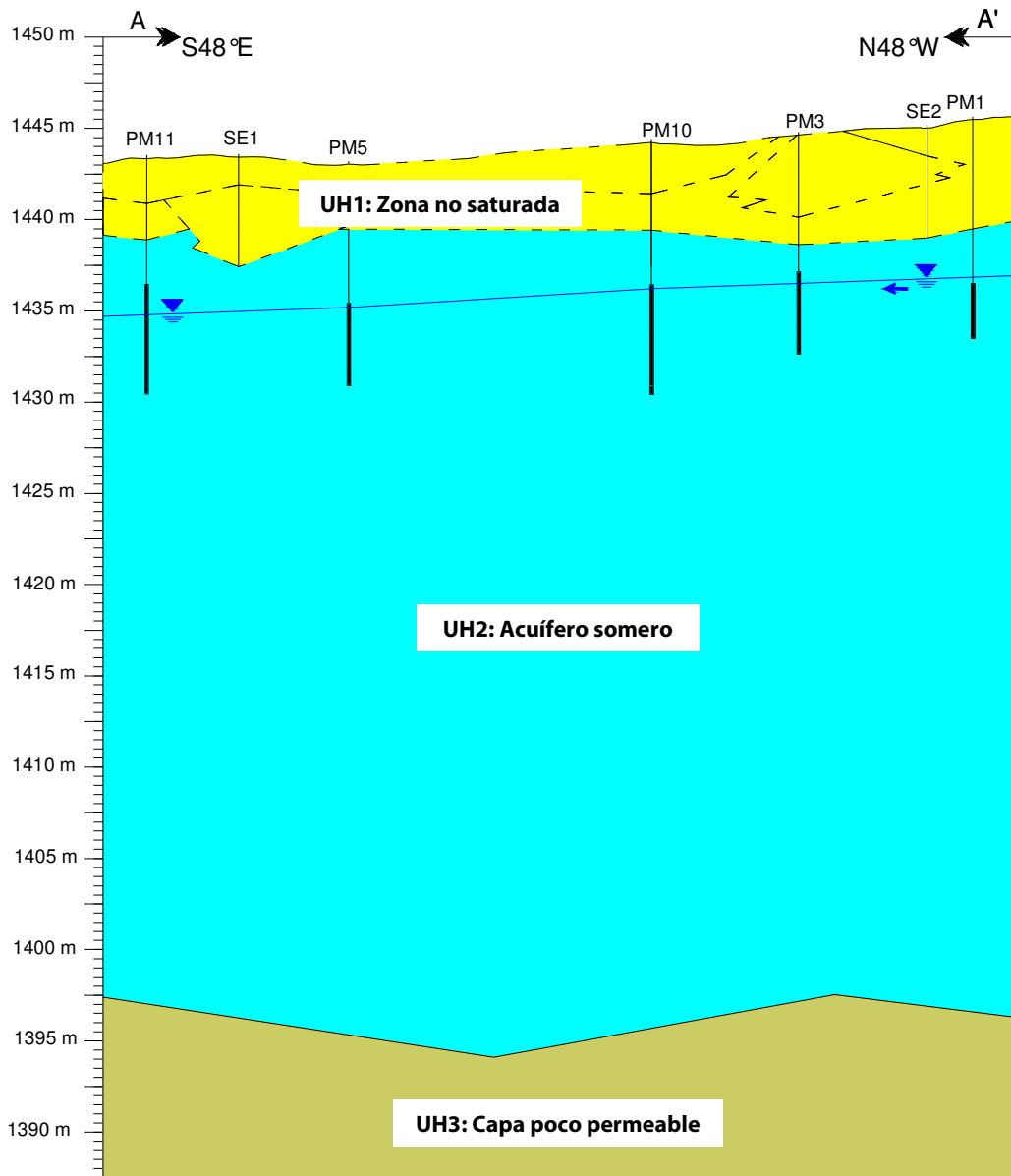
Figura 5.13. Comportamiento de las unidades hidroestratigráficas en el medio. Las líneas discontinuas representan el contacto entre las unidades geológicas presetes.
