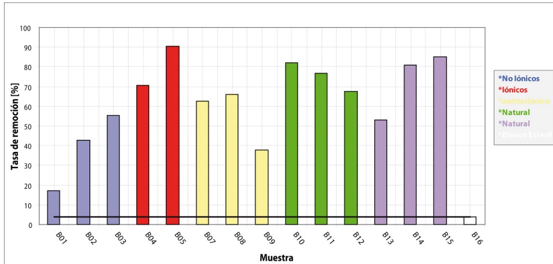
Figura 4.27. Eficiencias de remoción del proceso de biodegradación. La línea negra representa el valor obtenido por el blanco estéril.
