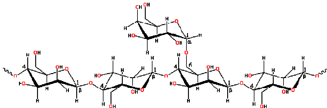
Figura A-3.4. Estructura molecular de la goma de algarrobo.
