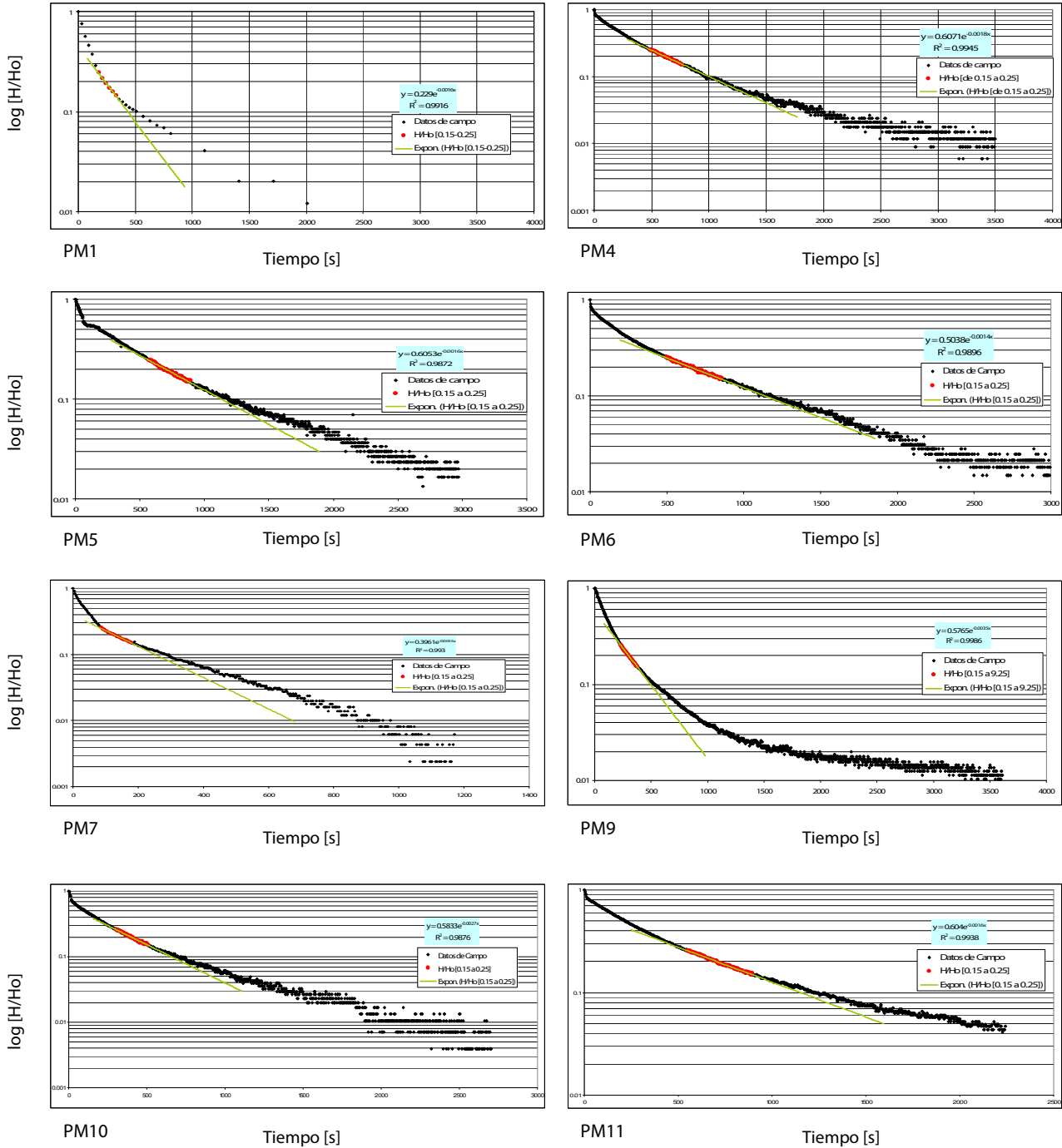
Figura 5.14. Interpretación de las pruebas slug. La línea de tendencia en verde representa la recta calculada para los valores de carga normalizada de 0.15 a 0.25 que Butler (1996) recomienda para el cálculo de la conductividad hidráulica.
