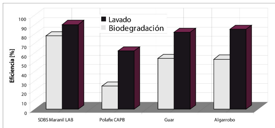
Figura 4.35. Eficiencia del lavado de suelo vs eficiencia de biodegradación.
