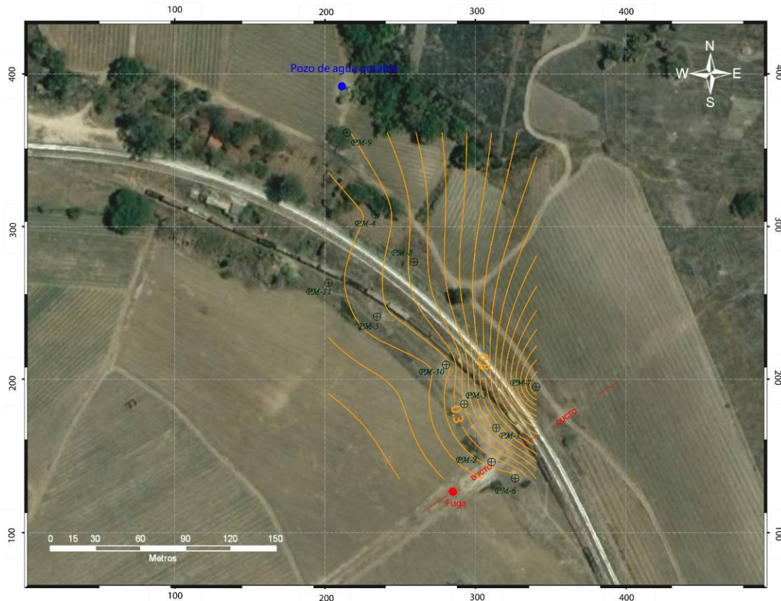
Figura 5.15. Mapa de isoconductividades. Los valores están expresados en m/día.
