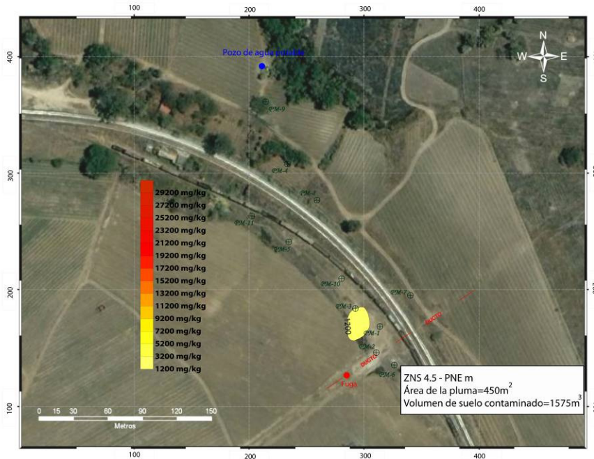
Figura 5.18. Pluma de suelo contaminado de 4.5m a PNE (8m).
