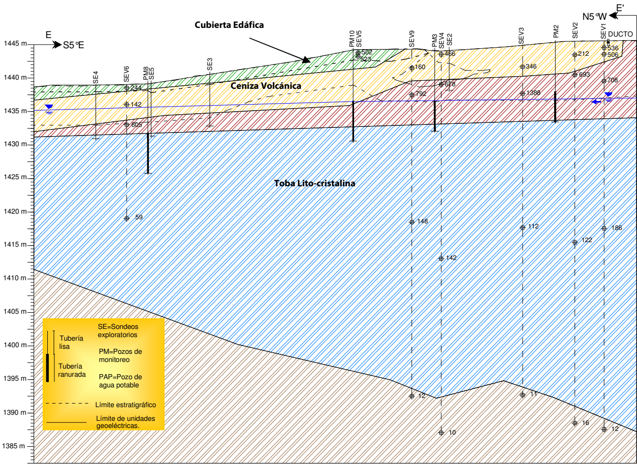
Figura 5.12. Sección geológica – geofísica EE'. Línea negra continua marca los límites entre las unidades geoelectricas. Línea negra discontinua delimita los límites estratigráficos.
