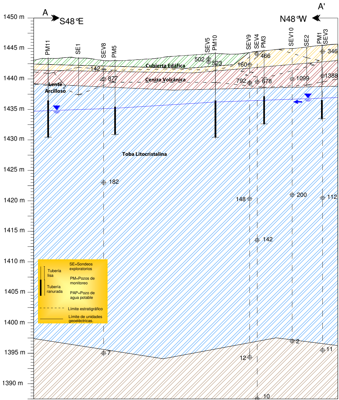
Figura 5.9. Sección geológica-geofísica AA'. Línea negra continua marca los límites entre las unidades geoelectricas. Línea negra discontinua delimita los límites estratigráficos.
