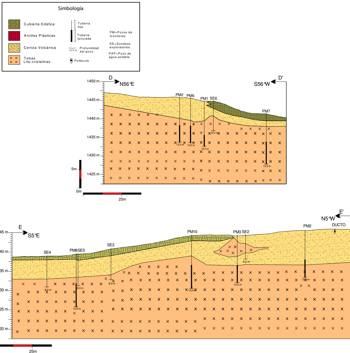
Figura 5.3. Secciones geológicas DD' y EE'.
