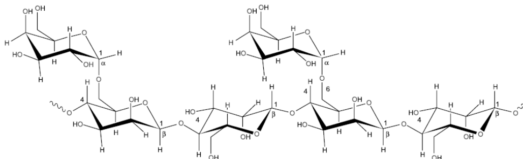
Figura 4.13. Estructura molecular de la goma de guar (Torres et al. , 2007).
