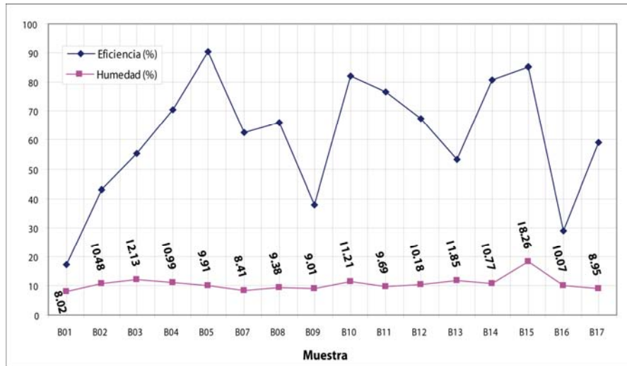
Figura 4.29. Comparación entre la humedad y la eficiencia de cada prueba.
