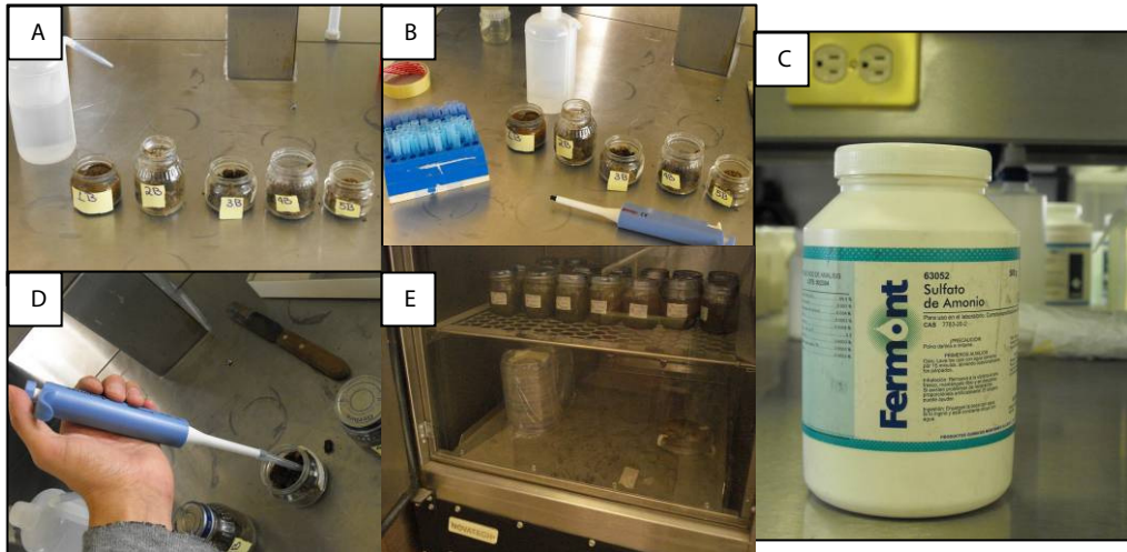
Figura 4.24. A) Frascos en donde se colocaron 30 g de suelo para ser sometidos al proceso de biodegradación; B) Adición de agua destilada para obtener las condiciones adecuadas de humedad. C) Sulfato de amonio; D) Acondicionamiento del suelo con los nutrientes necesarios; E) Incubadora que almaceno los frascos por 3 meses.
