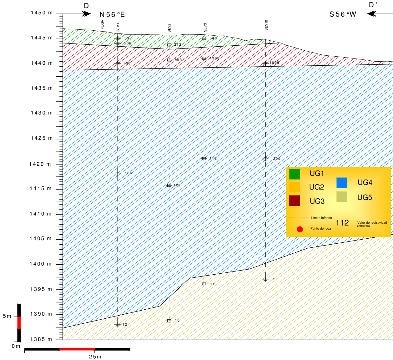
Figura 5.7. Sección geoelectrica DD'.
