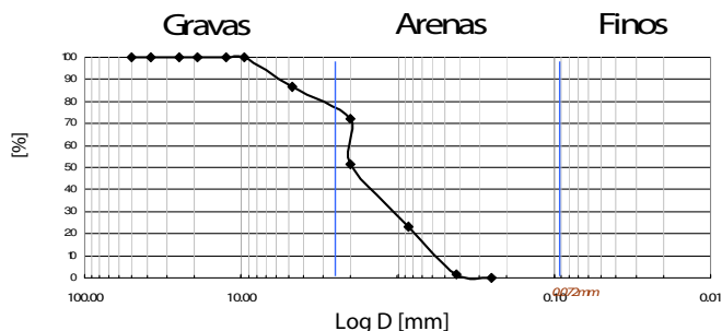
Figura 4.12. Curva granulométrica del suelo contaminado
