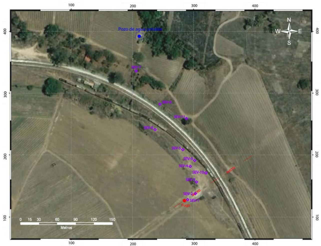
Figura 4.4. Ubicación de los Sondeos Eléctricos Verticales realizados en el sitio.
