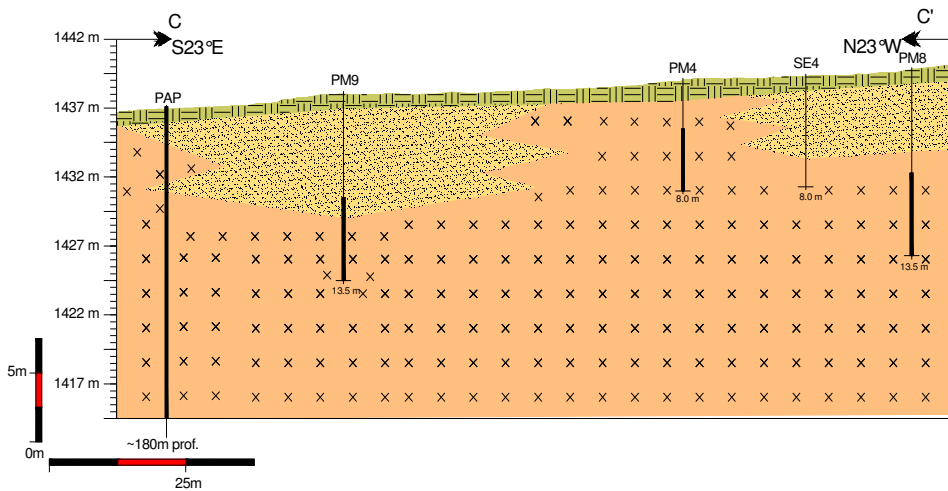
Figura 5.2. Secciones geológicas AA', BB' y CC'.
