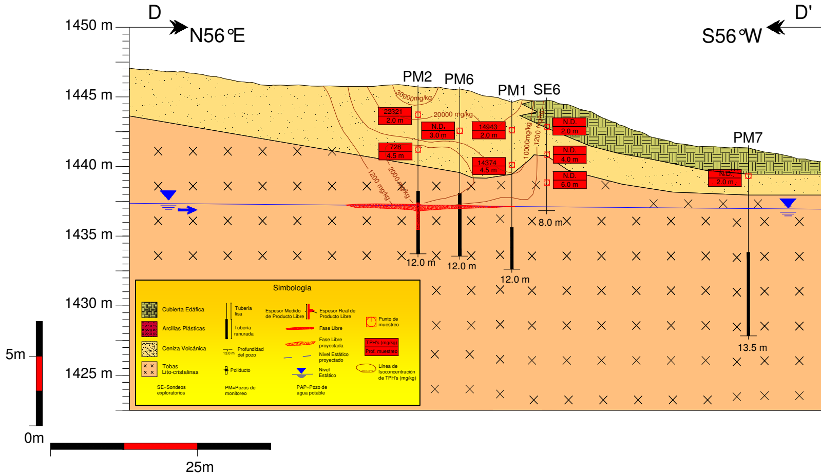
Figura 5.20. Sección de isoconcentraciones. Corte transversal al LNAPL presente.
