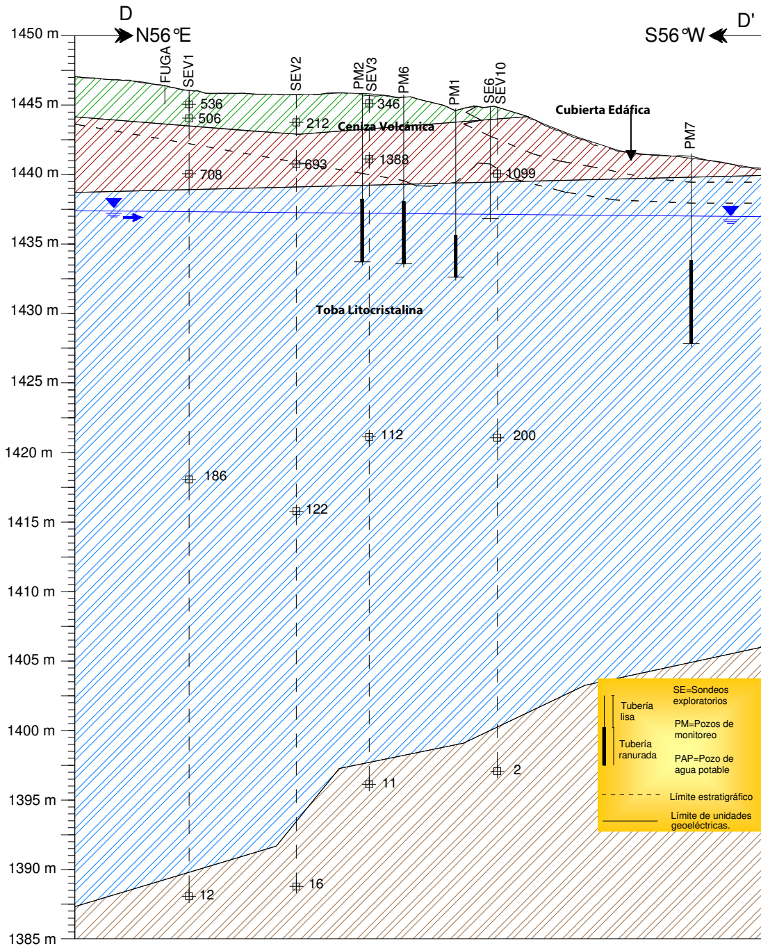
Figura 5.11. Sección geológica – geofísica DD'. Línea negra continua marca los límites entre las unidades geoelectricas. Línea negra discontinua delimita los límites estratigráficos.
