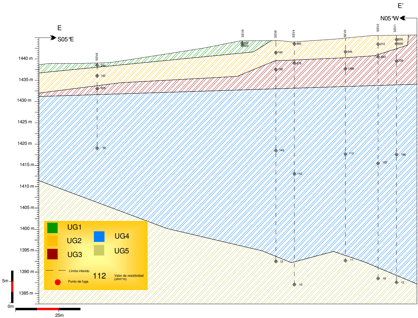
Figura 5.8. Sección geoelectrica EE'.
