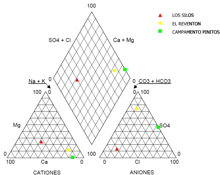
Figura 3.33. Diagrama de Piper con los resultados de los análisis químicos obtenidos en laboratorio. Tomado de IMTA (2007).
