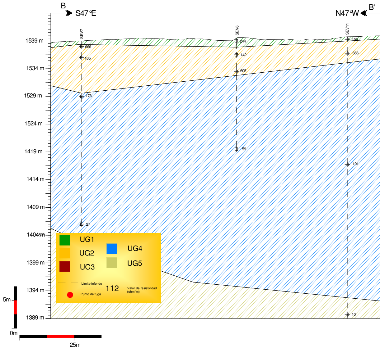
Figura 5.6. Sección geoelectrica BB'.
