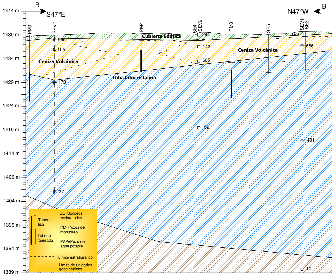
Figura 5.10. Sección geológica – geofísica BB'. Línea negra continua marca los límites entre las unidades geoeléctricas. Línea negra discontinua delimita los límites estratigráficos.
