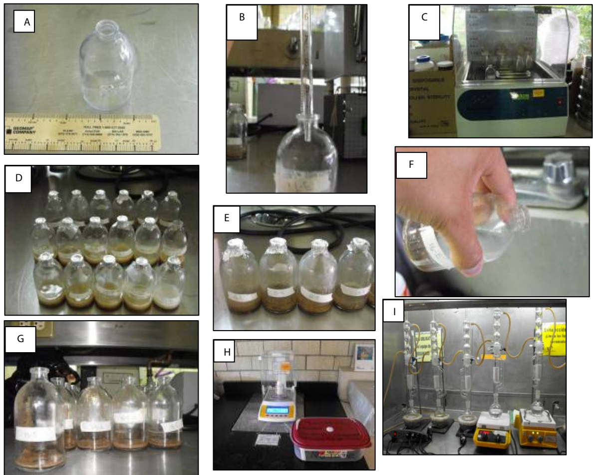
Figura 4.15. Proceso de lavado de suelo. A) dimensión de los viales empleados para almacenar el suelo; B) solución hecha con agua destilada y surfactantes; C) Agitadora que mantuvo girando a los viales a 150 rpm; D) Los 17 viales desarrollados puestos a 1 hr de reposo; E) separación de la fase líquida y el suelo; F) extracción del sobrenadante; G) Suelo después del proceso del lavado; H) Preparativos para la prueba de extracción de TPH; I) Desarrollo de la extracción de TPH del suelo lavado.
