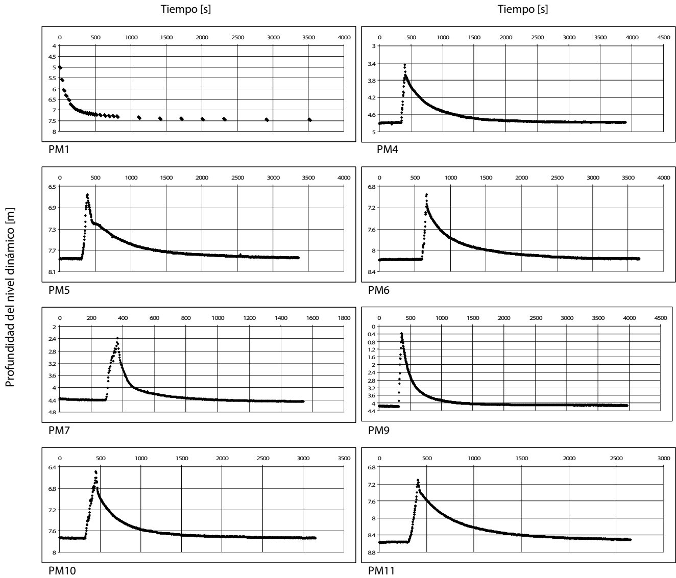
Figura 4.5. Gráficas de las pruebas slug realizadas en los pozos de monitoreo existentes.
