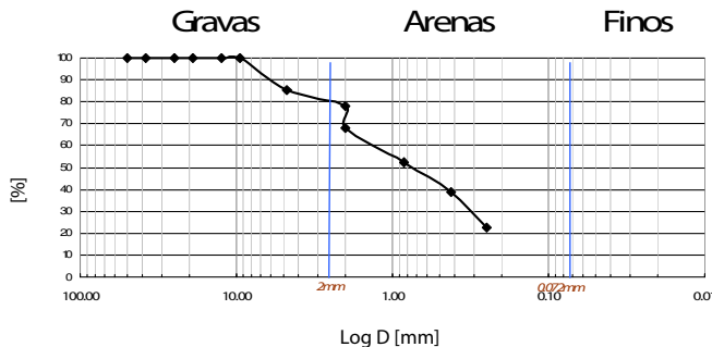
Figura 4.11. Curva granulométrica del suelo sin contaminar.
