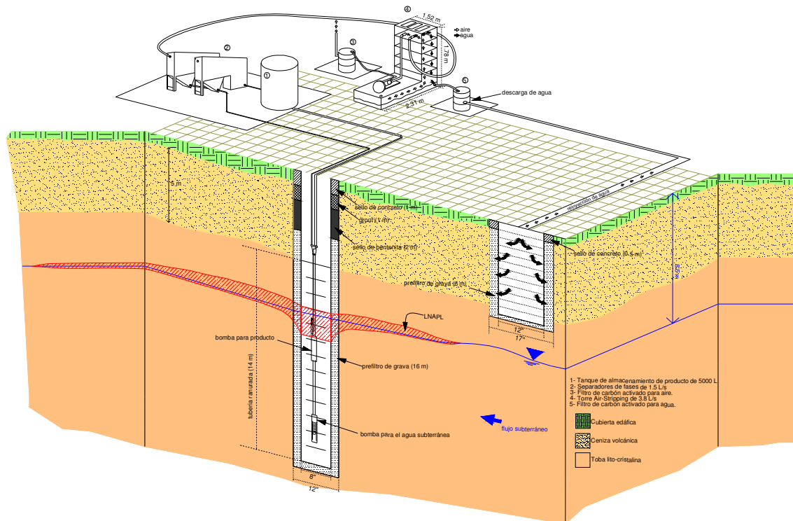
Figura 5.31. Diagrama constructivo de un pozo WER
