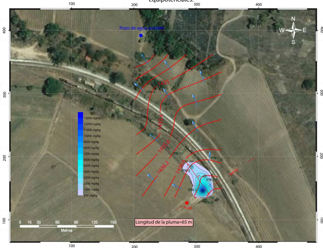
Figura 5.28. Pluma en fase disuelta de xilenos totales. Adicionalmente se muestra la dirección de flujo del agua subterránea y las líneas equipotenciales.
