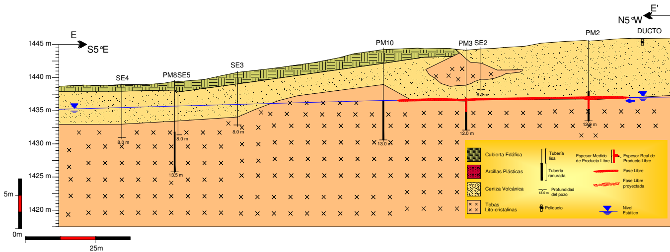
Figura 5.24. Sección EE'. Capa roja esquematiza la fase libre presente en el subsuelo.
