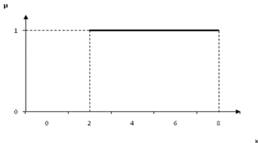
Figura 16 Intervalo [2, 8]
