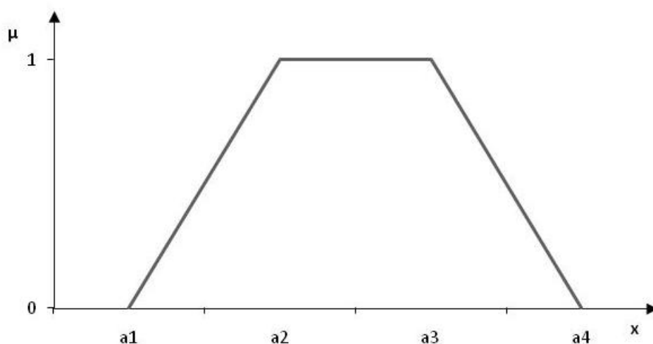
Figura 19 Número borroso trapezoidal (NBTr)
