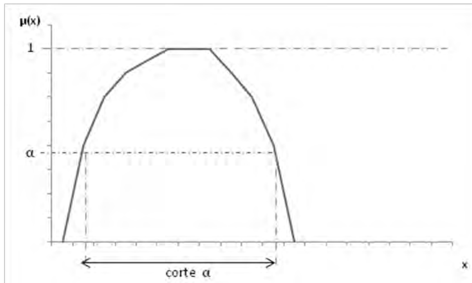
Figura 12 Conjunto convexo
