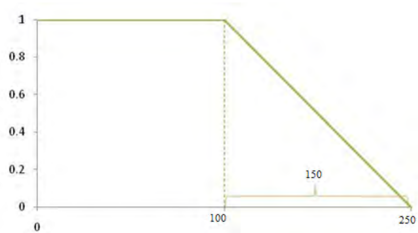
Figura 23 Comportamiento de la demanda para el período t=1.
