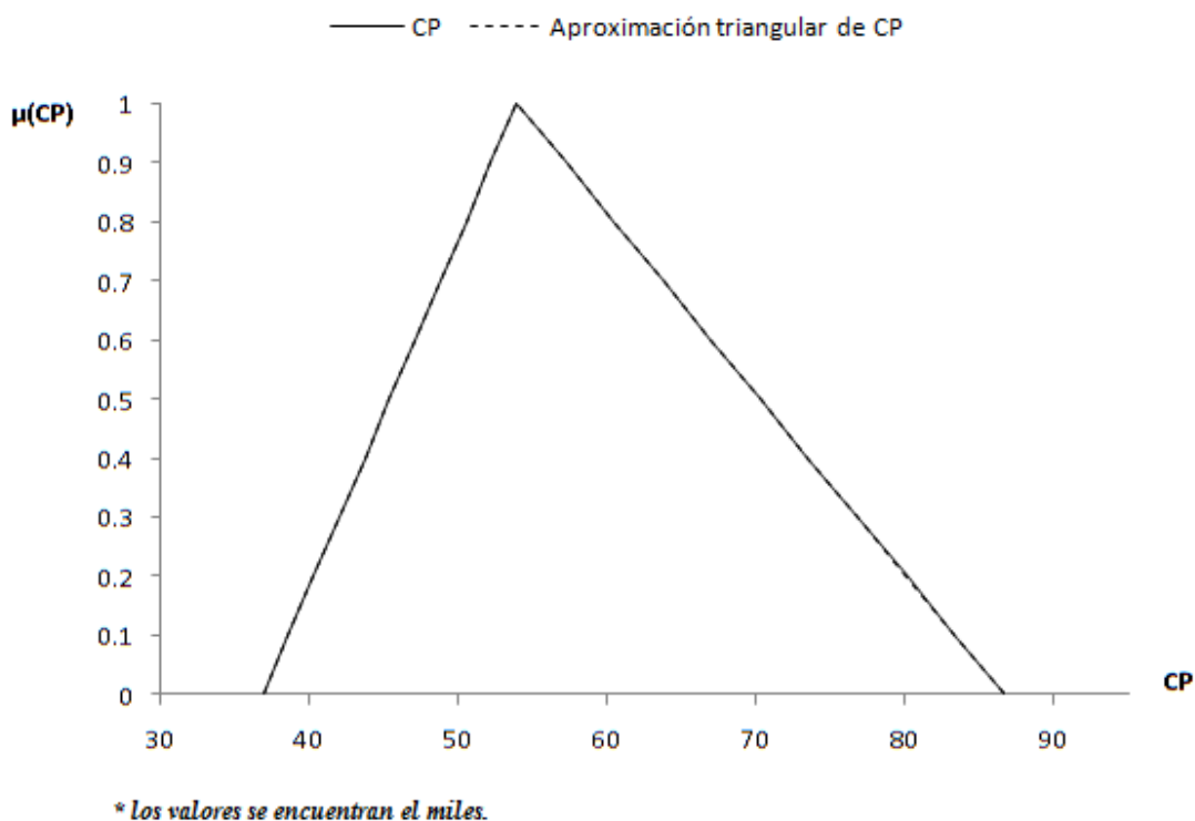
Figura 29 Representación gráfica del costo promedio
