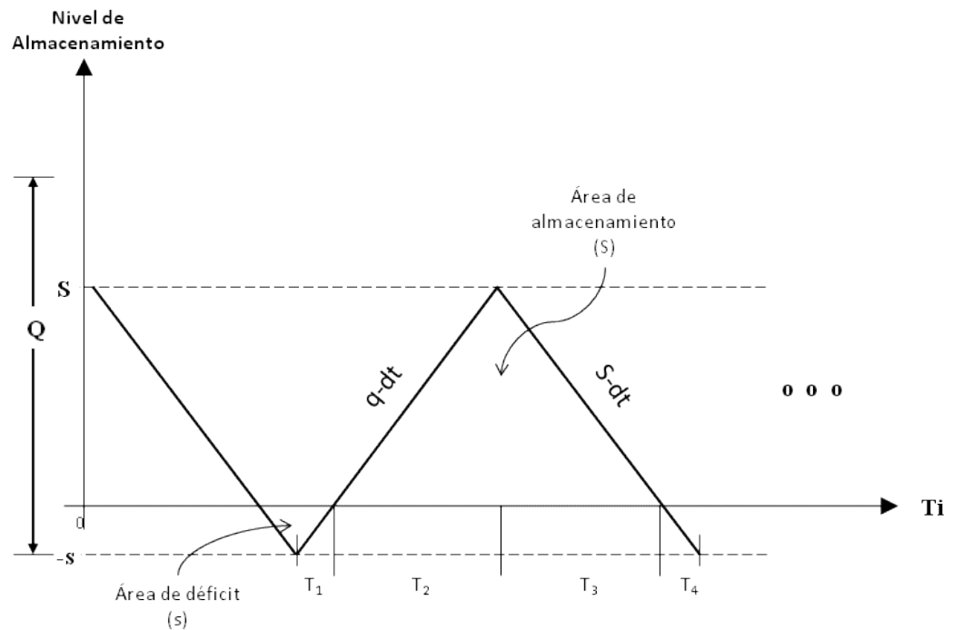
Figura 9 Comportamiento del nivel del inventario
