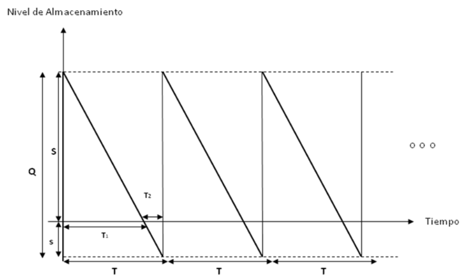
Figura 8 Modelo sin producción con déficit
