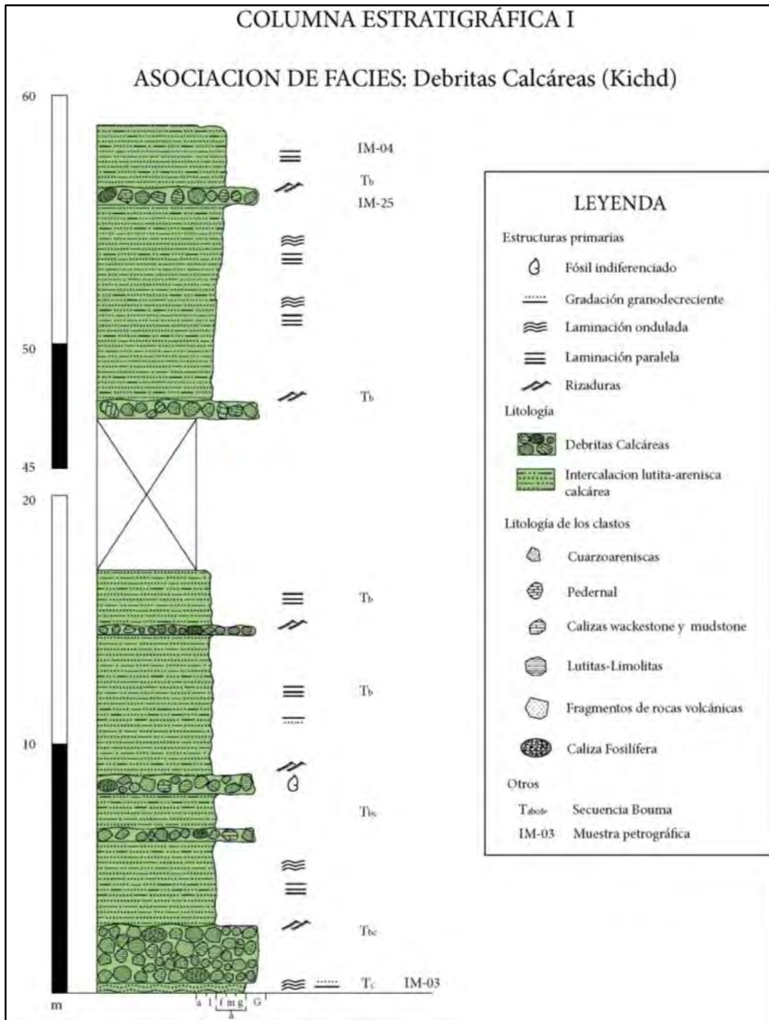
Figura 4.IV.2. Columna estratigráfica I, medida a partir de la coordenadas Latitud 18°29'41.71'' N y Longitud 97°22'10.92'' W, (Ver Mapa de Asociación de Facies para seguir trayectoria de medición).
