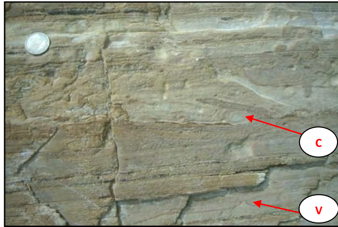
Figura 4.V.1. Intercalación de litofacies Limo (Li) y Lutita (Lu) con estructuras de escape de agua como volcanes de arena (Va) y laminación convoluta (C). Longitud de la moneda 2 cm. Localización del afloramiento: nivel ~ 286 m de la columna medida II.
