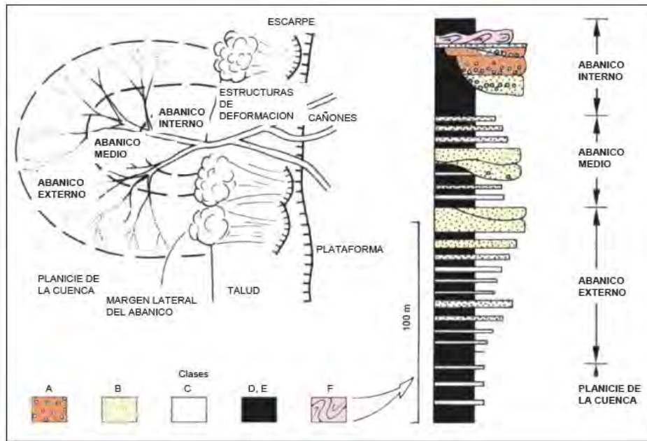
Figura 2.5. Vista en planta del modelo de abanico submarino conceptualizado y secuencia regresiva hipotética de un modelo de abanico submarino. Tomado de: Mutti y Ricci-Lucci (1972 en Santillán-Piña, 2009).
