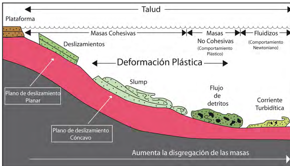
Figura 2.4. Esquema donde se muestran los cuatro procesos básicos de transporte de sedimentos hacia aguas profundas. Tomado de Shanmugam y Moiola, (1994 en Shanmugam, 2006).
