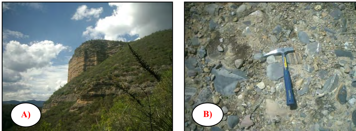
Figura 3.5. Conglomerado San Isidro, A) vista panorámica hacia el norte del Cerro Colorado desde el sur donde se observa estratificación, B) Conglomerado San Isidro; polimíctico, con abundantes fragmentos de calizas de la Formación Miahuatpec, longitud del martillo 33 cm. Localización del afloramiento: Latitud 18° 28' 41.73'' N y Longitud 97° 19' 38.98'' W.
