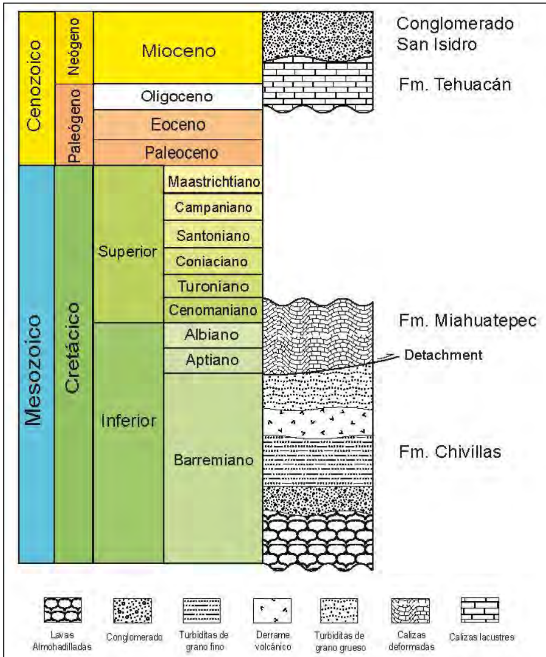
Figura 3.2. Columna estratigráfica del área de estudio.
