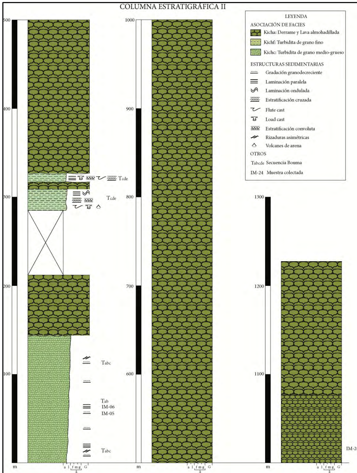
Figura 4.I.1. Columna estratigráfica II, medida en la Barranca Las Salinas a partir de las coordenadas: Latitud 18°29'13.44'' N y Longitud 97°22'7.10'' W, (Ver Mapa de Asociación de Facies para seguir la trayectoria de medición).
