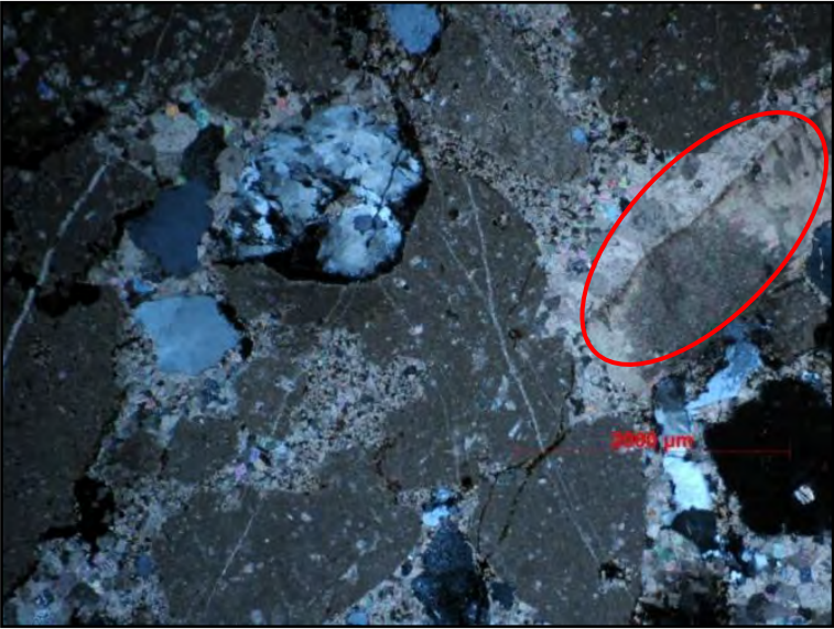
Fotomicrografía con nicols cruzados 2.5x: Se observan fragmentos redondeados de mudstones y en la esquina superior derecha (Fp) se encuentra el corte transversal de pelecípodo. Los fragmentos de cuarzo monocristalino son subangulares.
