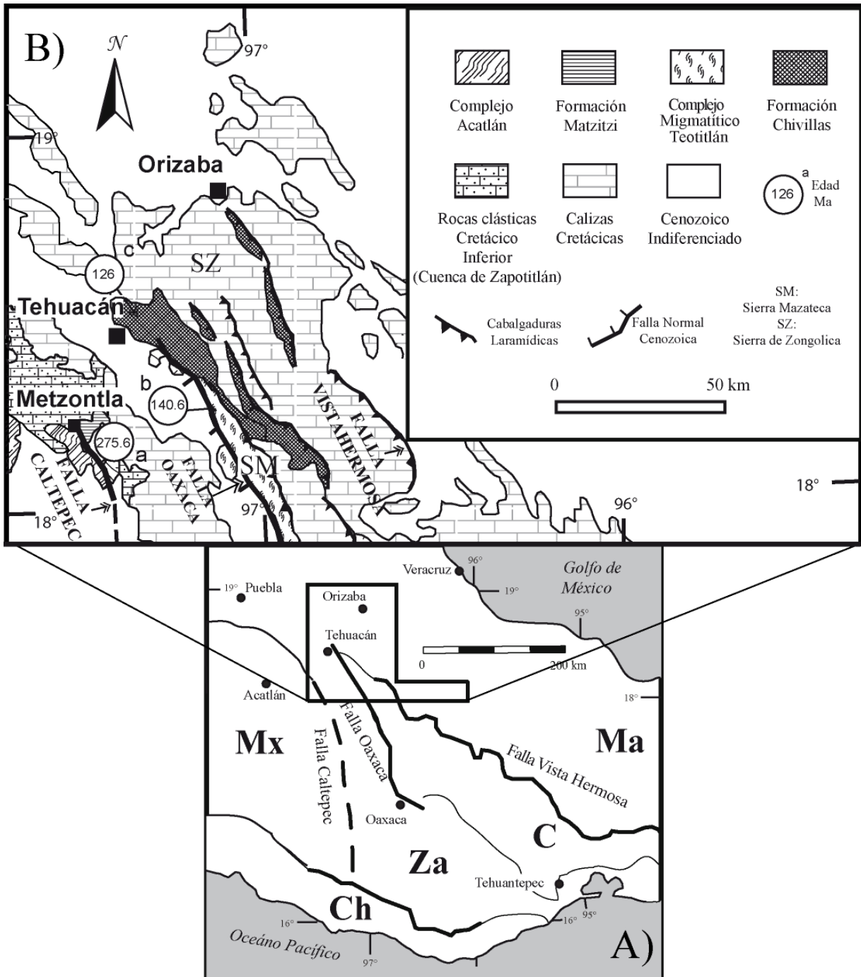
Figura 3.1. Mapa Geológico Regional, modificado de: Mendoza-Rosales et al., 2010. A) Mapa de terrenos tectonoestratigráficos del Sureste de México (Sedlock et al. 1993) Mx; Mixteco, Za; Zapoteco, C; Cuicateco, Ma; Maya, Ch; Chatino. B) Mapa modificado de INEGI, 1994; Ortuño-Arzate et al., 1992; Ángeles-Moreno, 2006. Círculos representan edades datadas por: (a) Elías Herrera et al., 2005 (b) Ángeles-Moreno, 2006; (c) Mendoza Rosales et al. 2010.
