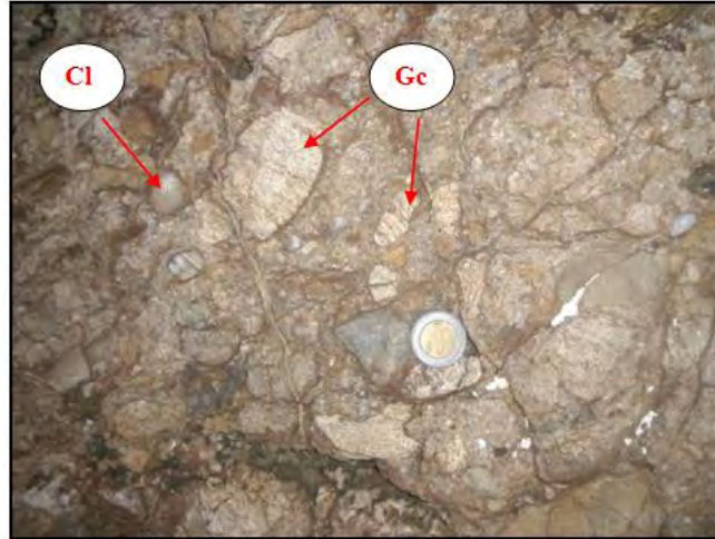
Figura 4.II.4. Conglomerado polimíctico soportado por matriz de arena gruesa. Se aprecian clastos de gneises (Gc) y cuarzo lechoso (Cl) entre otros clastos de areniscas y lutitas soportados por matriz de arena gruesa. Longitud de la moneda 2 cm. Localización del afloramiento: Latitud 18°19'0.34''N y Longitud 97°22'15.88''W.
