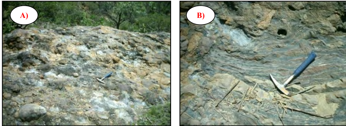
Figura 4.II.1. A) Depósito de flujo de detritos con el espesor más potente de la formación. B) Turbiditas de grano fino intercaladas entre las debritas; se aprecia como la superficie de contacto es irregular. Longitud de martillo 33 cm: Localización del afloramiento: Latitud 18°31'48.83''N y Longitud 97°20'53.06''W.
