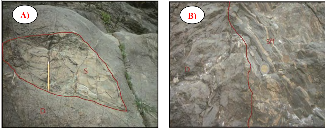
Figura 4.I.4. Litofacies de peperitas (Exp). A) Sedimento (S) atrapado en un flujo de lava (D), longitud del lápiz 18 cm. Localización del afloramiento: Latitud 18°30'52.33'' N y Longitud 97°21'29.61''W, B) contacto entre flujo de lava (D) y sedimentos del tipo flujos fluidizados (Sff), longitud de la moneda 2.5 cm. Localización del afloramiento: Latitud 18°33'5.58''N y Longitud 97°21'20.77''W.
