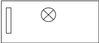
Ubicación de fotomicrografías en lámina delgada
