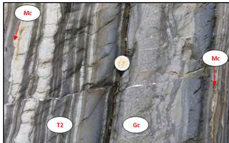
Figura 4.V.4. Imagen representativa de litofacies Lu y Li con estructuras sedimentarias parte de la Secuencia Stow, T_2 Lam. delgada irregular. Otras estructuras presentes son: gradación granocreciente (Gc) y (Mc) marcas de carga. Longitud de la moneda 2.5 cm. Localización del afloramiento: Latitud 18^{\circ} 32' 8.95'' N y longitud 97^{\circ} 21' 2.28'' W.
