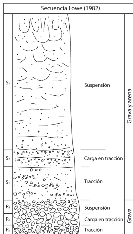
Figura 2.3. Redibujado de Lowe, (1982). Secuencia de Lowe para el reconocimiento de depósitos de corrientes turbidíticas de alta densidad. Note que los mecanismos de sedimentación son clave para diferenciación de estos depósitos.
