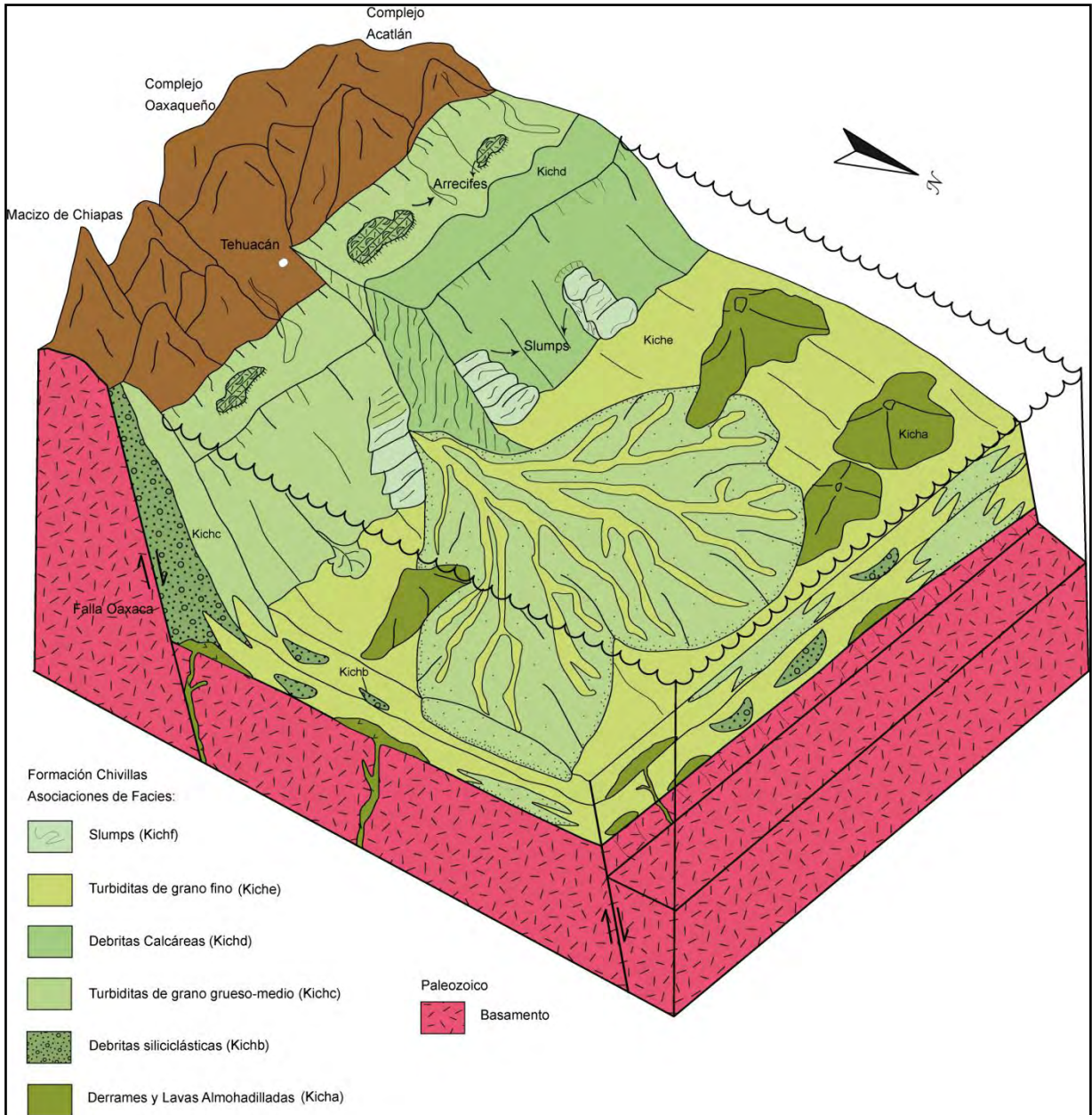
Figura 5.3. Modelo de facies para la Formación Chivillas, donde se aprecia la distribución de las asociaciones de facies en el abanico submarino, las progradación de los lóbulos, las principales fuentes detríticas y las fallas que controlaron la depositación.
