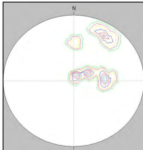
Figura 4.VI.1. Red estereográfica con los datos de inclinación de planos axiales de los pliegues sin-sedimentarios. El promedio de los datos estructurales es: 42° de inclinación al NE 83°.
