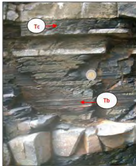
Figura 4.V.2. Detalle de estructuras de la asociación de facies Kiche. Las facies de la Secuencia Bouma T_b , laminación paralela, T_c estratificación cruzada y T_e horizontes de lutita homogéneas. Longitud de la moneda 2.5 cm. Localización del afloramiento: Latitud 18^{\circ}33'25.4'' N y Longitud 97^{\circ}21'22.01'' W.
