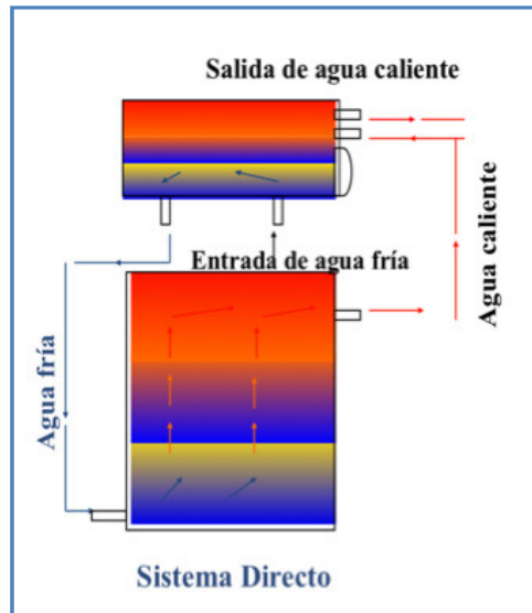
Figura 4.5 Esquema de funcionamiento de los calentadores solares instalados en el conjunto habitacional. Fuente: Heliocol, 2009
