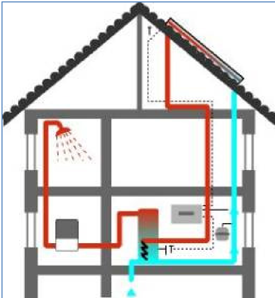
Figura 2.13 Esquema de funcionamiento de un calentador solar en una vivienda. Fuente: Wikipedia, 2009
