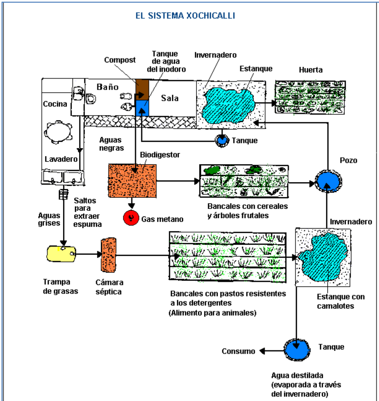
Figura A 3 Esquema de tratamiento de aguas en la casa "Xochicalli"
