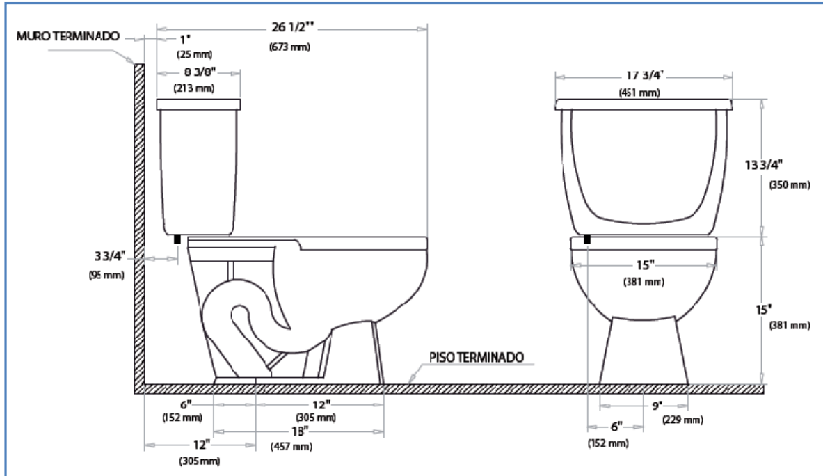
Figura 4.3. Esquema de las dimensiones del inodoro Marathon Fuente: Vitromex, 2010
