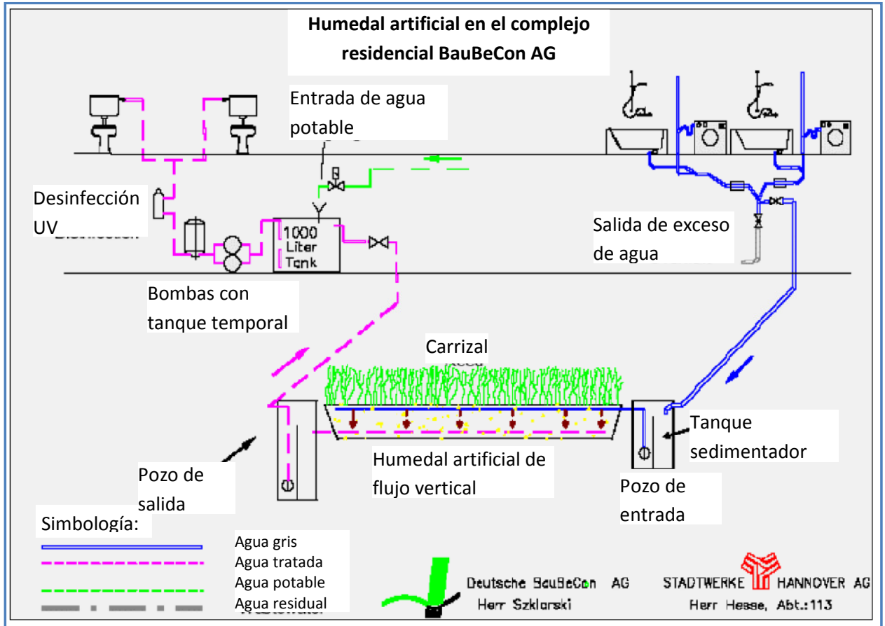
Figura 2.4 Esquema 3 de manejo integral del agua residual por uso de humedal artificial. Fuente: Oeko-Technik-Park
