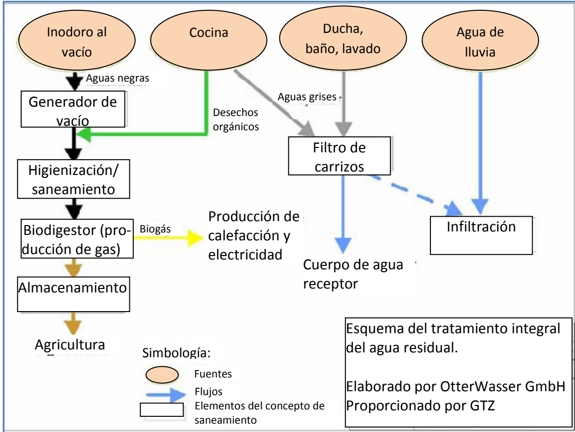
Figura 2.2 Esquema 1 de manejo integral del agua residual. Fuente: OW GmbH
