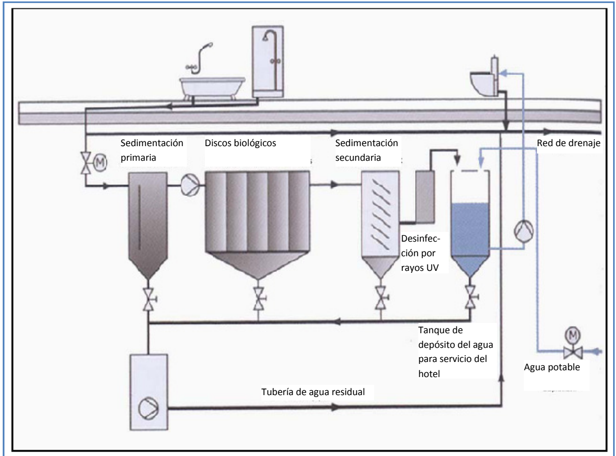
Figura 2.3 Esquema 2 del manejo integral del agua residual (proceso de recolección, tratamiento y reciclaje de aguas grises) Fuente: DVA, GTZ
