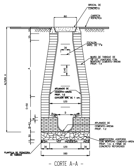
- CORTE A-A - POZOS DE VISITA SOBRE TUBERIAS DE 30 A 61 cm. DE DIAMETRO
