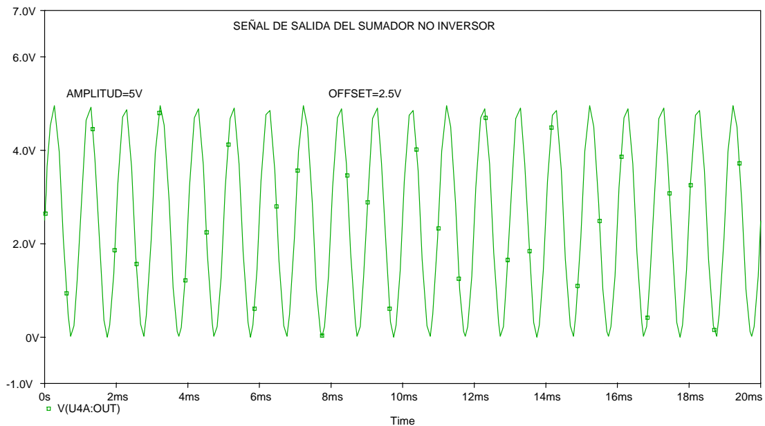
FIGURA 5.24- SALIDA DEL SUMADOR NO INVERSOR
