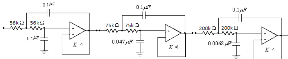
FIGURA 5.7- FILTRO BUTTERWORTH DE 6 o ORDEN, FRECUENCIA DE CORTE 30 HZ
