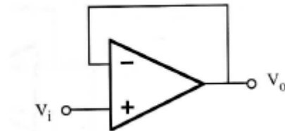
FIGURA 2.7. AMPLIFICADOR SEGUIDOR
