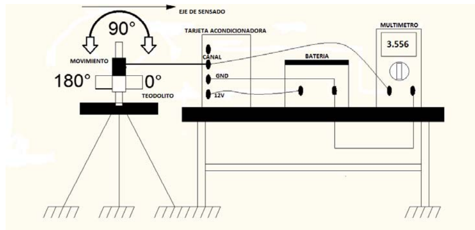
FIGURA 6.1- PRUEBA DE CALIBRACIÓN DEL ACCELERÓMETRO
