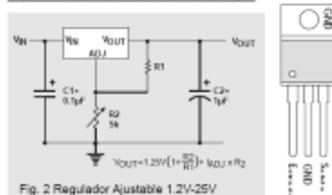
Fig. 2 Regulador Ajustable 1.2V-25V
