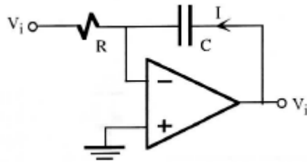
FIGURA 2.10- AMPLIFICADOR INTEGRADOR
