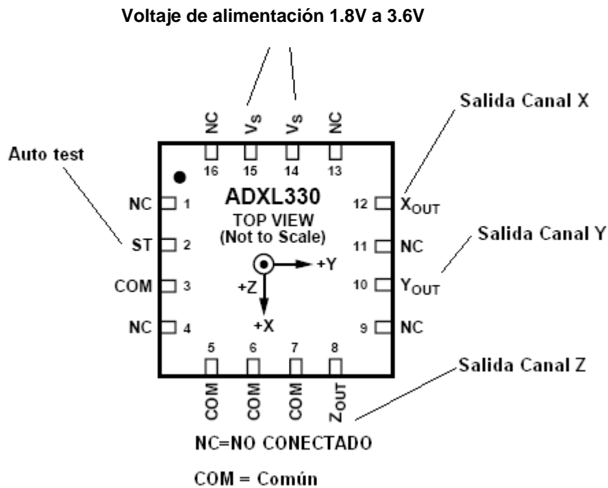
FIGURA 1.6- DISTRIBUCIÓN DE PINES DEL ADXL330
