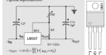
Fig. 3 Regulador de Voltaje Negativo
