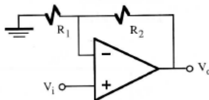
FIGURA 5.16- AMPLIFICADOR NO INVERSOR
