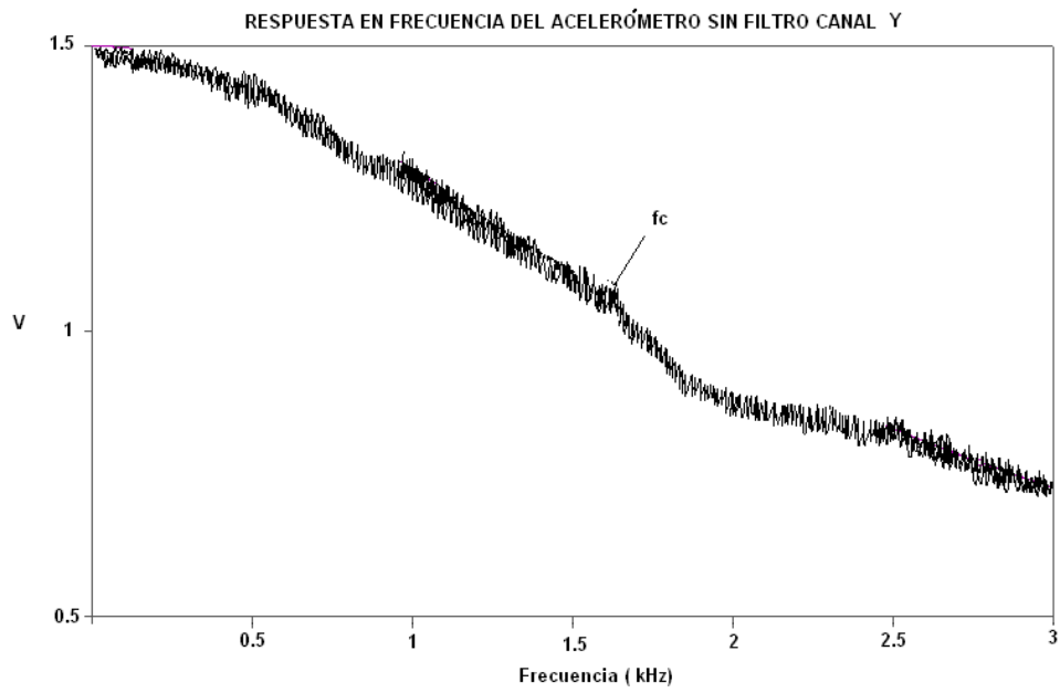
FIGURA 6.12- RESPUESTA EN FRECUENCIA CANAL Y DEL ACELERÓMETRO ADXL SIN FILTRO
