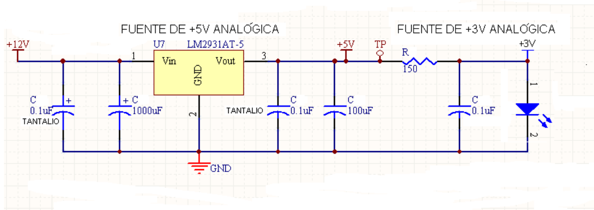
FIGURA 5.28- FUENTE ANALÓGICA DE 3V
