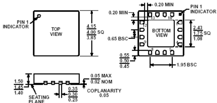
FIGURA 1.7- DIMENSIONES DEL ADXL330 EN MILÍMETROS [6]
