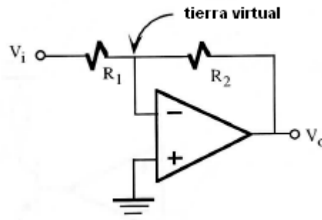
FIGURA 2.5- AMPLIFICADOR INVERSOR
