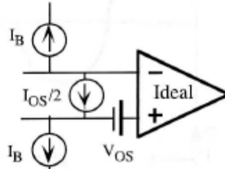
FIGURA 2.14- MODELO DE UN AMPLIFICADOR OPERACIONAL CON CORRIENTES Y VOLTAJES DE OFFSET
