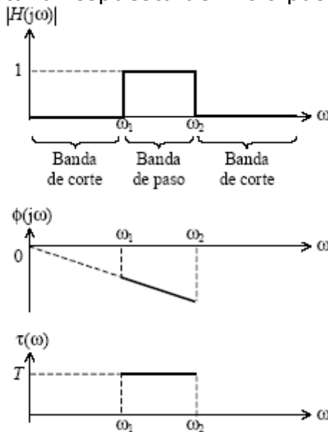
FIGURA 3.7- MAGNITUD, FASE Y RETRASO DE GRUPO DE UNA RESPUESTA PASO BANDA [14]
