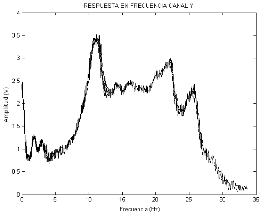
FIGURA 6.15- RESPUESTA EN FRECUENCIA CANAL Y
