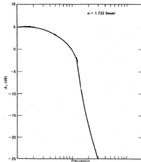
FIGURA 3.12-FILTRO BESSEL
