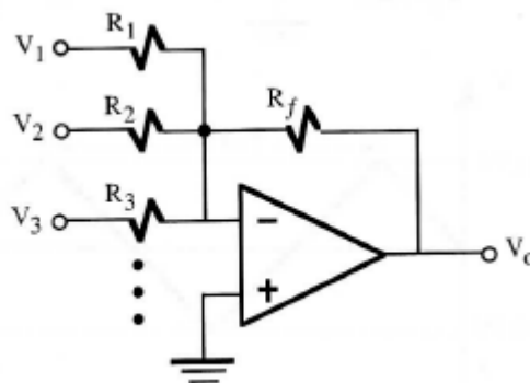
FIGURA 5.20- AMPLIFICADOR SUMADOR
