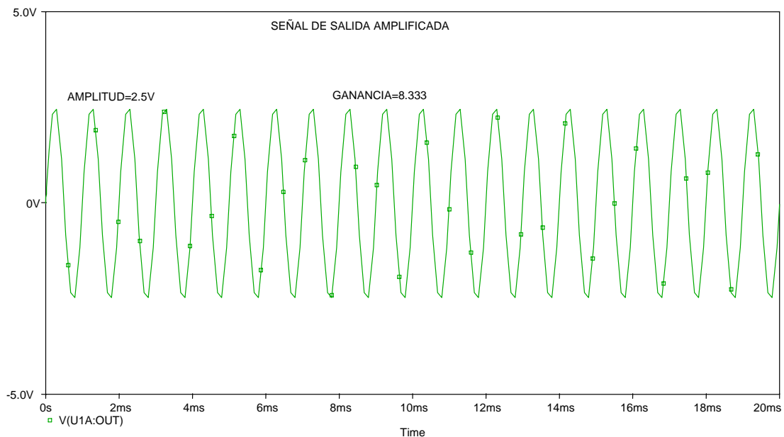
FIGURA 5.19- SEÑAL DE SALIDA AMPLIFICADA A=8.333
