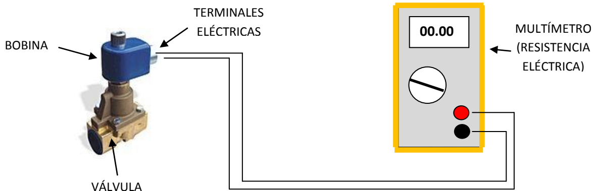
FIG. 6.5 CIRCUITO DE PRUEBA PARA ELECTROVÁLVULA HIDRÁULICA. RESISTENCIA DE LA BOBINA
