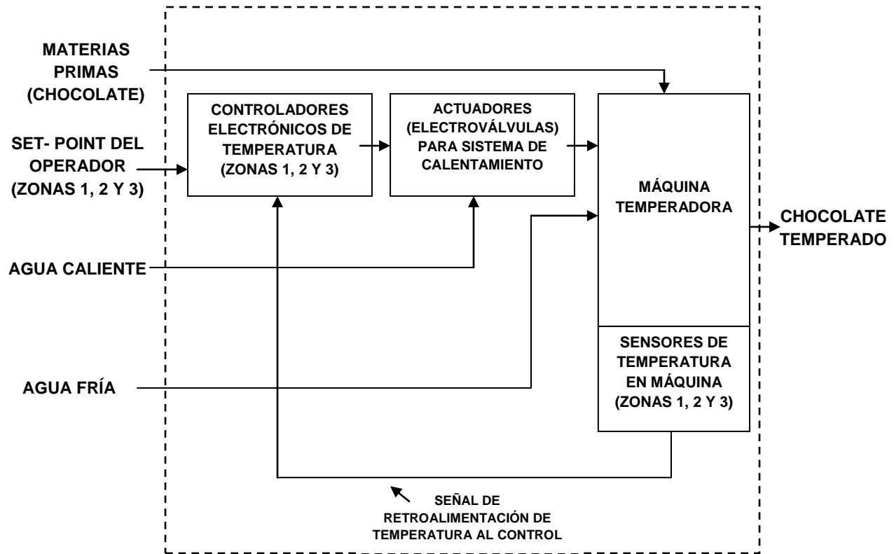
FIGURA 3.2 DIAGRAMA PARA DEFINIR LA ESTRUCTURA FUNCIONAL
