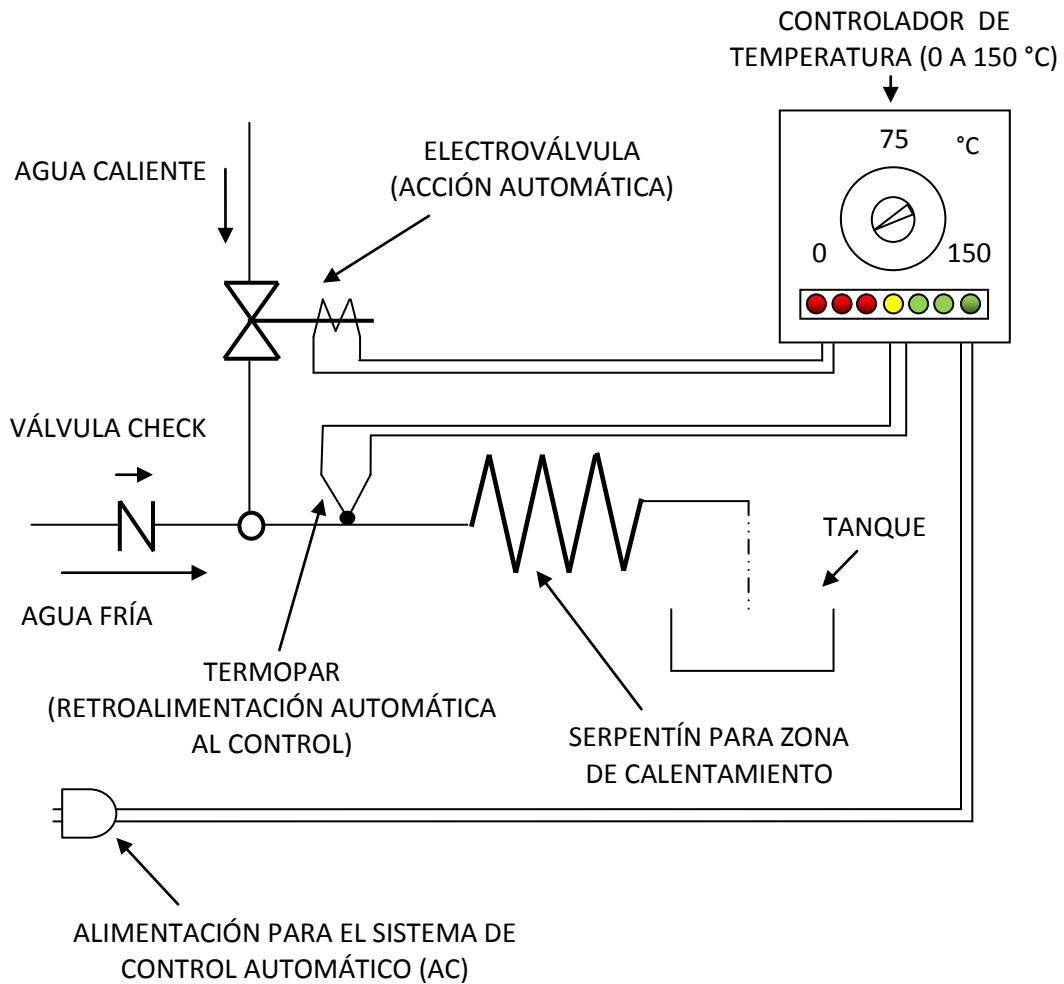
FIGURA 7.2 INTEGRACIÓN DE COMPONENTES MECATRÓNICOS
