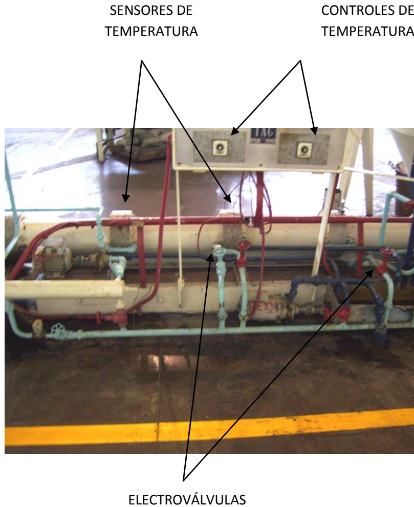
FIG 7.3 COMPONENTES MECTRONICOS INTEGRADOS EN LA MÁQUINA TEMPERADORA
