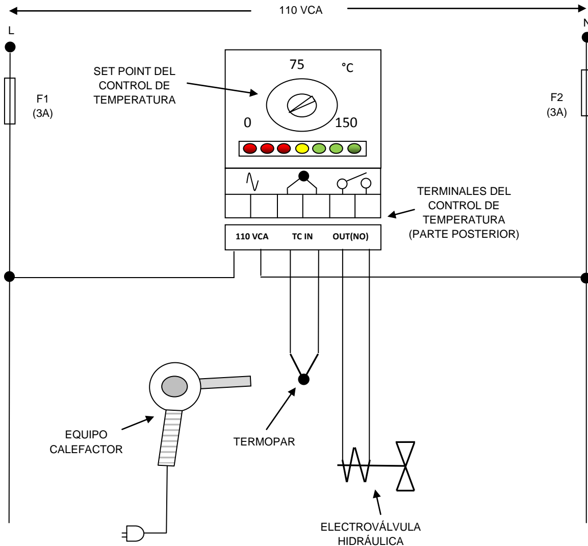
FIG. 7.1 CIRCUITO DE LA INTEGRACIÓN DE COMPONENTES
