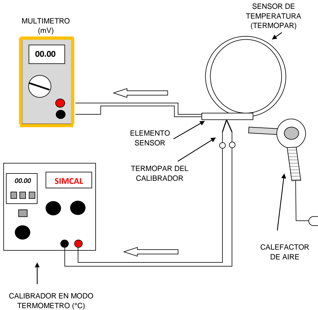
FIG. 6.4 CIRCUITO DE PRUEBA PARA EL SENSOR DE TEMPERATURA
