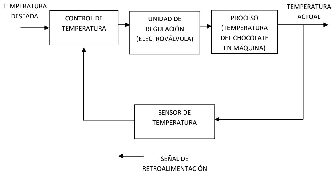
FIG. 7.8 DIAGRAMA DE BLOQUES DEL SISTEMA DE CONTROL DE TEMPERATURAS EN LA MÁQUINA TEMPERADORA.
