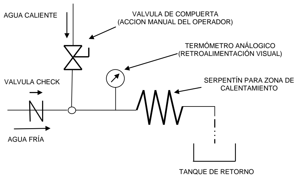
FIG. 4.3 SISTEMA DE CONTROL MANUAL DE TEMPERATURA
