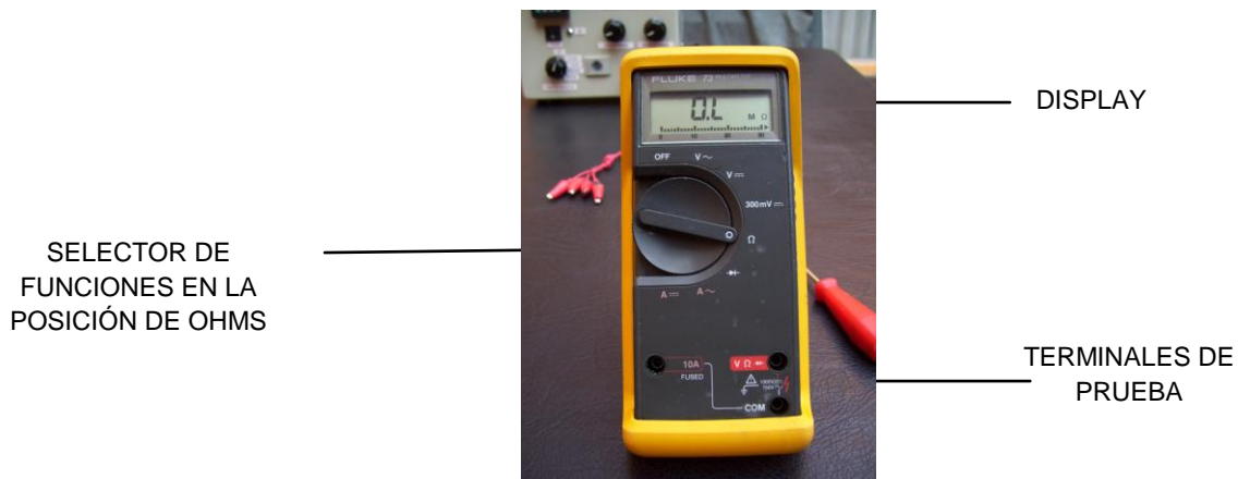
FIG. 6.2 MULTÍMETRO MARCA FLUKE MODELO 73
