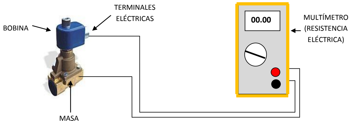
FIG 6.6 CIRCUITO DE PRUEBA PARA ELECTROVÁLVULA. RESISTENCIA DEL AISLAMIENTO
