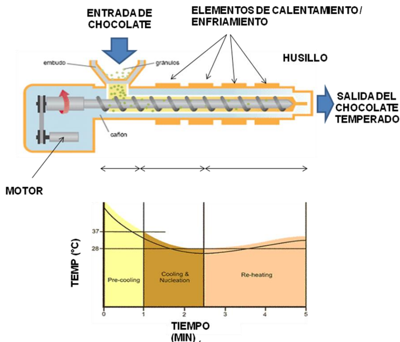
FIG 1. DIAGRAMA GENERAL DE MÁQUINA TEMPERADORA (ARRIBA). ESPECIFICACIONES DEL PROCESO (ABAJO)
