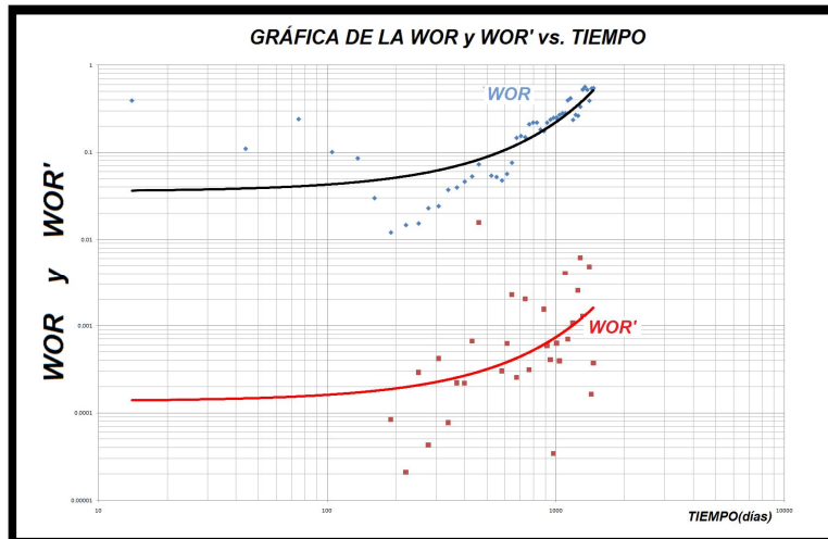
Figura 5.14 Gráfica de la WOR y WOR' vs. tiempo para el pozo Otumba-22. Periodo de producción de agosto de 2003 a agosto de 2007 para la producción del intervalo 4810-4840 m.
