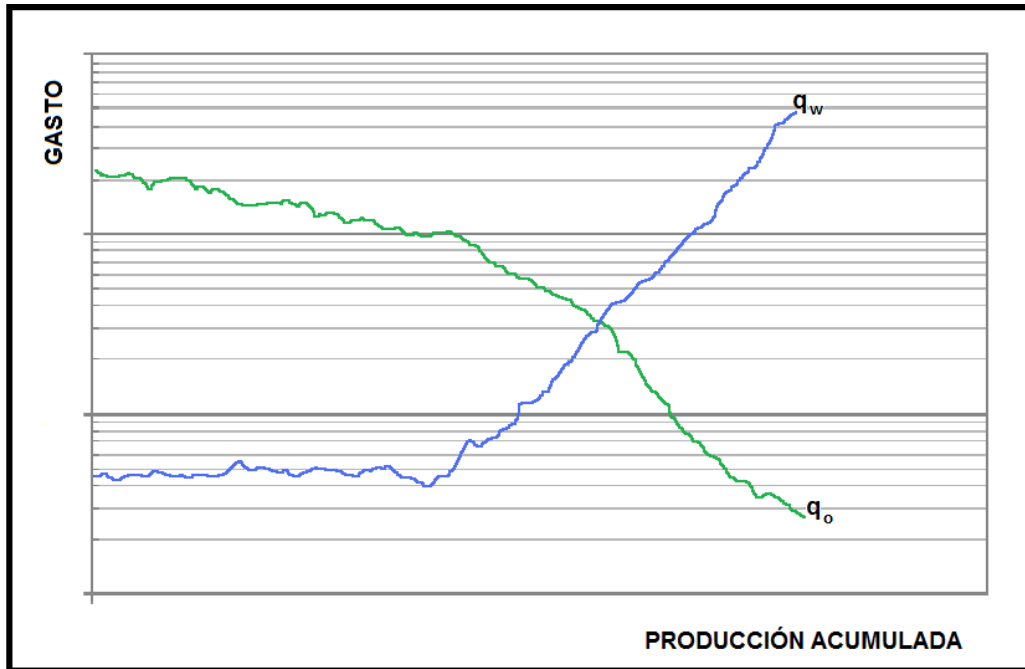
Figura 3.9 Muestra un cambio brusco en las pendientes de aceite y agua, constituyendo una advertencia de que el exceso de agua puede estar afectando la producción normal.
