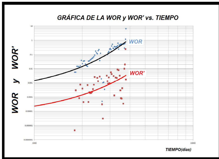
Figura 5.23 Gráfica de la WOR y WOR' vs. tiempo para el pozo Unam-31.
