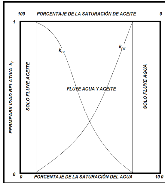
Figura 1.8 Curvas de permeabilidad relativa.
