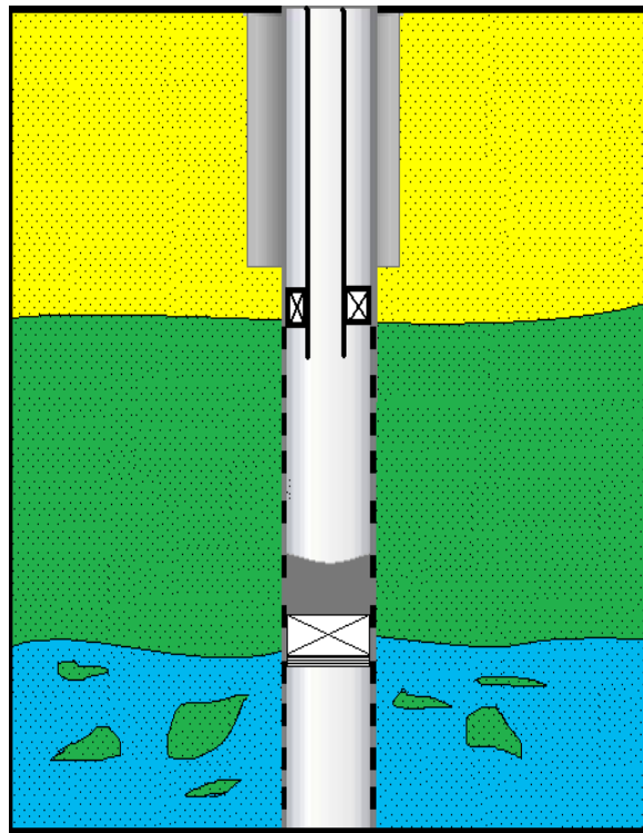
Figura 4.7 Tapón de cemento colocado para aislar un estrato invadido.
