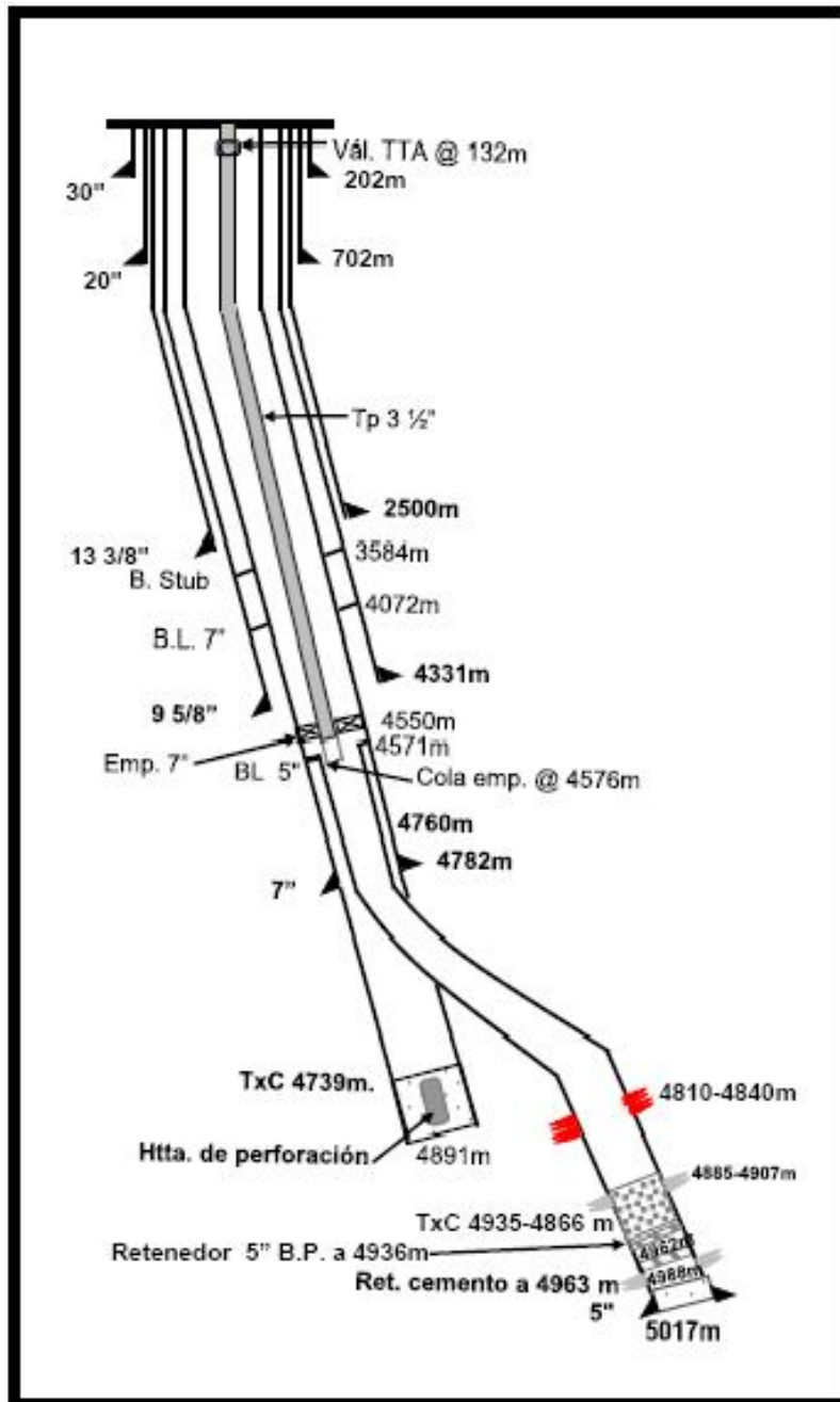
Figura 5.10 Estado mecánico del pozo Otumba-22.
