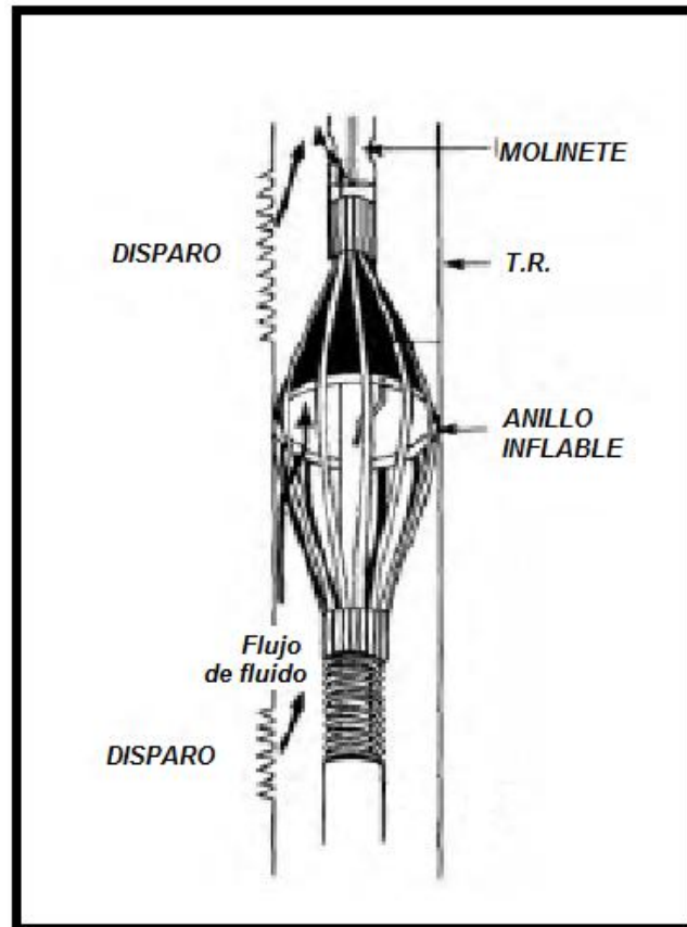
Figura 3.24 Medidor de flujo con empacador inflable.
