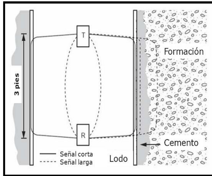
Figura 3.31 Diagrama esquemático de la herramienta CBL.
