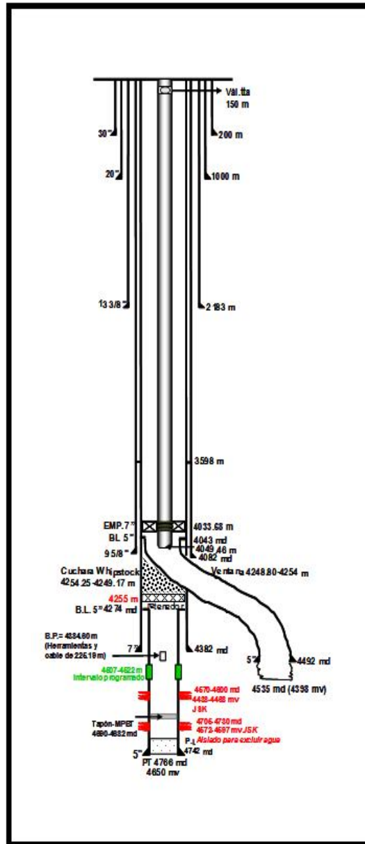
Figura 5.29 Estado mecánico del pozo Puma-13.
