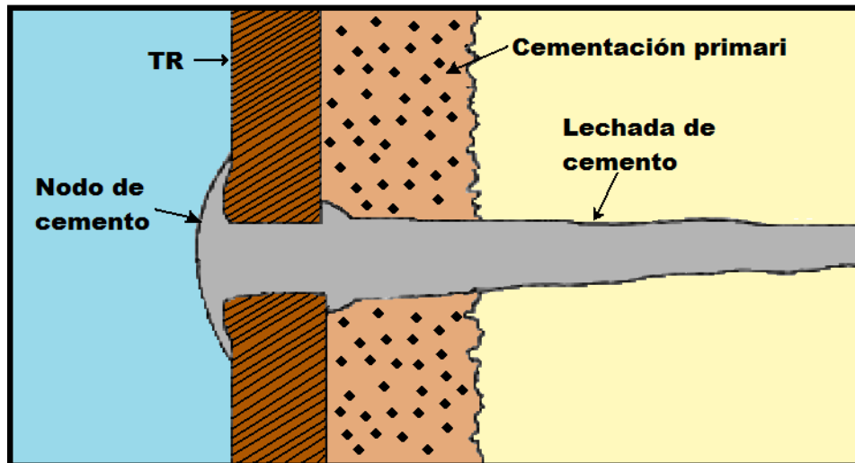
Figura 4.19 Cementación forzada con bombeo continuo.
