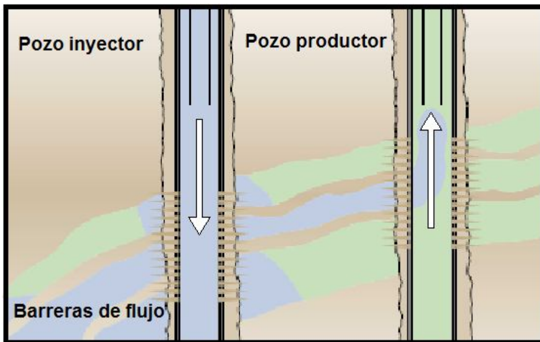
Figura 2.8 Digitalización en yacimiento estratificado con barreras de flujo.
