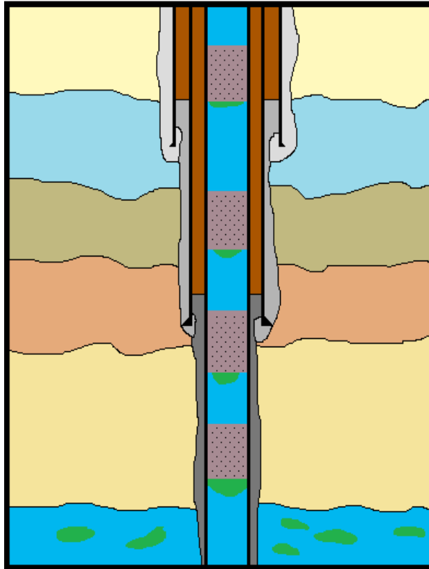
Figura 4.8 Tapones de cemento para abandonar un pozo.
