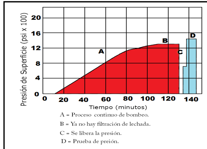
Figura 4.20 Diagrama para el proceso por el cual se bombea una lechada de forma continua.
