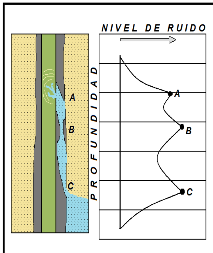
Figura 3.30 La onda de ruido es un indicador de la profundidad a la cual se tiene movimiento de fluidos.
