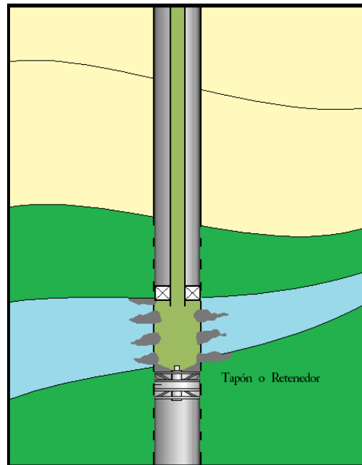
Figura 4.16 Cementación forzada para aislar un intervalo invadido de agua, utilizando un tapón mecánico o un retenedor para no afectar la zona inferior.
