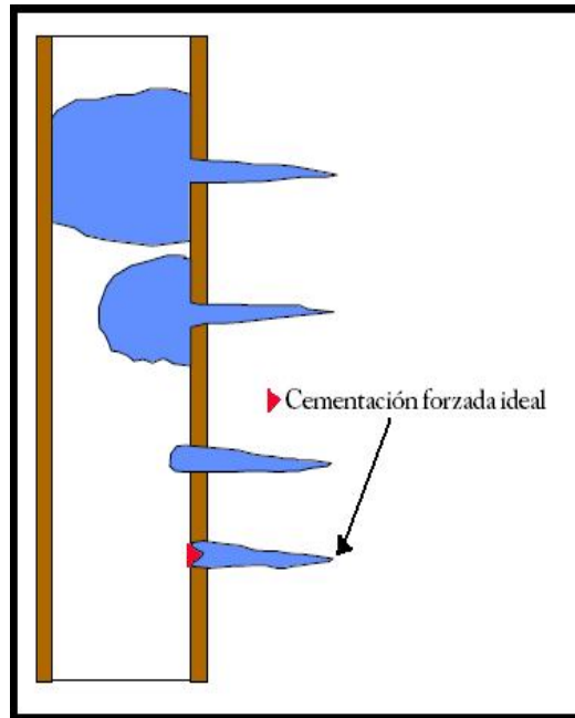
Figura 4.17 Cementación forzada ideal, dejando la menor cantidad de cemento dentro de la TR.
