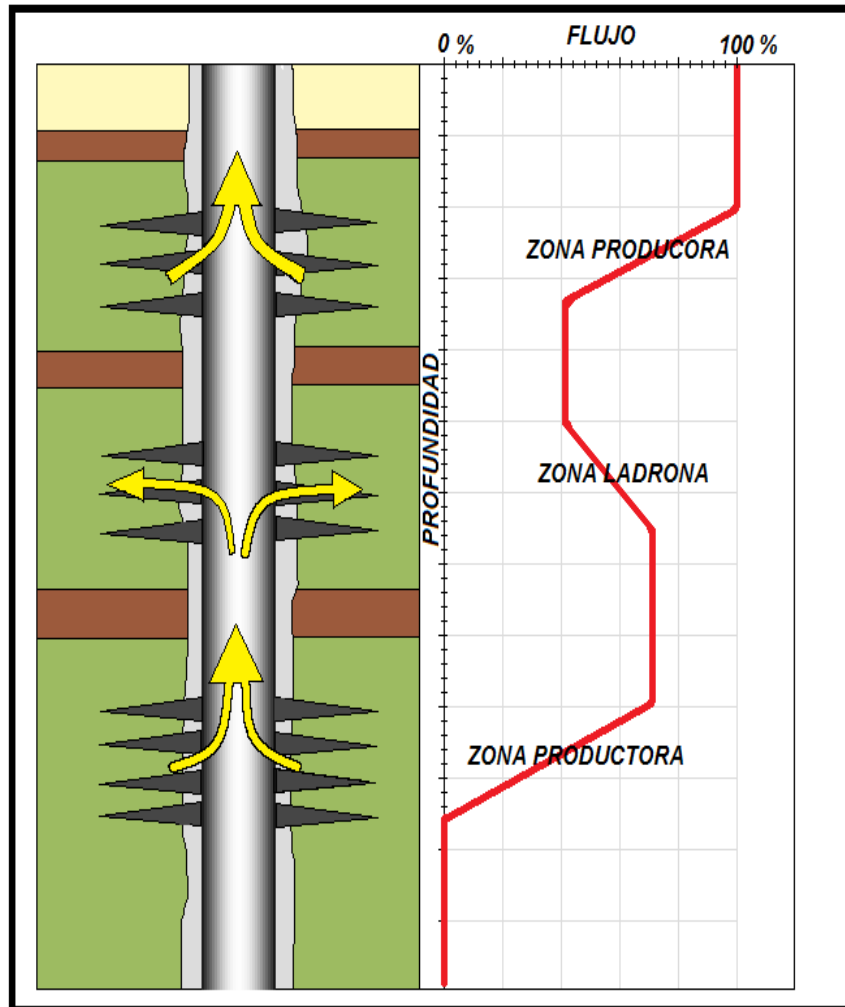
Figura 3.22 Identificación de zonas ladronas y productoras utilizando el medidor de flujo (molinete).
