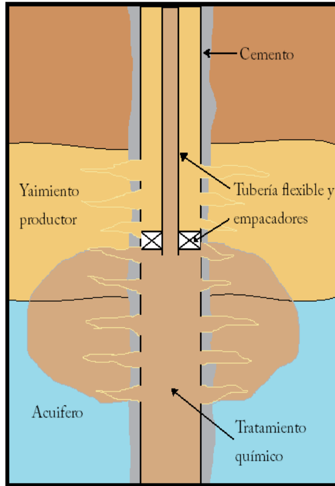
Figura 4.26 Colocación de tratamiento químico con ayuda de tubería flexible y empacador recuperable.
