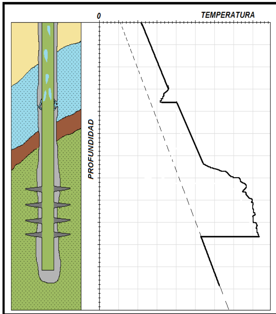
Figura 3.21 Anomalía fría causada por la entrada de líquidos en un intervalo superior.
