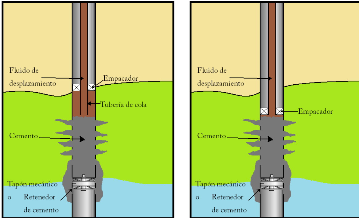
Figura 4.24 Cementación forzada utilizando empacadores, con cola de tubería y sin cola de tubería.
