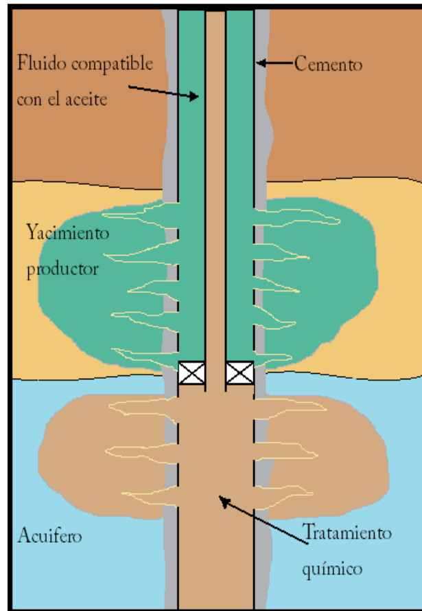
Figura 4.27 Colocación del tratamiento químico utilizando tubería flexible y doble inyección.
