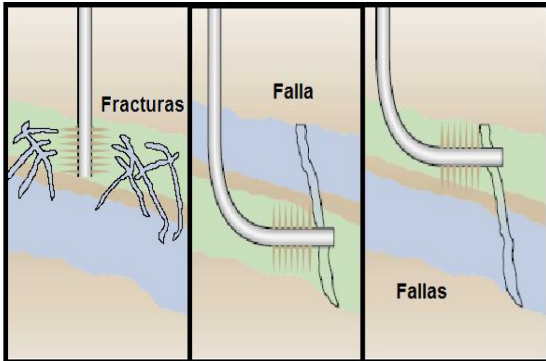
Figura 2.11 Fracturas o fallas en una capa de agua.
