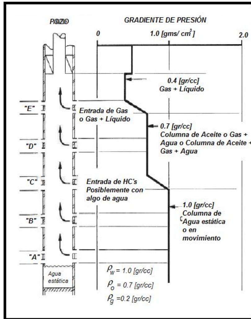
Figura 3.26 Perfil de densidad de flujo indicando entradas de fluidos.
