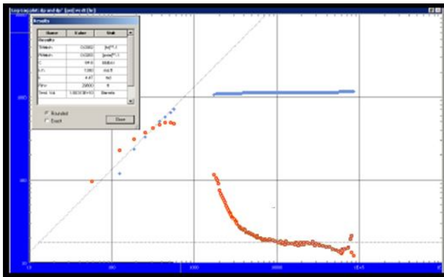
Figura 5.4 Prueba presión producción para el pozo Otumba-11.
