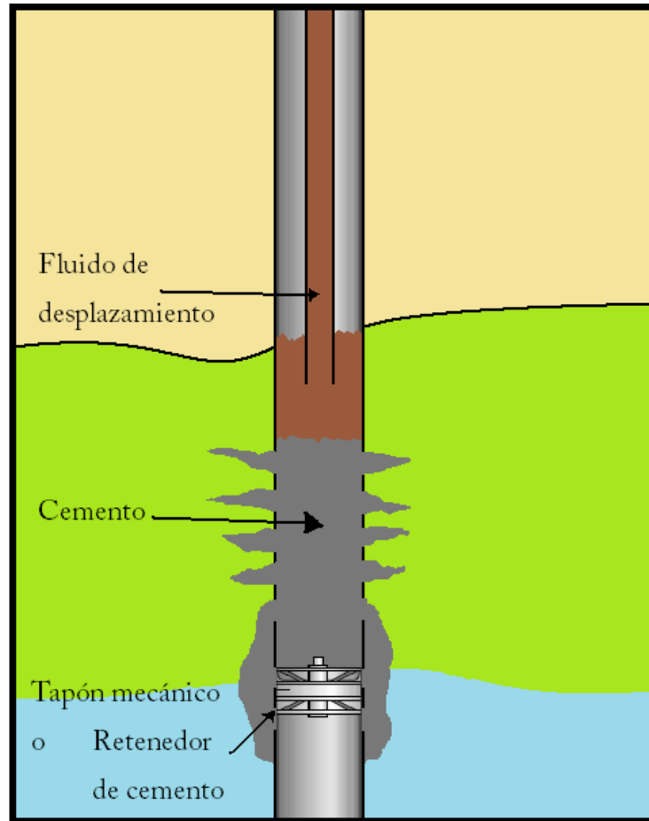
Figura 4.23 Cementación forzada sin utilizar empacador.
