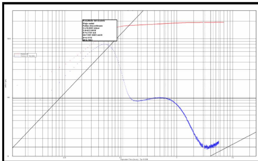
Figura 5.31 Prueba presión producción para el pozo Puma-13.
