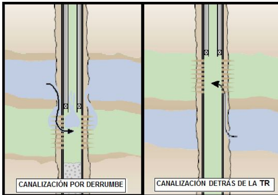
Figura 2.5 Canalización detrás de la TR causada por una mala cementación.
