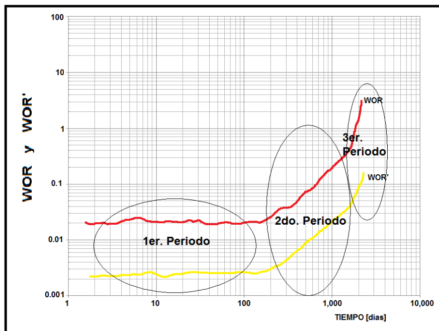
Figura 3.14 Tendencia de la WOR y WOR' para identificar digitalización de agua hacia el pozo, con tres periodos característicos.
