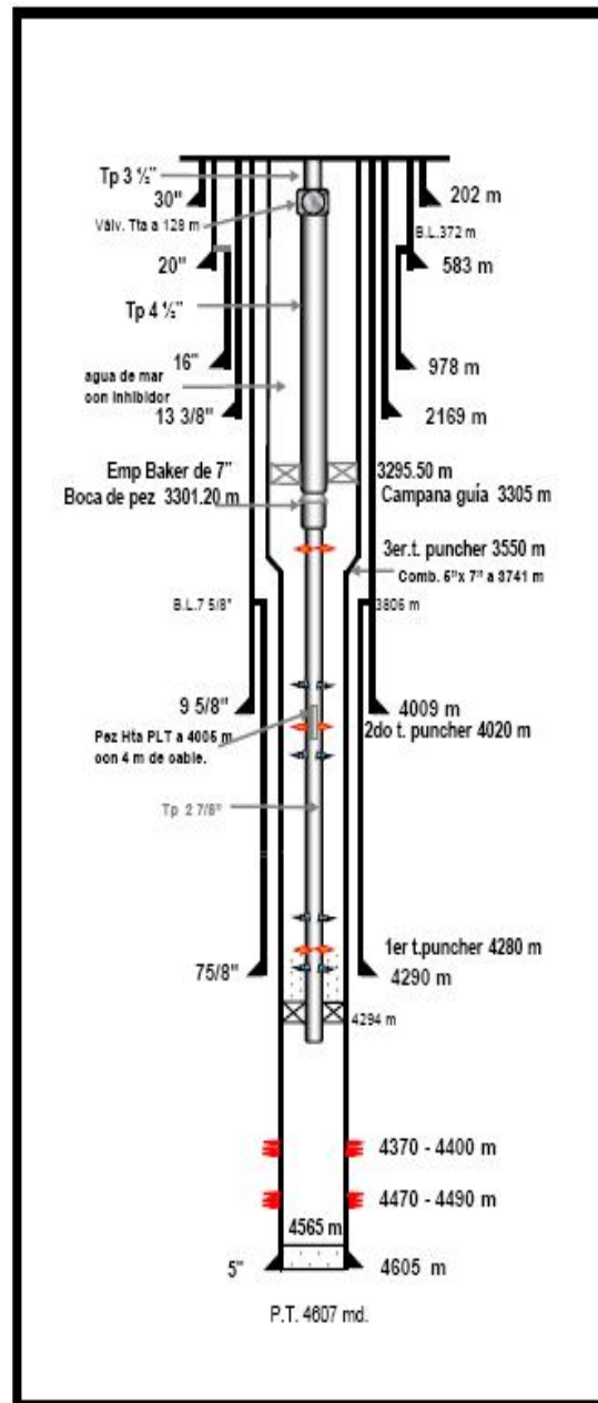
Figura 5.25 Estado mecánico del pozo Puma-1.
