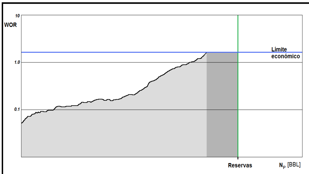
Figura 3. 4 Gráfica de WOR vs. N_p , llegando al límite económico antes de recuperar el volumen total contemplado en la reserva.
