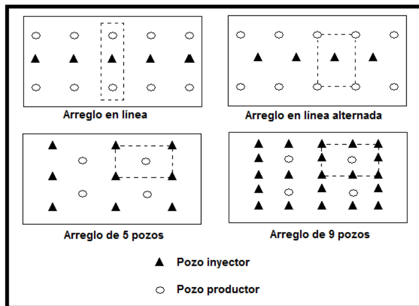
Figura 2.6 Arreglo de pozos inyector y productores.
