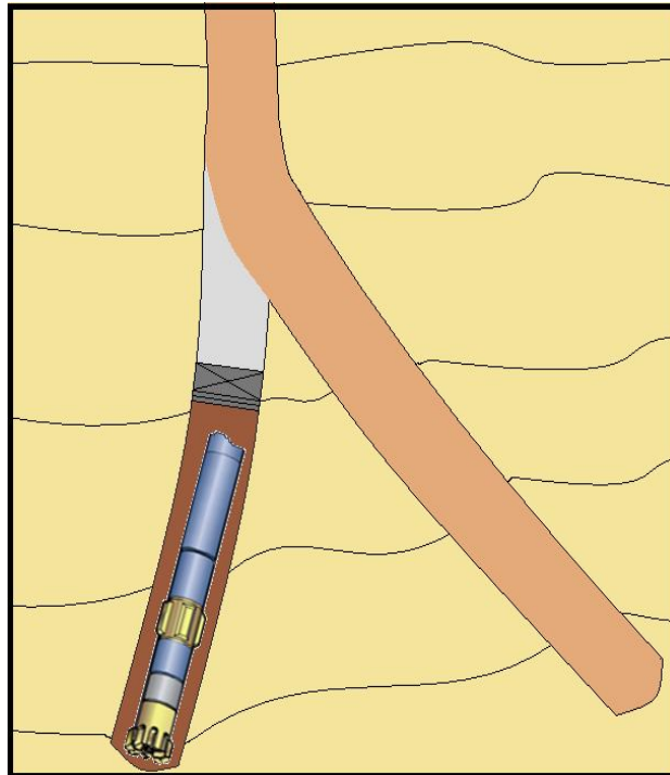
Figura 4.5 Tapón de desvío colocado para esquivar un pescado.
