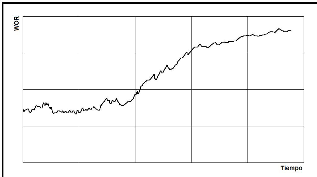
Figura 3.3 Gráfica de la WOR contra el tiempo, que muestre un incremento de la WOR en corto tiempo.
