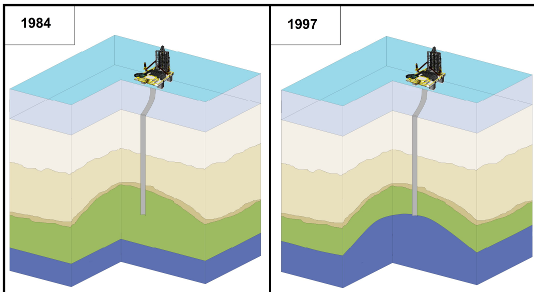
Figura 3.17 Identificación de la fuente de agua mediante la sísmica 4D.
