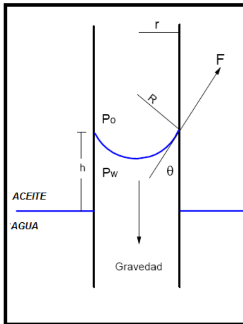
Figura 1.12 Diagrama de fuerzas presentes en la presión capilar.
