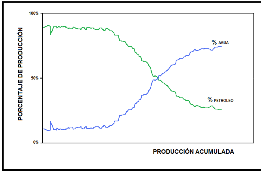
Figura 3.10 Gráfica con los porcentajes de producción tanto de agua como de aceite.
