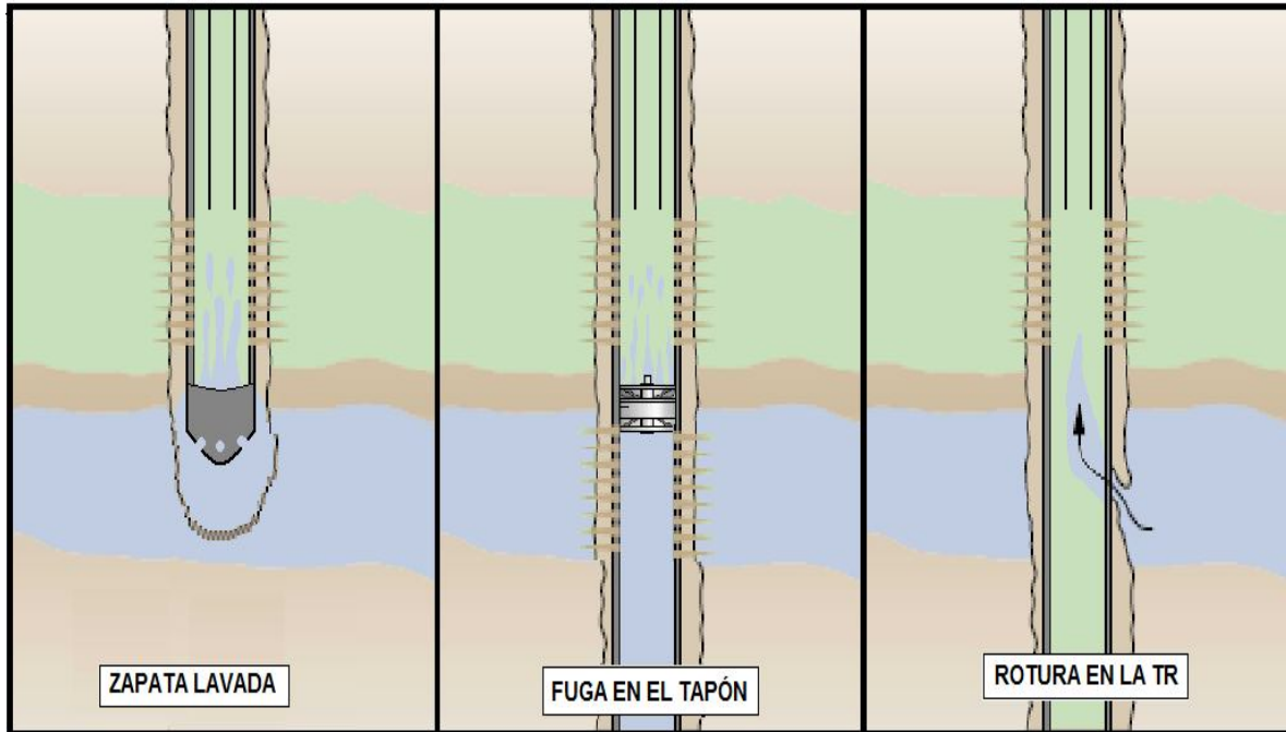
Figura 2.4 Entrada de agua causada por fugas.
