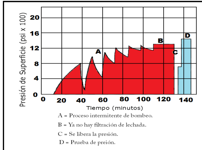
Figura 4.22 Diagrama para el proceso por el cual se bombea una lechada de forma intermitente.
