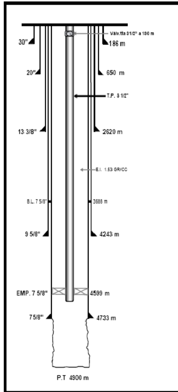
Figura 5.20 Estado mecánico del pozo Unam-31.
