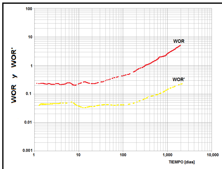
Figura 3.12 Tendencia de la WOR y WOR' para el comportamiento normal de un pozo.
