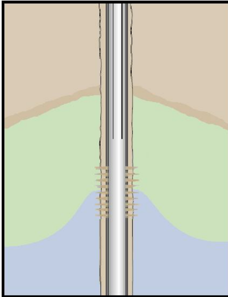
Figura 2. 13 Conificación de agua.
