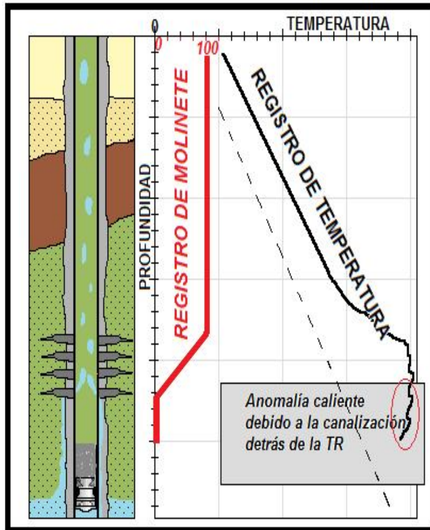
Figura 3.19 Identificación de canalización utilizando el registro de temperatura.
