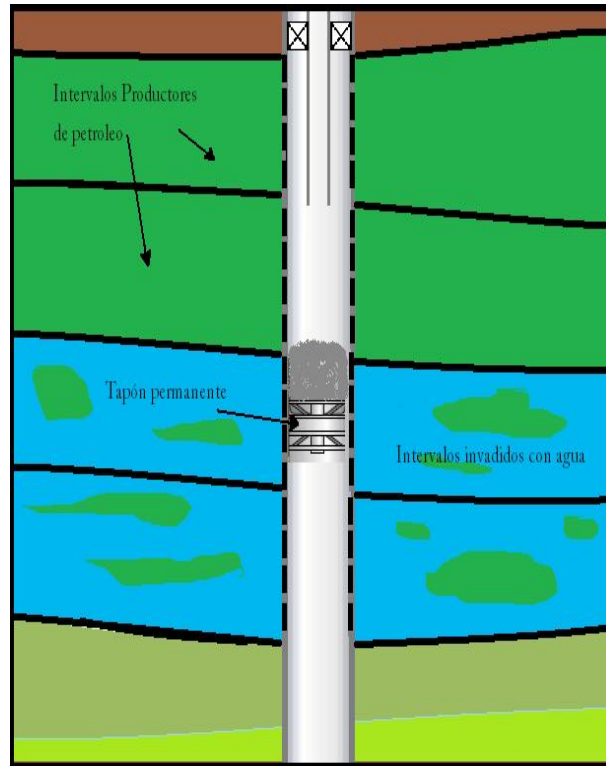
Figura 4.3 Colocación de un tapón mecánico permanente, acompañado de cemento, para aislar una zona invadida de agua.
