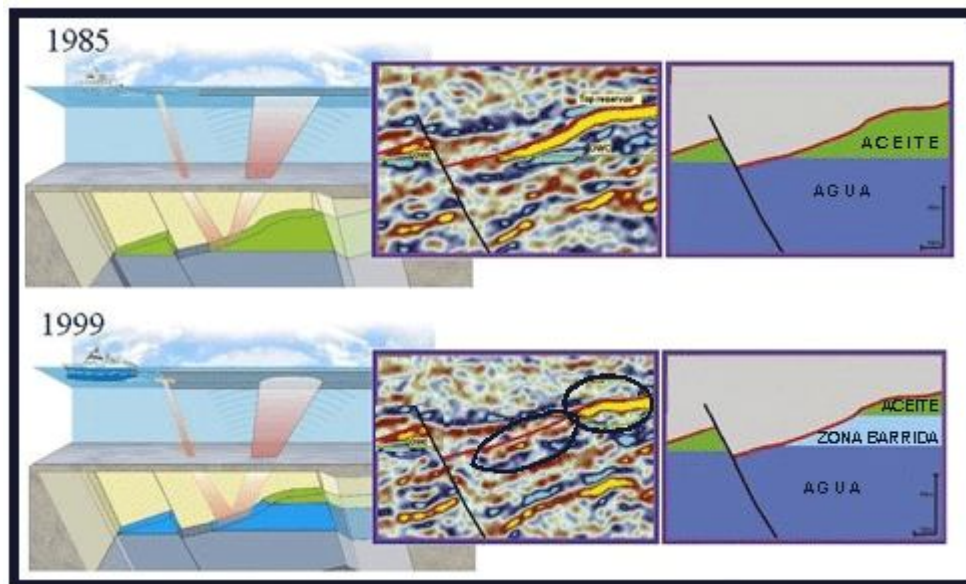
Figura 3.16 Monitoreo del movimiento de los fluidos mediante la sísmica de lapso 4D.
