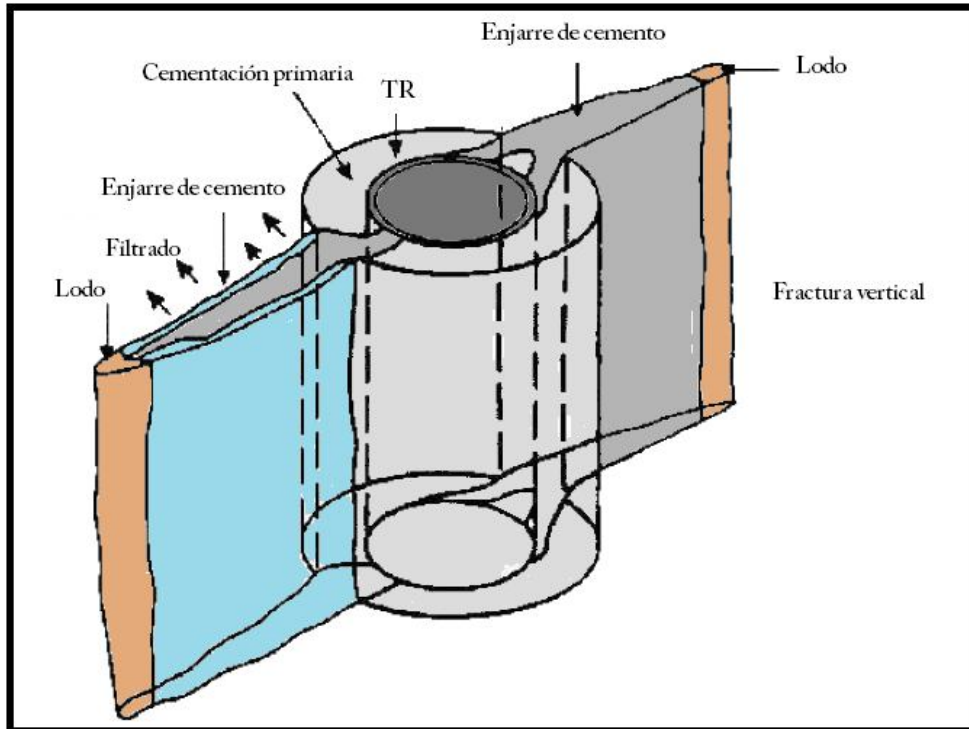
4.18 Fracturas verticales causadas por cementación forzada a alta presión.
