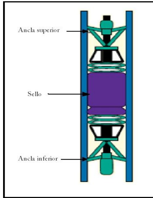
Figura 4.1 Esquema general de un Tapón mecánico
