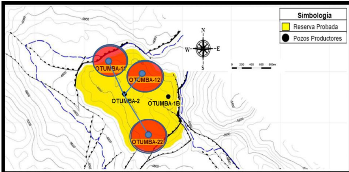
Figura 5.1 Configuración estructural del campo Otumba.
