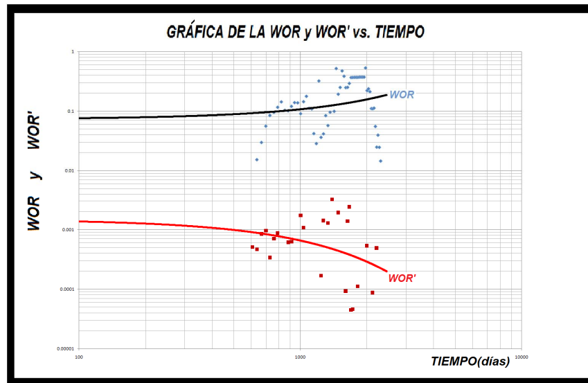
Figura 5.28 Gráfica de la WOR y WOR' vs. tiempo para el pozo Puma-1.
