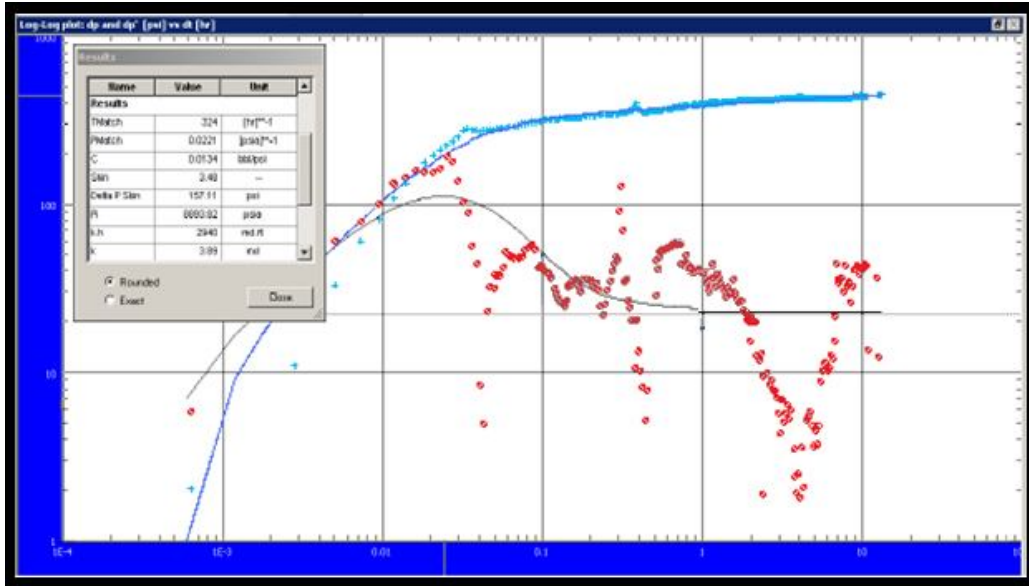
Figura 5.8 Prueba presión producción para el pozo Otumba-12.
