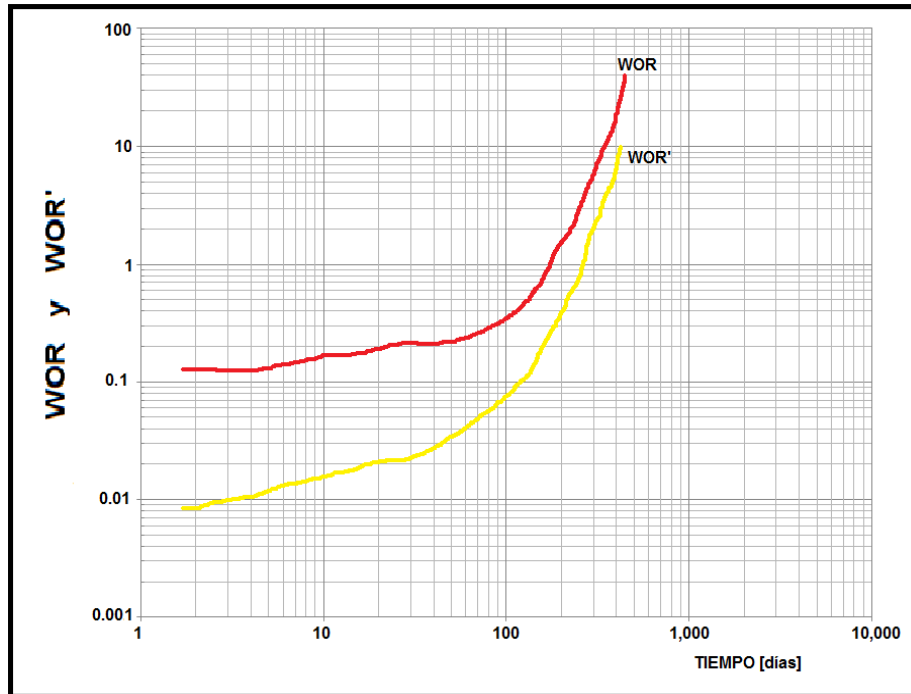
Figura 3.13 Tendencia de la WOR y WOR' para identificar problemas de canalización y roturas en la TR.
