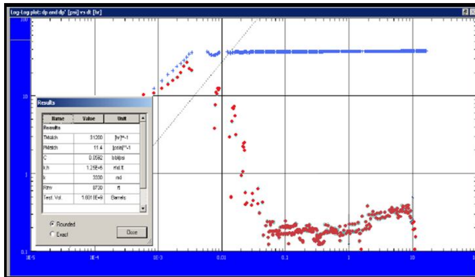
Figura 5.18 Prueba de presión producción para el pozo Unam-11.
