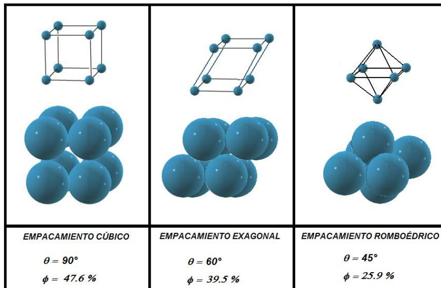
Figura 1.5 Arreglos geométricos del empaque de granos.
