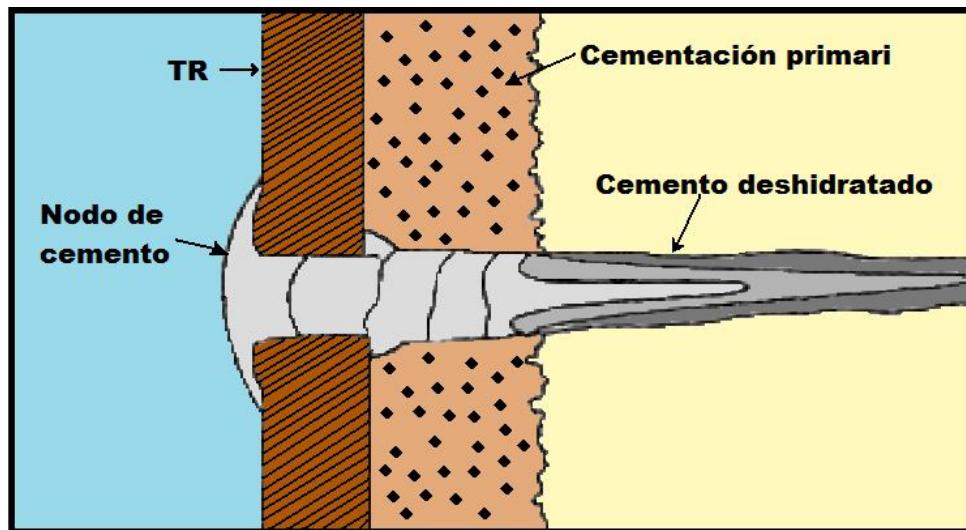
Figura 4.21 Cementación forzada con bombeo intermitente.
