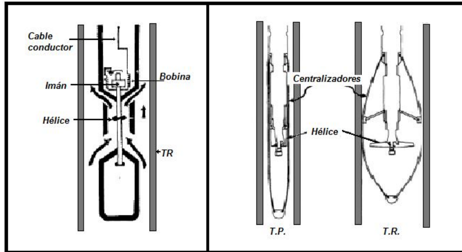
Figura 3.23 Medidores de flujo continuo de diámetro reducido y diámetro total.
