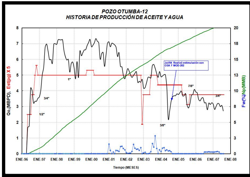
Figura 5.7 Historia de producción de aceite y agua del pozo Otumba-12.
