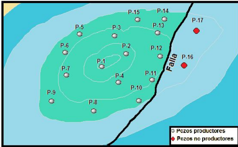
Figura 3.2 Mapa estructural de un anticlinal con una falla que conecta un acuífero con pozos cercanos a ella, que tienen producción de agua.
