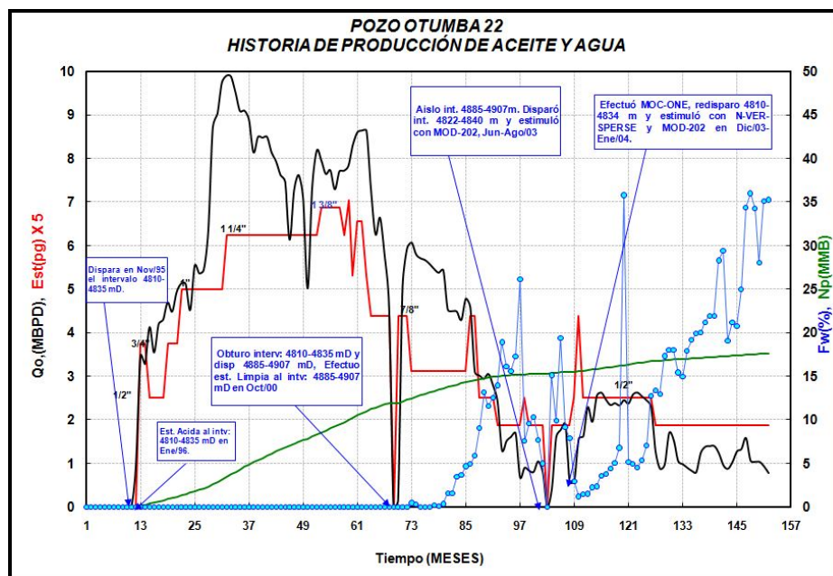
Figura 5.11 Historia de producción de aceite y agua para el pozo Otumba-22.
