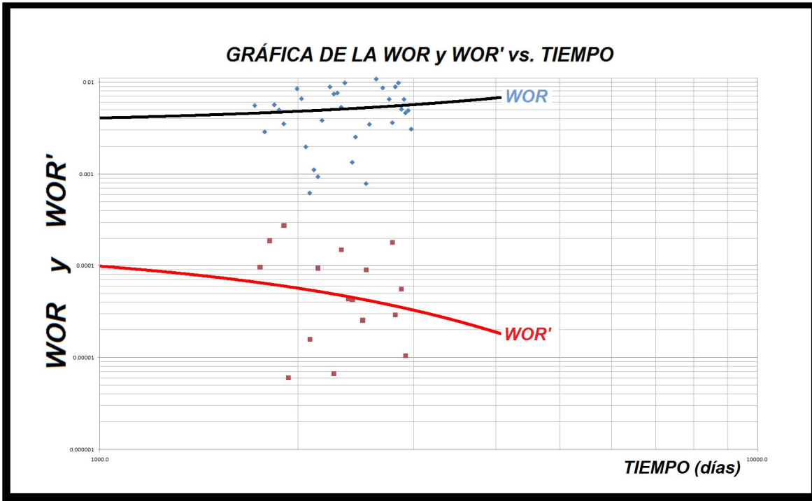
Figura 5.9 Gráfica de la WOR y WOR' vs. tiempo para el pozo Otumba-12.
