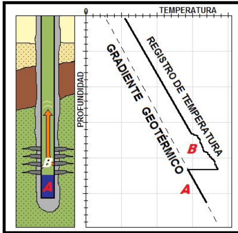
Figura 3.18 Comportamiento del registro de temperatura ante la entrada de líquidos.
