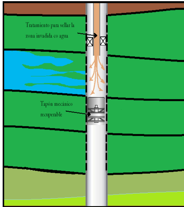
Figura 4.2 Uso de tapón recuperable para la aplicación de un tratamiento de control de agua en yacimientos estratificados.
