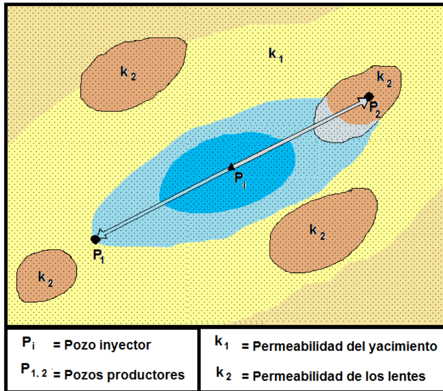
Figura 2.7 Mapa de iso-propiedades.
