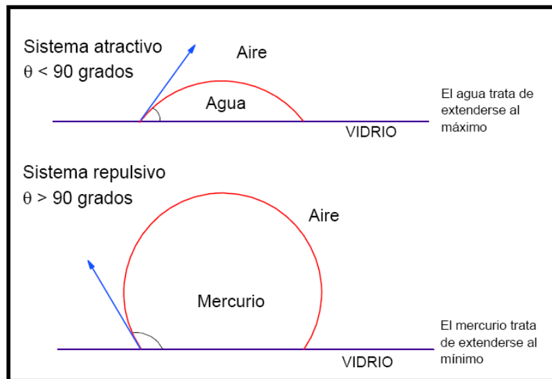
Figura 1.10 Ángulos de contacto para fluidos mojantes y no mojantes.
