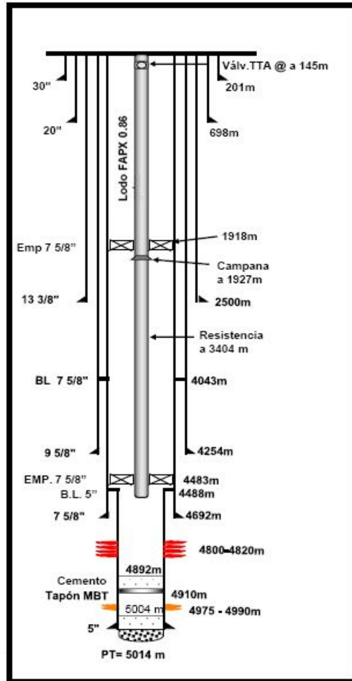
Figura 5.6 Estado mecánico del pozo Otumba-12.
