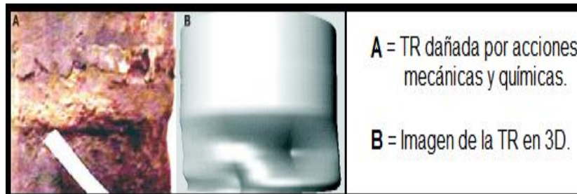
Figuras 2.3 Fugas en TR causadas por acciones mecánicas y químicas.
