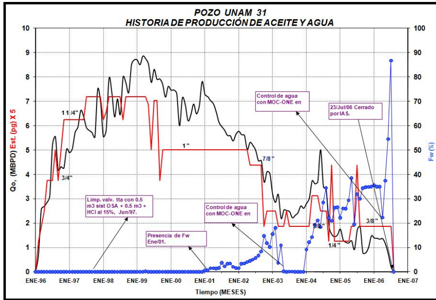
Figura 5.21 Historia de producción de aceite y agua para el pozo Unam-31.
