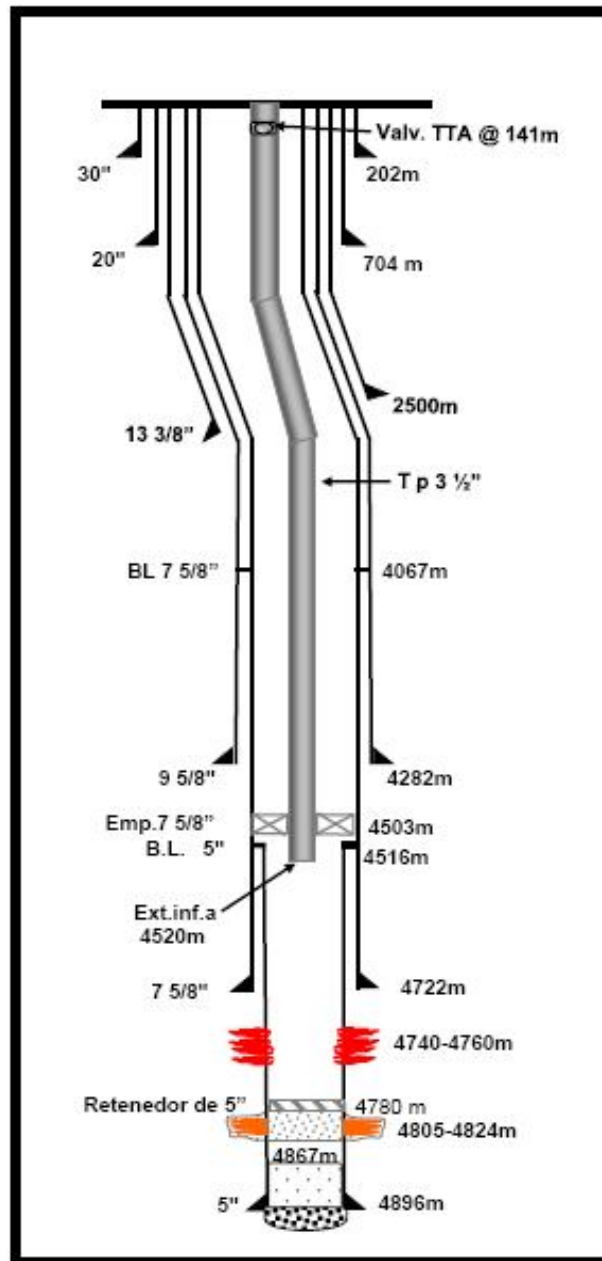
Figura 5.2 Estado mecánico del pozo Otumba-11.
