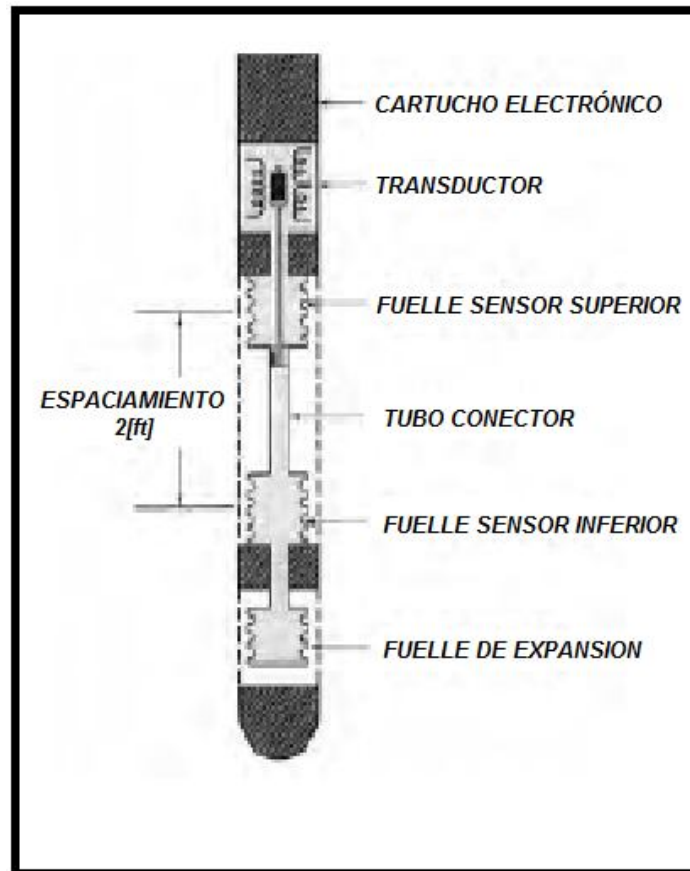
Figura 3.25 Diagrama del gradiomanómetro.
