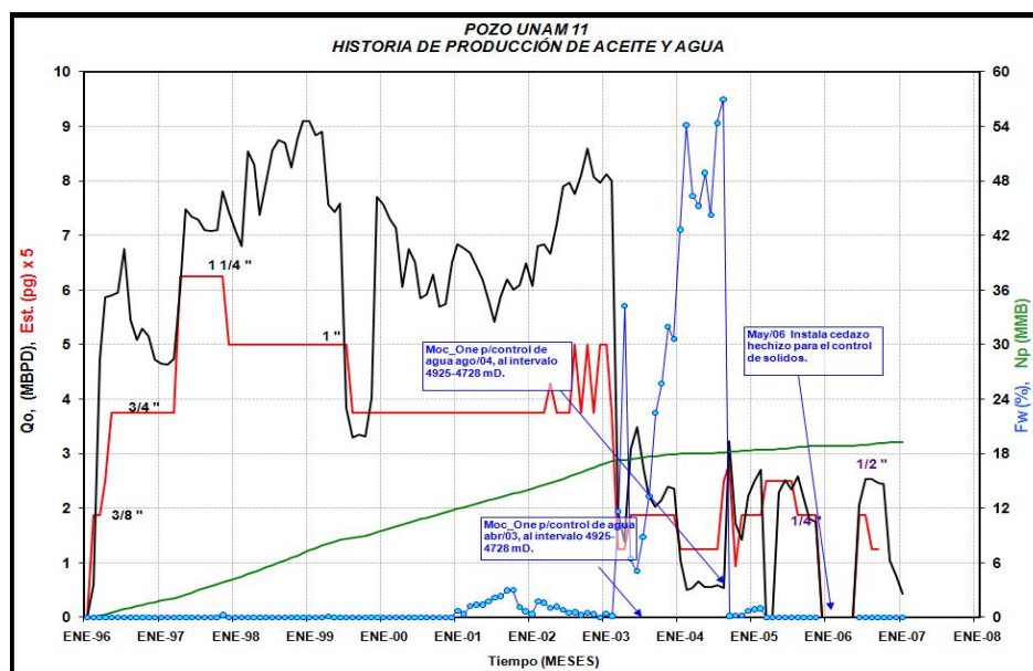
Figura 5.17 Historia de producción de aceite y agua para el pozo Unam-11.
