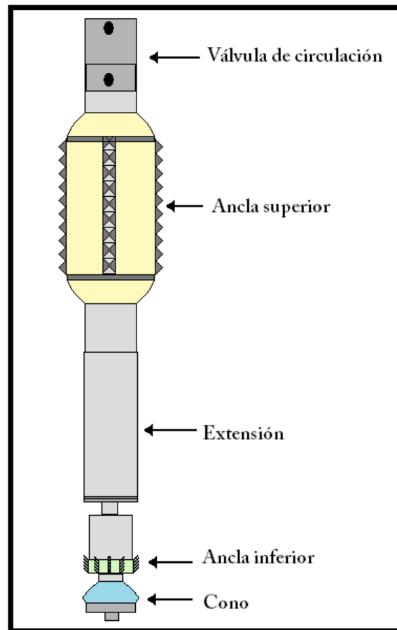
Figura 4.12 Principales elementos en la herramienta utilizada para colocar un parche de TR.
