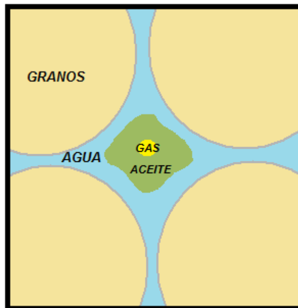
Figura 1.9 Distribución de los fluidos en el espacio poroso de una roca.
