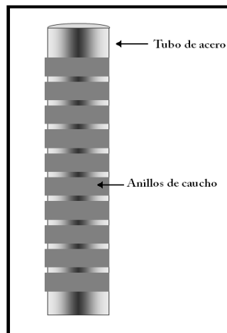
Figura 4.14 Parche de TR con anillos de caucho.
