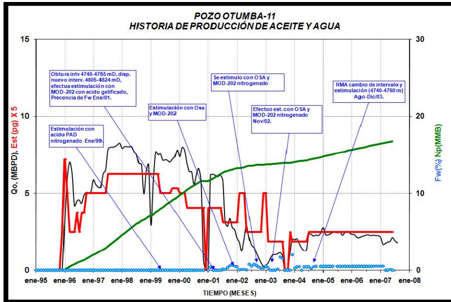
Figura 5.3 Historia de producción de aceite y agua para el pozo Otumba-11.
