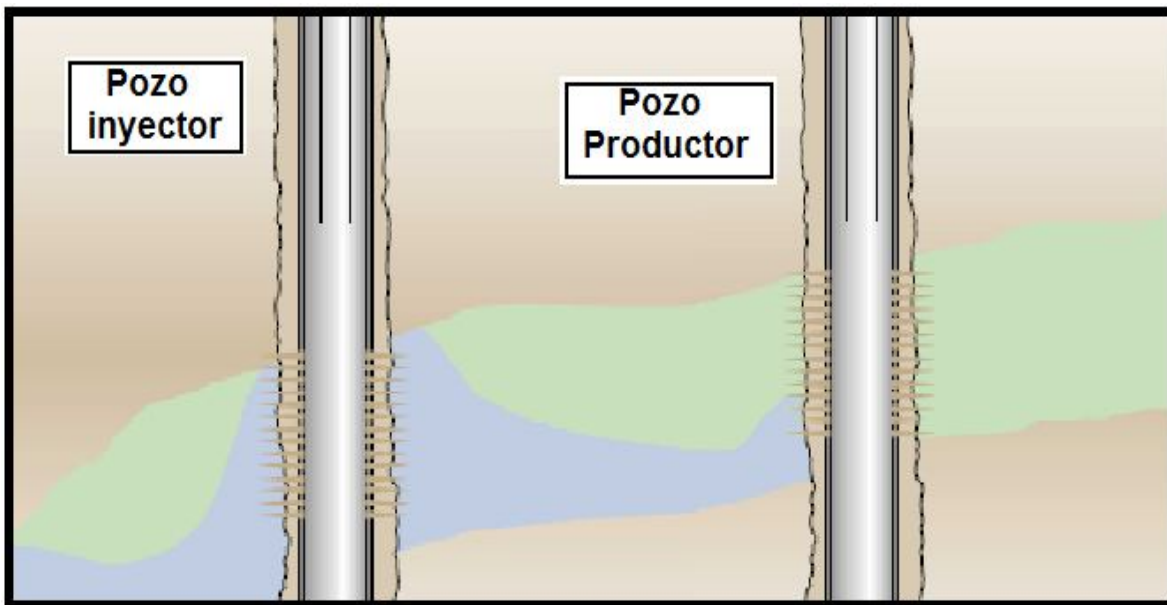
Figura 2.15 Segregación gravitacional.
