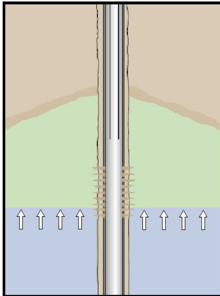
Figura 2.14 Contacto agua-aceite dinámico.
