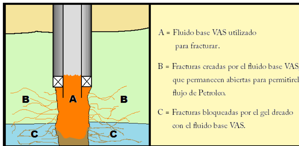
Figura 4.25 Fluido base VAS utilizado para fracturar.
