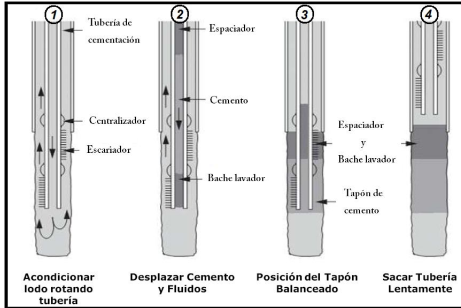
Figura 4.9 Tapón balanceado.
