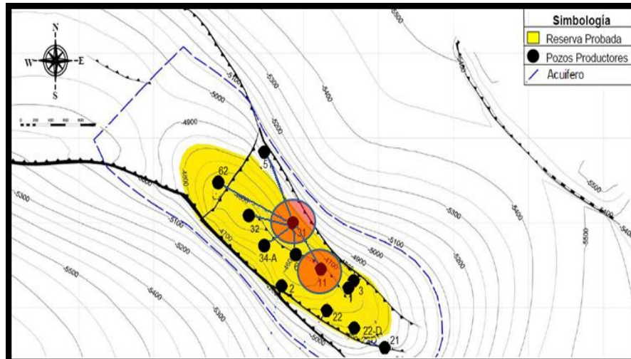
Figura 5.15 Configuración estructural del campo Unam.
