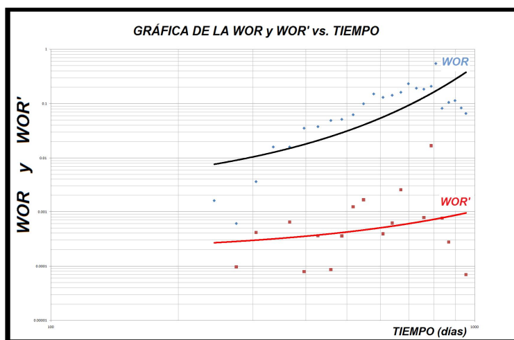
Figura 5.13 Gráfica de la WOR y WOR' vs. tiempo para el pozo Otumba-22. Periodo de producción de enero de 2001 a junio de 2003 para la producción del intervalo 4885-4907 m.
