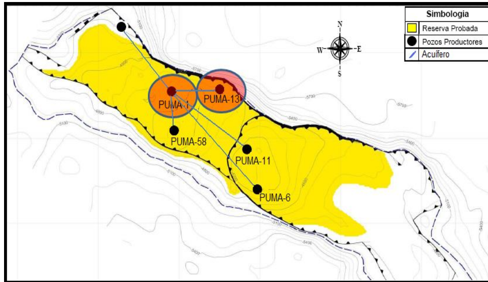
Figura 5.24 Configuración estructural del campo Puma.
