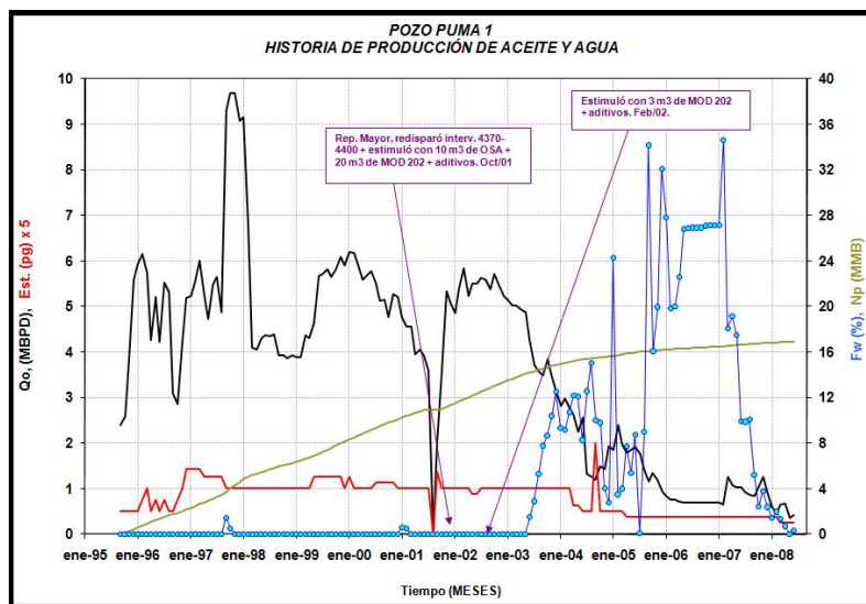
Figura 5.26 Historia de producción de aceite y agua para el pozo Puma-1.
