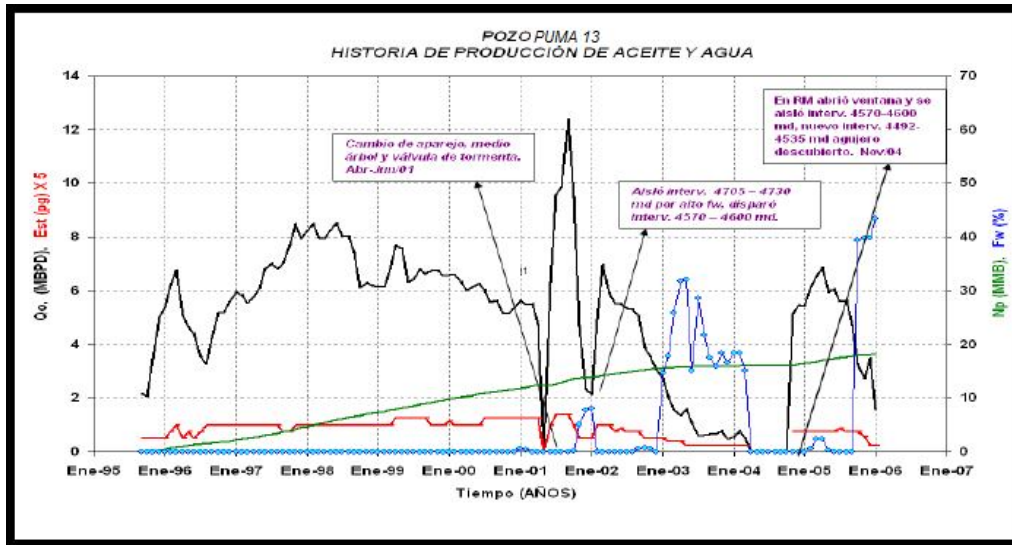
Figura 5.30 Historia de producción de aceite y agua para el pozo Puma-13.
