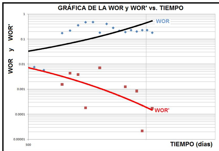
Figura 5.32 Gráfica de la WOR y WOR' para el pozo Puma-13.
