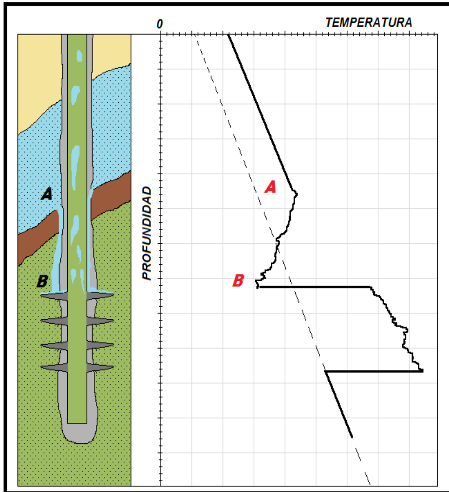
Figura 3.20 Canalización de un fluido frío hacia la zona disparada, identificada con ayuda del registro de temperatura.
