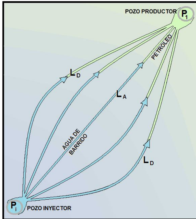
Figura 2.2 Líneas de flujo que representan el flujo de agua desde el pozo inyector hasta el pozo productor.
