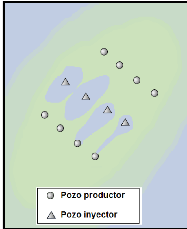
Figura 2.12 Yacimiento que presenta barrido areal deficiente.
