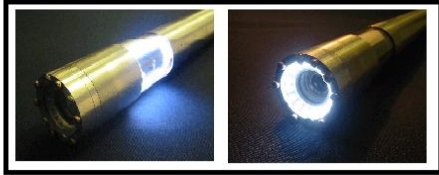
Figura 3.34 Sistema de iluminación para el Borehole Video.
