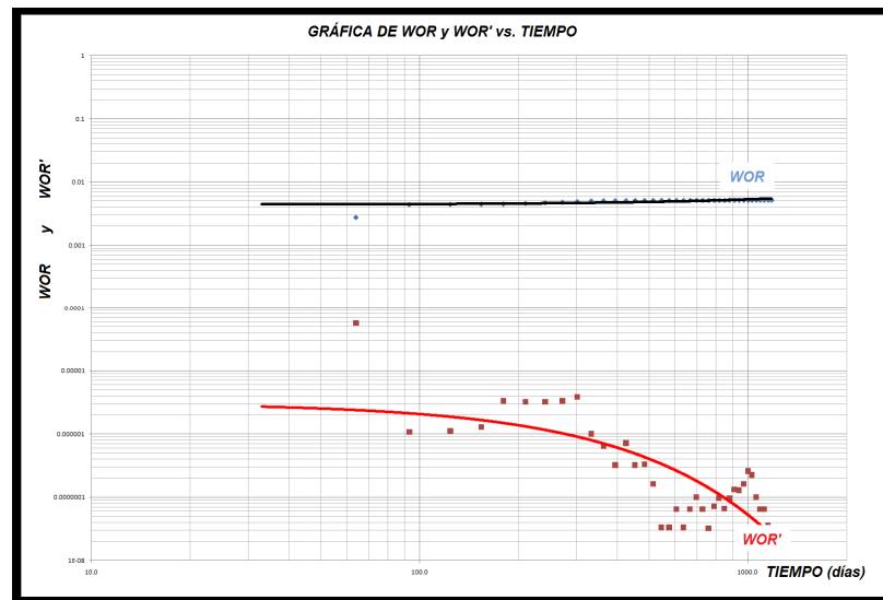
Figura 5.5 Gráfica de la WOR y WOR' vs. tiempo para el pozo Otumba-11.
