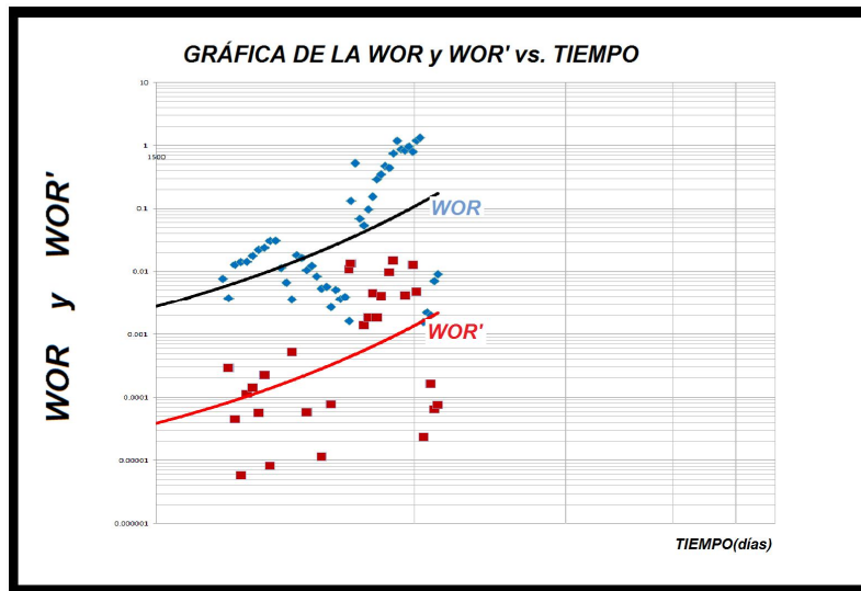
Figura 5.19 Gráfica de la WOR y WOR' vs. tiempo para el pozo Unam-11.
