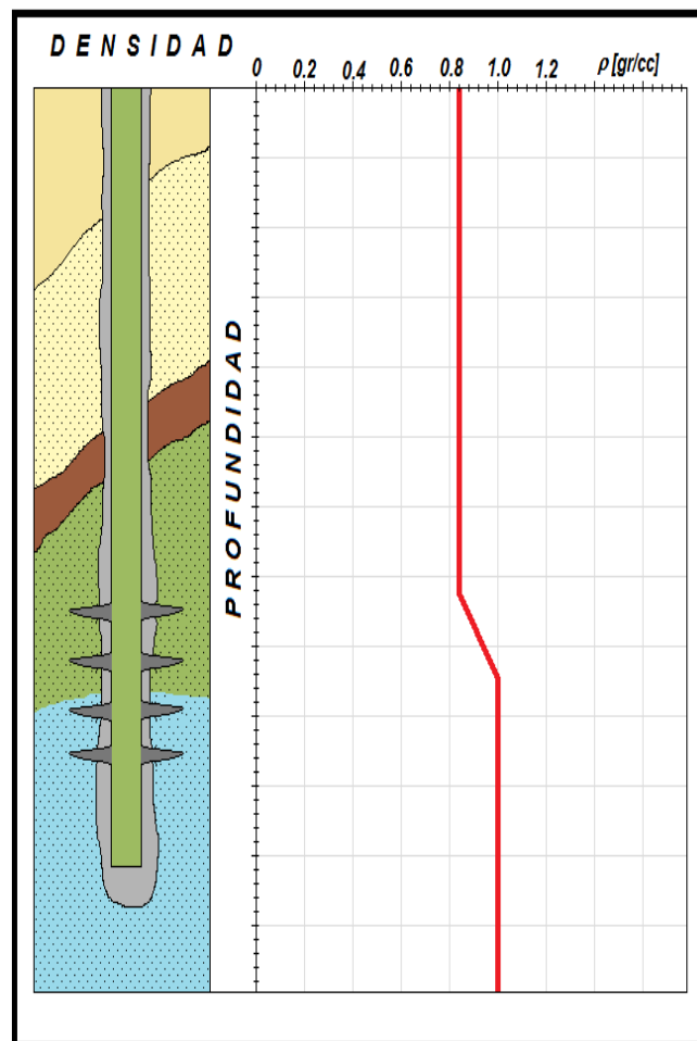
Figura 3.27 Empleo del gradimanómetro para identificar puntos de entrada de agua.
