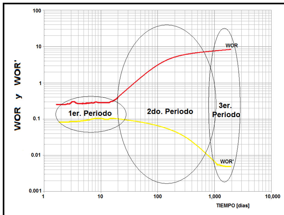
Figura 3.15 Tendencia de la WOR y WOR' para identificar conificación en el pozos productores con tres periodos característicos.
