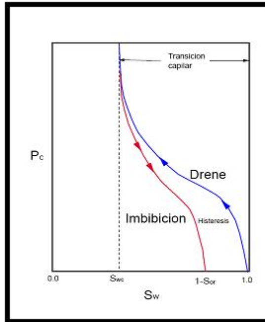
Figura 1.13 Histéresis de la curva de presión capilar.
