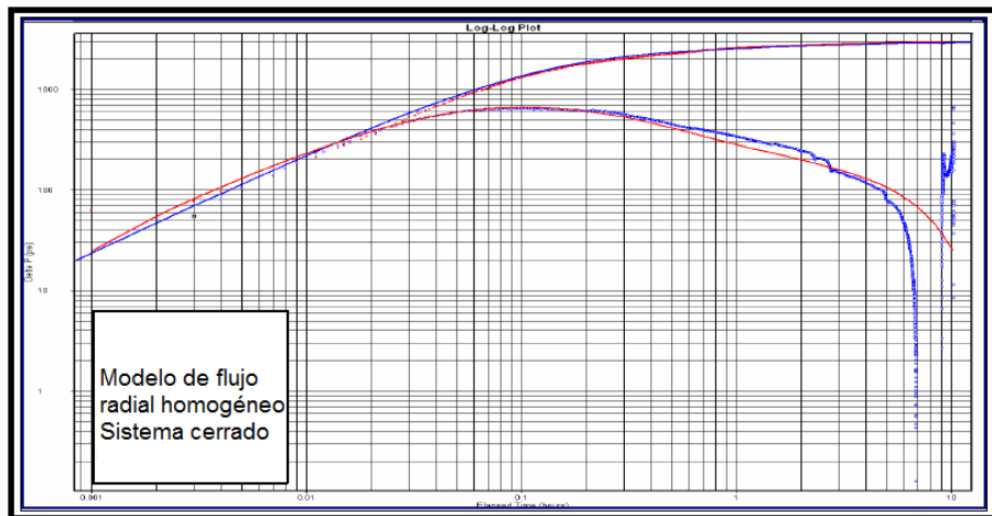
Figura 5.27 Prueba presión producción para el pozo Puma-1.
