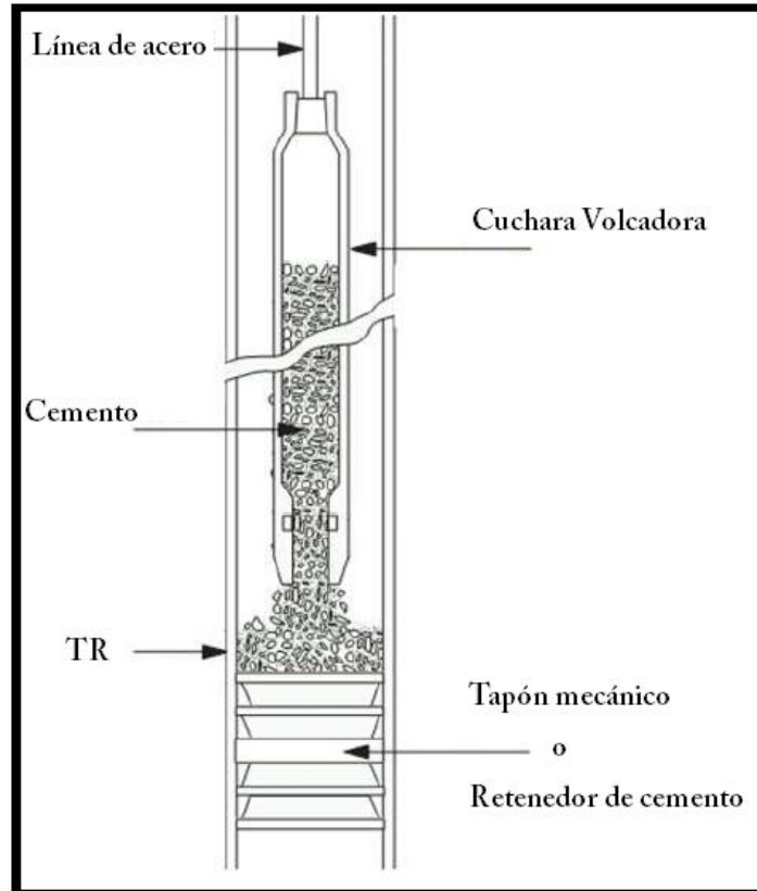
Figura 4.10 Tapón de cemento con cuchara Volcadora.
