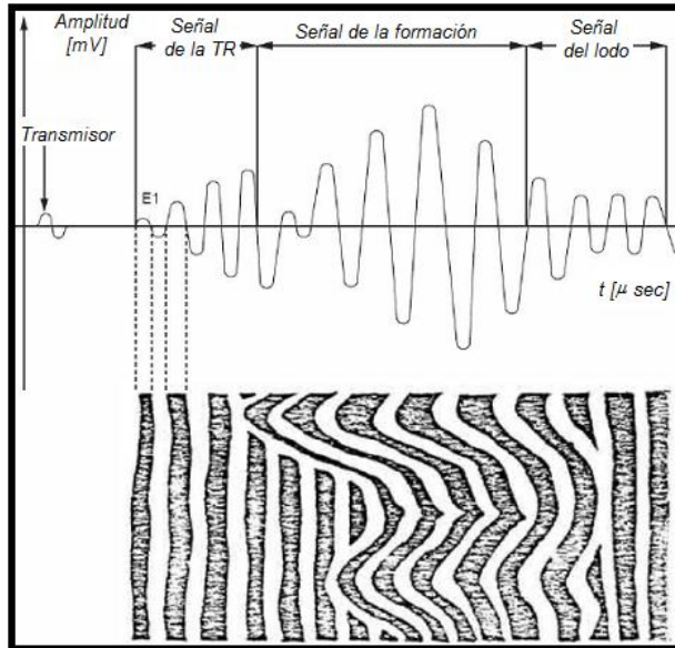
Figura 3.32 Señales recibidas por el VDL.
