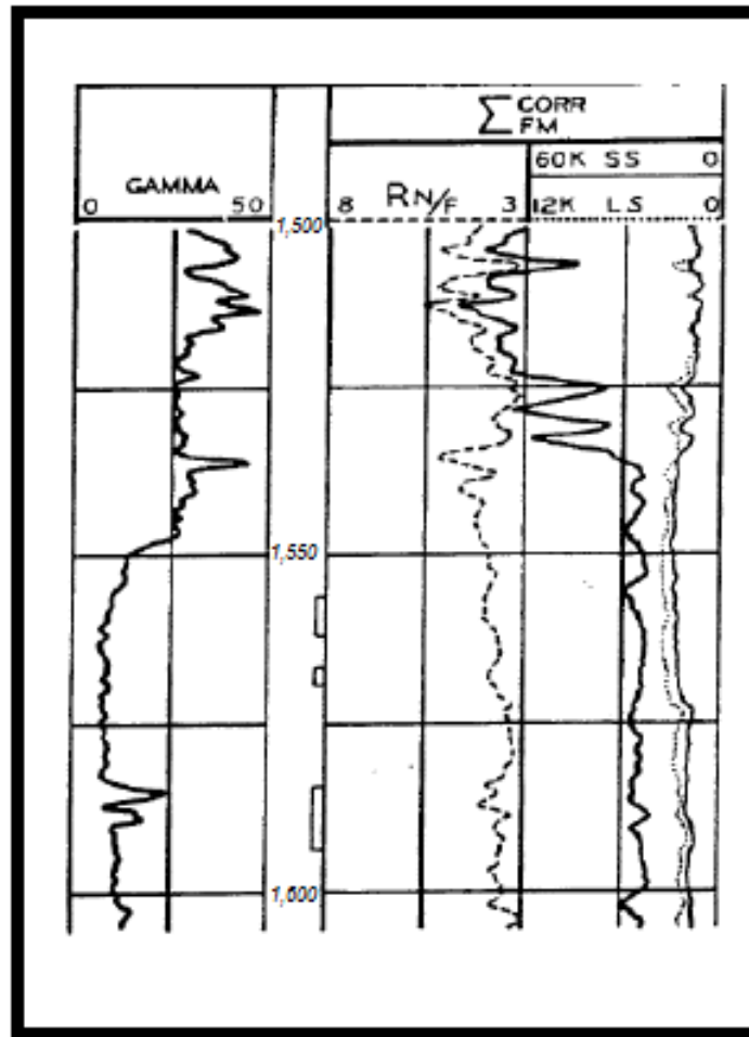
Figura 3.29 Registro de neutrón pulsado.
