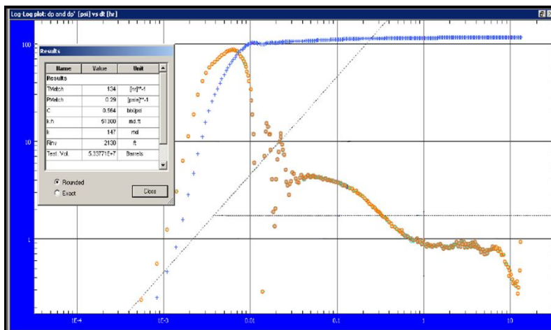
Figura 5.22 Prueba de presión-producción para el pozo Unam-31.
