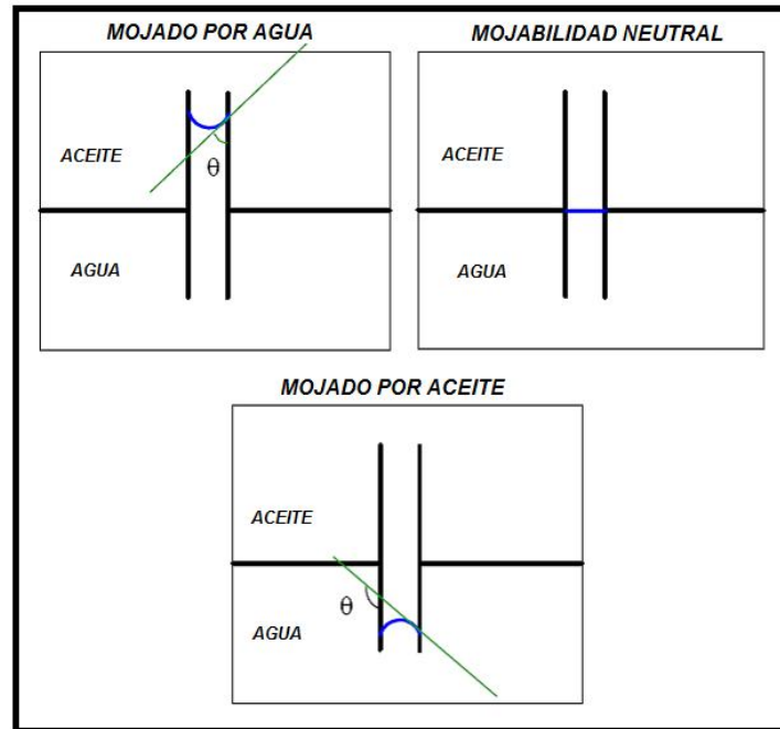
Figura 1.11 Tipos de mojabilidad.
