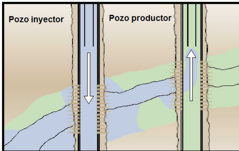
Figura 2.9 Digitalización en yacimiento estratificado sin barreras de flujo.
