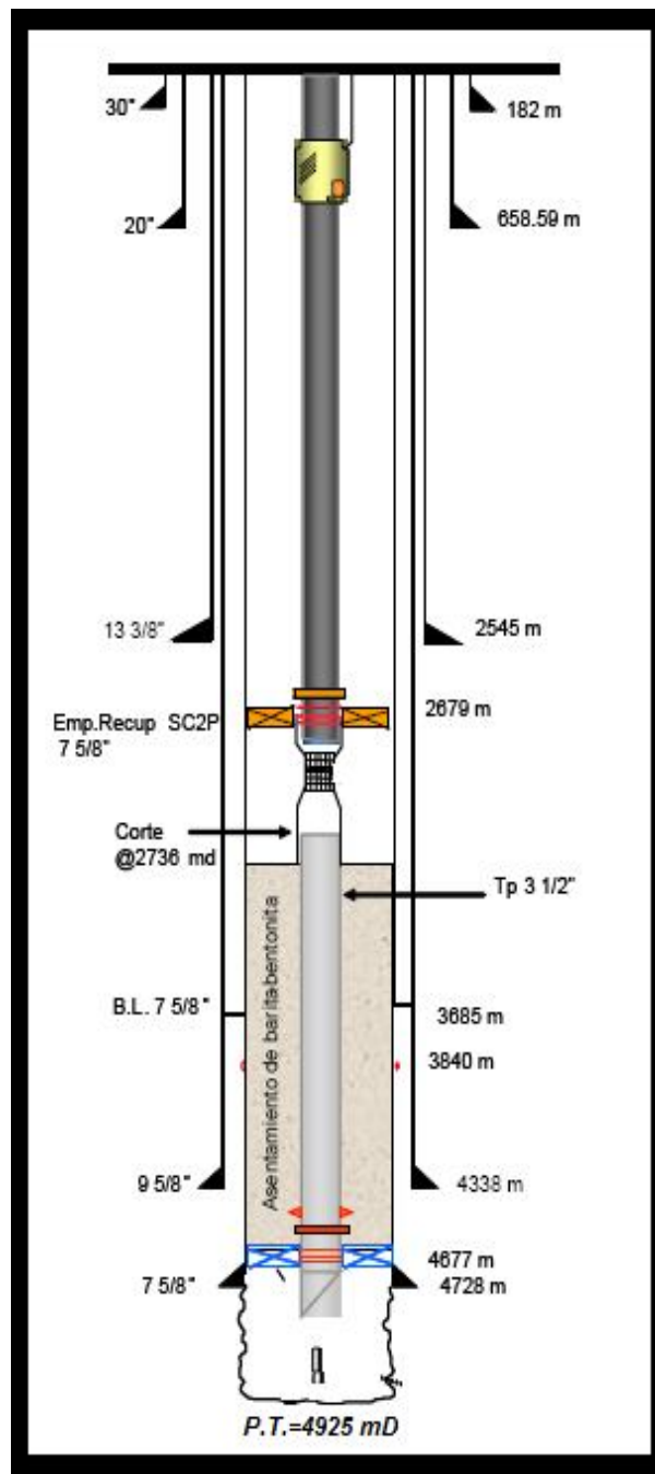
Figura 5.16 Estado mecánico del pozo Unam-11.
