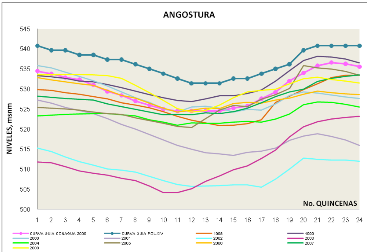
Figura 4.4 Elevaciones simuladas con el registro histórico y política XIV. Presa Angostura.
