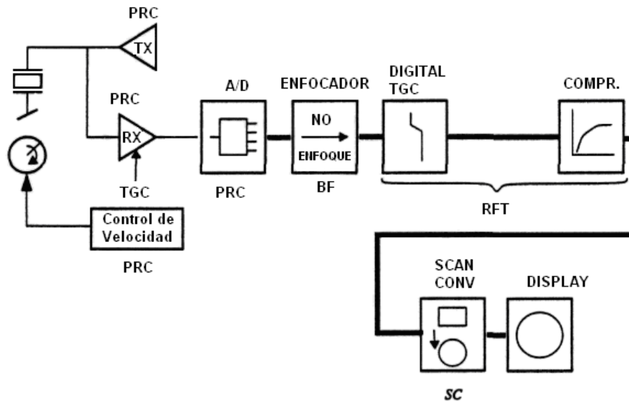
Figura 2.32 Flujo de Datos
