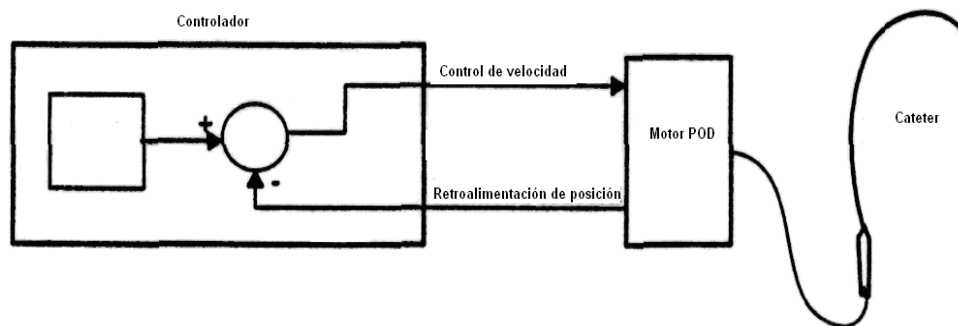
Figura 2.30 Controlador de motor
