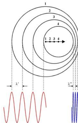
Figura 1.18 Fuente en movimiento.
