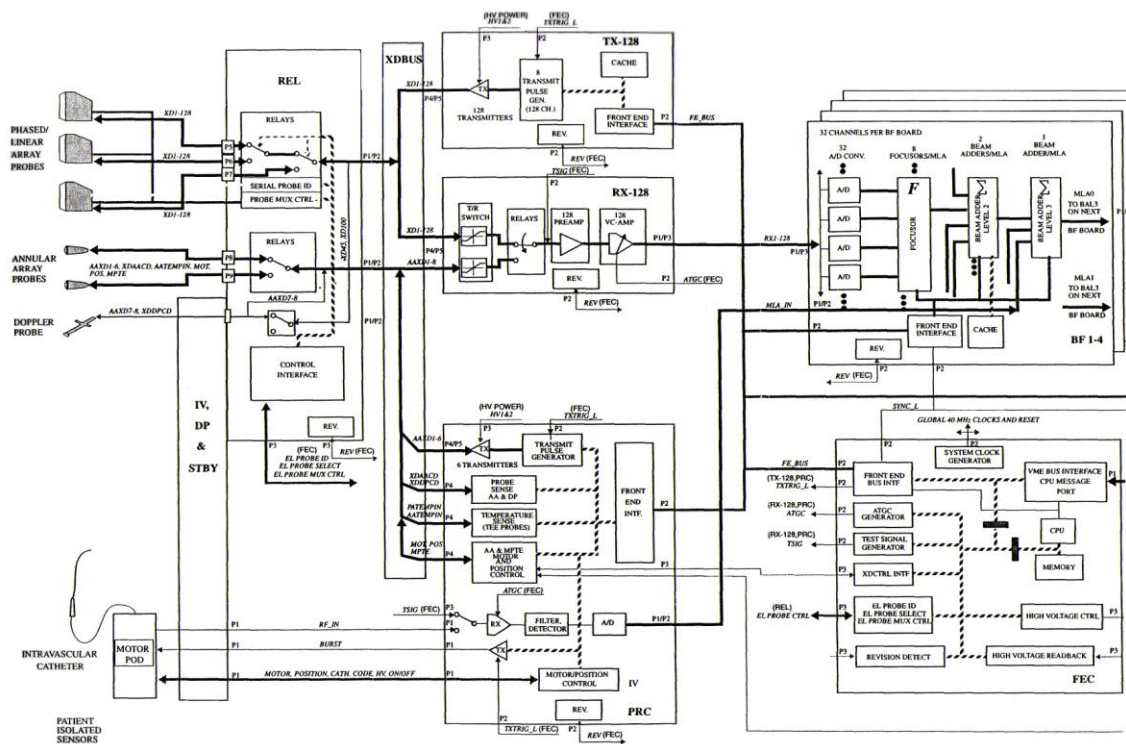
Figura 3.3 Diagrama de bloque extremo delantero
