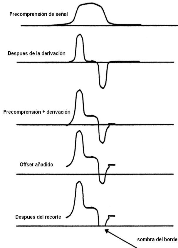
Figura 2.37 Realce del borde
