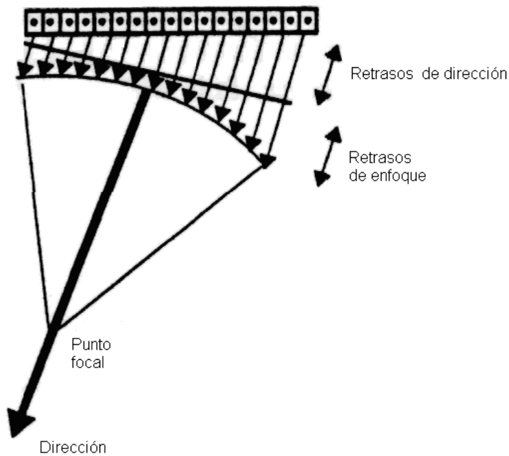
Figura 2.7 Retraso de enfoques.
