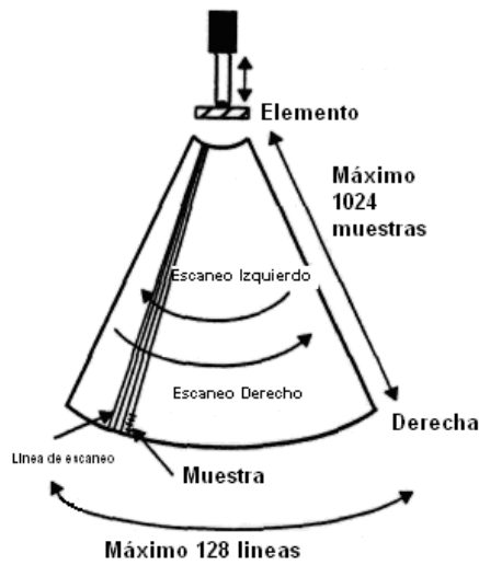
Figura 2.22 Pantalla de un sector del tejido 2D.
