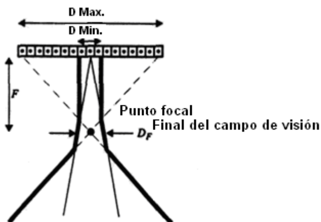
Figura 2.12 Ancho del rayo, apertura variable.
