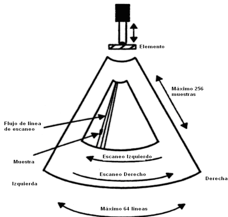
Figura 2.24 Pantalla del Sector del flujo en 2D
