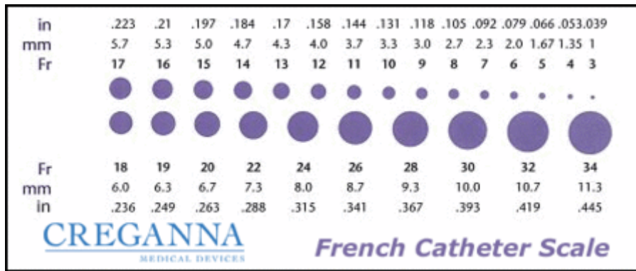
Figura 2.28 Escala de catéteres French
