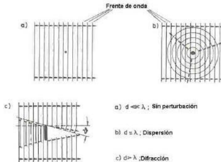
Figura 1.8 Dispersión y difracción de ondas.
