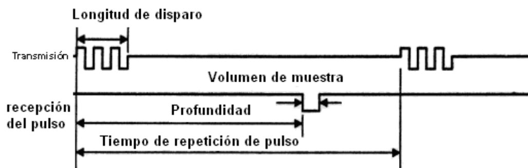
Figura 2.39 Pulsado de onda Doppler
