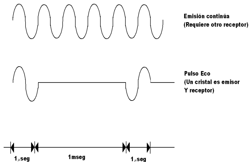
Figura 1.13 Formas de emisión continua y pulsada de la onda ultrasónica.
