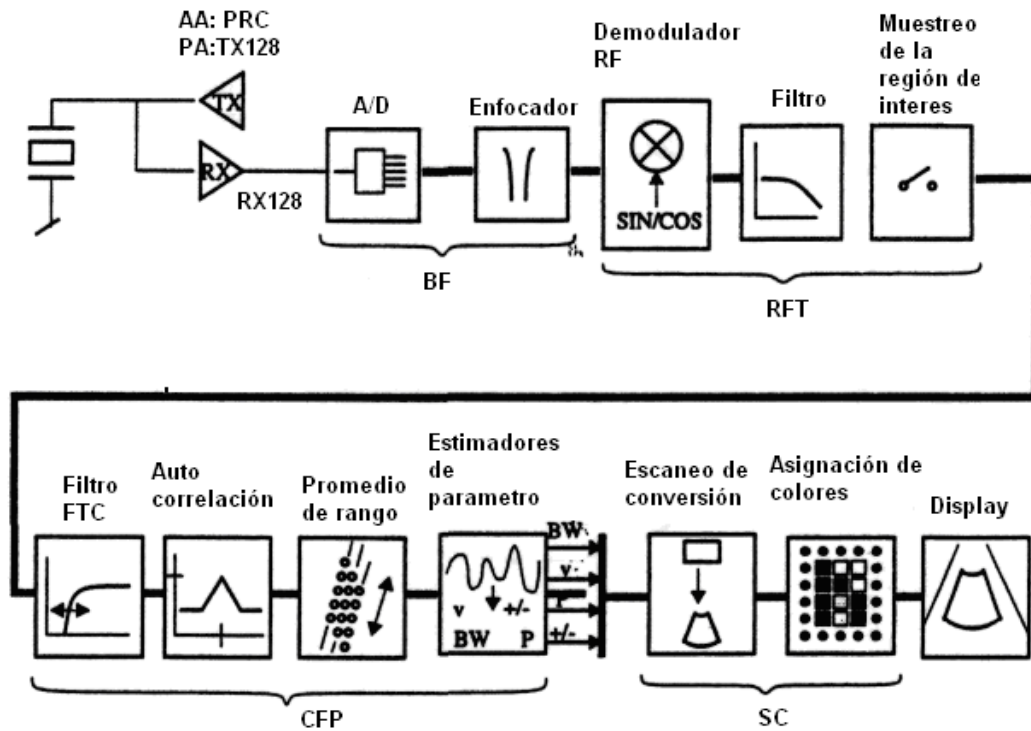
Figura 2.43 Flujo de datos 2D
