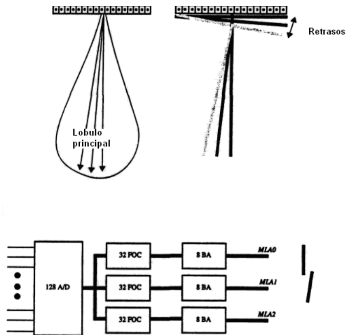
Figura 2.14 Multi Línea de Adquisición (MLA).
