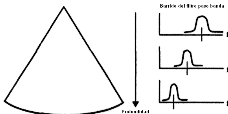
Figura 2.34 Barrido de filtro
