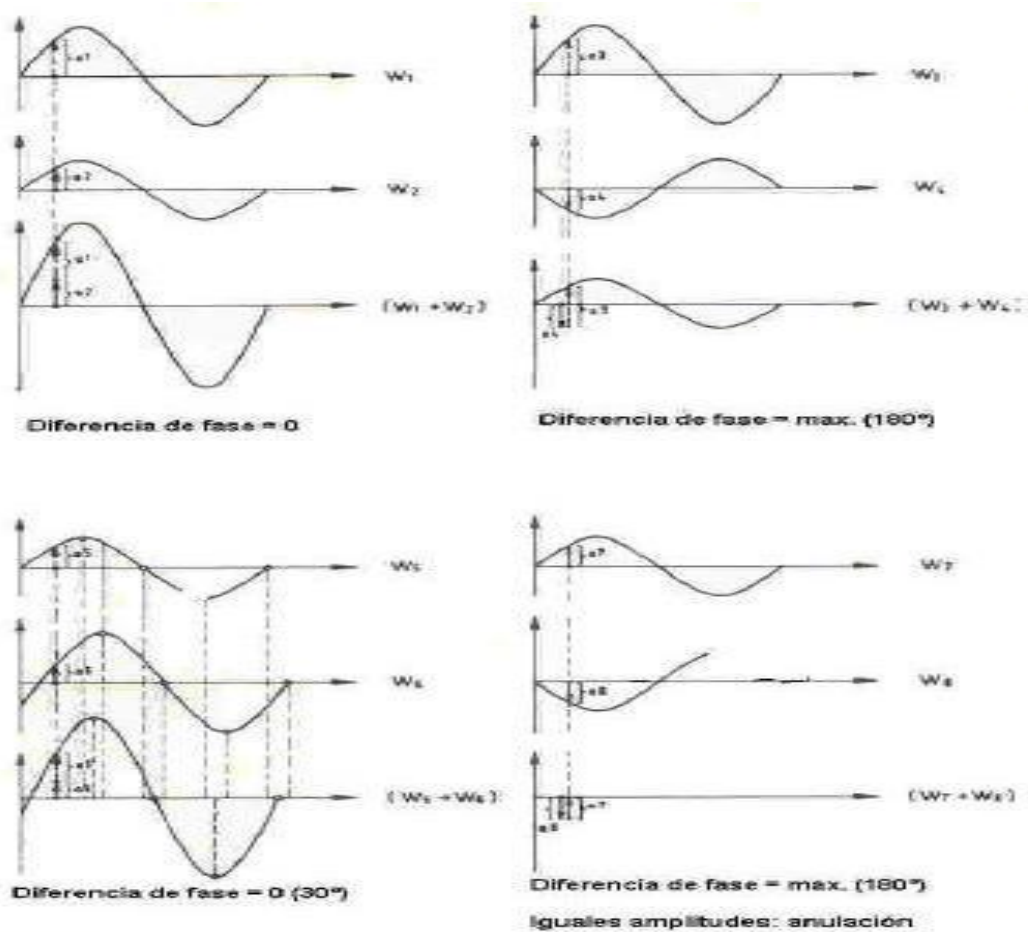
Figura 1.9 Superposición de ondas
