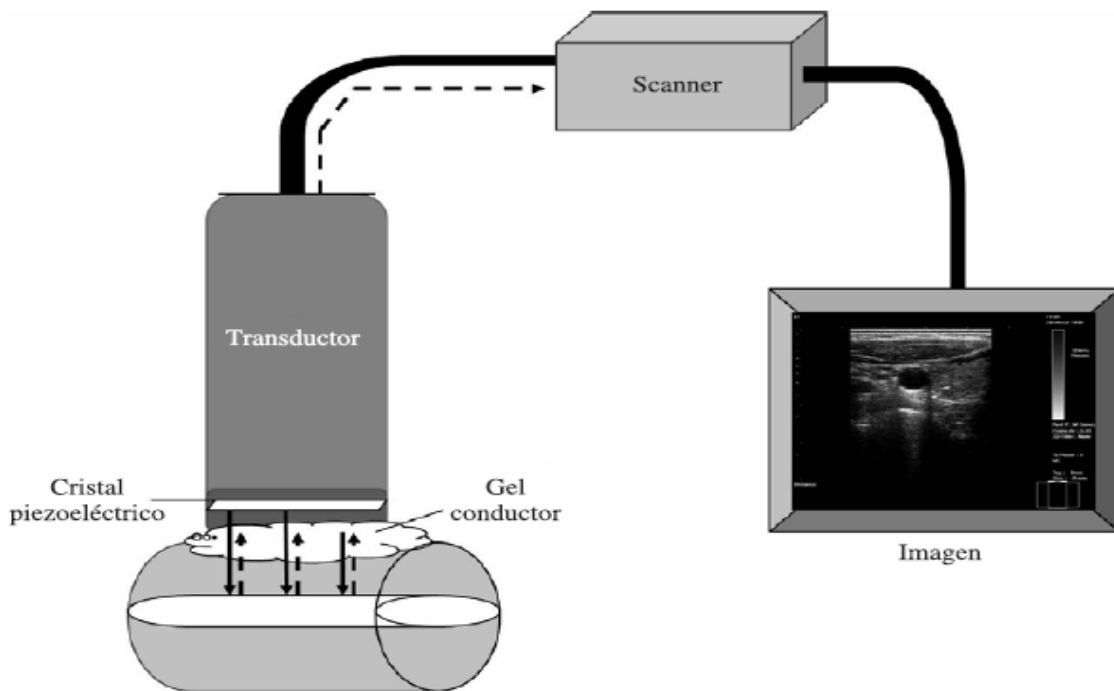
Figura 1.19 Sistema típico de escaneo por ultrasonido.
