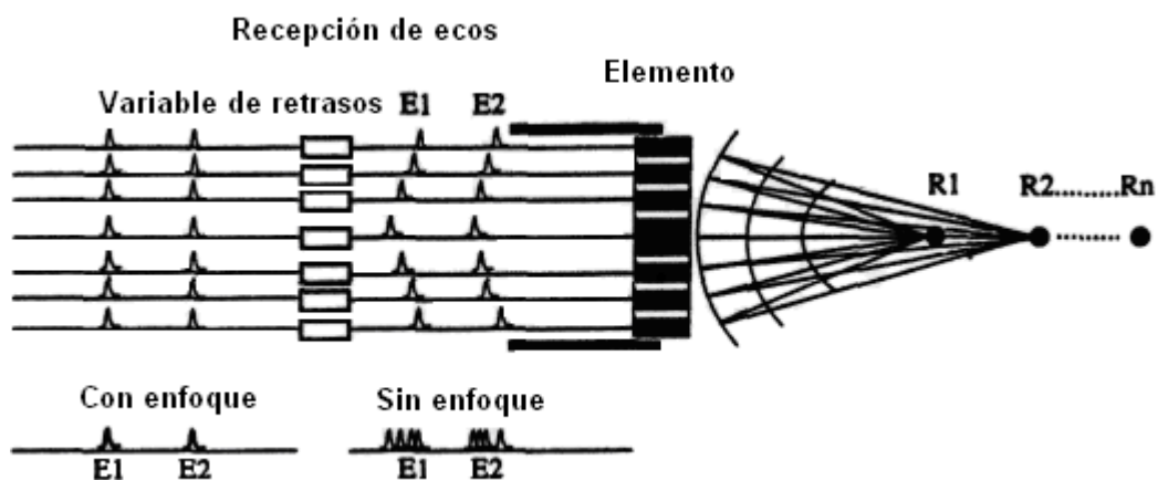
Figura 2.20 Enfoque de Recepción.
