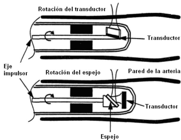
Figura 2.27 Tecnologías del Transductor
