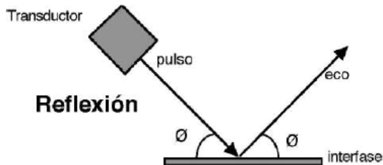
Figura 1.6 Reflexión en una interfase.
