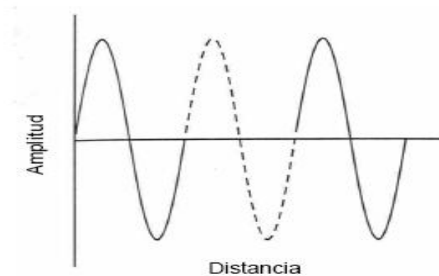
Figura 1.1 Ciclo Variación completa de una variable acústica.
