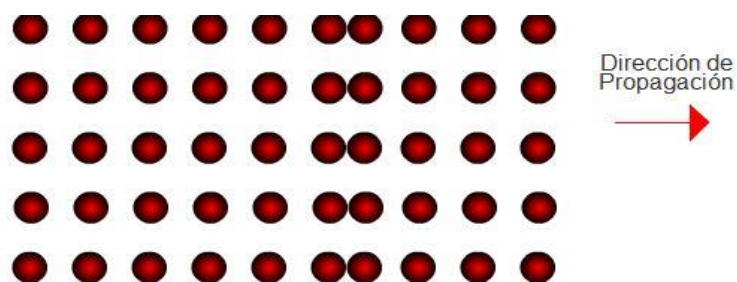
Figura 1.3 Propagación de ondas longitudinales
