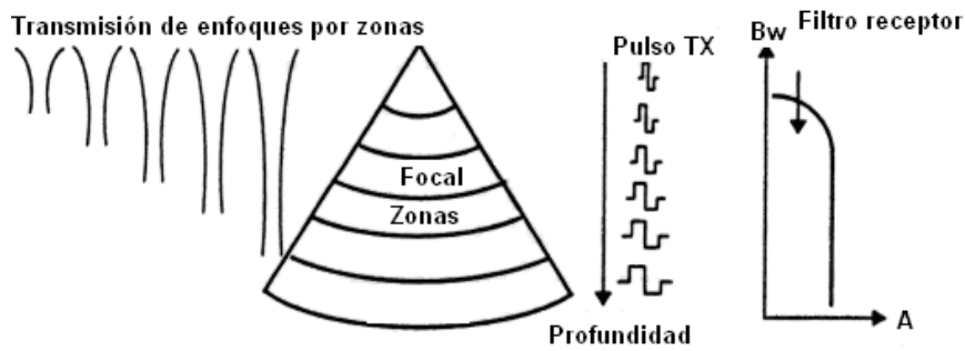
Figura 2.36 Composición del rayo.
