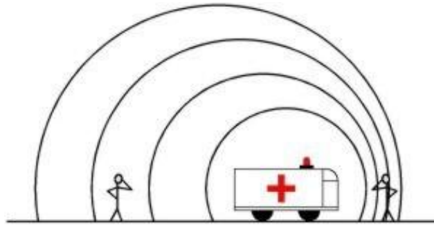
Figura 1.16 Efecto Doppler.
