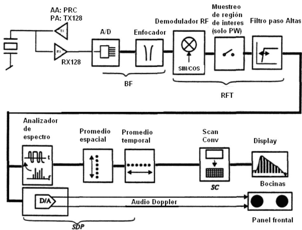
Figura 2.38 Flujo de datos Doppler
