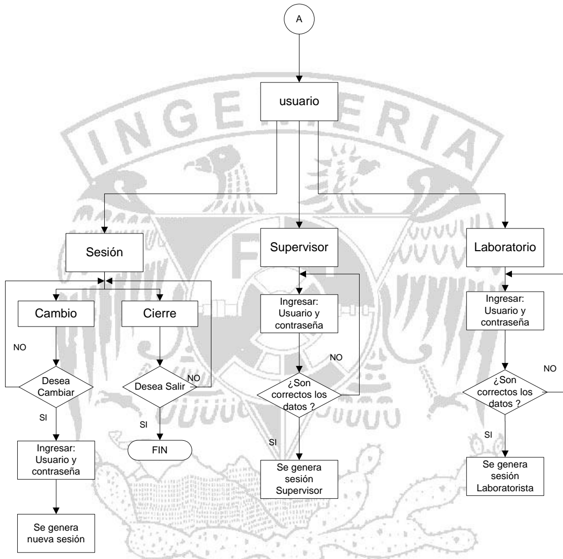
Figura 4.2.1.3 Diagrama de Flujo módulo usuario
