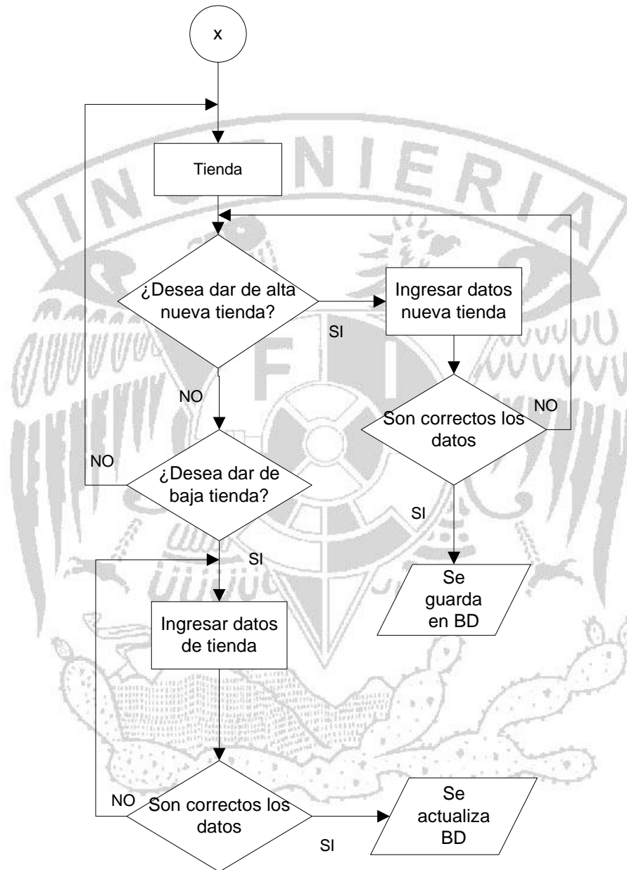
Figura 4.2.1.8 Diagrama de Flujo módulo Altas bajas
