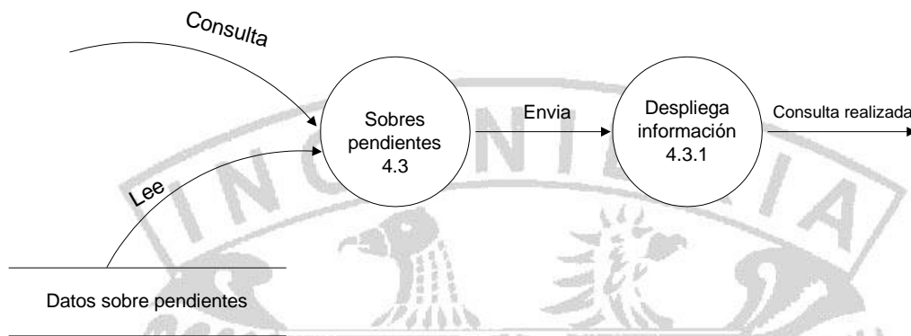
Figura 4.2.2.7 Diagrama de proceso sobres pendientes (nivel 3)
