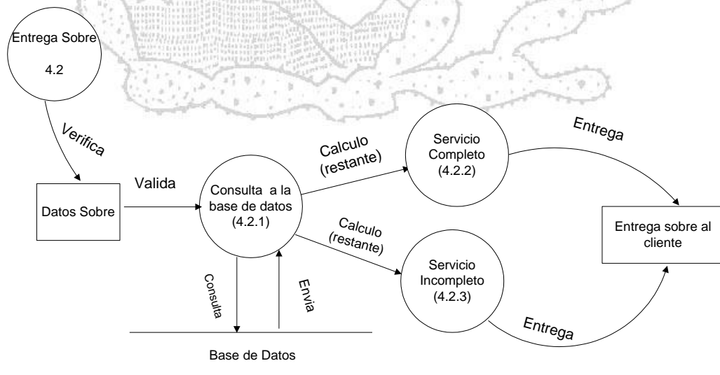
Figura 4.2.2.6 Diagrama de proceso entrega sobre (nivel 3)
