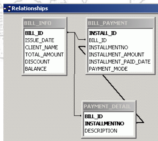
Figura 4.6.3 Relación entre tablas mostrado por Crystal Reports
