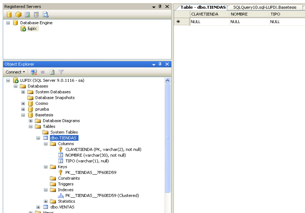
Figura. 4.3.6 Detalle Tabla TIENDAS.
