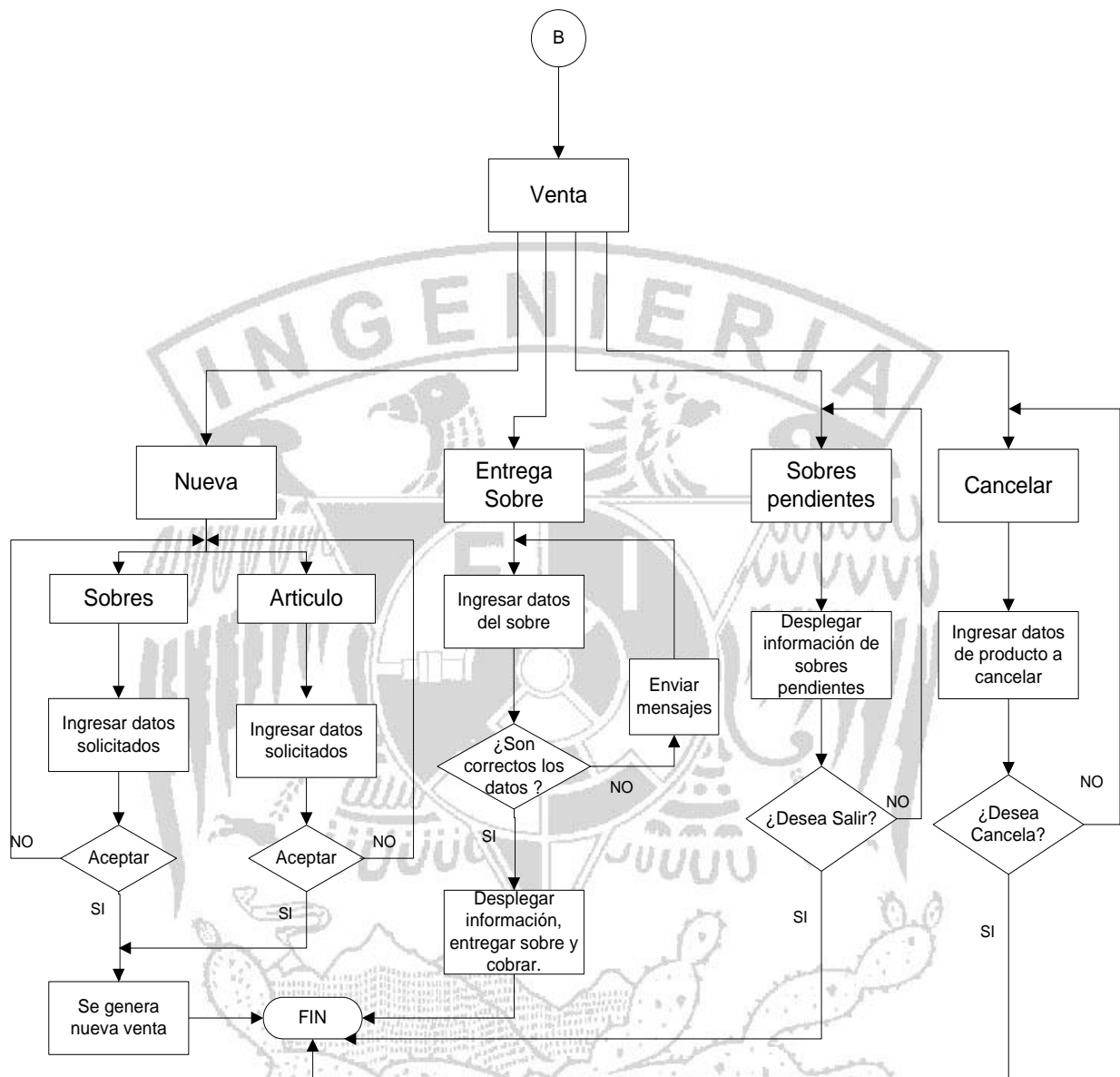
Figura 4.2.1.4 Diagrama de Flujo módulo venta
