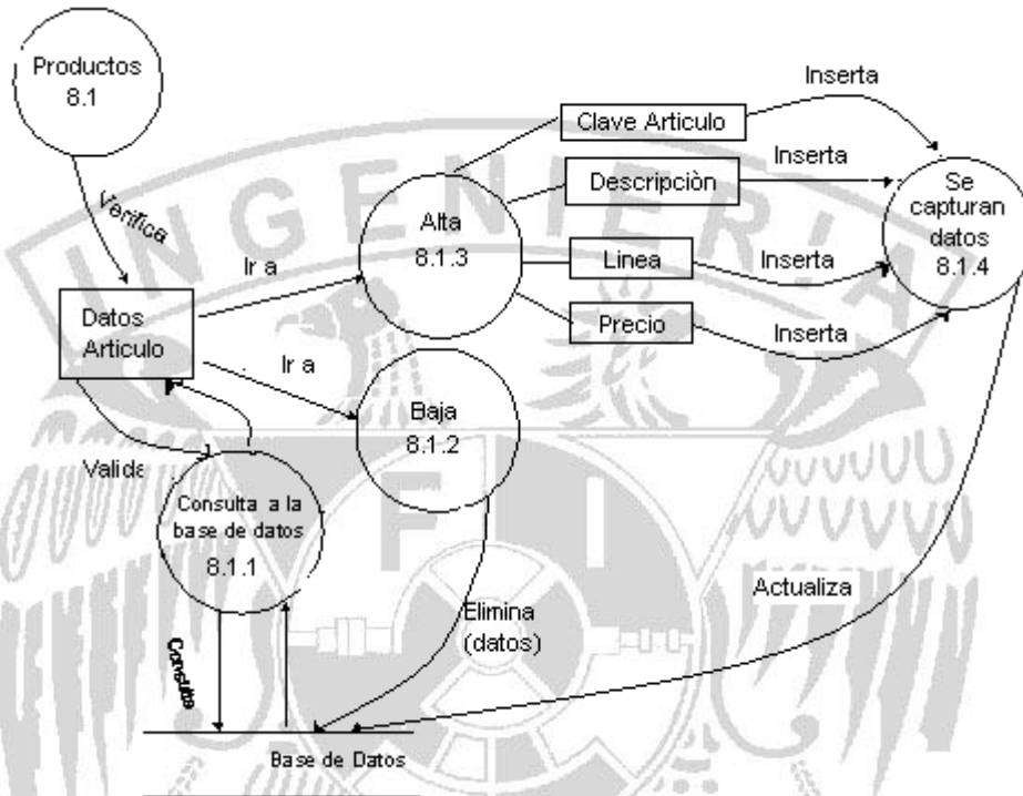
Figura 4.2.2.9 Diagrama de proceso Altas y Bajas de un Producto (nivel 3)
