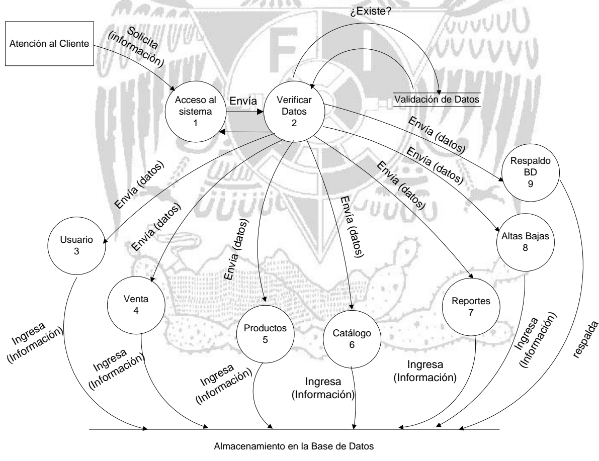
Figura 4.2.2.3 Diagrama de procesos general (Nivel 1)
