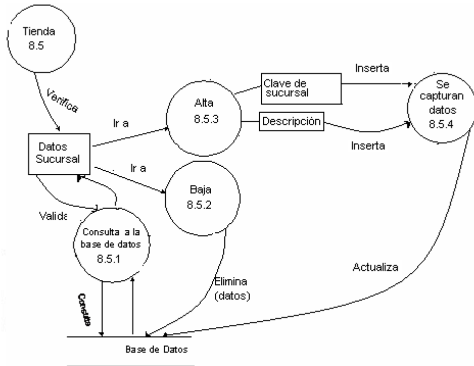
Figura 4.2.2.10 Diagrama de proceso Altas y Bajas de una Sucursal (nivel 3)
