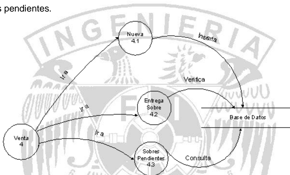
Figura 4.2.2.4 Diagrama de proceso venta (Nivel 2)
