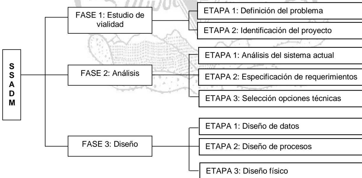
Figura 2.1.9 Fases y etapas de SSADM
