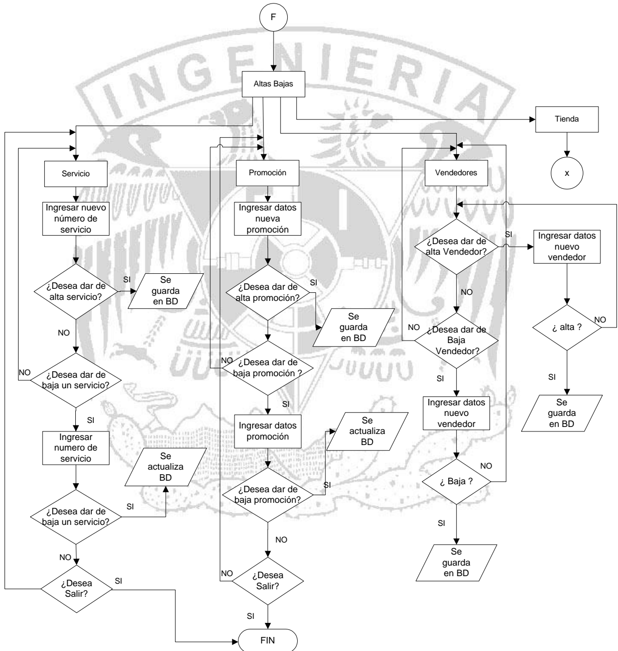
Figura 4.2.1.7 Diagrama de Flujo módulo Altas bajas
