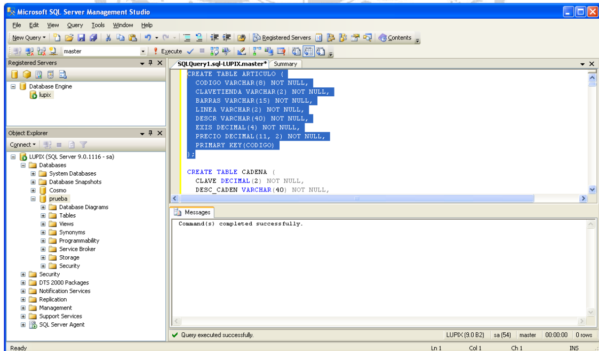
Figura. 4.3.7 Scripts de tablas
