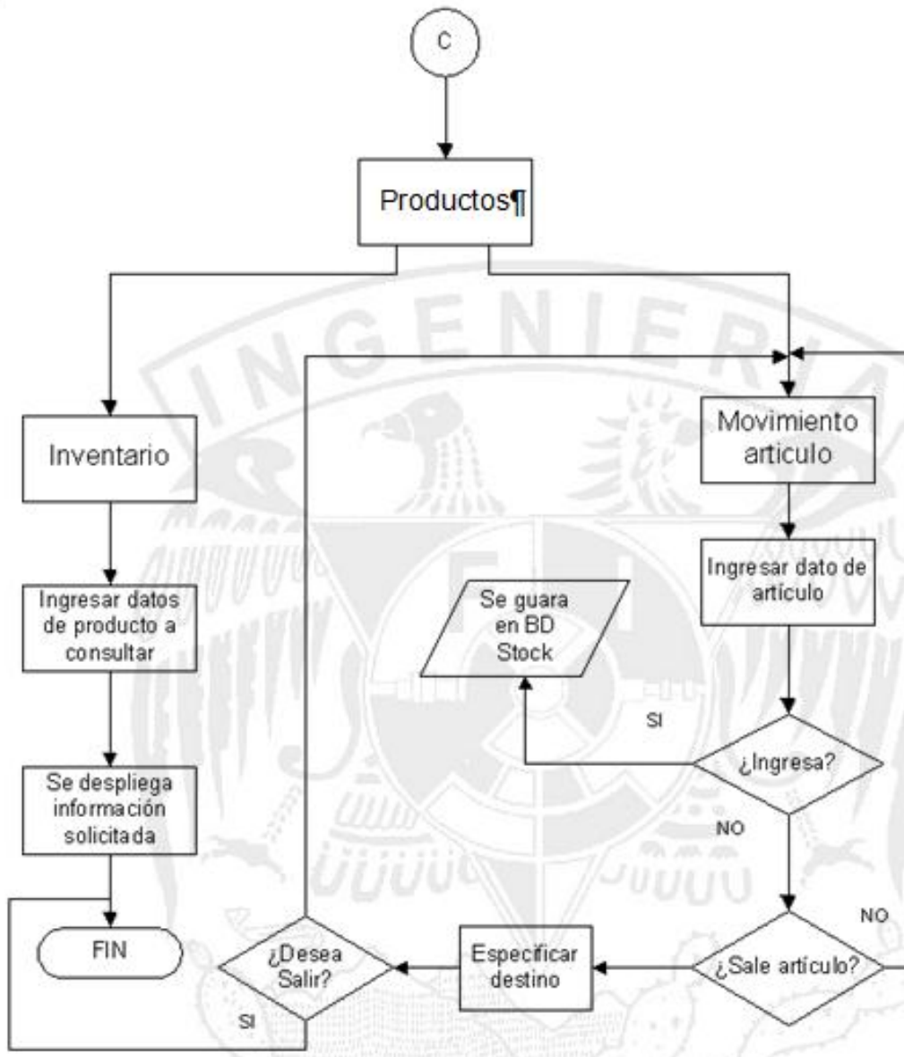
Figura 4.2.1.5 Diagrama de Flujo módulo productos
