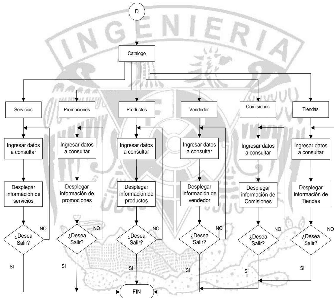
Figura 4.2.1.6 Diagrama de Flujo módulo catálogos
