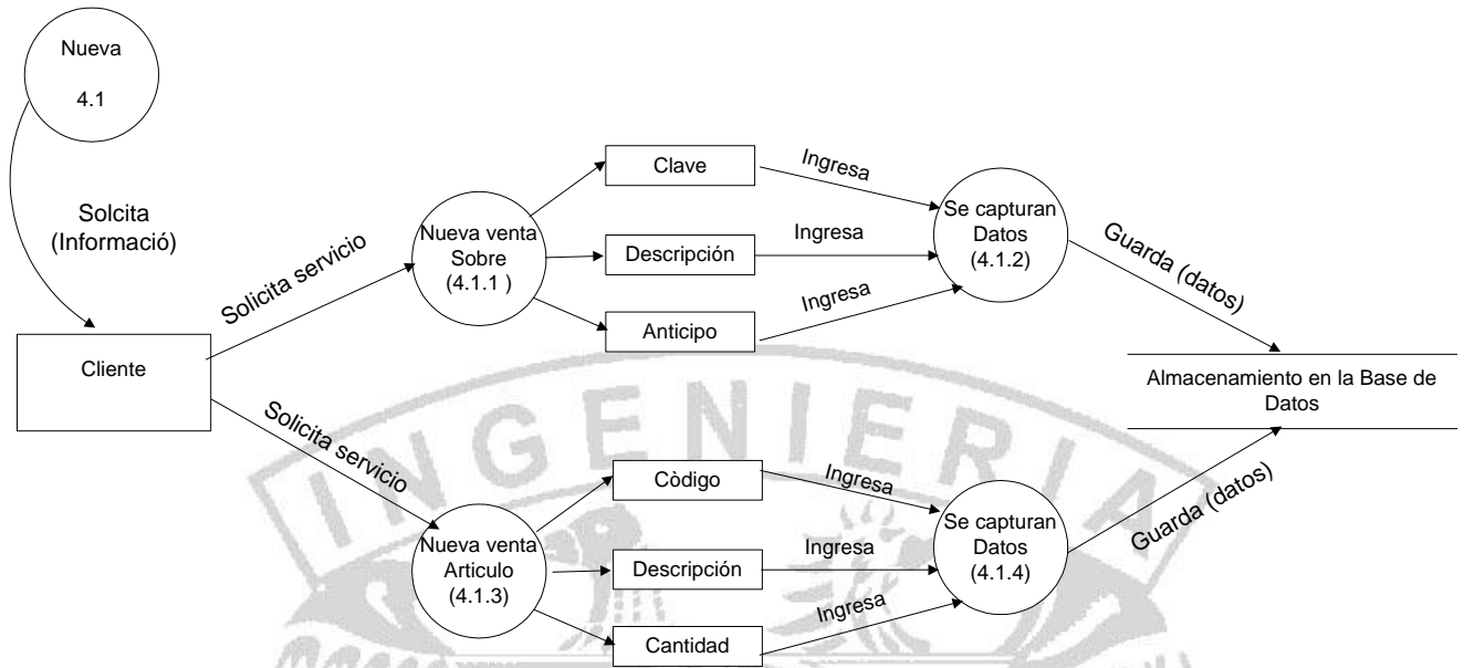
Figura 4.2.2.5 Diagrama de proceso venta (Nivel 3)
