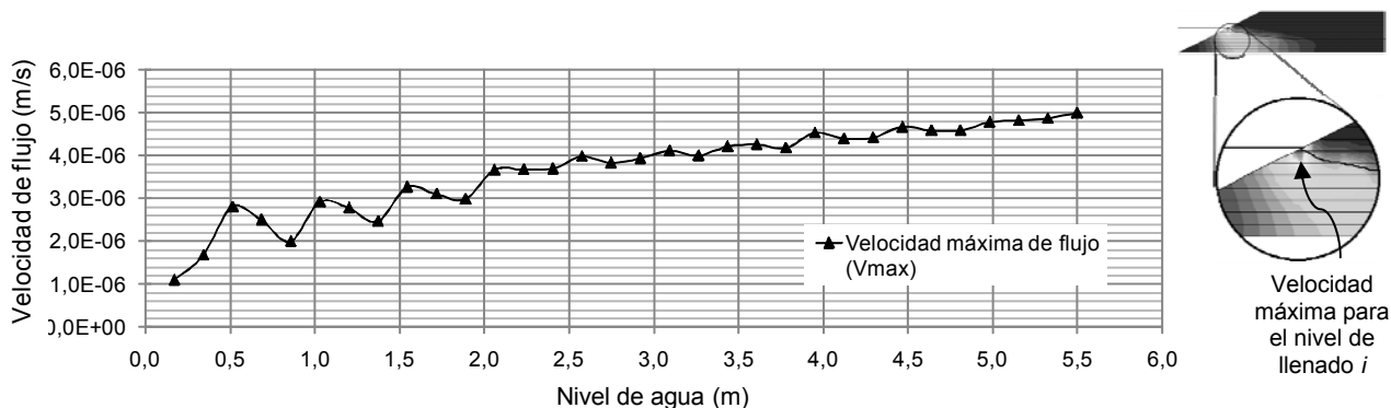
Figura 5.34 Variación de la magnitud de la velocidad máxima de flujo para diferentes tiempos de llenado.
