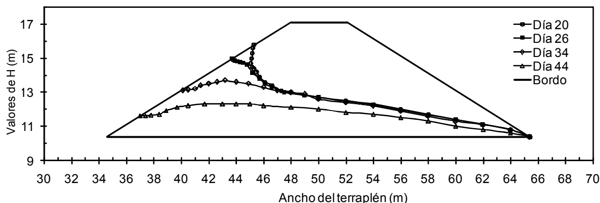
Figura 5.57 Líneas de saturación durante el llenado.
