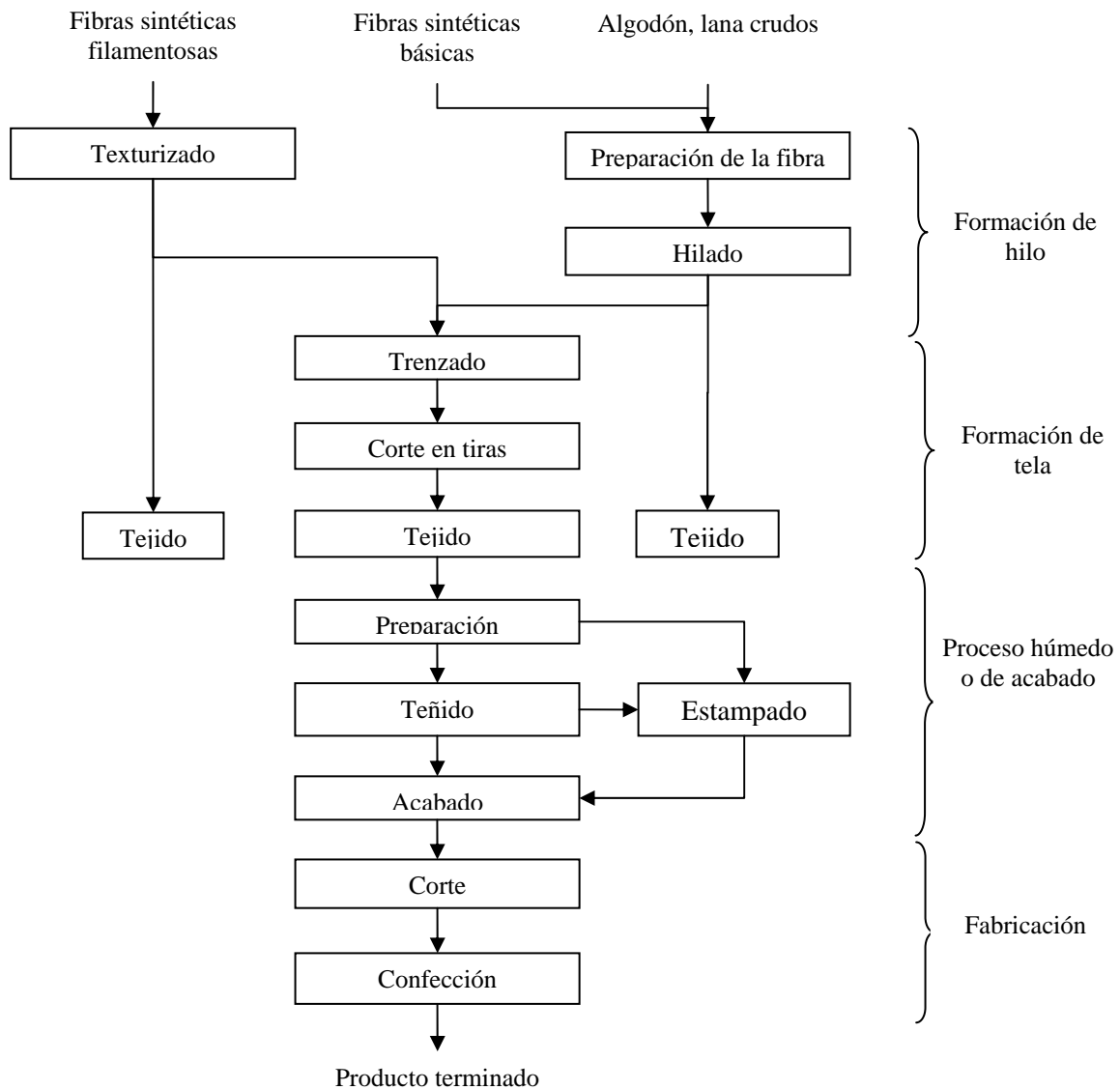
Figura 1.1. Diagrama de flujo de un proceso textil típico (EPA, 1997)
