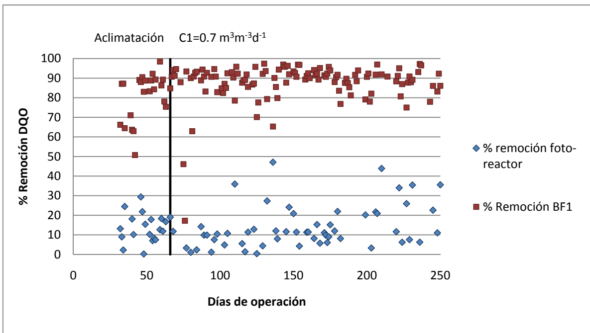
Figura 4.10. Porcentajes de remoción de materia orgánica (medida como DQO) del foto-reactor y BF1
