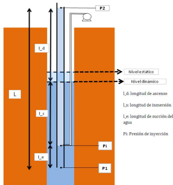
Figura 3.5 Dimensiones de un sistema air-lift [El autor]
