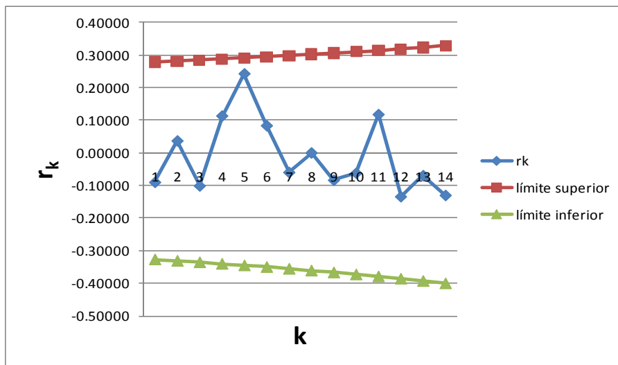
Figura 2.7. Gráfico del r_k y límites superior e inferior (Santa Cruz)
