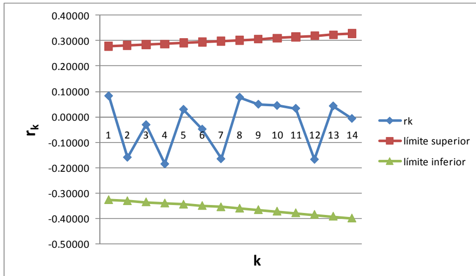
Figura 2.6. Gráfico del r k y límites superior e inferior (Jaina)
