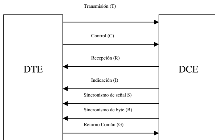
Circuitos de nivel físico de X.25
