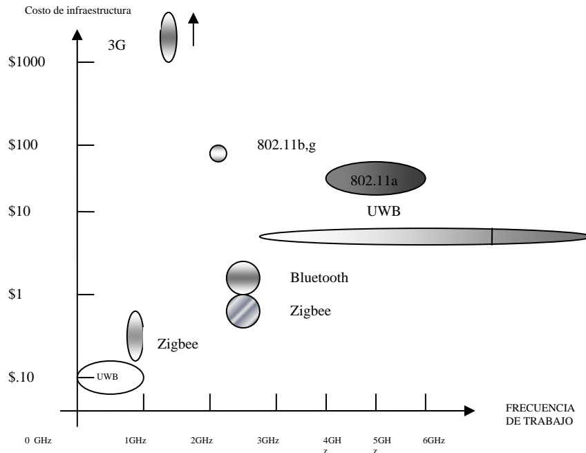
Figura 7 Costo de las tecnologías inalámbricas
