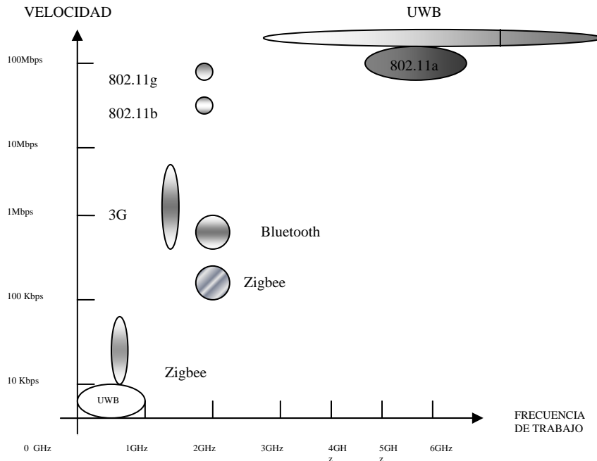
Figura 4 Velocidad de las tecnologías inalámbricas
