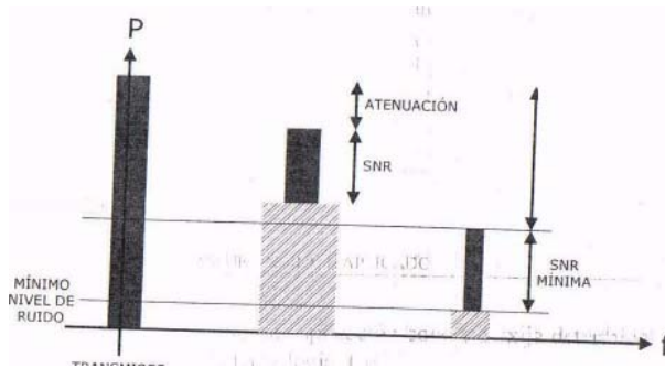
Figura 8. Relación entre los parámetros de cobertura.
