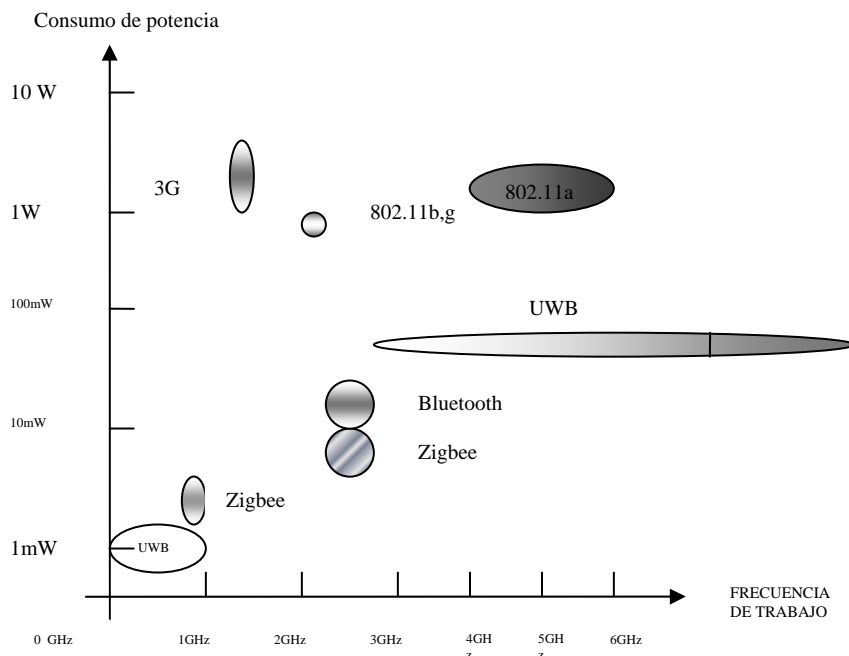
Figura 6 Consumo de Potencia de las tecnologías inalámbricas
