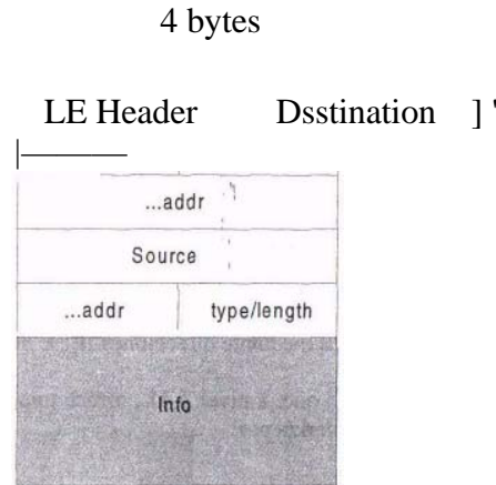
Formato de trama LANE
